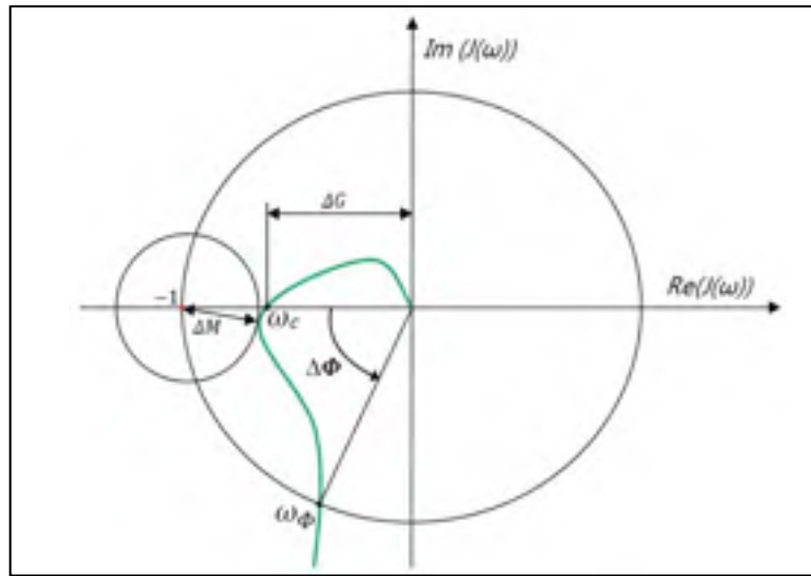
Figure 2.7 Diagramme de Nyquist de la boucle ouverte J(s) tracée en verte Tirée et reproduite de Retif (2008)
