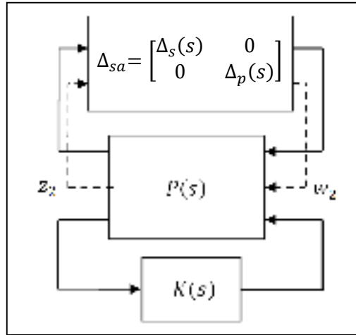
Figure 5.16 Boucle fermée perturbée pour robuste performance
