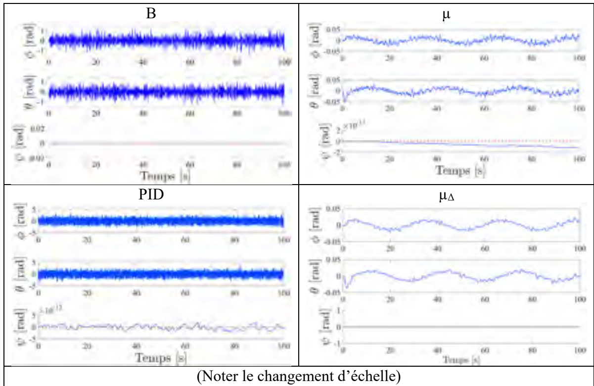
Figure 7.123 Déplacement des angles \phi , \theta , \psi lors d'une consigne hélicoïdale définie en (7.4), en présence de perturbation en sortie avec le processus non linéaire pour les compensateurs B, \mu , \mu_\Delta , PID
