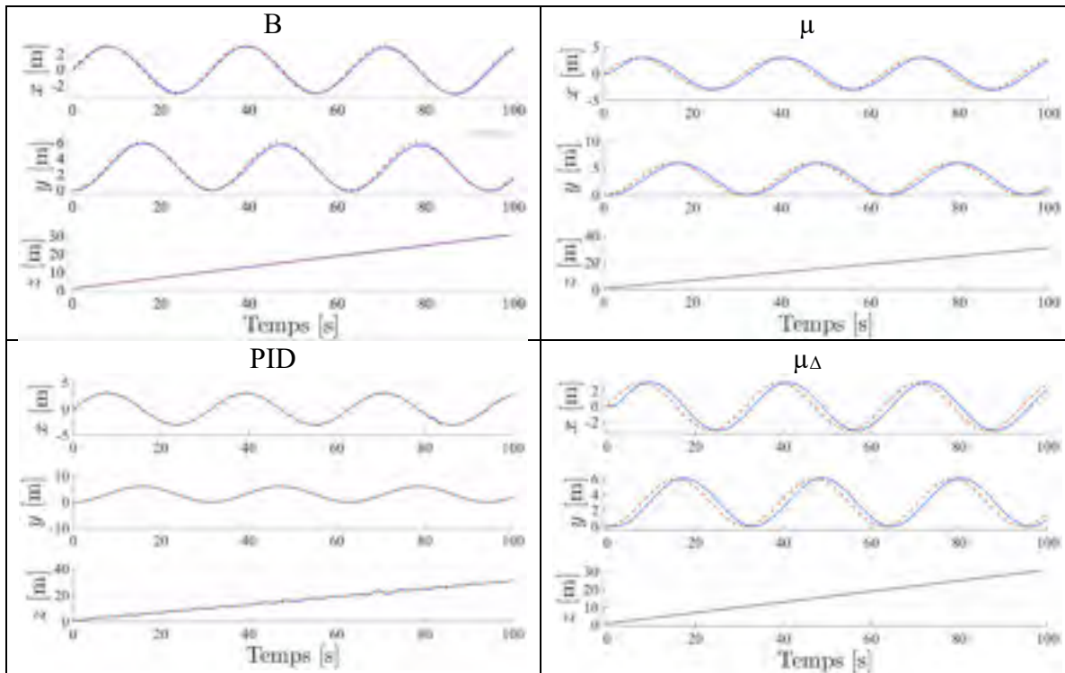
Figure 7.122 Déplacements sur les axes x, y, z lors d'une consigne hélicoïdale en pointillé rouge définie en (7.4), sur le processus non linéaire en présence de perturbation en sortie pour les compensateurs B, \mu , \mu_\Delta , PID
