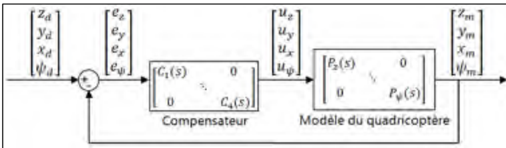
Figure 3.10 Boucle fermée avec le processus diagonal linéarisé pour une commande en translation et de rotation en cascade
