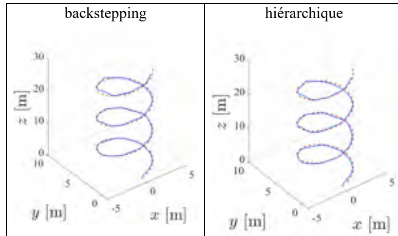
Figure 7.127 Déplacements en 3D sur x, y, z lors d'une consigne hélicoïdale en pointillé rouge définie en (7.4), avec perturbation en sortie pour les compensateurs backstepping et hiérarchique
