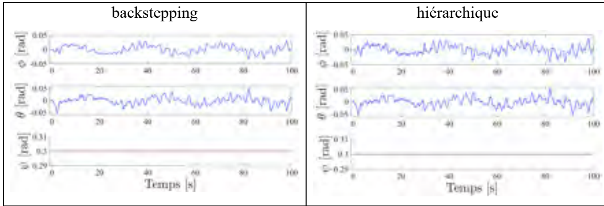
Figure 7.129 Déplacement des angles \phi , \theta , \psi lors d'une consigne hélicoïdale définie en (7.4), en présence de perturbation en sortie pour les compensateurs backstepping et hiérarchique
