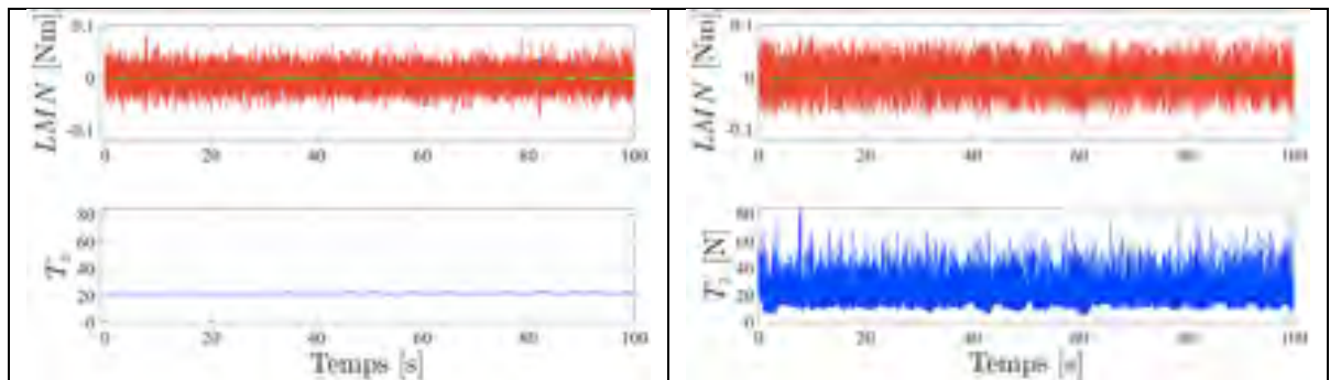
Figure 7.100 Commandes L , M , N , T_z lors d'un vol stationnaire en présence de perturbation en sortie pour les compensateurs backstepping et hiérarchique
