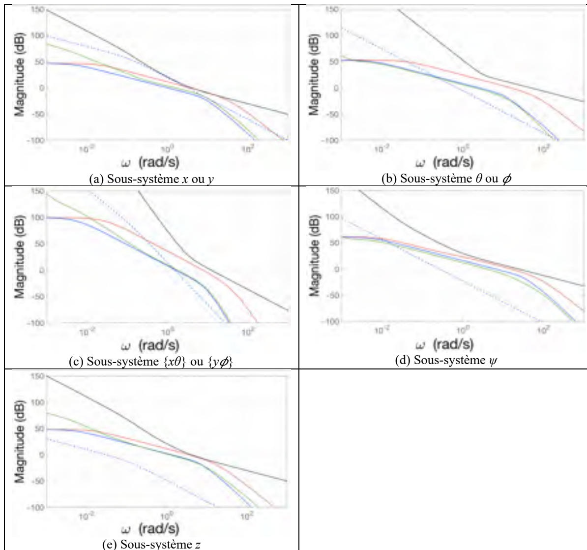
Figure 7.3 Diagramme de Bode de gain de la boucle ouverte J(s) sur les axes x ou y (a), \{x\theta\} ou \{y\phi\} (c), z (e) et autour des angles \theta ou \phi (b), \psi (d) pour le système seul (pointillés bleus) et avec compensateurs B (rouge), \mu (bleue), \mu_\Delta (verte) et PID (noire)
