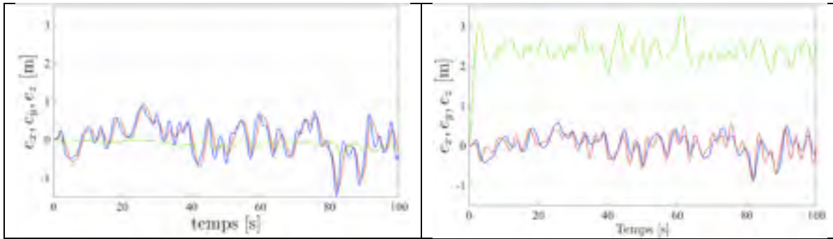
Figure 7.101 Erreurs e_x (rouge), e_y (bleue), e_z (verte) lors d'un vol stationnaire en présence de perturbation en sortie pour les compensateurs backstepping et hiérarchique
