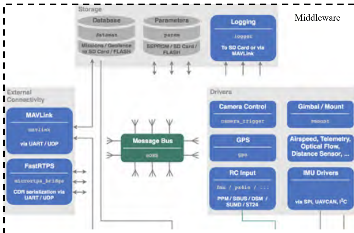
Figure 8.18 Architecture générale du logiciel embarqué PX4 12 (suite page suivante)
