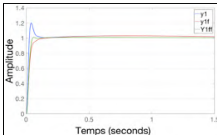
Figure 4.56 Réponse indicielle de y_1(t) , y_{1f}(t) et y_{1ff}(t)
