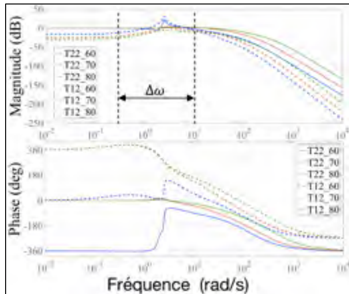
Figure 4.12 Bode des transmittances T_{22}(s) et T_{12}(s) pour trois valeurs du gain k_1
