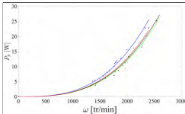
Figure 8.28 P_p en fonction de \omega , mesures pratiques en pointillés et fonctions approximées k\omega^3 en trait plein pour les moteurs : M 1 (vert), M 2 (noir), M 3 (bleu), M 4 (rouge)
