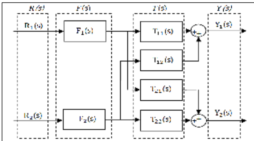
Figure 4.45 Schéma bloc du système multivariable avec préfiltres
