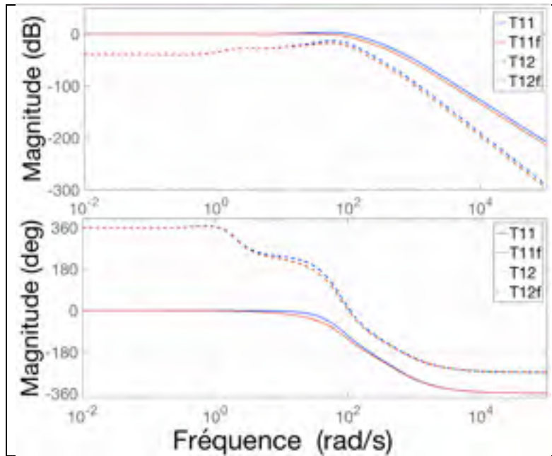
Figure 4.47 Bode de T_{11}(s) , T_{12}(s) , T_{11f}(s) , T_{12f}(s) dans le cas sans erreur statique
