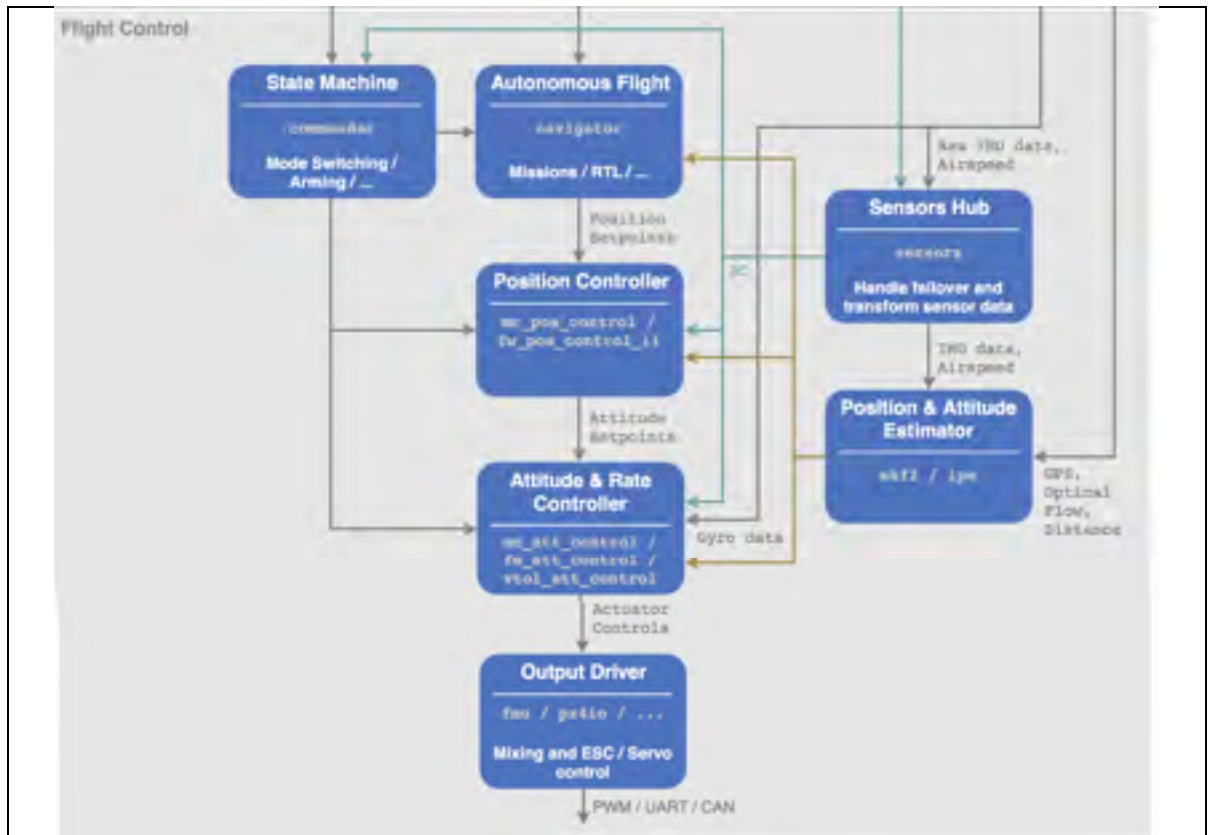
Figure 8.18 hitecture générale du logiciel embarqué PX4 (suite)
