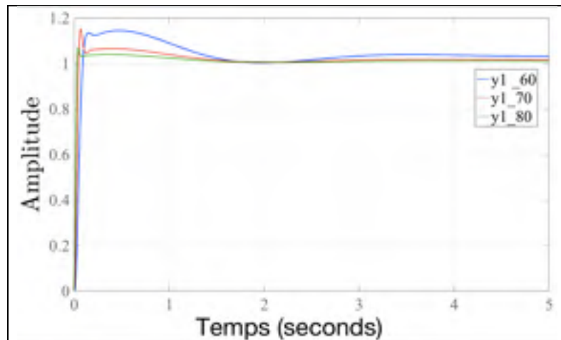
Figure 4.23 Allure de y_1(t) optimisé pour C_{max} = 60, 70 et 80 dB
