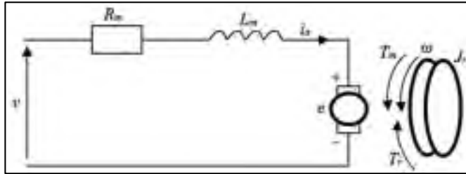
Figure 3.16 Diagramme d'un moteur DC
