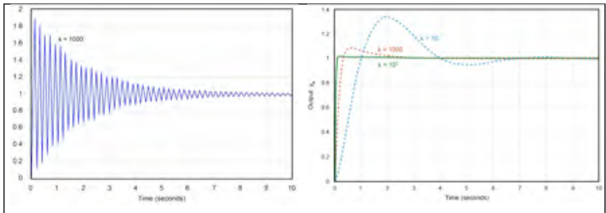
Figure 1.15 Comparaison des résultats obtenus pour une commande de déplacement en position entre une commande PID (à gauche) et la commande B (à droite) Tirée de Bensoussan (2015)
