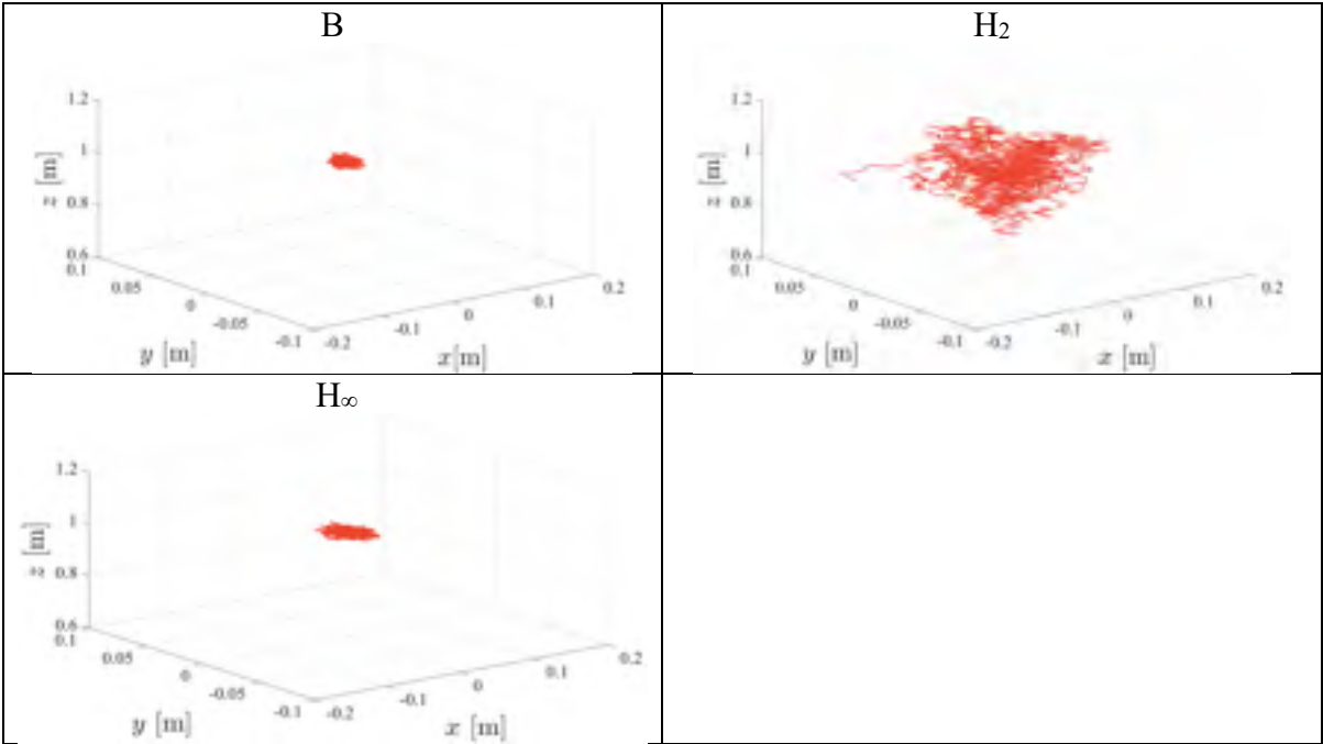
Figure 7.85 Variations des axes x, y, z lors d'un vol stationnaire en présence de perturbation sur la sortie pour les compensateurs B, H 2 , H ∞ appliqués sur le modèle non linéaire de drone
