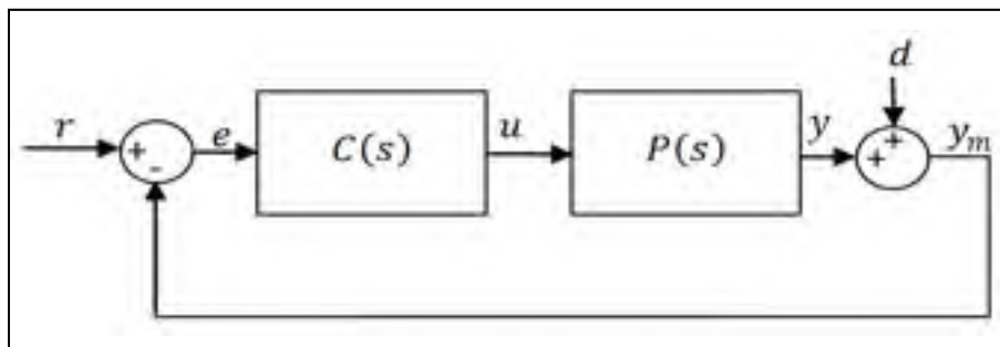
Figure 7.1 Schéma de la boucle de commande
