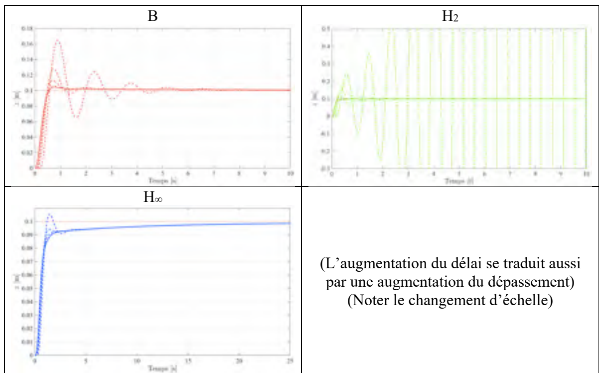
Figure 7.141 Réponses unitaires nominales en trait plein sur l'axe z et en pointillés avec l'ajout de délais de mesure, pour les compensateurs : B (rouge), H 2 (vert), H ∞ (bleu) pour le processus non linéaire
