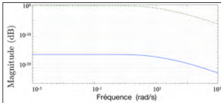
Figure 5.34 \mu_{\Delta_s} et \|\mathcal{F}_l(P(j\omega), K(j\omega))\|_{\infty} pour l'axe \psi avec incertitude
