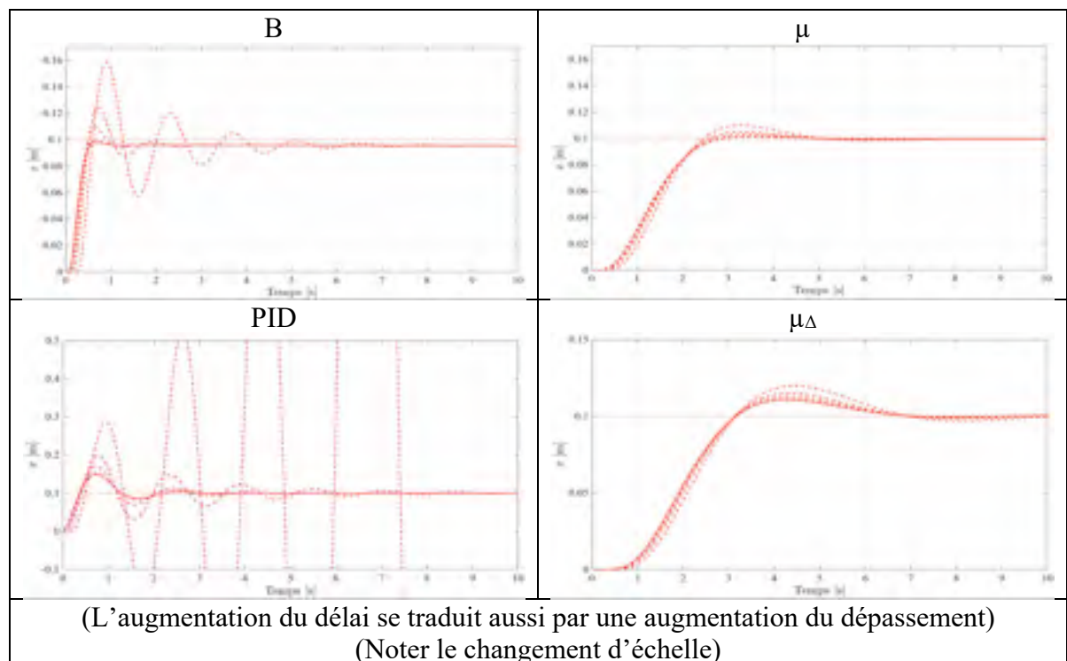
Figure 7.143 Réponses unitaires nominales (trait plein) sur les axes \{x\theta\} ou \{y\phi\} avec délais de mesure (trait en pointillé), pour les compensateurs : B, \mu , PID, \mu_\Delta (processus non linéaire)
