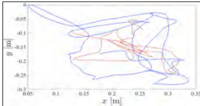
Figure 8.40 Mesures expérimentales avec le drone F450J des déplacements en 2D sur x, y lors d'un vol stationnaire pour les compensateurs : \text{PID}_{\phi} (bleu) ; B (rouge)
