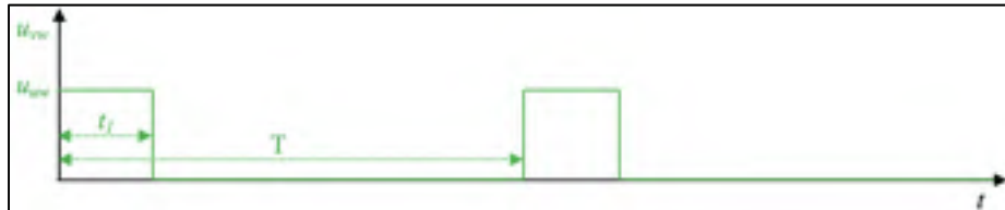
Figure 8.6 Exemple de signaux PWM
