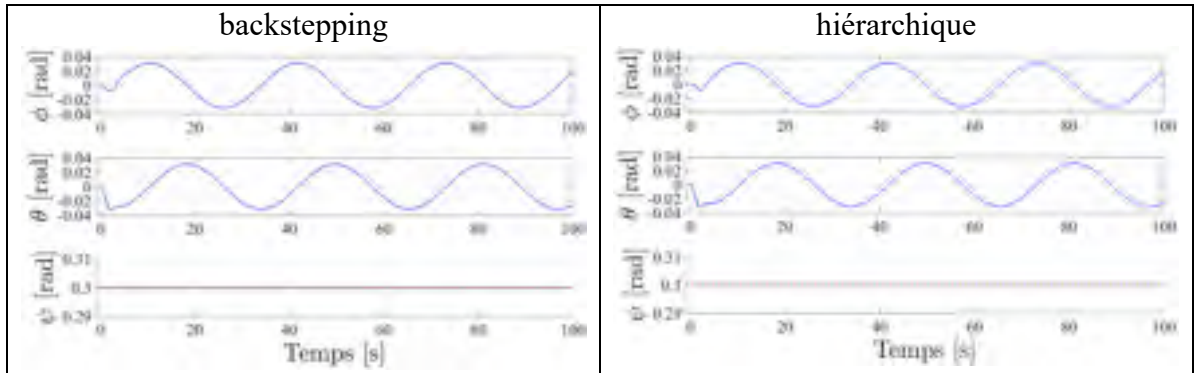
Figure 7.68 Déplacement des angles \phi , \theta , \psi lors d'une consigne hélicoïdale définie en (7.4), pour les compensateurs backstepping et hiérarchique
