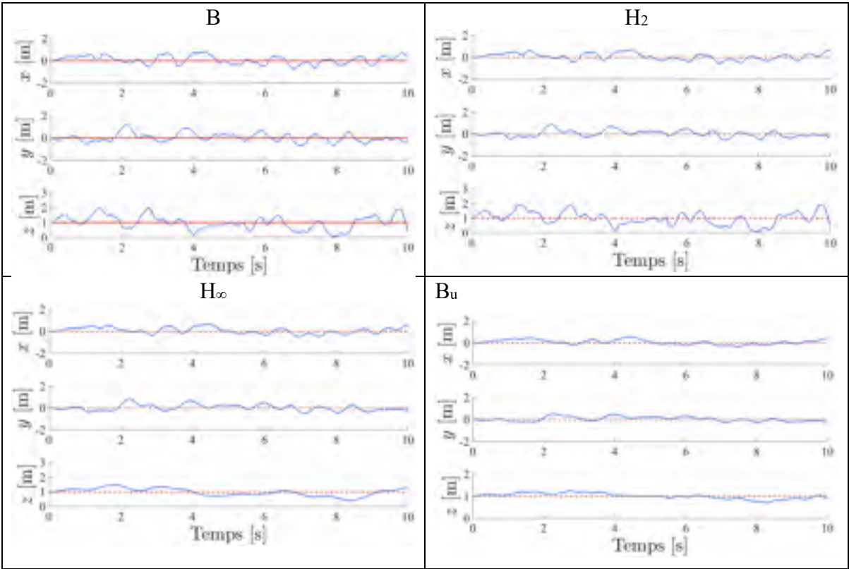
Figure 7.156 Déplacements sur les axes x, y, z lors d'un vol stationnaire en présence de perturbation en sortie pour les compensateurs B, H 2 , H ∞ , B u appliqués sur le modèle linéaire de drone
