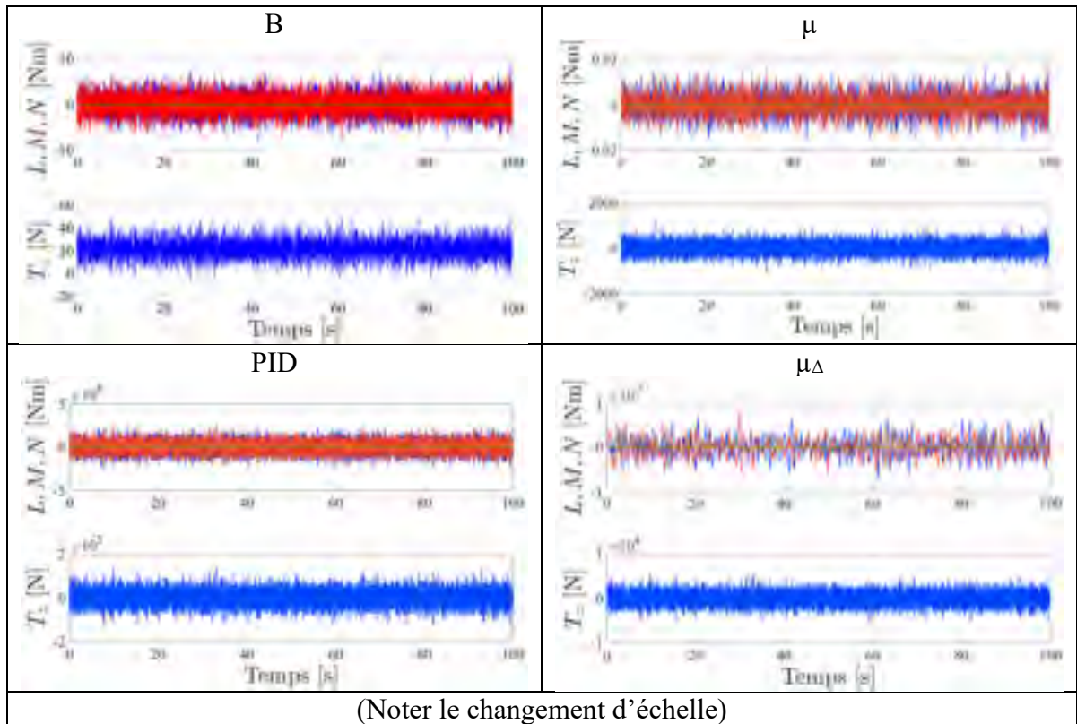
Figure 7.125 Commandes L (bleue), M (rouge), N (verte), T_z lors d'une consigne hélicoïdale définie en (7.4), présence de perturbation en sortie avec le processus non linéaire pour les compensateurs B, \mu , \mu_\Delta , PID
