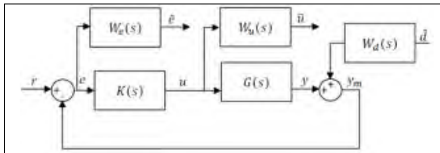
Figure 5.8 Boucle fermée avec ajout des fonctions de pondération
