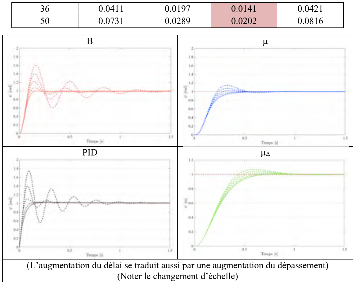
Figure 7.139 Réponses unitaires nominales en trait plein autour de l'angle \psi et en pointillés avec l'ajout de délais de mesure, pour les compensateurs : B (rouge), \mu (bleu), PID (noir), \mu_{\Delta} (vert) dans le cas d'un processus linéaire
