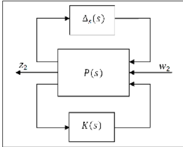
Figure 5.15 Boucle fermée sous forme standard avec perturbations structurées et perturbations exogènes
