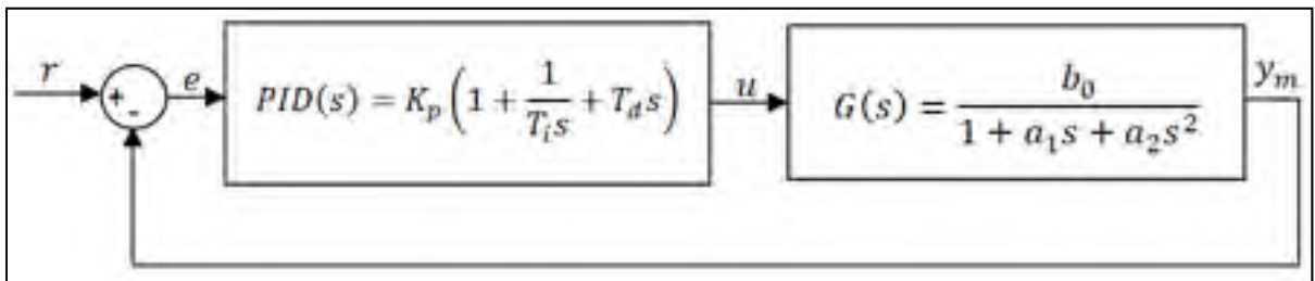
Figure 5.1 Boucle fermée d'un compensateur PID associé à un processus du second ordre
