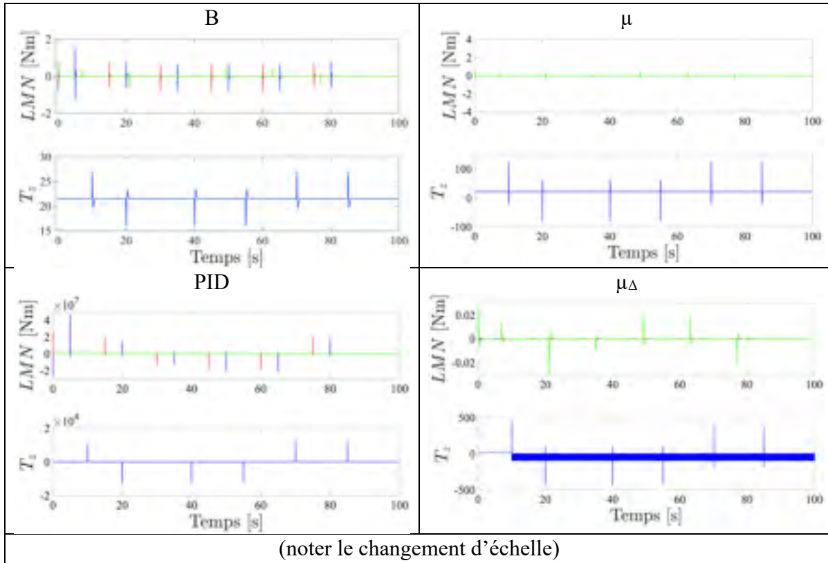
Figure 7.30 Réponses des commandes L , M , N et T_z pour le scénario de référence en pointillé rouge défini en (7.2), avec les compensateurs B , \mu , PID , \mu_\Delta sur le processus non linéaire
