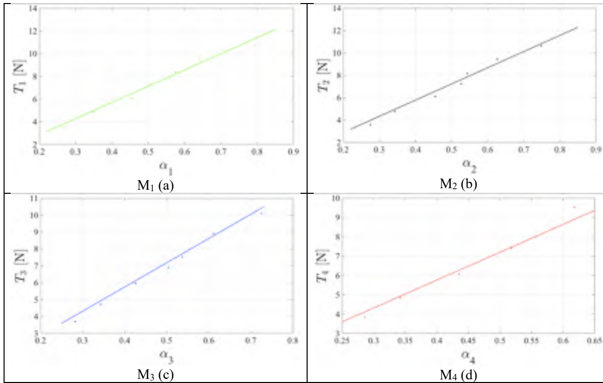
Figure 8.29 T en fonction de \alpha , mesures pratiques en pointiller et fonctions approximées k_i \alpha_i en trait plein pour les moteurs : M 1 (a), M 2 (b), M 3 (c), M 4 (d)
