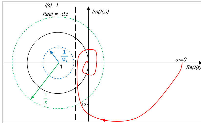
Figure 4.3 Diagramme de Nyquist de J(\omega) Tirée et reproduite de Retif (2008)
