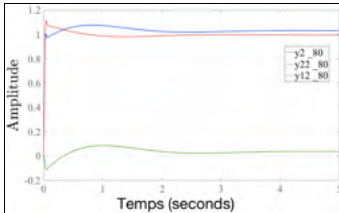
Figure 4.30 Allure de y_2(t) , y_{12}(t) et y_{22}(t) optimisées pour C_{max} = 80 dB
