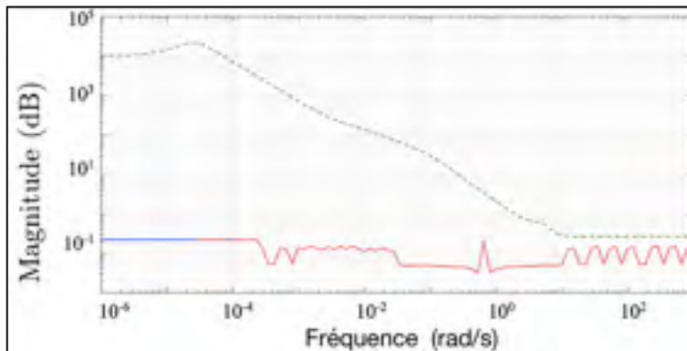
Figure 5.31 \mu_{\Delta s} et \|\mathcal{F}_l(P(j\omega), K(j\omega))\|_{\infty} pour l'axe x - y avec incertitude
