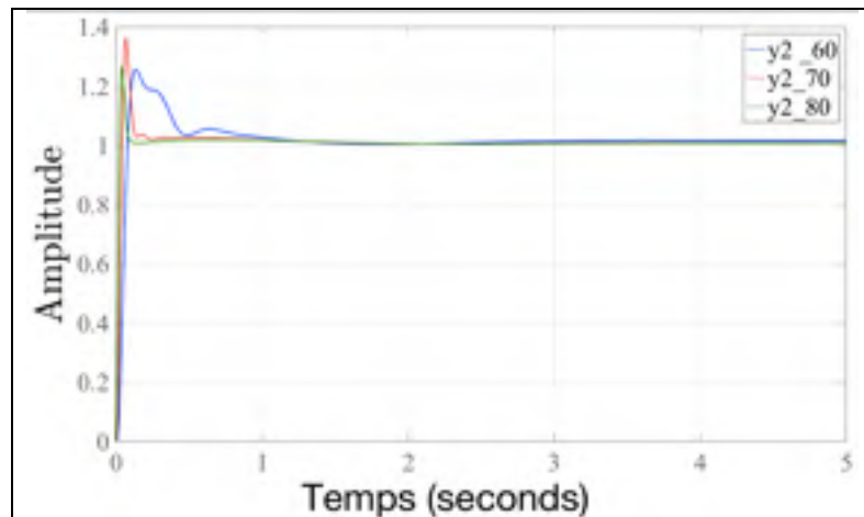
Figure 4.38 Réponse temporelle de y_2(t) pour C_{max} = \{60, 70, 80\} dB, dans le cas sans erreur statique
