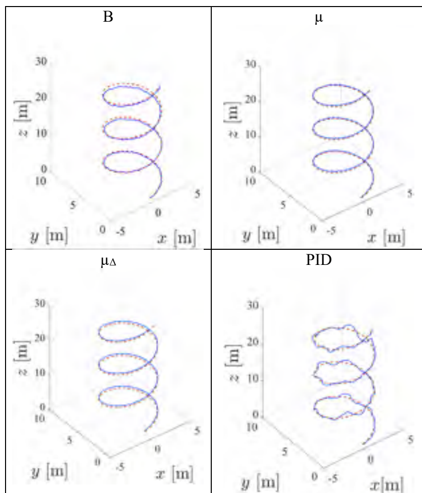
Figure 7.121 Déplacements en 3D sur les axes x , y , z lors d'une consigne hélicoïdale en pointillé rouge définie en (7.4), en présence de perturbation en sortie avec le processus non linéaire pour les compensateurs B , \mu , \mu_{\Delta} , PID
