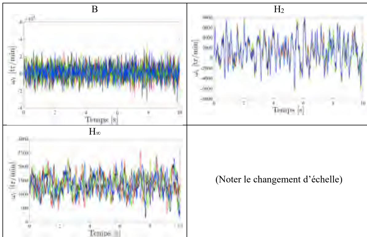
Figure 7.78 Vitesses \omega_1 (noire), \omega_2 (rouge), \omega_3 (verte), \omega_4 (bleue) lors d'un vol stationnaire en présence sur la sortie pour les compensateurs B, H 2 , H ∞ appliqués sur le modèle linéaire de drone
