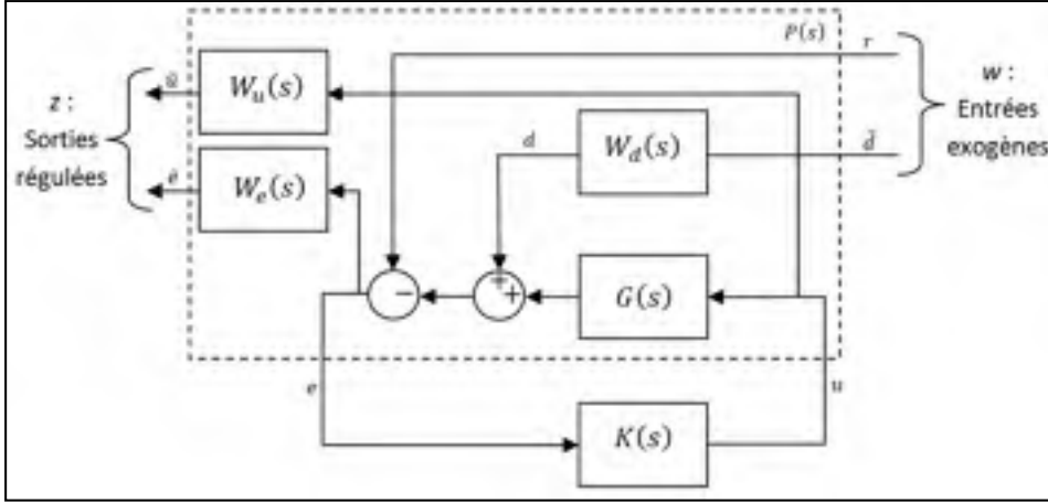
Figure 5.9 Boucle fermée sous forme standard
