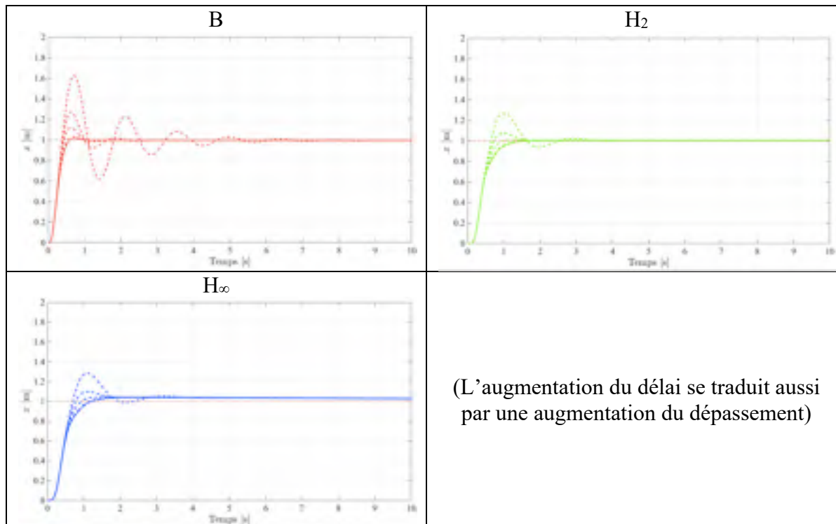
Figure 7.134 Réponses unitaires nominales en trait plein sur les axes \{x\theta\} ou \{y\phi\} et en pointillés avec l'ajout de délais de mesure, pour les compensateurs : B (rouge), H_2 (vert), H_\infty (bleu) pour un processus linéaire
