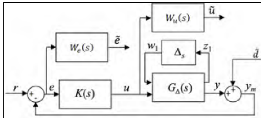
Figure 5.11 Boucle fermée avec ajout des fonctions de pondération et la matrice \Delta_s
