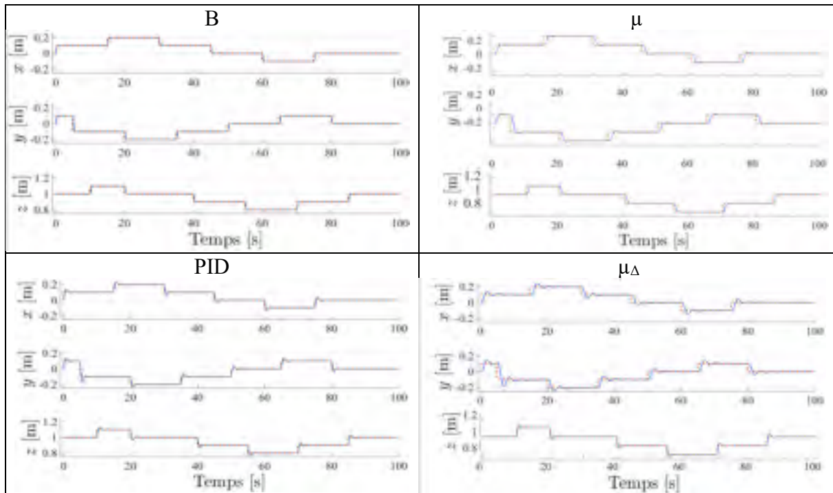
Figure 7.20 Réponses temporelles sur les axes x , y , z pour le scénario de référence en pointillé rouge défini en (7.2), avec les compensateurs B , \mu , PID, \mu_{\Delta} sur le processus linéaire
