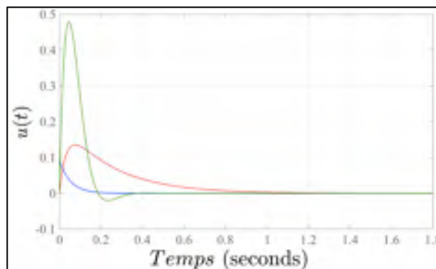
Figure 8.38 Réponse temporelle de la commande u(t) pour les compensateurs : \text{PID}_{\phi} (bleu) ; B (rouge) ; B amélioré (vert)
