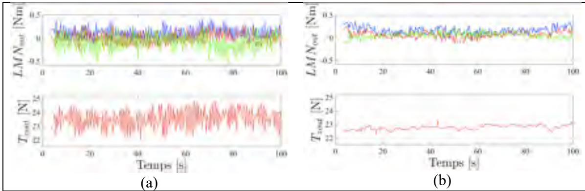
Figure 8.46 Mesures expérimentales avec le drone F450J en couples L, M, N et en poussée T_z venant du drone pour les compensateurs : \text{PID}_\phi (a) ; B (b)
