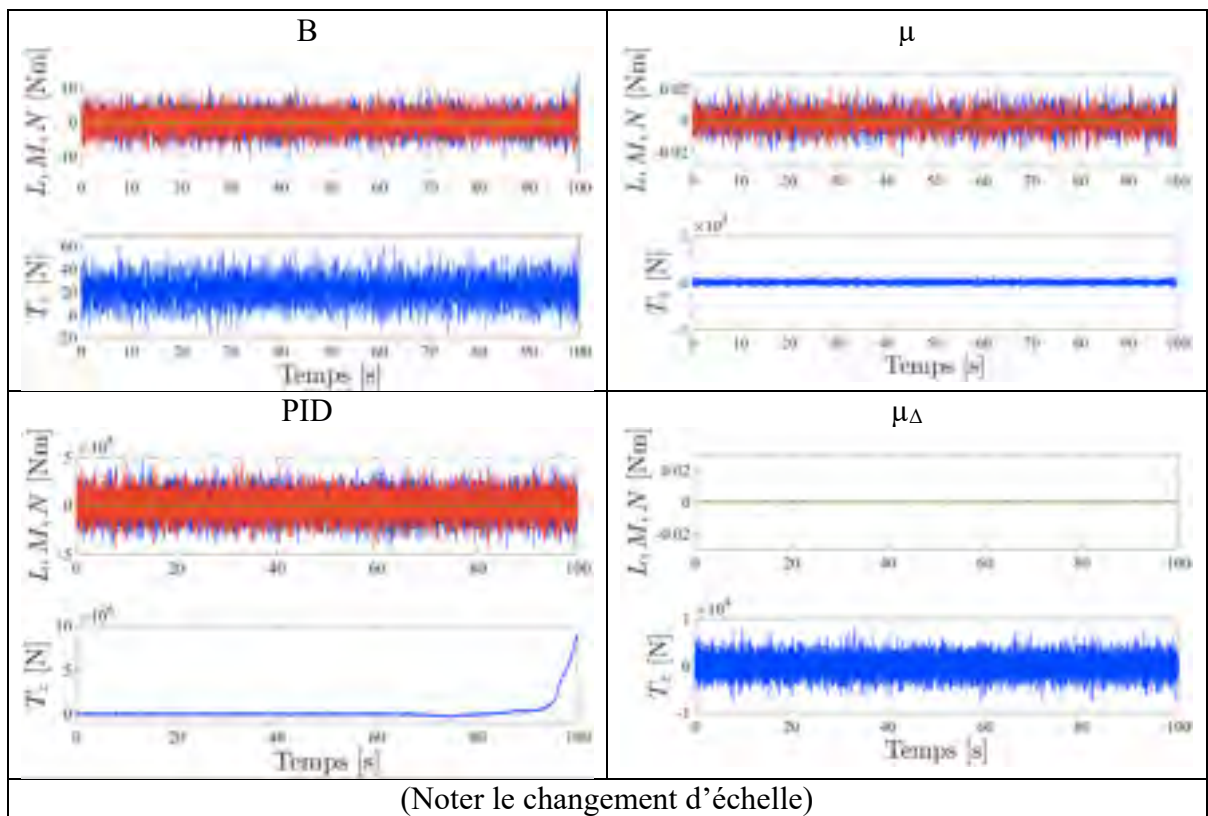
Figure 7.94 Commandes L , M , N , T_z lors d'un vol stationnaire en présence de perturbation en sortie pour les compensateurs B, \mu , \mu_\Delta , PID appliqués sur le modèle non linéaire de drone
