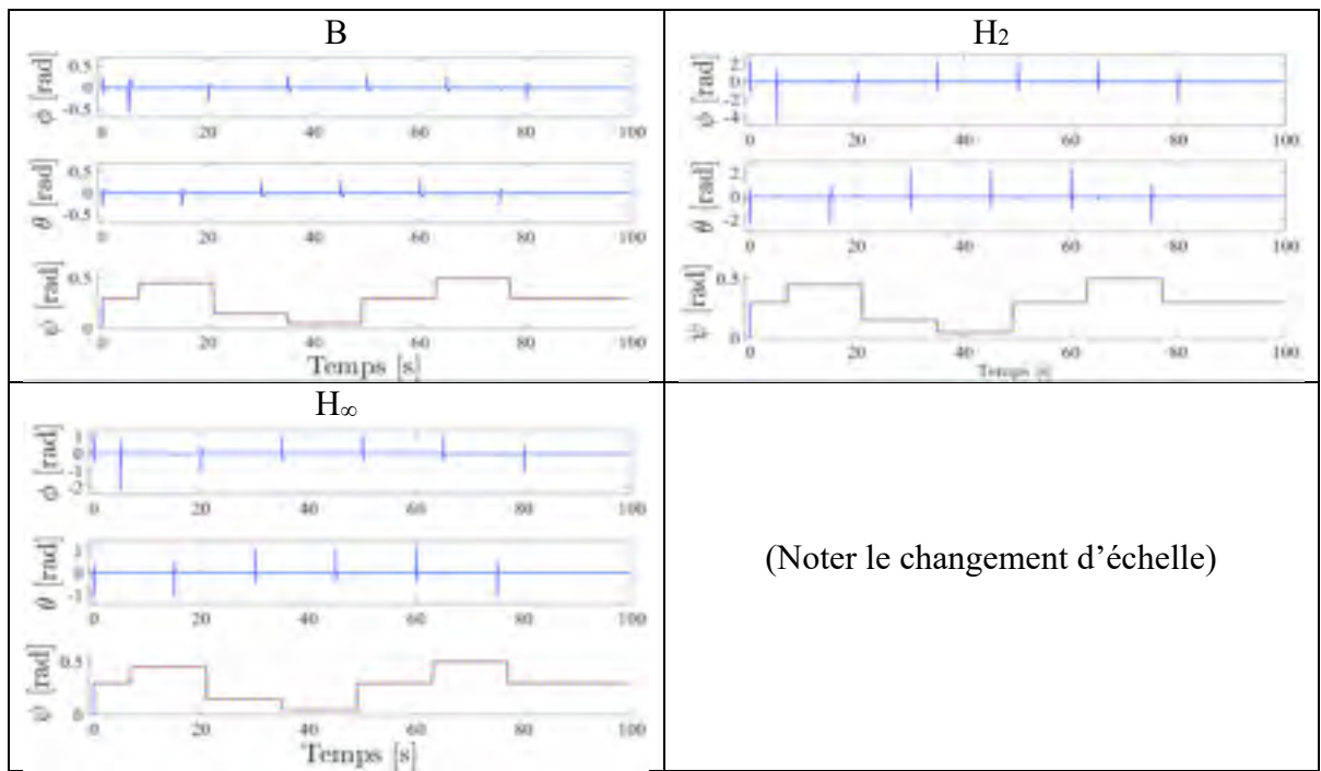
Figure 7.25 Réponses temporelles des angles \phi , \theta , \psi pour le scénario de référence en pointillé rouge (7.2), avec les compensateurs B, H_2 , H_\infty sur le processus non linéaire
