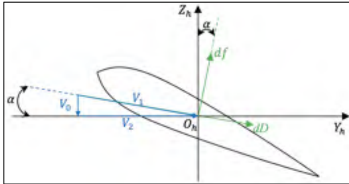
Figure 3.5 Représentation des forces appliquées sur un élément infiniment petit de l'hélice
