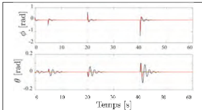
Figure 7.39 Réponses temporelles sur les angles \phi et \theta pour le scénario de référence y_d défini en (7.3), avec les compensateurs : B (rouge), \mu (bleu), \mu_\Delta (vert), PID (noir)
