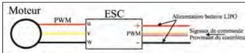
Figure 8.5 Connexion d'ESC à un moteur
