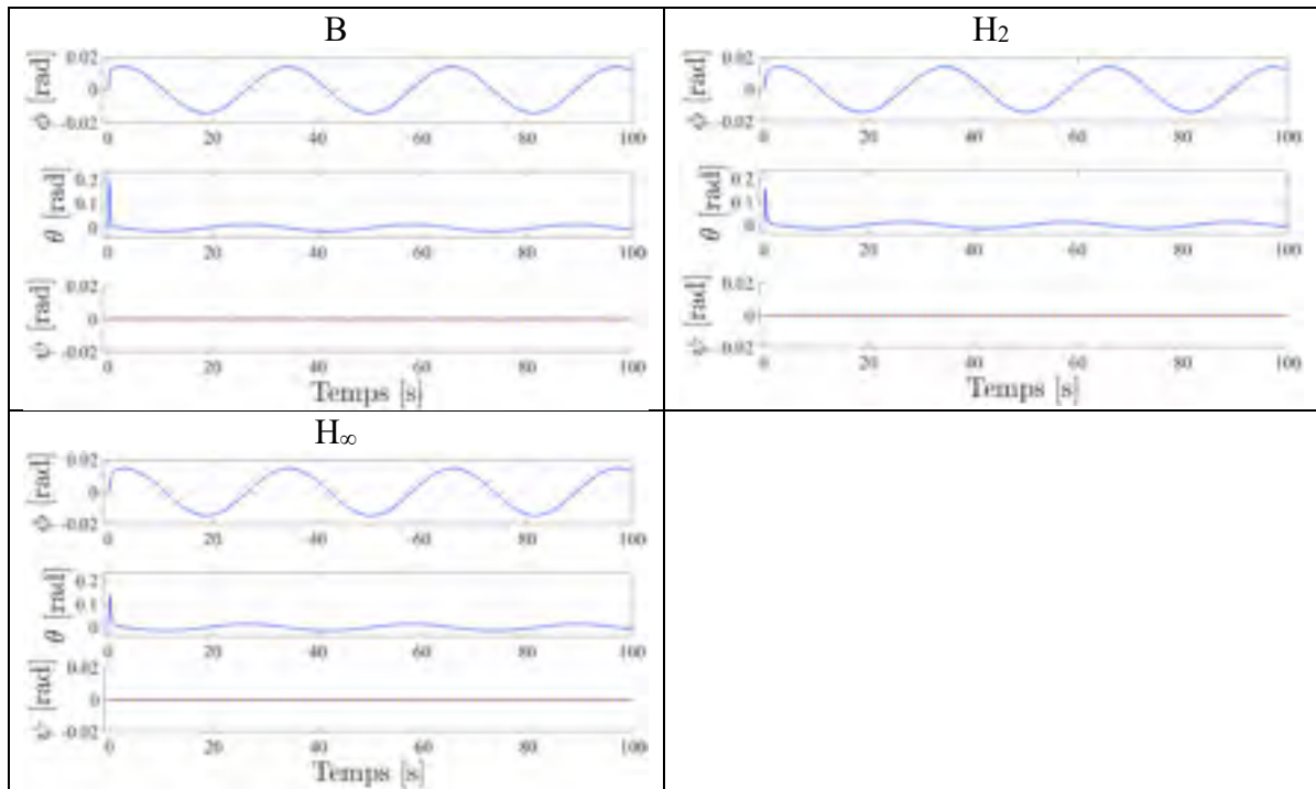
Figure 7.44 Déplacement des angles \phi , \theta , \psi lors d'une consigne hélicoïdale définie en (7.4), pour les compensateurs : B, H_2 , H_\infty
