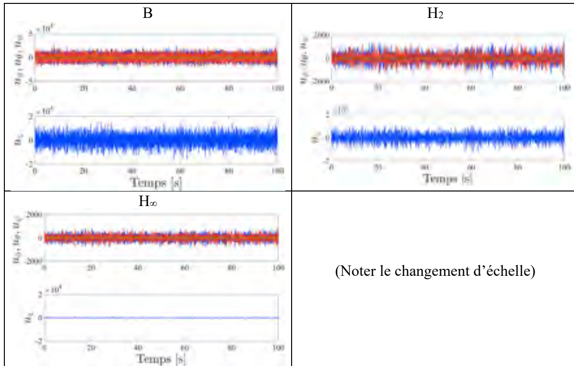
Figure 7.107 Commandes u_\phi (bleue), u_\theta (rouge), u_\psi (verte), u_z lors d'une consigne hélicoïdale en pointillé rouge et définie en (7.4), en présence de perturbation en sortie pour les compensateurs B, H_2 , H_\infty sur le processus linéaire
