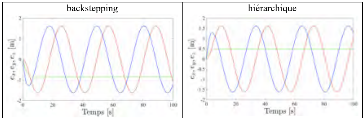
Figure 7.69 Erreurs e_x (bleue), e_y (rouge), e_z (verte) lors d'une consigne hélicoïdale définie en (7.4), pour les compensateurs backstepping et hiérarchique
