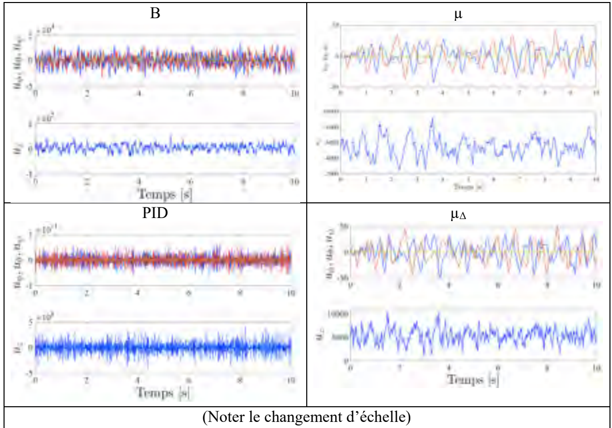
Figure 7.82 Commandes u_\phi (bleue), u_\theta (rouge), u_\psi (verte), u_z lors d'un vol stationnaire en présence de perturbation sur la sortie pour les compensateurs B, \mu , \mu_\Delta , PID appliqués sur le modèle linéaire de drone
