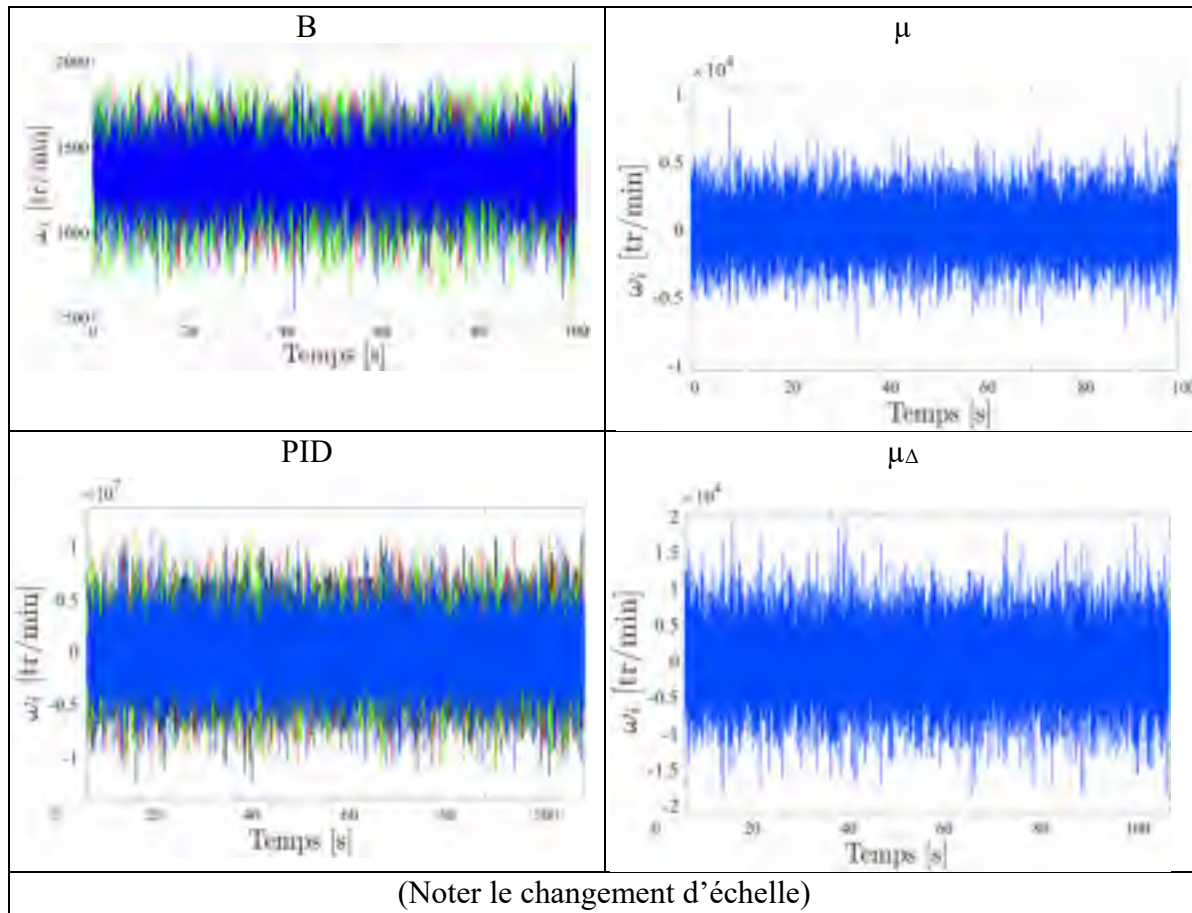
Figure 7.126 Vitesses \omega_1 (noire), \omega_2 (rouge), \omega_3 (verte), \omega_4 (bleue) lors d'une consigne hélicoïdale définie en (7.4), en présence de perturbation en sortie sur le processus non linéaire pour les compensateurs B, \mu , \mu\Delta , PID
