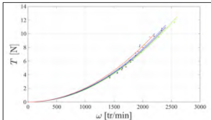
Figure 8.26 T en fonction de \omega , mesures pratiques en pointiller et fonctions approximées x\omega^2 en trait plein pour les moteurs : M 1 (vert), M 2 (noir), M 3 (bleu), M 4 (rouge)
