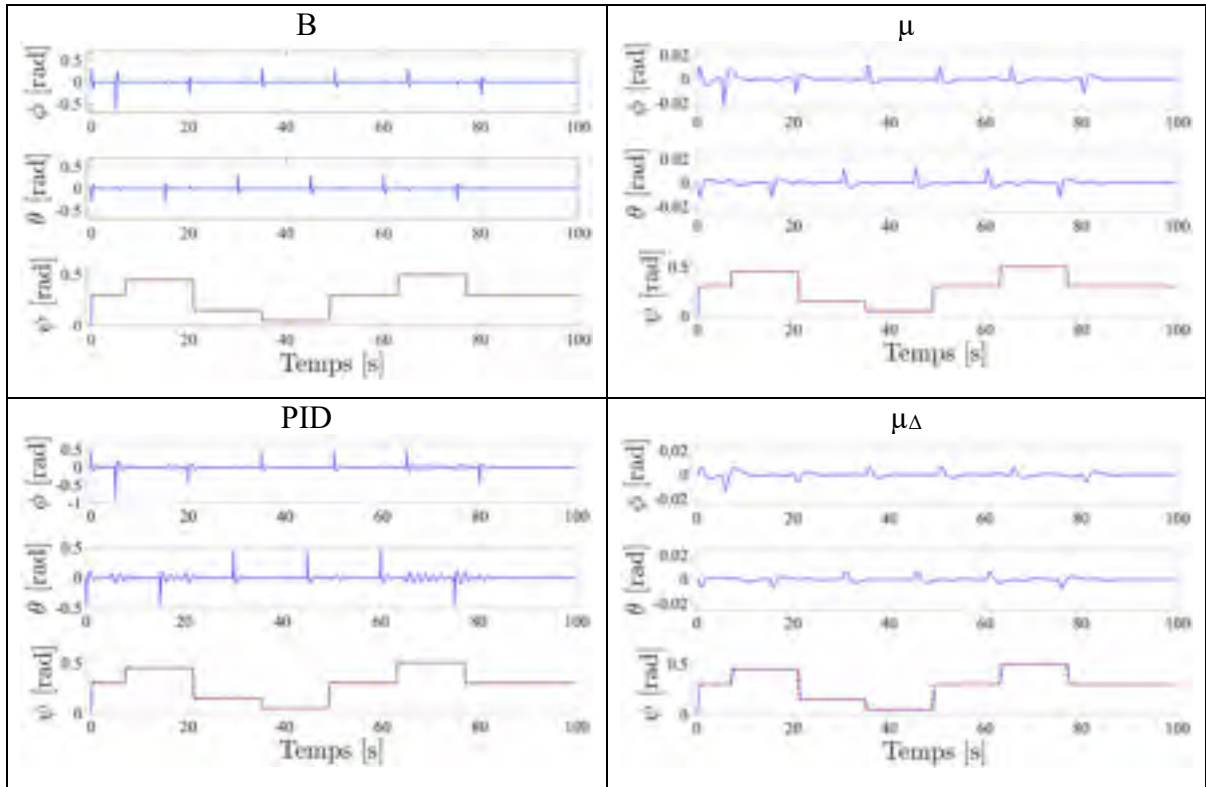
Figure 7.29 Réponses temporelles des angles \phi , \theta , \psi pour le scénario de référence en pointillé rouge (7.2), avec les compensateurs B, \mu , PID, \mu_{\Delta} sur le processus non linéaire
