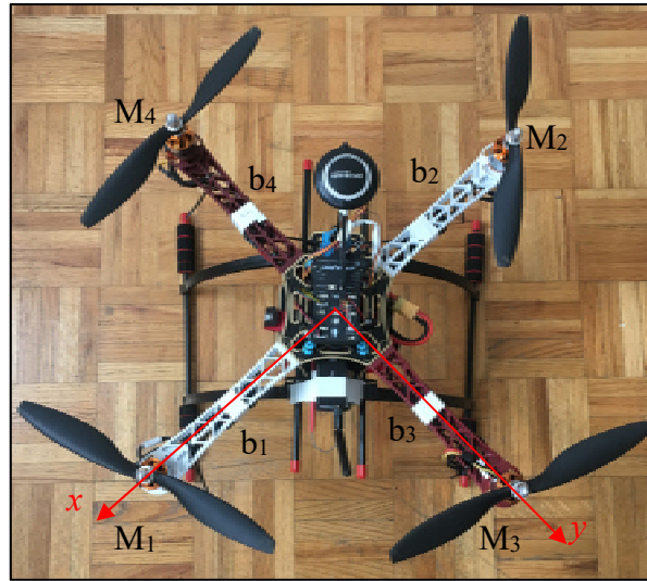
Figure 8.31 Localisation des moteurs M_1 , ... M_4 et des bras b_1 , ... b_4 sur le drone réel
