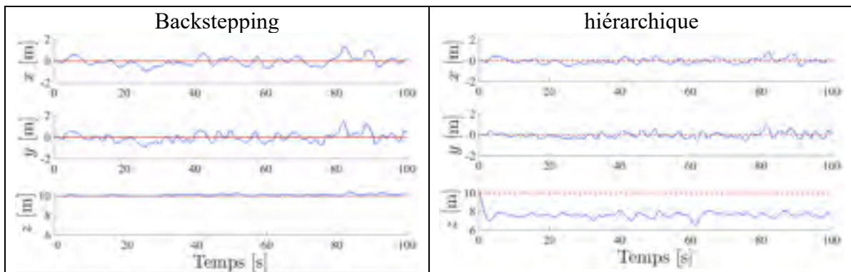
Figure 7.98 Déplacements sur les axes x , y , z lors d'un vol stationnaire en présence de perturbation en sortie pour les compensateurs backstepping et hiérarchique
