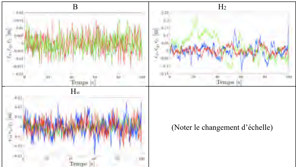
Figure 7.89 Erreurs e_x (bleue), e_y (rouge), e_z (verte) lors d'un vol stationnaire en présence de perturbation en sortie pour les compensateurs B, H_2 , H_\infty appliqués sur le modèle non linéaire de drone
