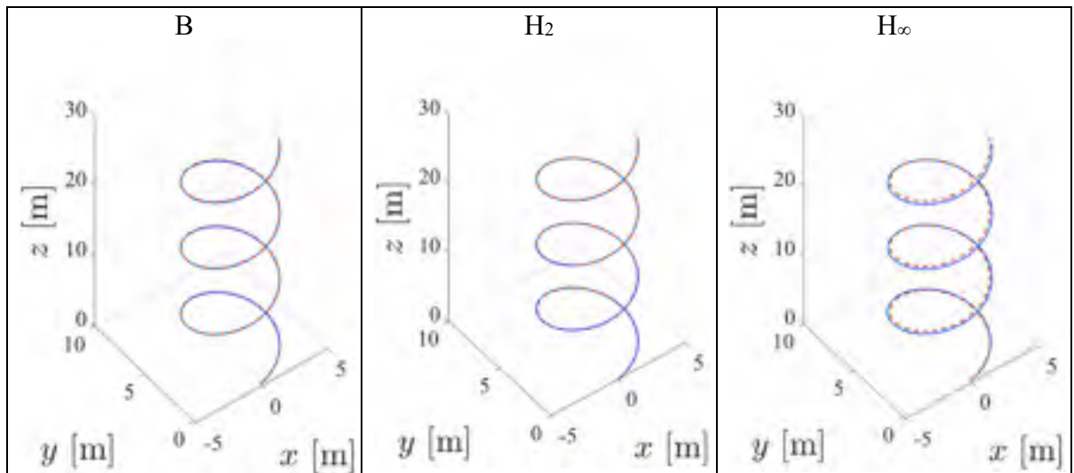
Figure 7.42 Déplacement en bleu sur x, y, z lors d'une consigne hélicoïdale en pointillé rouge et définie en (7.4), pour les compensateurs : B, H_2 , H_\infty
