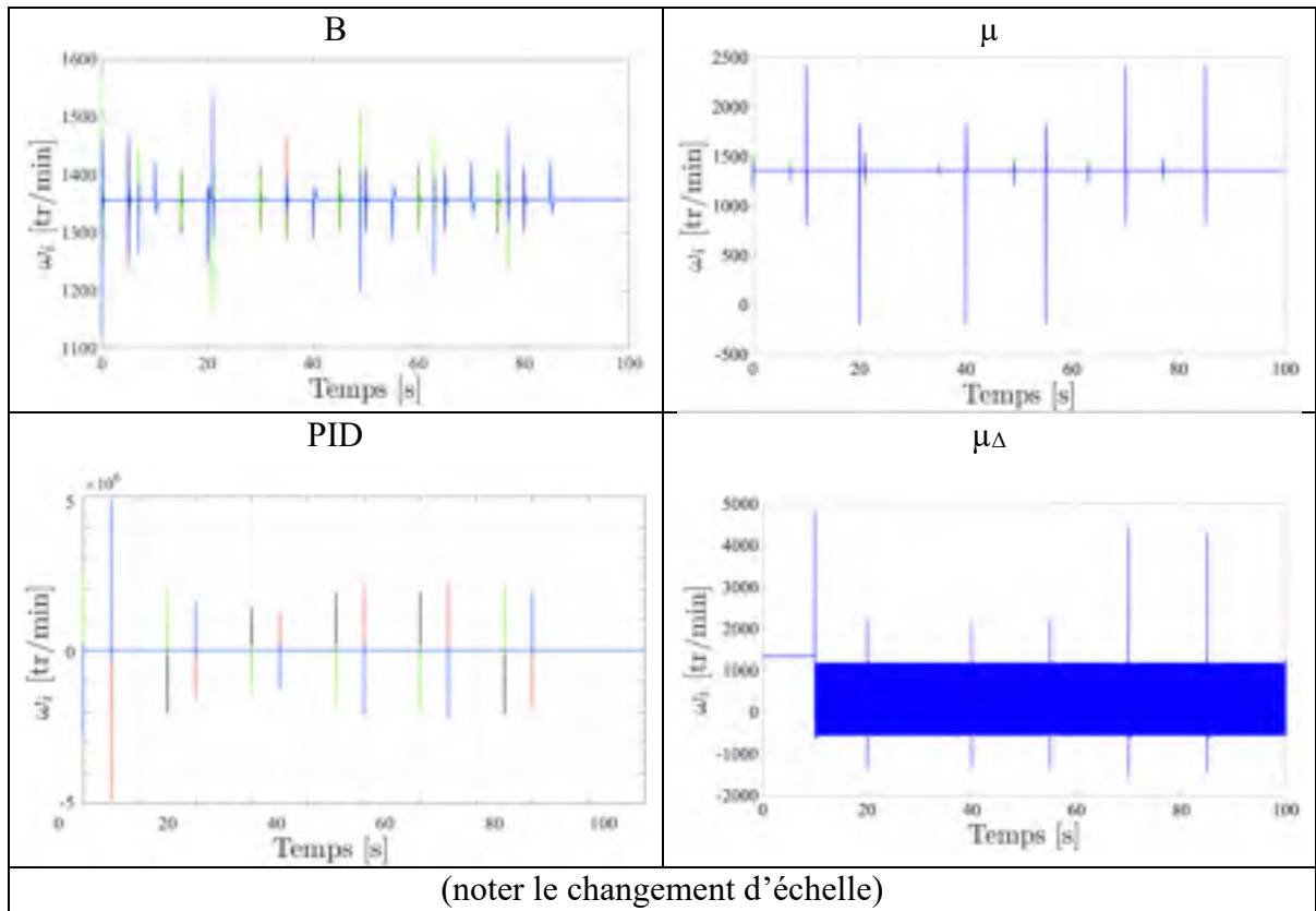
Figure 7.31 Vitesses \omega_1 (noire), \omega_2 (rouge), \omega_3 (verte), \omega_4 (bleue) pour le scénario de référence en pointillé rouge et défini en (7.2), avec les compensateurs B, \mu , PID, \mu_\Delta sur le processus non linéaire
