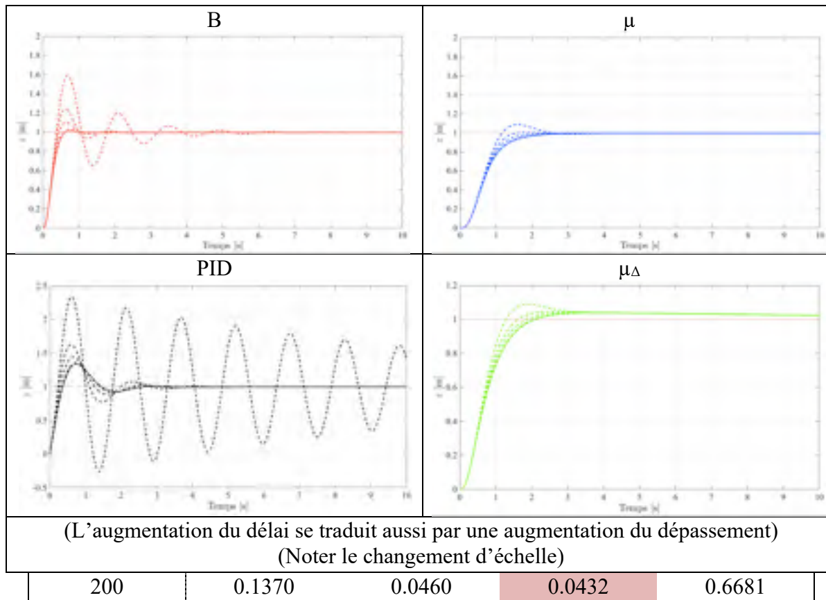
Figure 7.138 Réponses unitaires nominales en trait plein sur l'axe z et en pointillés avec l'ajout de délais de mesure, pour les compensateurs : B (rouge), \mu (bleu), PID (noir), \mu_{\Delta} (vert) dans le cas d'un processus linéaire
