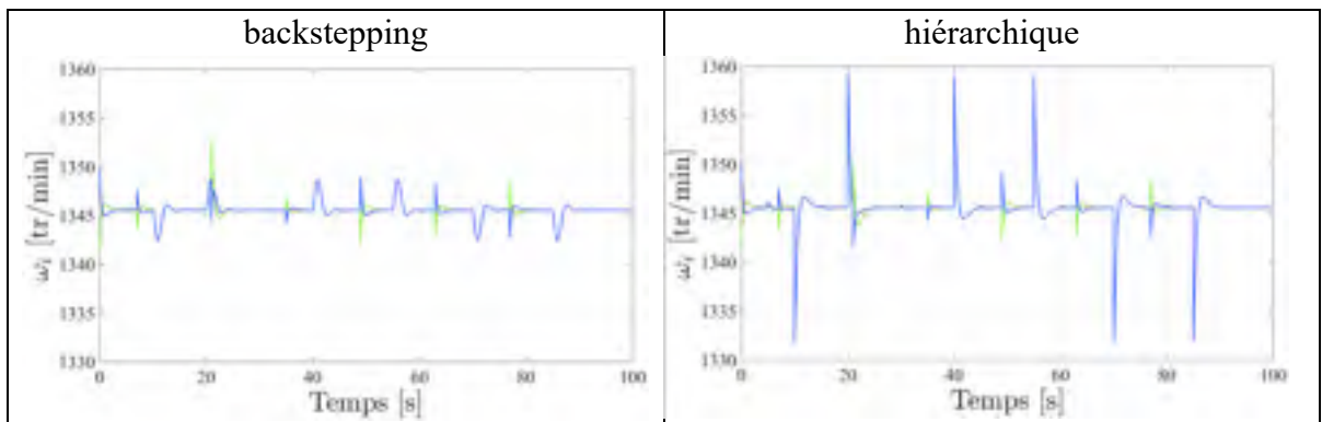
Figure 7.35 Vitesse \omega_1 (noire), \omega_2 (rouge), \omega_3 (verte), \omega_4 (bleue) pour le scénario de référence défini en (7.2), avec les compensateurs backstepping et hiérarchique
