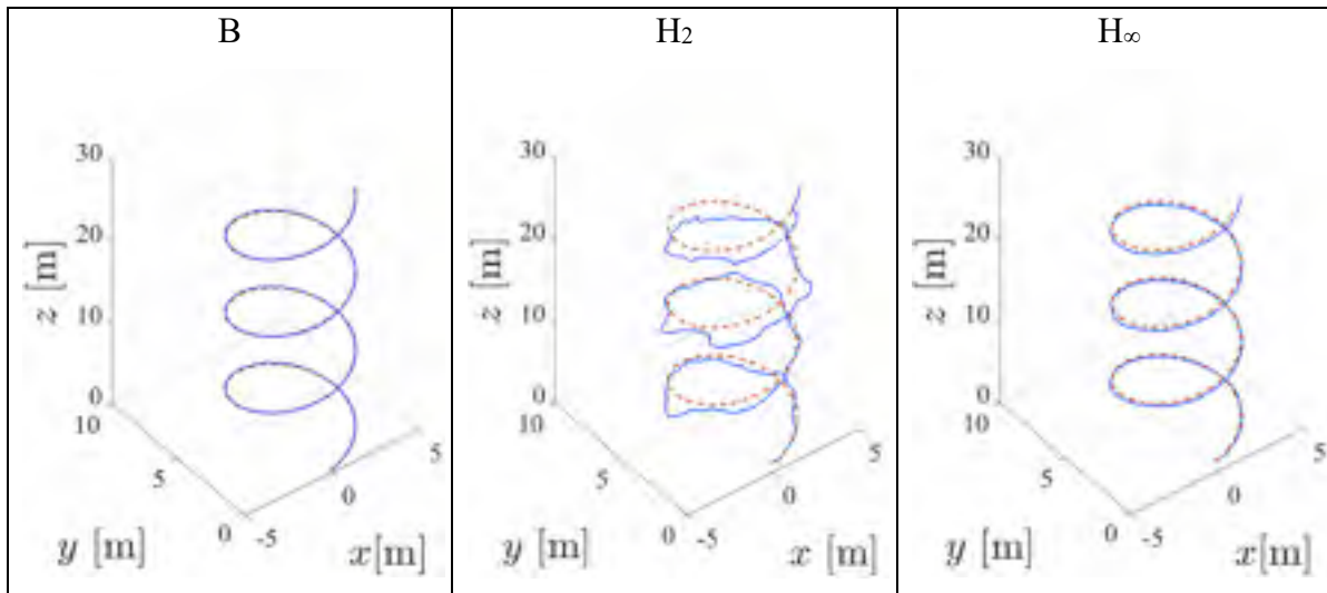
Figure 7.115 Déplacements en 3D sur les axes x , y , z lors d'une consigne hélicoïdale définie en (7.4), en présence de perturbation en sortie pour les compensateurs B, H_2 , H_\infty sur le processus non linéaire
