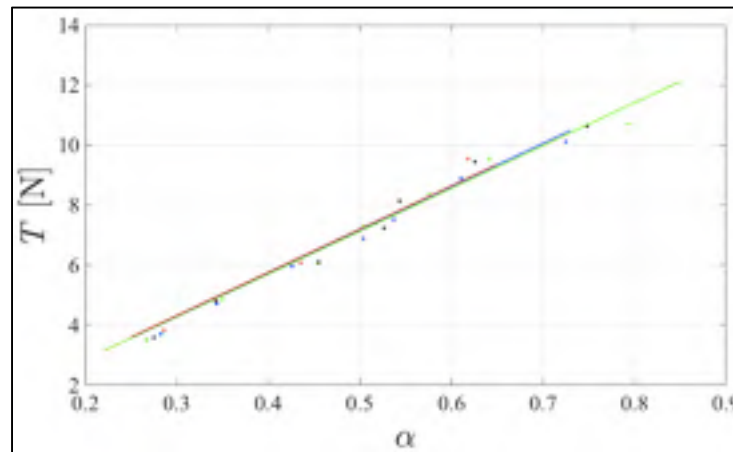
Figure 8.30 T_i en fonction de \alpha_i , mesures pratiques en pointiller et fonctions approximées k_i \alpha_i en trait plein pour les moteurs : M_1 (vert), M_2 (noir), M_3 (bleu), M_4 (rouge)
