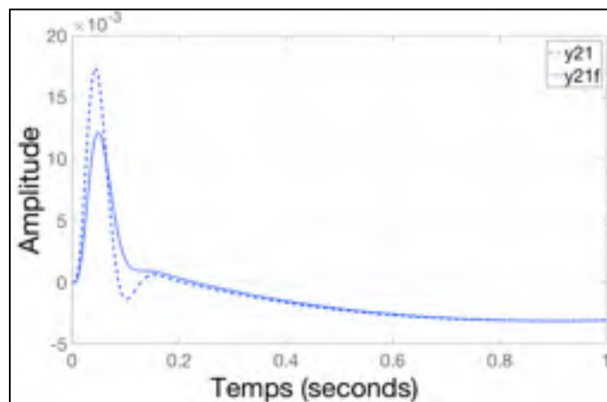
Figure 4.52 Réponse indicielle de y_{21}(t) et y_{21f}(t)
