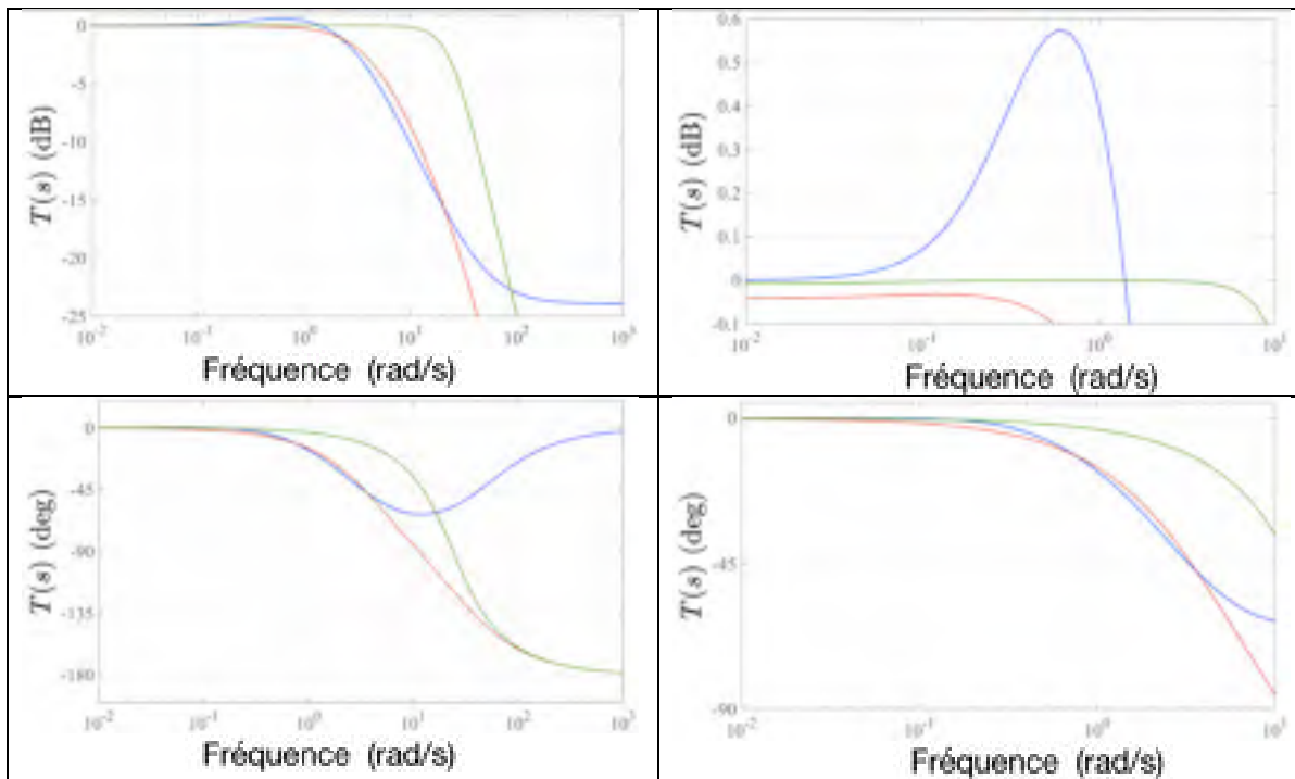
Figure 8.36 Bode des fonctions de transfert en boucle fermée T(s) à gauche et zoom autour de 0 dB à droite pour les compensateurs (gains sur la première ligne et phases sur la deuxième ligne) : PID_{\dot{\phi}} (bleu) ; B (rouge) ; B amélioré (vert)
