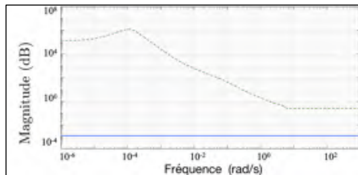
Figure 5.29 \mu_{\Delta s} et \|\mathcal{F}_l(P(j\omega), K(j\omega))\|_{\infty} pour l'axe x - y sans incertitude
