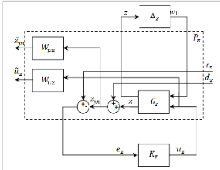
Figure 5.22 Mise sous forme canonique avec insertion des fonctions de pondérations W_{pz} , W_{uz} et du compensateur K_z
