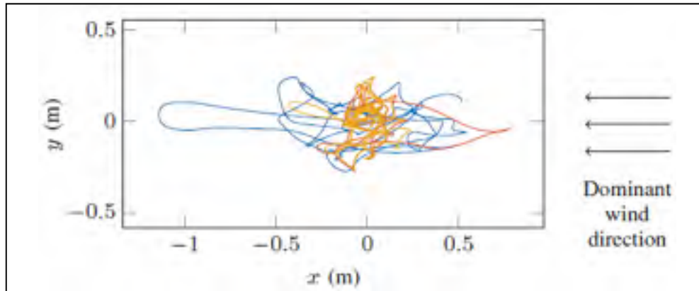
Figure 1.14 Variation des positions sur les axes x/y pour un vol stationnaire de 60 s avec un vent de travers de 5 m/s.
