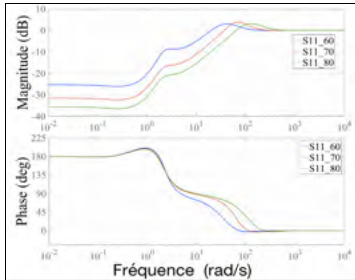
Figure 4.21 Bode de S_{11}(s) pour C_{max} = 60, 70 et 80 dB dans le cas avec erreur statique
