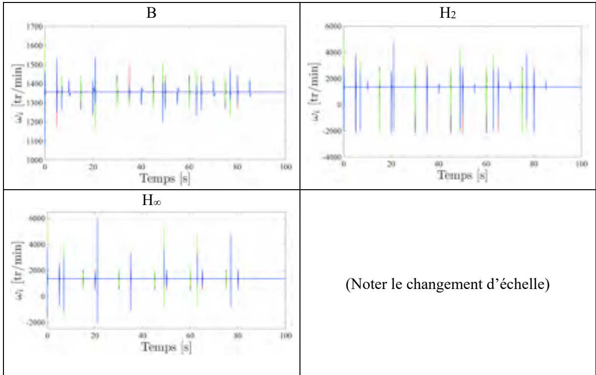
Figure 7.27 Vitesses \omega_1 (noire), \omega_2 (rouge), \omega_3 (verte), \omega_4 (bleue) pour le scénario de référence défini en (7.2), avec les compensateurs B, H 2 , H ∞ sur le processus non linéaire
