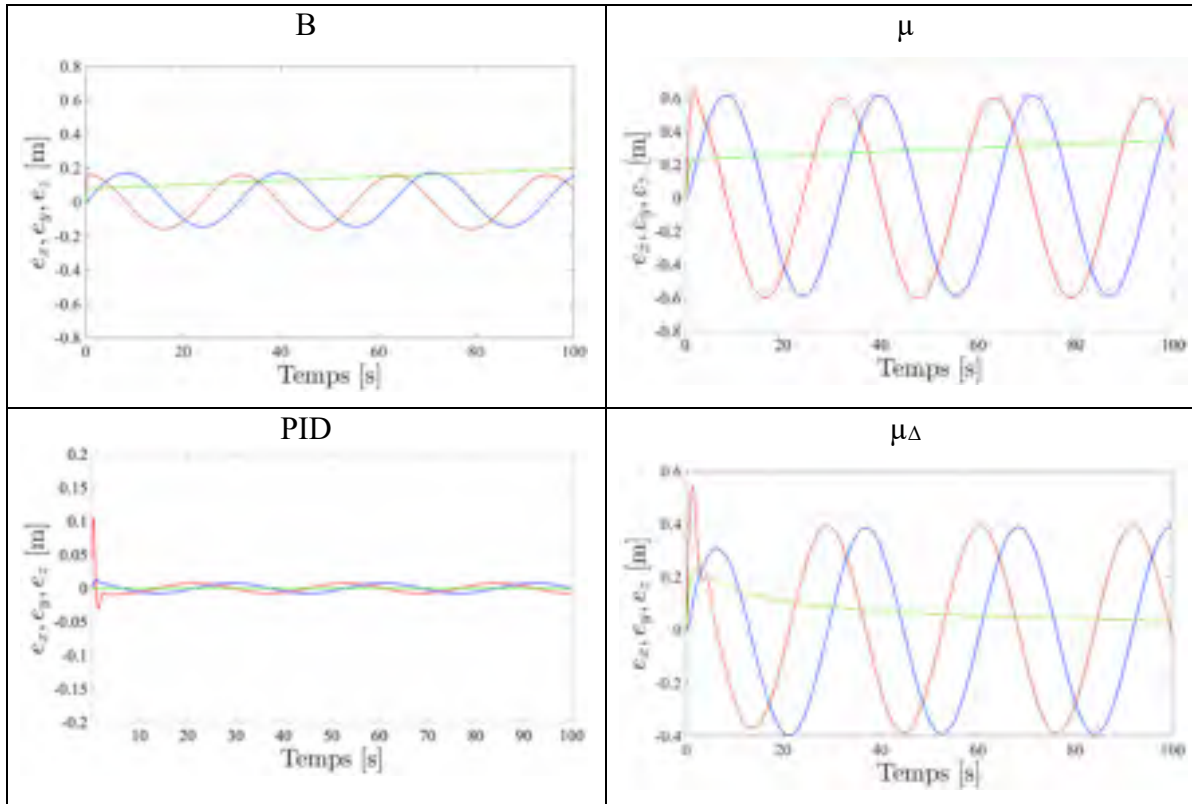
Figure 7.51 Erreurs e_x (bleue), e_y (rouge), e_z (verte) lors d'une consigne hélicoïdale définie en (7.4), pour les compensateurs : B, \mu , PID, \mu_\Delta
