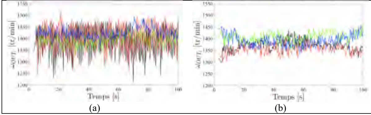
Figure 8.45 Mesures expérimentales avec le drone F450J des vitesses \omega_1, \omega_2, \omega_3, \omega_4 venant du drone pour les compensateurs : \text{PID}_\phi (a) ; B (b)
