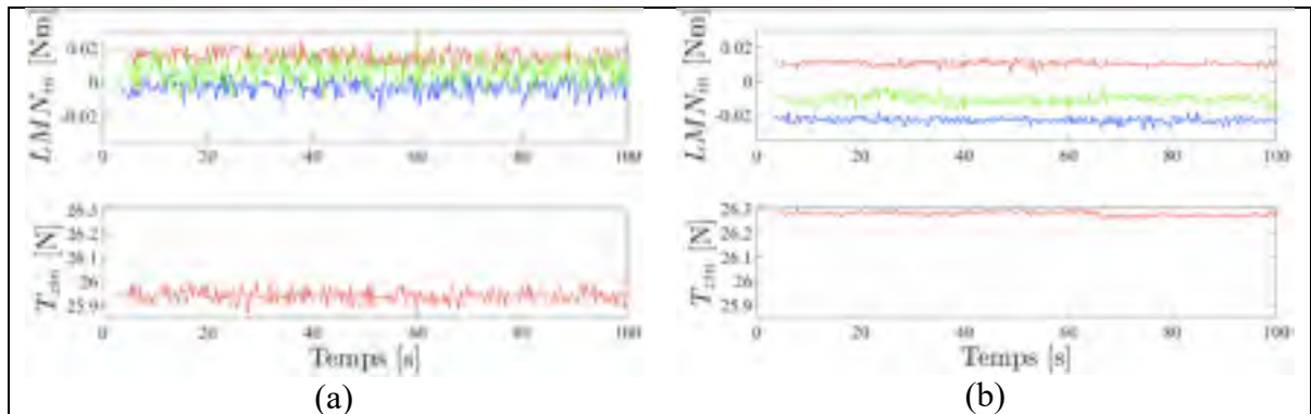
Figure 8.44 Commandes expérimentales avec le drone F450J en couples L, M, N et en poussée T_z envoyées au drone pour les compensateurs : PID _{\phi} (a) ; B (b)
