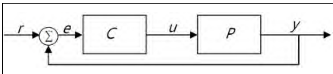
Figure 7.10 Schéma général de la boucle de commande
