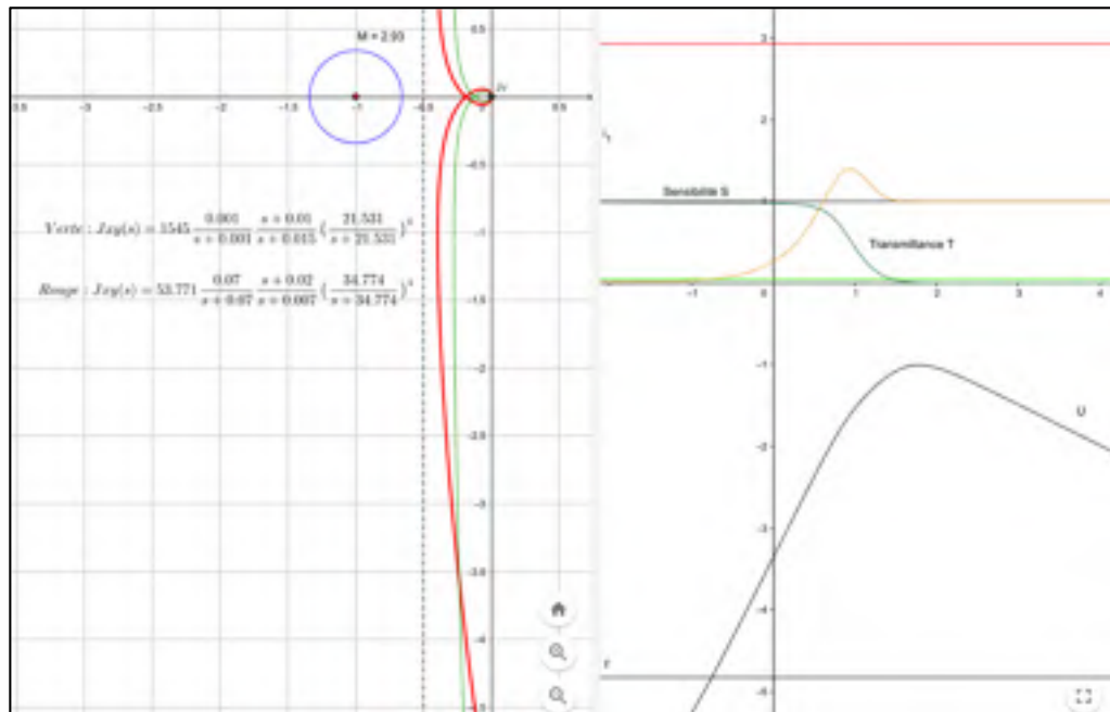
Figure 7.149 Conception de la commande B pour des axes x et y avec GeoGebra avec sur la partie de gauche : commande B (rouge) ; commande B_u (vert) ; Cercle de sensibilité S_{ey}(s) (bleu). À droite pour le compensateur B uniquement : Sensibilité S_{ey}(s) (jaune) ; Transmittance T(s) (verte foncée) ; \varepsilon (vert clair) ; M_s (rouge) ; U(s) (noir)
