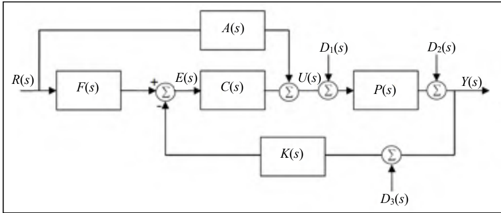
Figure 2.4 Schéma de commande avec préfiltre et préfiltre anticipatif
