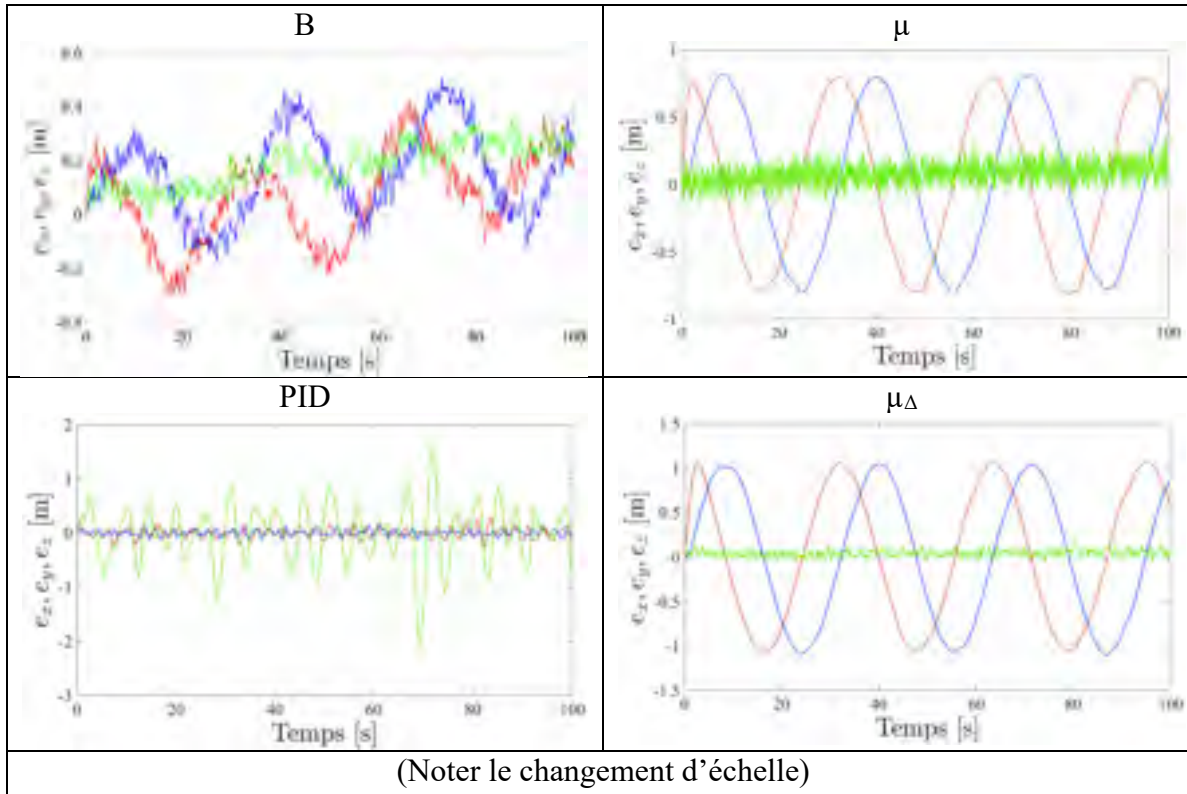
Figure 7.124 Erreurs e_x (bleue), e_y (rouge), e_z (verte) lors d'une consigne hélicoïdale définie en (7.4), en présence de perturbation en sortie avec le processus non linéaire pour les compensateurs B, \mu , \mu_\Delta , PID
