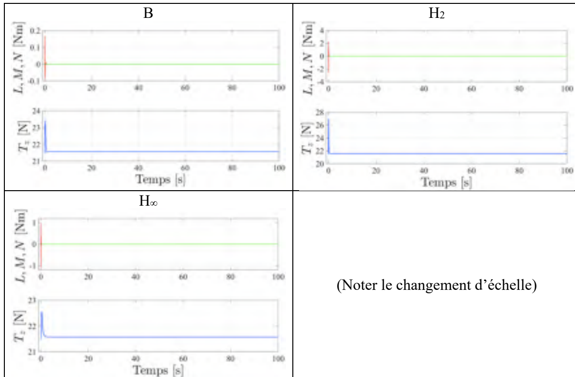
Figure 7.58 Commandes L , M , N , T_z lors d'une consigne hélicoïdale définie en (7.4), pour les compensateurs : B, H_2 , H_\infty
