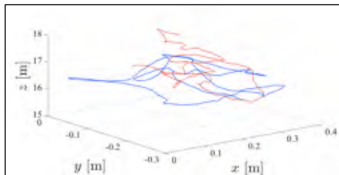
Figure 8.39 Mesures expérimentales avec le drone F450J des déplacements en 3D sur x, y, z pour un vol stationnaire pour les compensateurs : PID _{\phi} (bleu) ; compensateur B (rouge)
