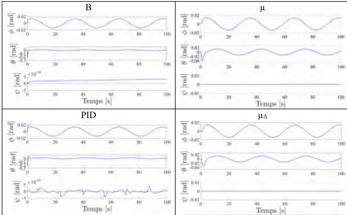
Figure 7.62 Déplacement des angles \phi , \theta , \psi lors d'une consigne hélicoïdale définie en (7.4), pour les compensateurs B, \mu , PID, \mu_{\Delta}
