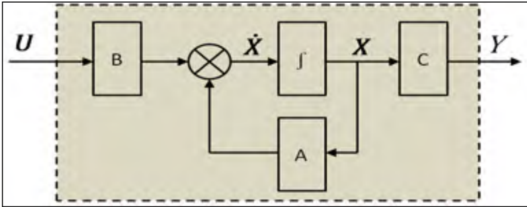
Figure 3.9 Représentation sous forme de schéma synoptique de la modélisation d'état d'un système
