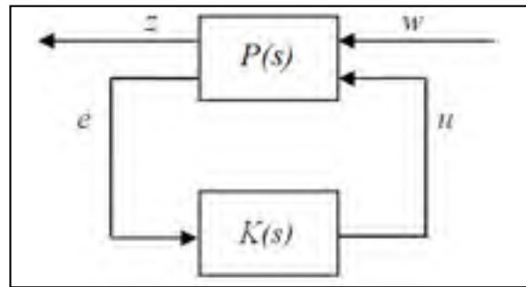
Figure 5.10 P(s) - K(s) sous forme standard
