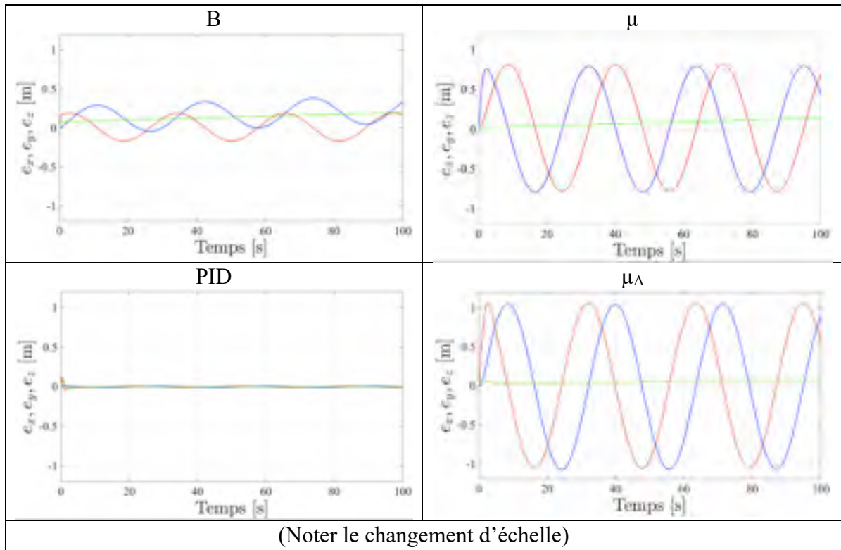
Figure 7.63 Erreurs e_x (bleue), e_y (rouge), e_z (verte) lors d'une consigne hélicoïdale définie en (7.4), pour les compensateurs B, \mu , PID, \mu_\Delta
