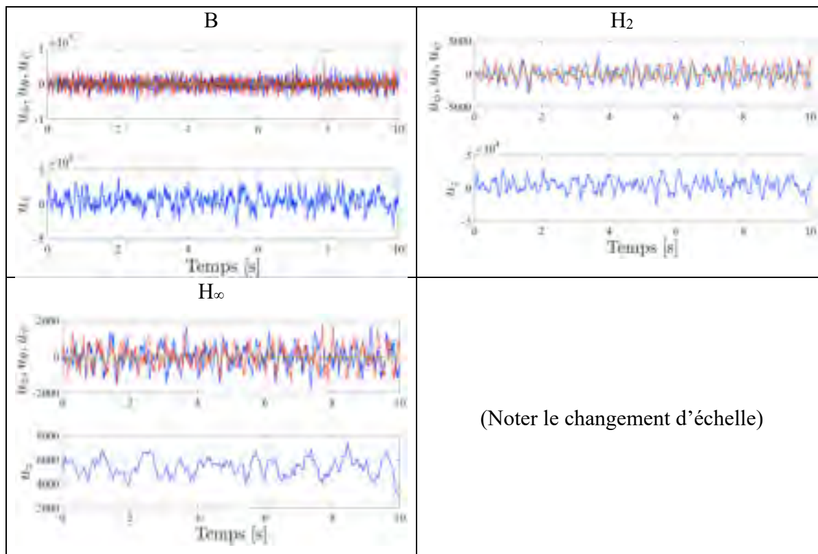
Figure 7.76 Commandes u_\phi (bleue), u_\theta (rouge), u_\psi (verte), u_z lors d'un vol stationnaire en présence de perturbation sur la sortie pour les compensateurs B, H 2 , H ∞ appliqués sur le modèle linéaire de drone
