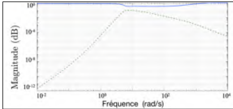
Figure 5.30 Stabilité robuste \|M_{d \rightarrow \tilde{u}}\|_{\infty} en pointillé vert et robuste performance \mu_{\tilde{Z}_p}(M(j\omega)) courbes rouge et bleue (superposées) pour les axes x - y , sans incertitudes
