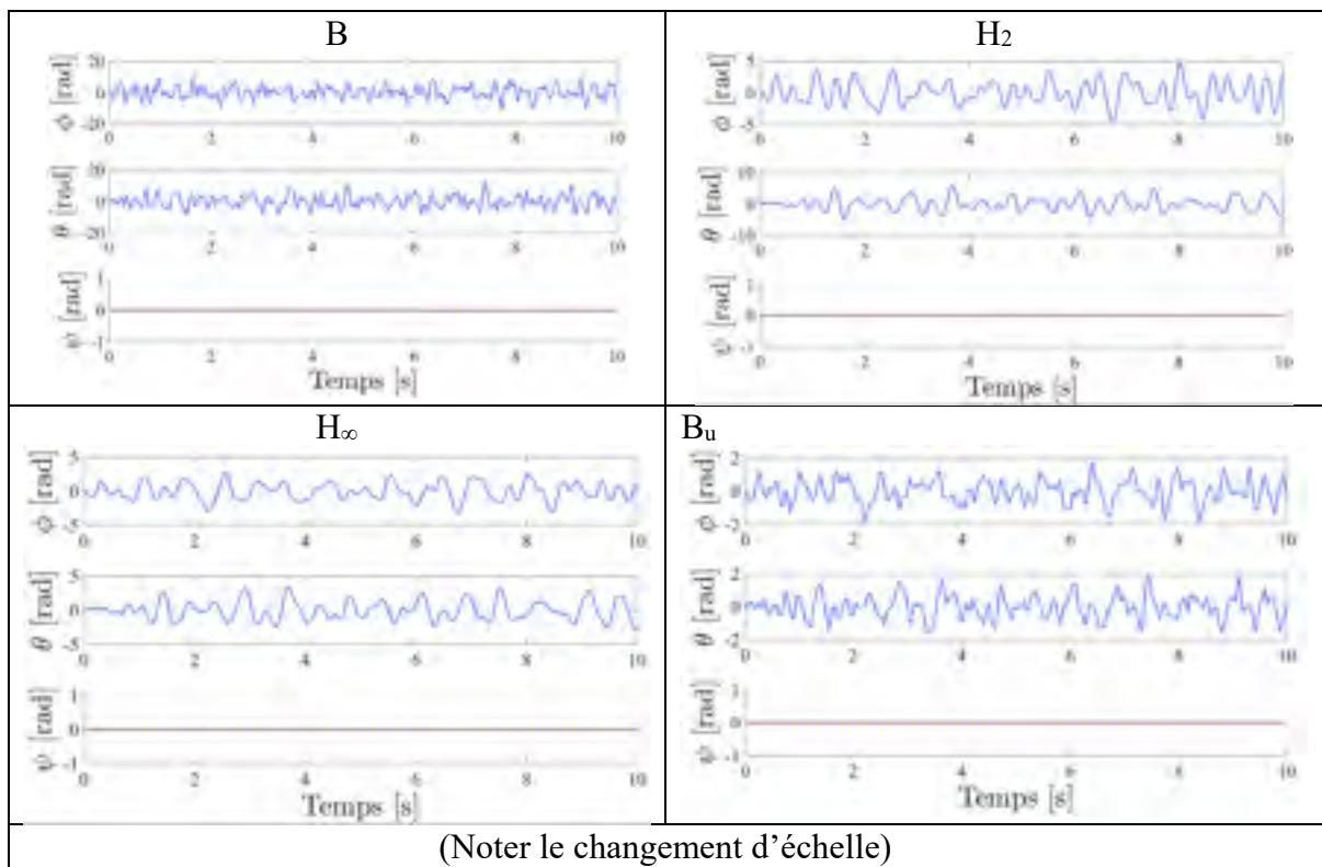
Figure 7.157 Déplacements autour des angles \phi , \theta , \psi lors d'un vol stationnaire en présence de perturbation en sortie pour les compensateurs B , H_2 , H_\infty , B_u appliqués sur le modèle linéaire de drone
