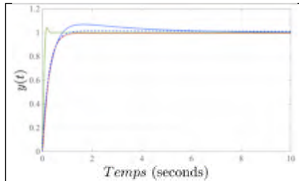
Figure 8.37 Réponse unitaire de la sortie y(t) pour les compensateurs : \text{PID}_{\phi} (bleu) ; B (rouge) ; B amélioré (vert)
