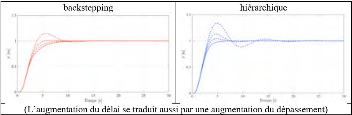
Figure 7.146 Réponses unitaires nominales en trait plein sur les axes {xθ} ou {yφ} et en pointillés avec l’ajout de délais de mesure, pour les compensateurs : backstepping (rouge), hiérarchique (bleu)
