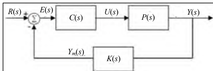
Figure 2.1 Boucle fermée d'un système entrée sortie
