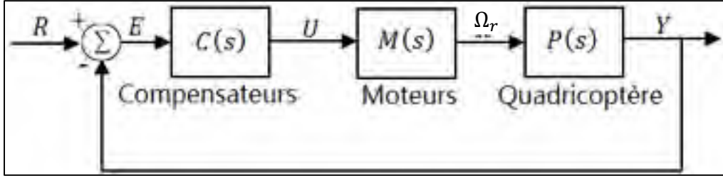
Figure 3.15 Boucle de commande avec insertion des moteurs
