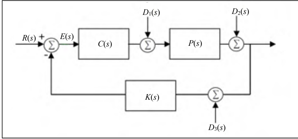
Figure 2.2 Boucle de commande avec les perturbations externes D_1(s) , D_2(s) , et D_3(s)
