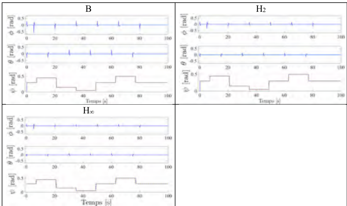
Figure 7.17 Réponses temporelles (bleue) des angles \phi , \theta , \psi pour le scénario de référence (pointillé rouge) défini en (7.2), avec les compensateurs B, H_2 , H_\infty sur le processus linéaire
