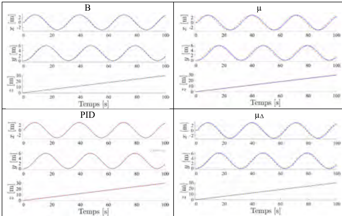
Figure 7.49 Déplacement sur x , y , z lors d'une consigne hélicoïdale définie en (7.4), pour les compensateurs : B, \mu , PID, \mu_{\Delta}
