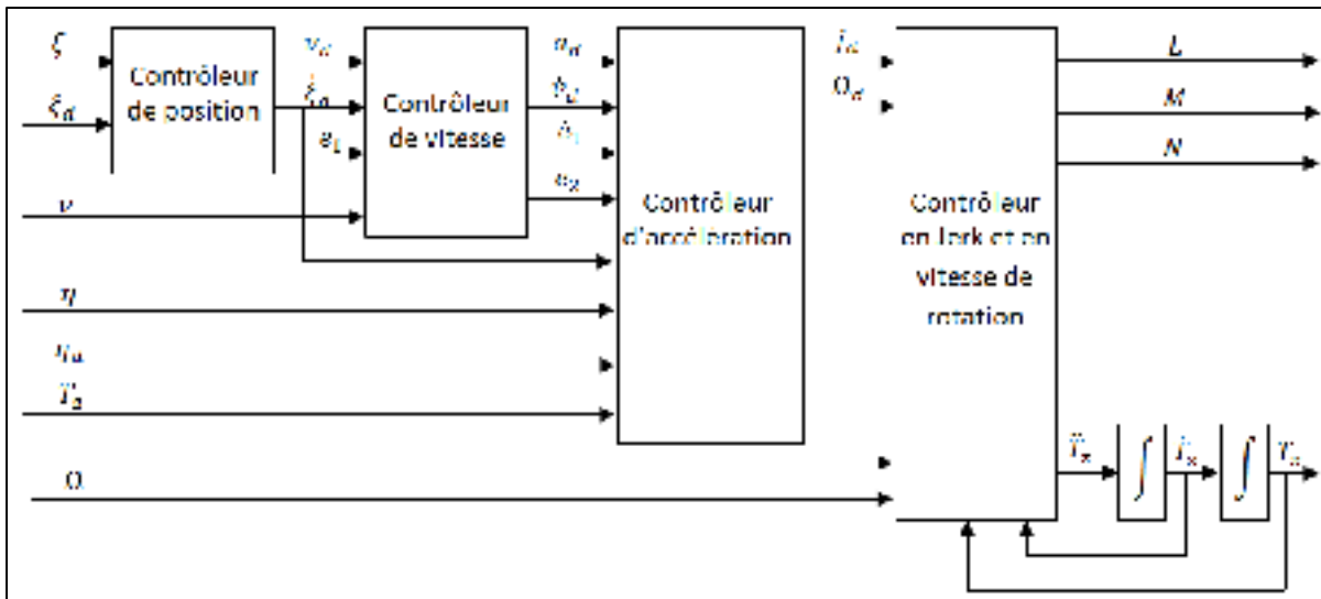
Figure 6.4 Schéma général de la structure de commande par backstepping
