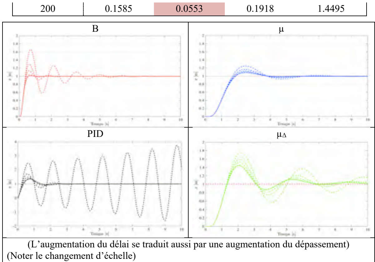
Figure 7.137 Réponses unitaires nominales en trait plein sur les axes \{x\theta\} ou \{y\phi\} et en pointillés avec l'ajout de délais de mesure, pour les compensateurs : B (rouge), \mu (bleu), PID (noir), \mu_\Delta (vert) dans le cas d'un processus linéaire
