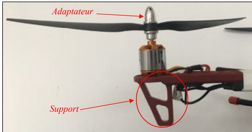
Figure 8.32 Localisation de l'adaptateur pour l'hélice et du support pour moteur
