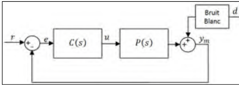
Figure 7.72 Insertion de bruit blanc dans la boucle fermée
