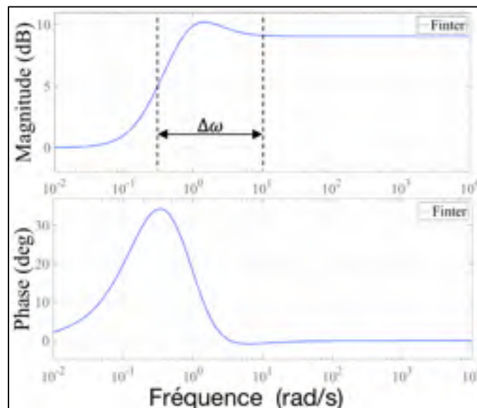
Figure 4.14 Bode du filtre intermédiaire F_{inter}
