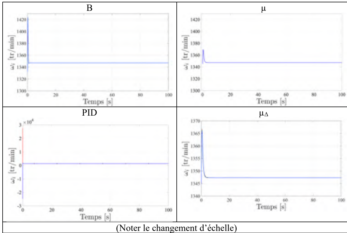
Figure 7.53 Vitesses \omega_1 (noire), \omega_2 (rouge), \omega_3 (verte), \omega_4 (bleue) lors d'une consigne hélicoïdale définie en (7.4), pour les compensateurs : B, \mu , PID, \mu_\Delta
