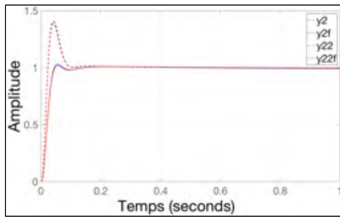
Figure 4.51 Réponse temporelle de y_2(t) , y_{2f}(t) , y_{22}(t) et y_{22f}(t)
