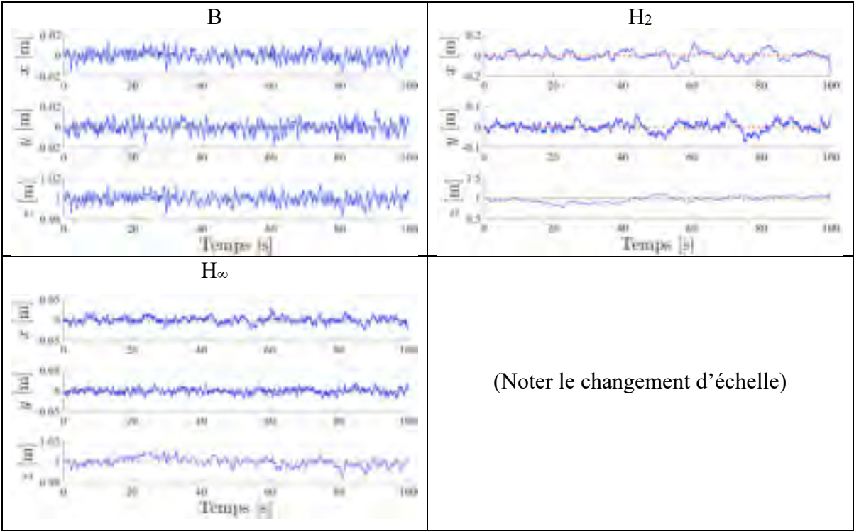
Figure 7.85 Variations des axes x, y, z lors d'un vol stationnaire en présence de perturbation sur la sortie pour les compensateurs B, H 2 , H ∞ appliqués sur le modèle non linéaire de drone
