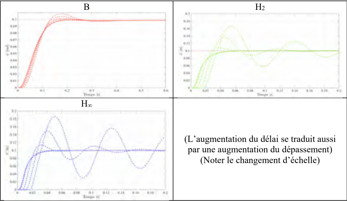
Figure 7.142 Réponses unitaires nominales en trait plein autour de l'angle \psi et en pointillés avec l'ajout de délais de mesure, pour les compensateurs : B (rouge), H 2 (vert), H ∞ (bleu) pour le processus non linéaire
