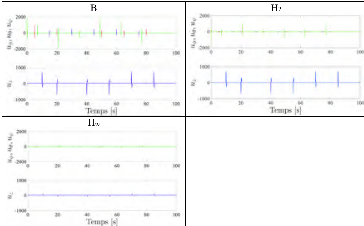
Figure 7.18 Réponses des commandes u_\phi (bleue), u_\theta (rouge), u_\psi (verte) et u_z pour le scénario de référence défini en (7.2), avec les compensateurs B, H_2 , H_\infty sur le processus linéaire
