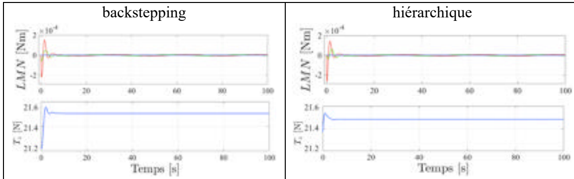
Figure 7.70 Commandes L, M, N, T_z lors d'une consigne hélicoïdale définie en (7.4), pour les compensateurs backstepping et hiérarchique
