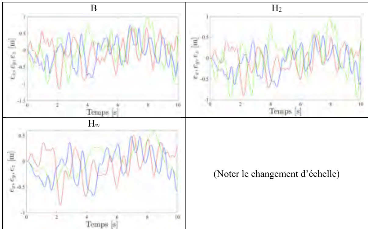
Figure 7.77 Erreurs e_x (bleue), e_y (rouge), e_z (verte) lors d'un vol stationnaire en présence de perturbation sur la sortie pour les compensateurs B, H 2 , H ∞ appliqués sur le modèle linéaire de drone
