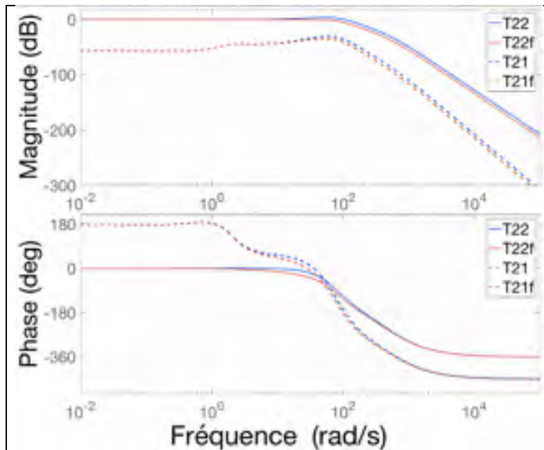
Figure 4.48 Bode de T_{22}(s) , T_{21}(s) , T_{22f}(s) , T_{21f}(s) dans le cas sans erreur statique
