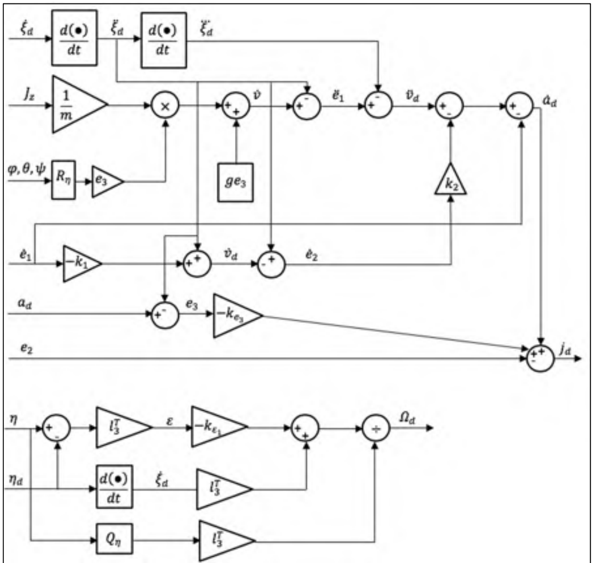
Figure 6.3 Schéma bloc des commandes virtuelles en jerk j_d et en vitesse de rotation \Omega_d
