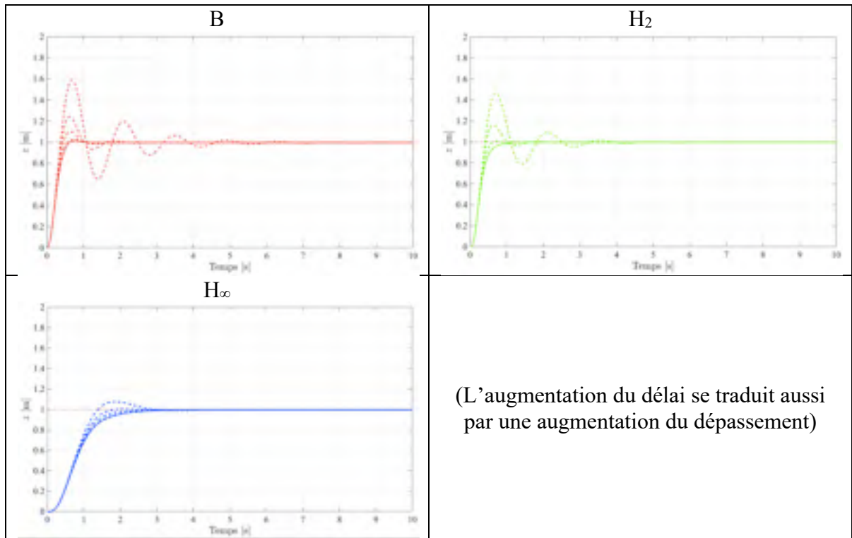
Figure 7.135 Réponses unitaires nominales en trait plein sur l'axe z et en pointillés avec l'ajout de délais de mesure, pour les compensateurs : B (rouge), H_2 (vert), H_\infty (bleu) pour un processus linéaire
