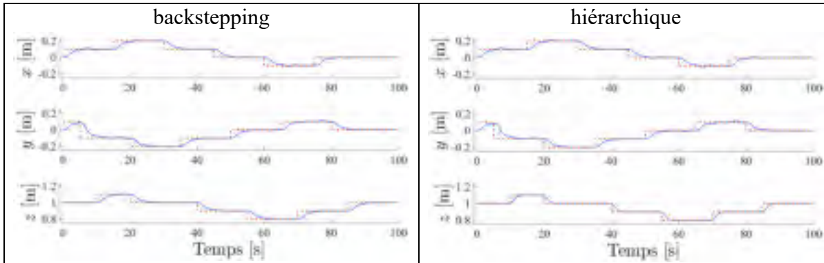
Figure 7.32 Réponses temporelles sur les axes x , y , z pour le scénario de référence en pointillé rouge et défini en (7.2), avec les compensateurs backstepping et hiérarchique
