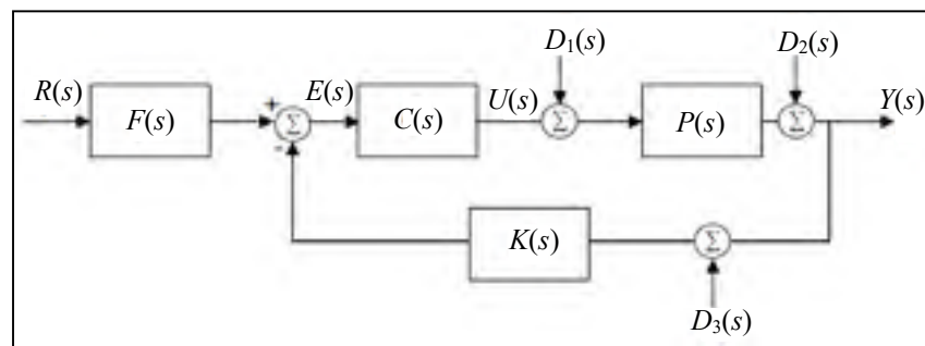
Figure 2.3 Schéma de commande avec préfiltre
