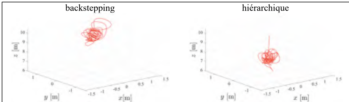
Figure 7.97 Déplacements sur les axes x , y , z lors d'un vol stationnaire en présence de perturbation en sortie pour les compensateurs backstepping et hiérarchique
