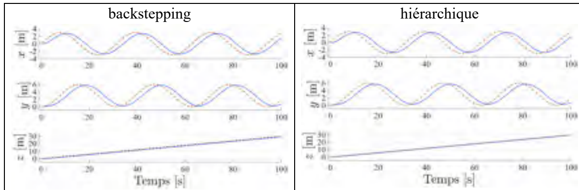
Figure 7.67 Déplacement sur x , y , z lors d'une consigne hélicoïdale définie en (7.4), pour les compensateurs backstepping et hiérarchique
