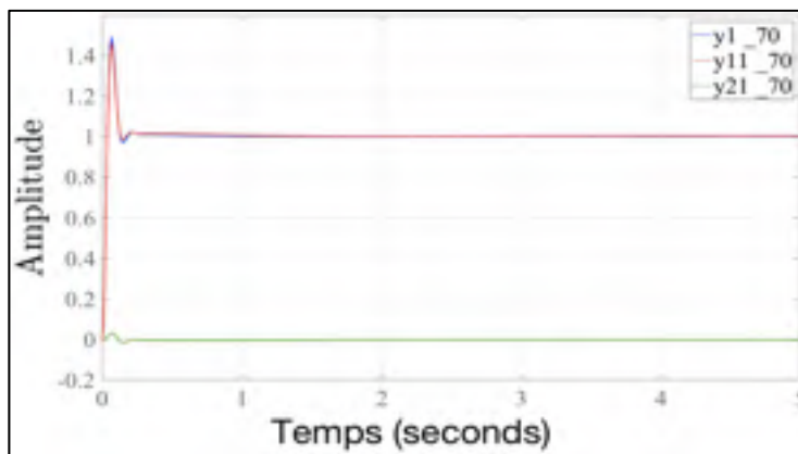
Figure 4.40 Réponse temporelle de y_1(t) , y_{11}(t) et y_{21}(t) pour C_{max} = 70 dB, dans le cas sans erreur statique
