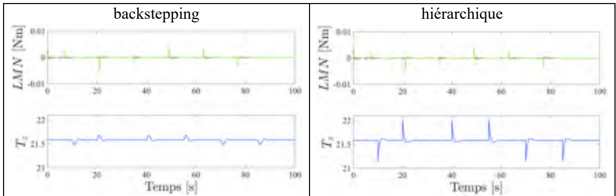
Figure 7.34 Réponses des commandes L , M , N , T_z pour le scénario de référence défini en (7.2), avec les compensateurs backstepping et hiérarchique
