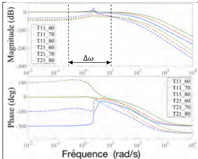
Figure 4.11 Bode des transmittances T_{11}(s) et T_{21}(s) pour trois valeurs du gain k_1
