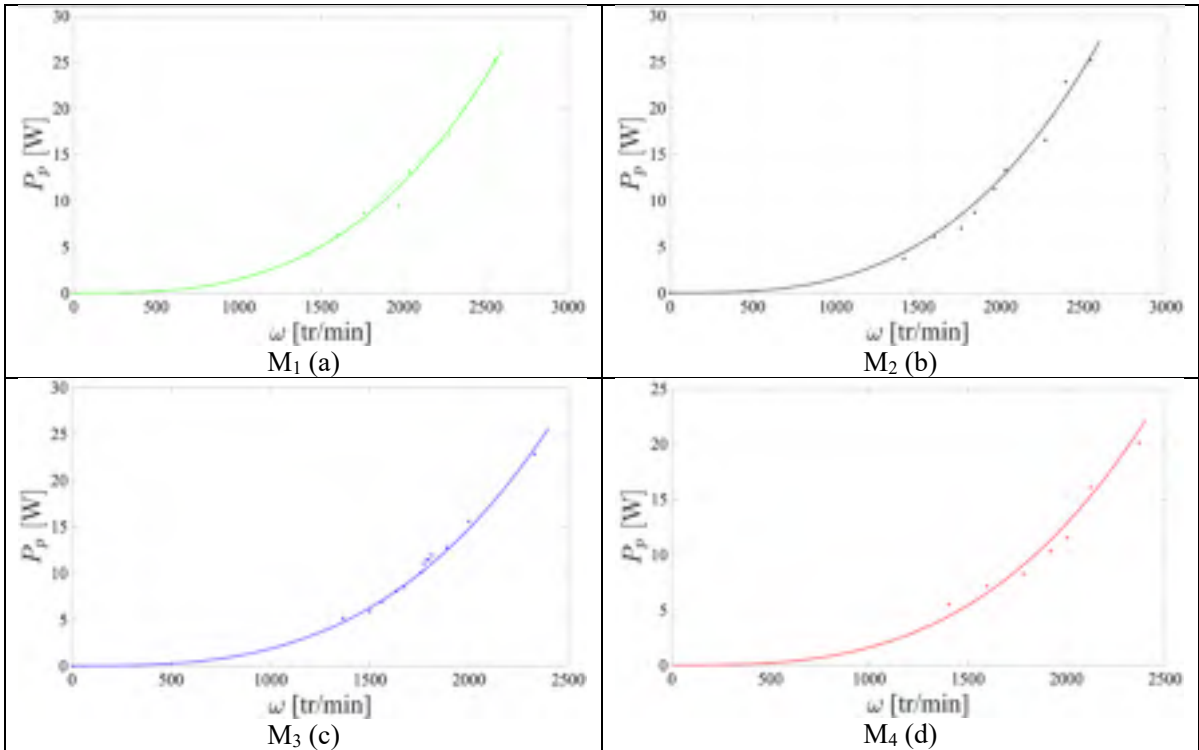
Figure 8.27 P_p en fonction de \omega mesures pratiques en pointiller et fonctions approximées k\omega^3 en trait plein pour les moteurs : M 1 (a), M 2 (b), M 3 (c), M 4 (d)
