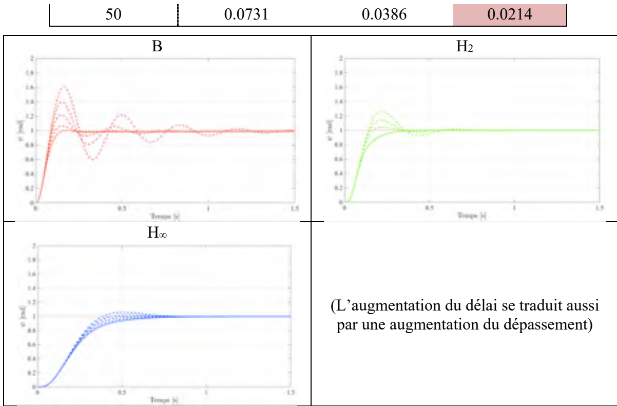
Figure 7.136 Réponses unitaires nominales en trait plein autour de l'angle \psi et en pointillés avec l'ajout de délais de mesure, pour les compensateurs : B (rouge) , H 2 (vert), H ∞ (bleu) pour un processus linéaire
