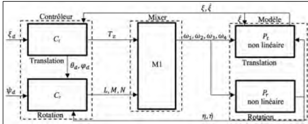
Figure 3.14 Boucle fermée avec le processus non linéaire pour une commande en translation et rotation séparée
