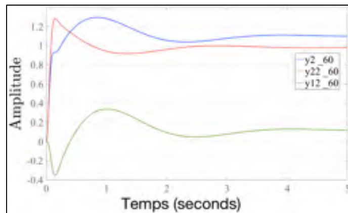
Figure 4.28 Allure de y_2(t) , y_{12}(t) et y_{22}(t) optimisées pour C_{max} = 60 dB
