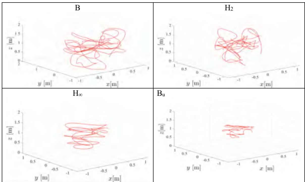
Figure 7.155 Déplacements sur les axes x , y , z lors d'un vol stationnaire en présence de vent pour les compensateurs B , H_2 , H_\infty , B_u appliqués sur le modèle linéaire de drone
