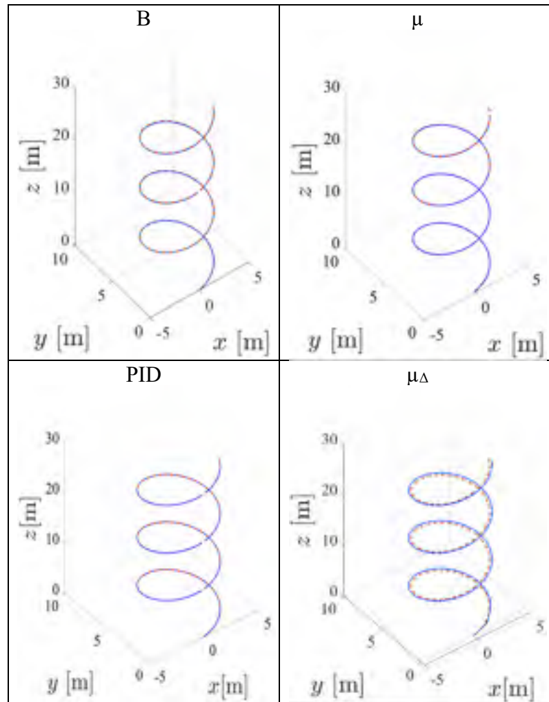
Figure 7.48 Déplacement en 3D sur x , y , z lors d'une consigne hélicoïdale définie en (7.4), pour les compensateurs : B, \mu , PID, \mu\Delta
