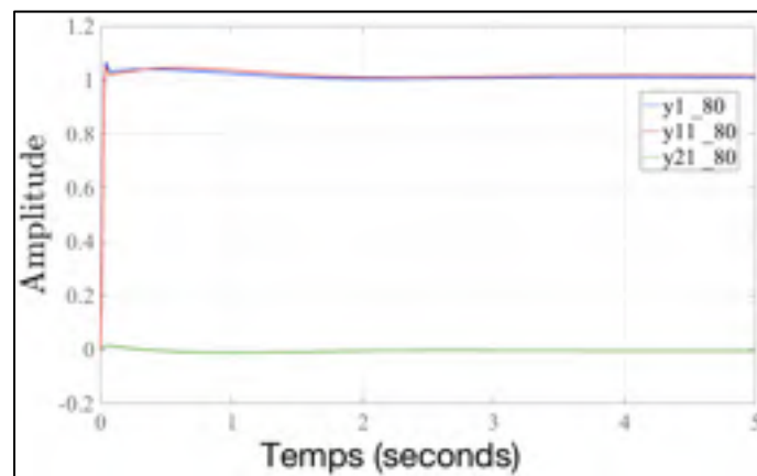
Figure 4.27 Allure de y_1(t) , y_{11}(t) et y_{21}(t) optimisées pour C_{max} = 80 dB
