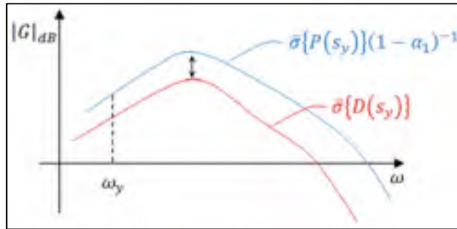
Figure 4.5 Représentation graphique de l'inégalité \bar{\sigma}\{D(s_y)\} < \bar{\sigma}\{P(s_y)\}(1 - \alpha_1)^{-1}
