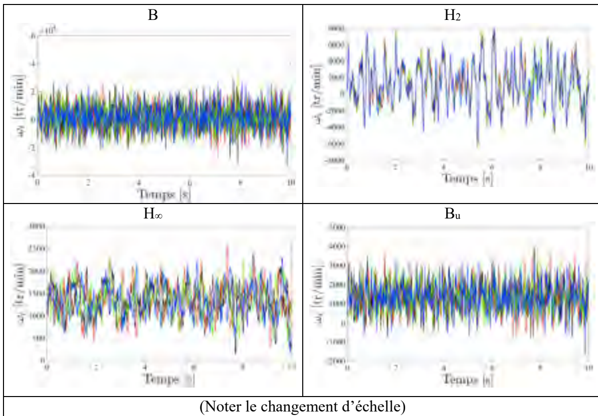
Figure 7.160 Vitesses \omega_1 (noire), \omega_2 (rouge), \omega_3 (verte), \omega_4 (bleue) lors d'un vol stationnaire en présence de perturbation en sortie pour les compensateurs B, H_2 , H_\infty , B_u appliqués sur le modèle linéaire de drone
