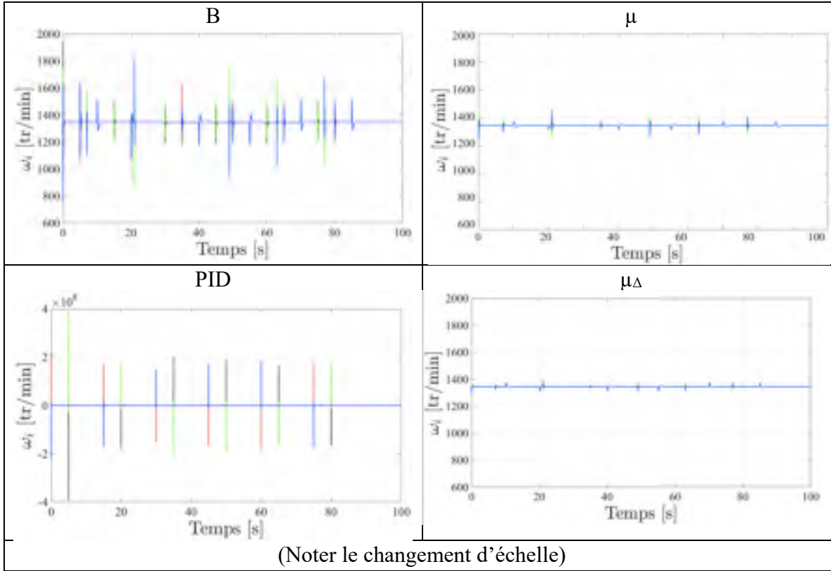
Figure 7.23 Vitesses \omega_1 (noire), \omega_2 (rouge), \omega_3 (verte), \omega_4 (bleue) pour le scénario de référence défini en (7.2), avec les compensateurs B, \mu , PID, \mu_\Delta sur le processus linéaire
