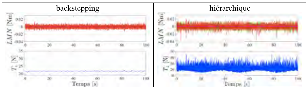
Figure 7.131 Commandes L (bleue), M (rouge), N (verte), T_z lors de la consigne hélicoïdale (7.4), avec perturbation en sortie pour les compensateurs backstepping et hiérarchique
