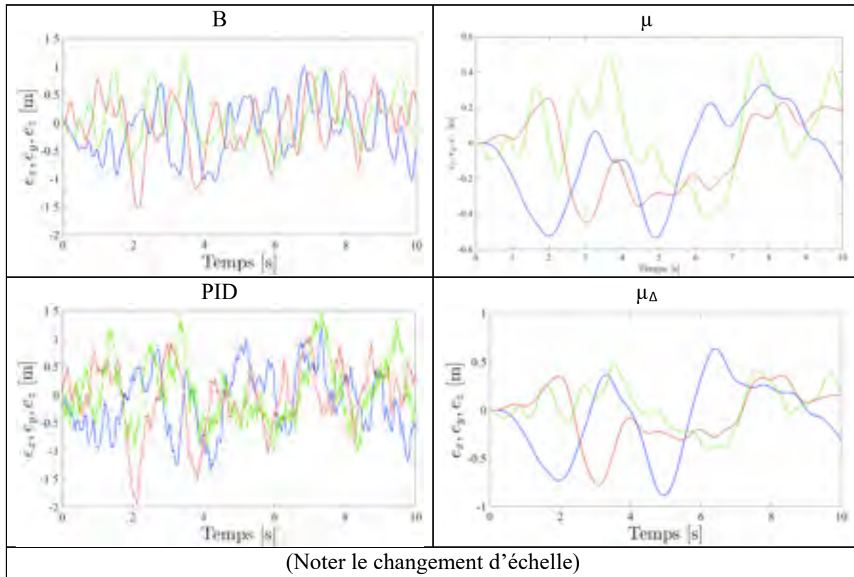
Figure 7.83 Erreurs e_x (bleue), e_y (rouge), e_z (verte) lors d'un vol stationnaire en présence de vent pour les compensateurs B, \mu , \mu_\Delta , PID appliqués sur le modèle linéaire de drone
