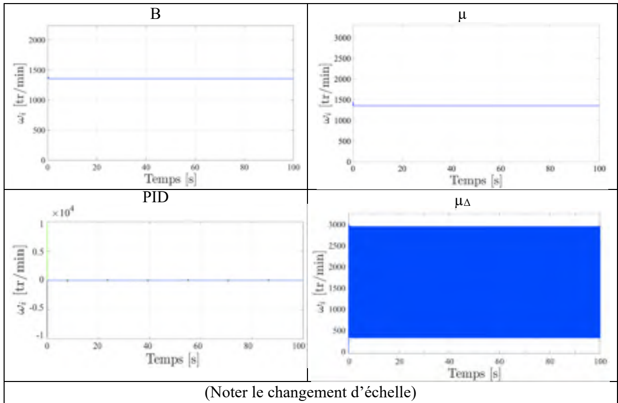
Figure 7.65 Vitesses \omega_1 (noire), \omega_2 (rouge), \omega_3 (verte), \omega_4 (bleue) lors d'une consigne hélicoïdale définie en (7.4), pour les compensateurs B, \mu , PID, \mu_\Delta
