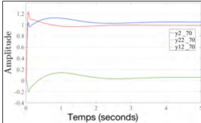
Figure 4.29 Allure de y_2(t) , y_{12}(t) et y_{22}(t) optimisées pour C_{max} = 70 dB
