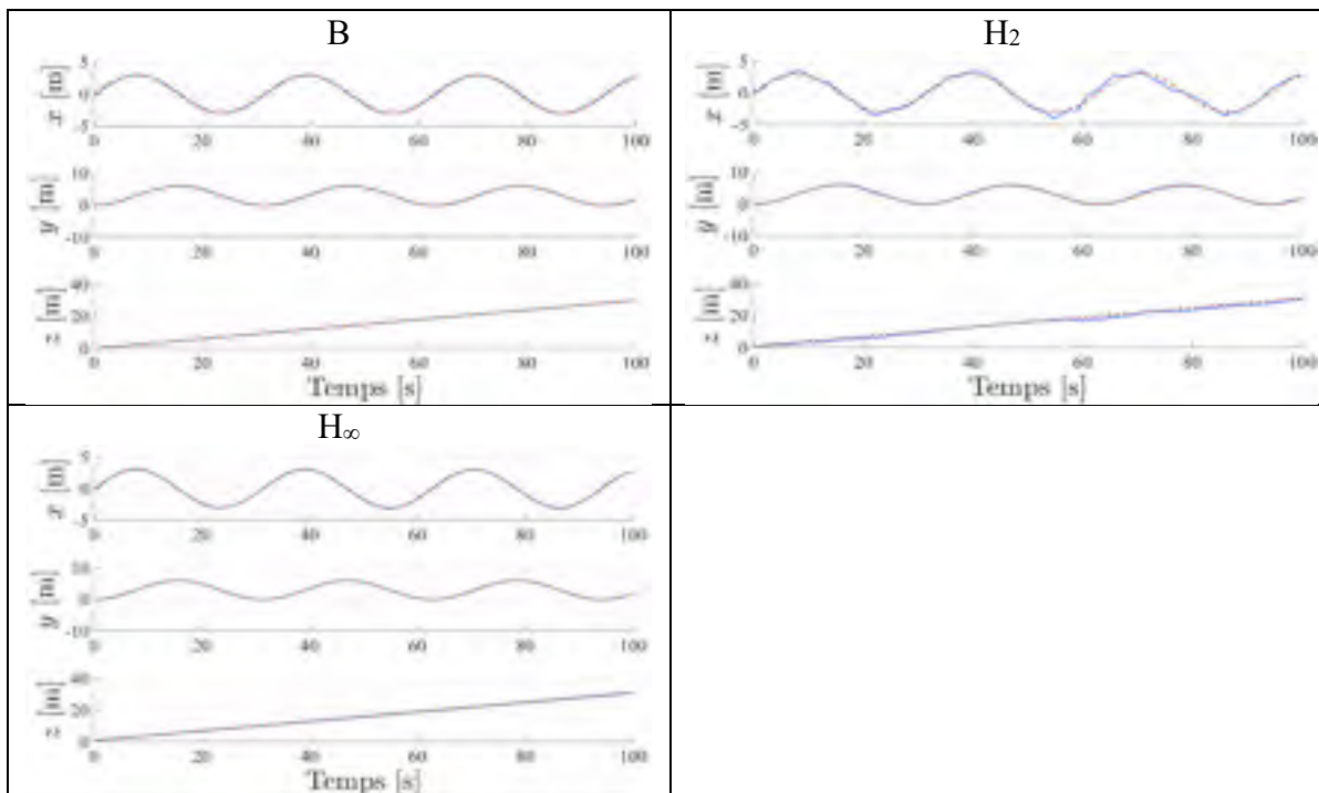
Figure 7.116 Variations des axes x , y , z pour une consigne hélicoïdale définie en (7.4), avec perturbation en sortie pour les compensateurs B, H_2 , H_\infty sur le processus non linéaire
