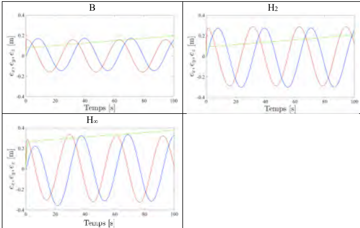
Figure 7.45 Erreurs e_x (bleue), e_y (rouge), e_z (verte) lors d'une consigne hélicoïdale définie en (7.4), pour les compensateurs : B, H 2 , H ∞
