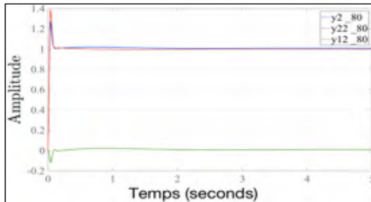
Figure 4.44 Réponse temporelle de y_2(t) , y_{22}(t) et y_{12}(t) pour C_{max} = 80 dB, dans le cas sans erreur statique
