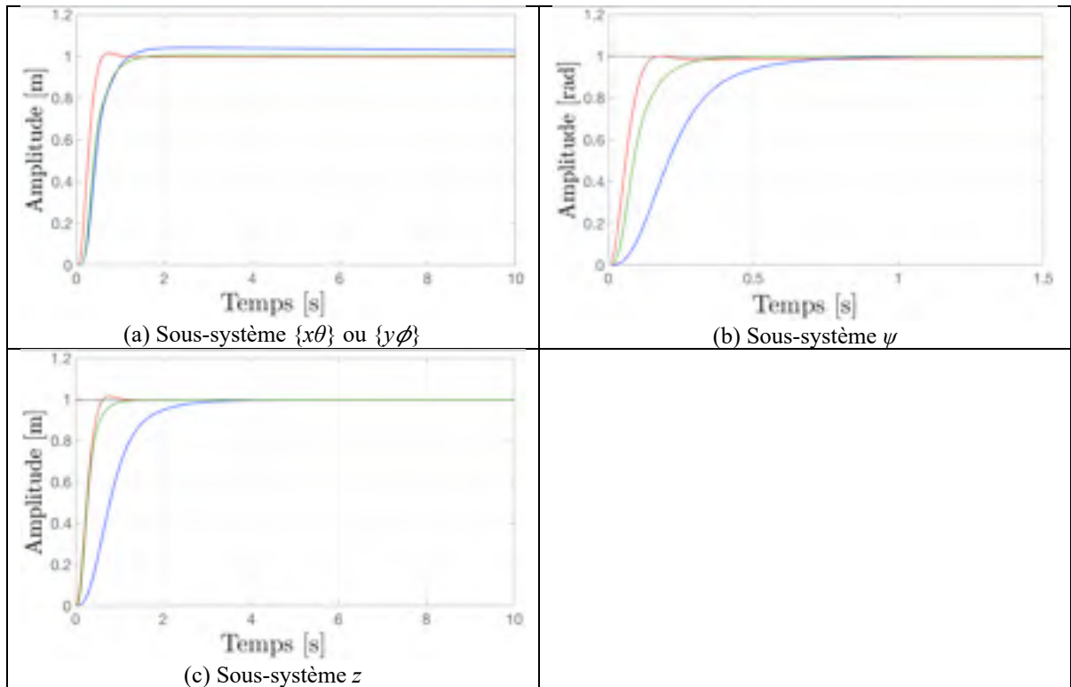
Figure 7.11 Réponse unitaire y(t) pour les compensateurs B (rouge), H_2 (vert) et H_\infty (bleu) sur le processus linéaire
