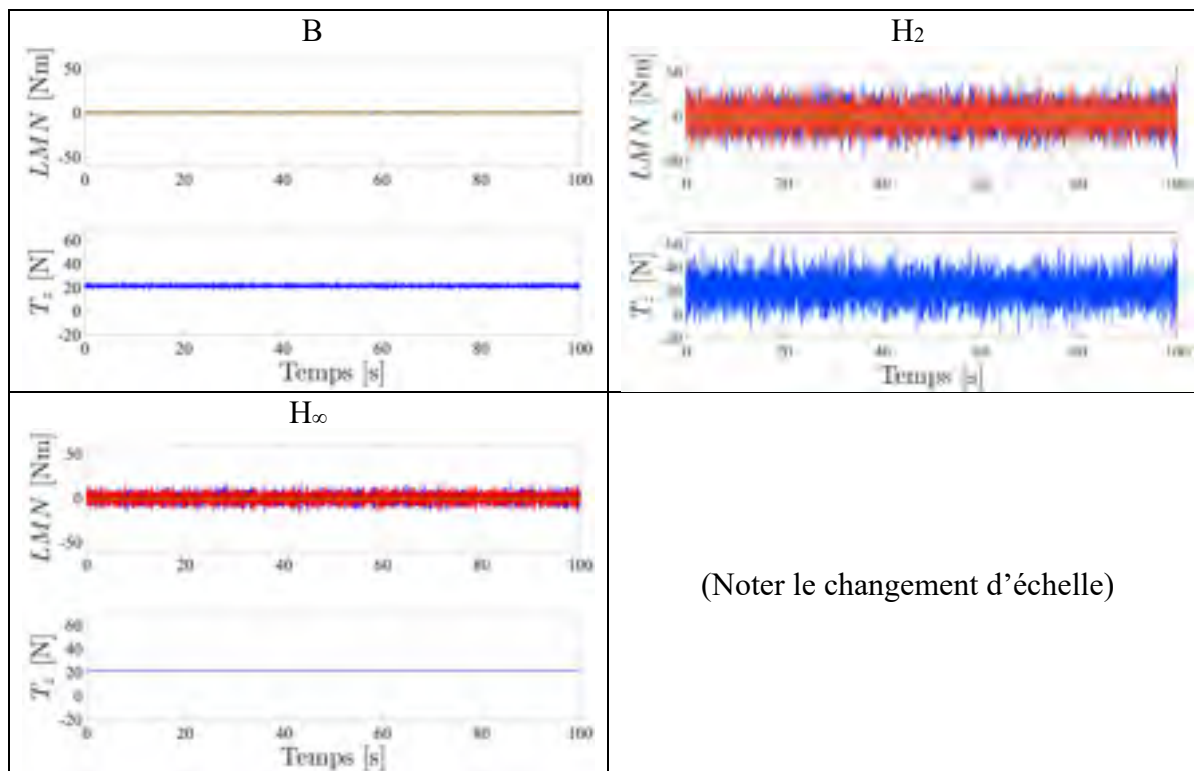
Figure 7.88 Commandes L , M , N , T_z lors d'un vol stationnaire en présence de vent pour les compensateurs B, H_2 , H_\infty appliqués sur le modèle non linéaire de drone
