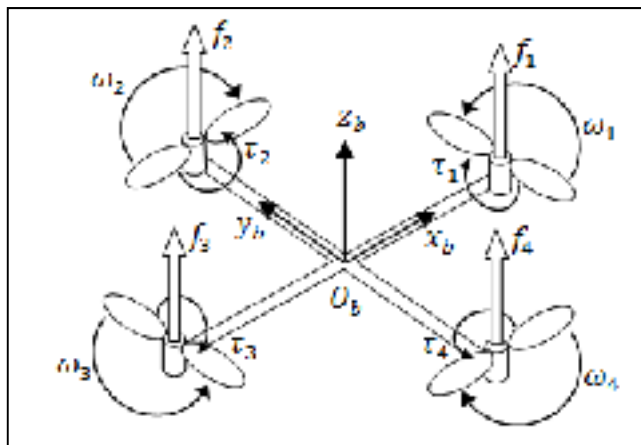
Figure 3.7 Représentation des forces, des vitesses des moteurs du quadricoptère et des couples agissant sur le quadricoptère
