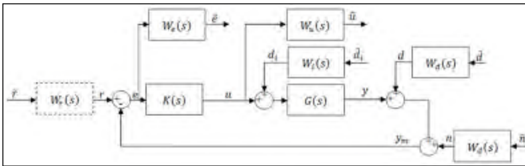
Figure 5.6 Boucle fermée standard avec fonctions de pondérations
