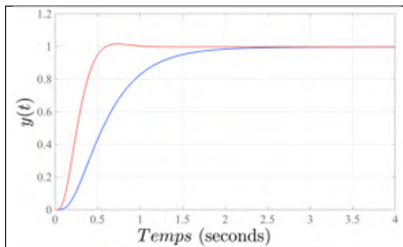
Figure 7.154 Réponses à un échelon sur x ou y pour le compensateur B (rouge) et le compensateur B_u (bleu)
