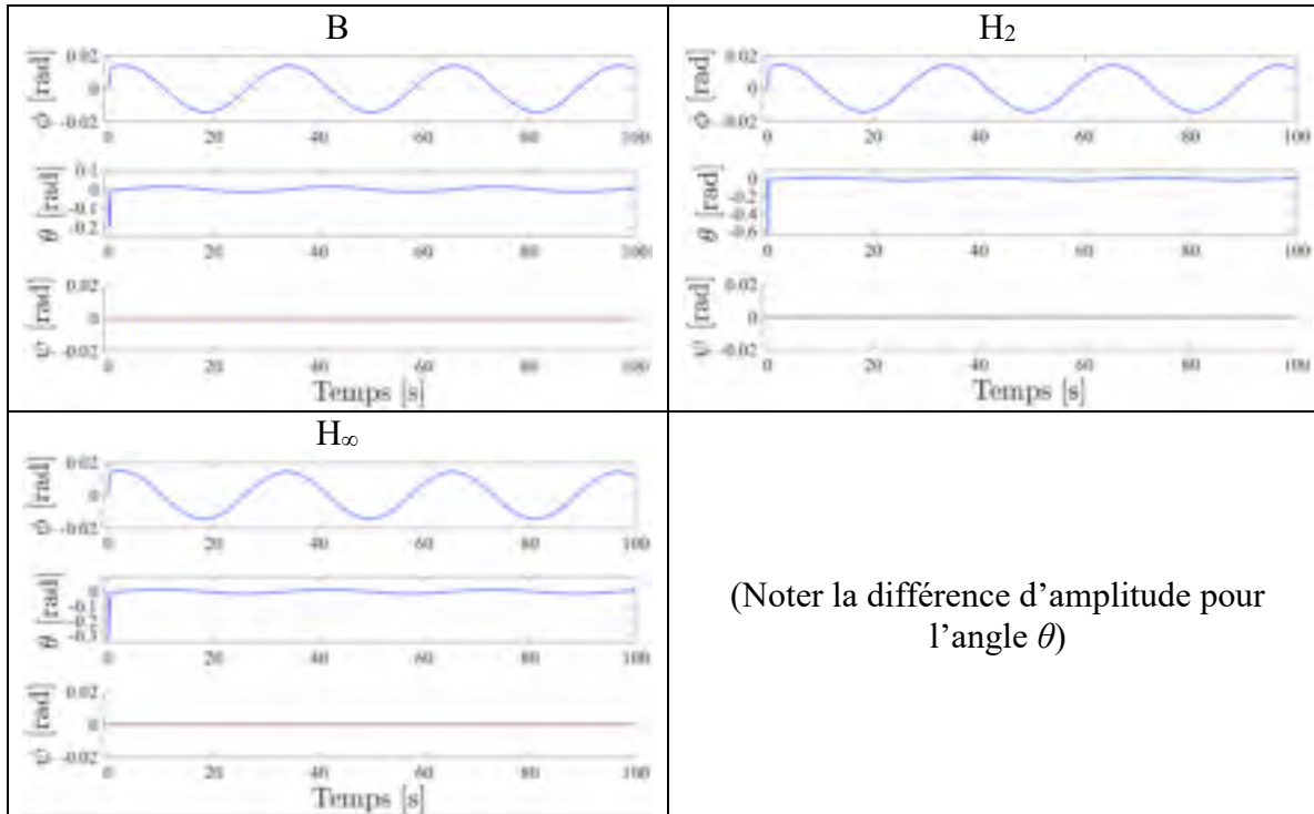
Figure 7.56 Déplacements des angles \phi , \theta , \psi lors d'une consigne hélicoïdale définie en (7.4), pour les compensateurs : B, H_2 , H_\infty
