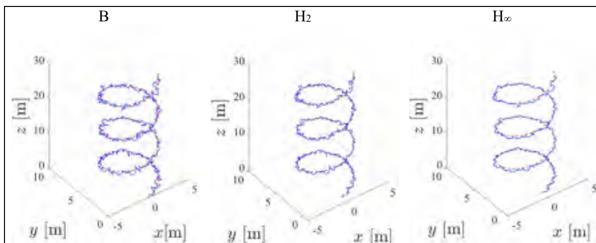
Figure 7.103 Déplacements en bleu sur les axes x , y , z lors d'une consigne hélicoïdale en pointillé rouge définie en (7.4), en présence de vent pour les compensateurs B, H_2 , H_\infty sur le processus linéaire
