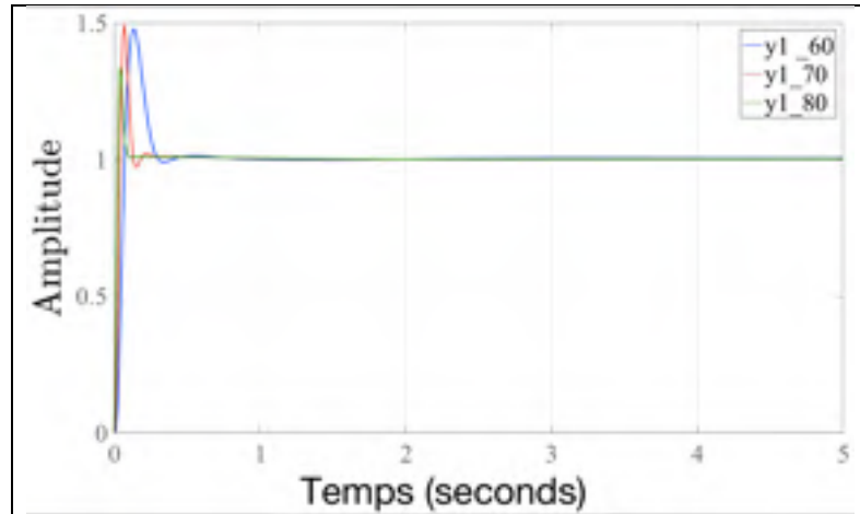
Figure 4.37 Réponse temporelle de y_1(t) pour C_{max} = \{60, 70, 80\} dB, dans le cas sans erreur statique
