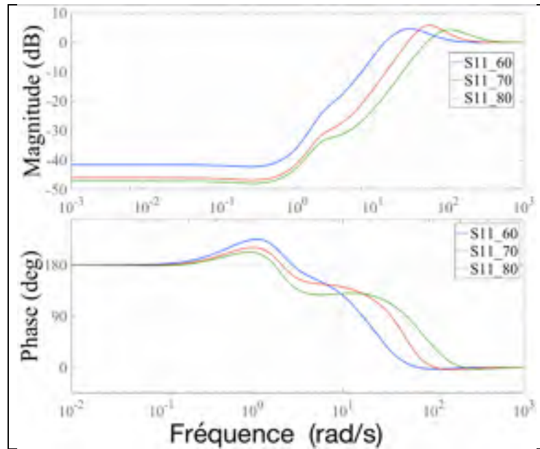
Figure 4.35 Bode de S_{11}(s) pour C_{max} = \{60, 70, 80\} dB, dans le cas sans erreur statique
