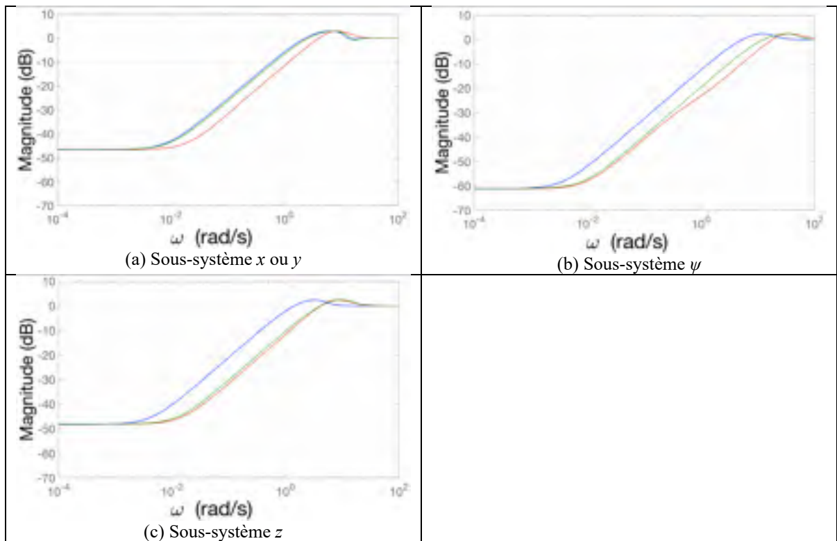
Figure 7.6 Diagramme de Bode du gain de la sensibilité S_{ey}(s) sur les axes x ou y (a), z (c) et autour de l'angle \psi (b) avec les compensateurs B (rouge), H_2 (vert) et H_\infty (bleu)
