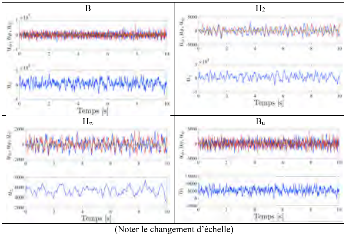
Figure 7.158 Commandes u_\phi (bleue), u_\theta (rouge), u_\psi (verte), u_z lors d'un vol stationnaire en présence de perturbation en sortie pour les compensateurs B, H_2 , H_\infty , B_u appliqués sur le modèle linéaire de drone
