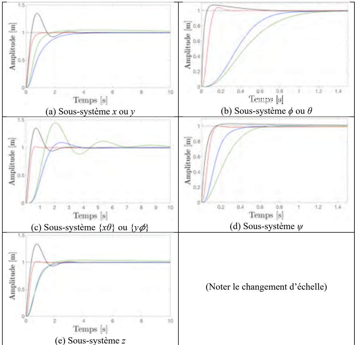
Figure 7.12 Réponse unitaire y(t) pour les compensateurs B (rouge), \mu (bleu), \mu_{\Delta} (vert) et PID (bleu) sur le processus linéaire
