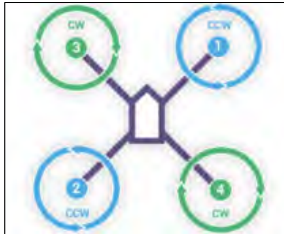
Figure 8.24 Configuration en X du quadricoptère F450J, emplacement et sens de rotation des moteurs 36
