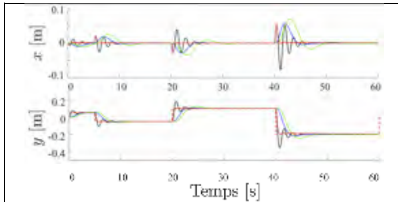
Figure 7.38 Réponses temporelles sur x , y pour le scénario de référence y_d en pointillé rouge et défini en (7.3), avec les compensateurs : B (rouge), \mu (bleu), \mu_\Delta (vert), PID (noir)
