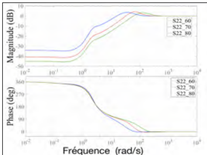
Figure 4.22 Bode de S_{22}(s) pour C_{max} = 60, 70 et 80 dB dans le cas avec erreur statique
