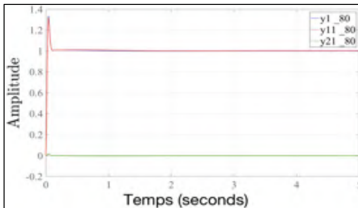
Figure 4.41 Réponse temporelle de y_1(t) , y_{11}(t) et y_{21}(t) pour C_{max} = 80 dB, dans le cas sans erreur statique
