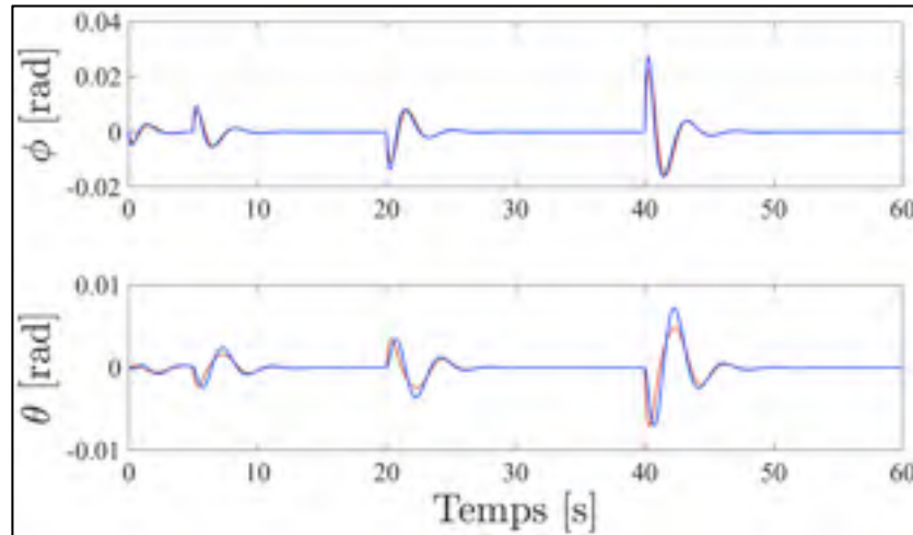
Figure 7.41 Réponses temporelles sur les angles \phi et \theta pour le scénario de référence y_d défini en (7.3) pour les compensateurs : backstepping (rouge) et hiérarchique (bleu)
