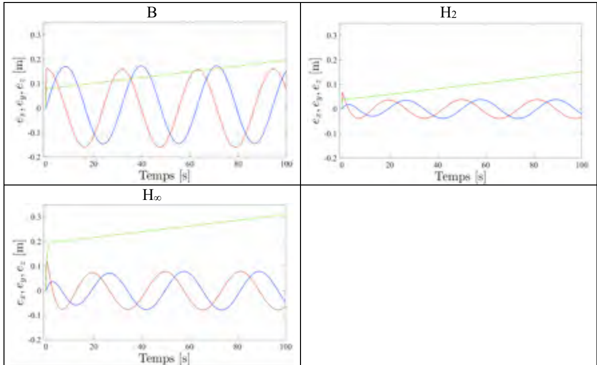
Figure 7.57 Erreurs e_x (bleue), e_y (rouge), e_z (verte) lors d'une consigne hélicoïdale définie en (7.4), pour les compensateurs : B, H_2 , H_\infty
