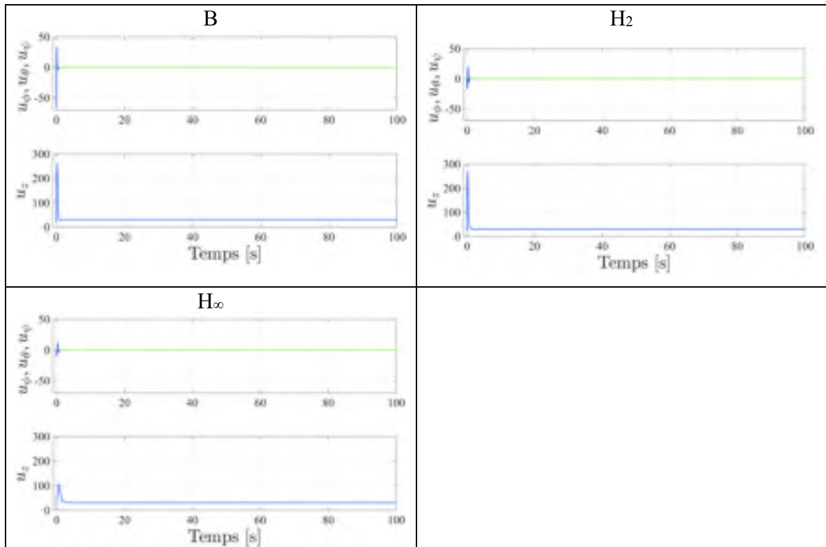
Figure 7.46 Commandes u_\phi (bleue), u_\theta (rouge), u_\psi (verte), u_z lors d'une consigne hélicoïdale définie en (7.4), pour les compensateurs : B, H_2 , H_\infty
