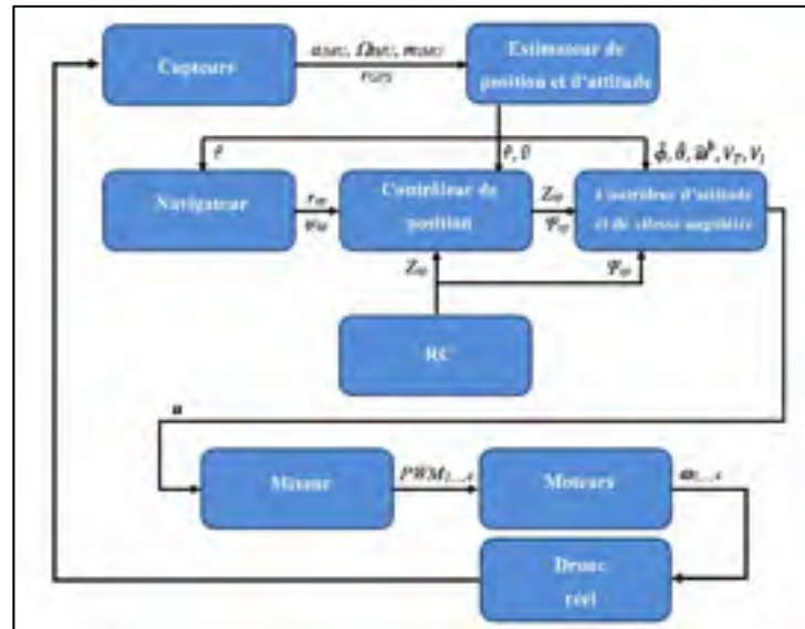
Figure 8.19 Aperçue de la "flight stack" Extrait et adaptée du site de développement du PX4 30
