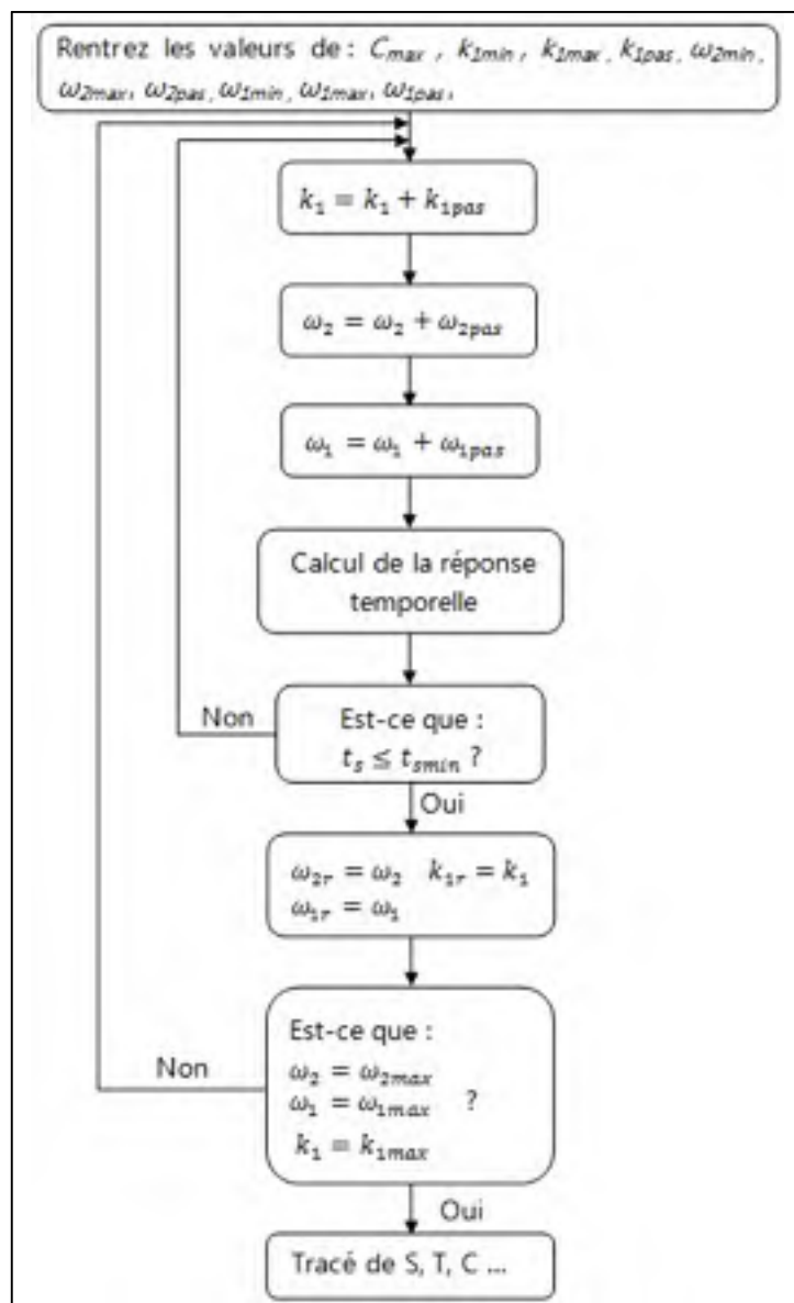
Figure 4.10 Organigramme du programme Matlab pour trouver les paramètres de C(s) avec erreur statique
