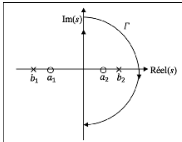
Figure 2.6 Pôles et zéros dans le plan de s
