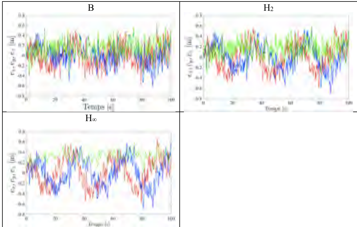
Figure 7.106 Erreurs e_x (bleue), e_y (rouge), e_z (verte) lors d'une consigne hélicoïdale en pointillé rouge et définie en (7.4), en présence de perturbation en sortie pour les compensateurs B, H 2 , H ∞ sur le processus linéaire
