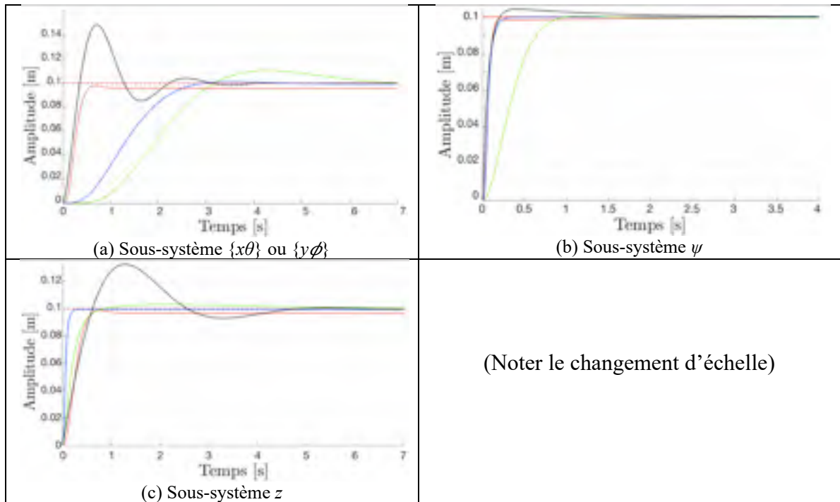
Figure 7.14 Réponse unitaire y(t) pour les compensateurs B (rouge), \mu (bleu), \mu_{\Delta} (vert) et PID (bleu) sur le processus non linéaire
