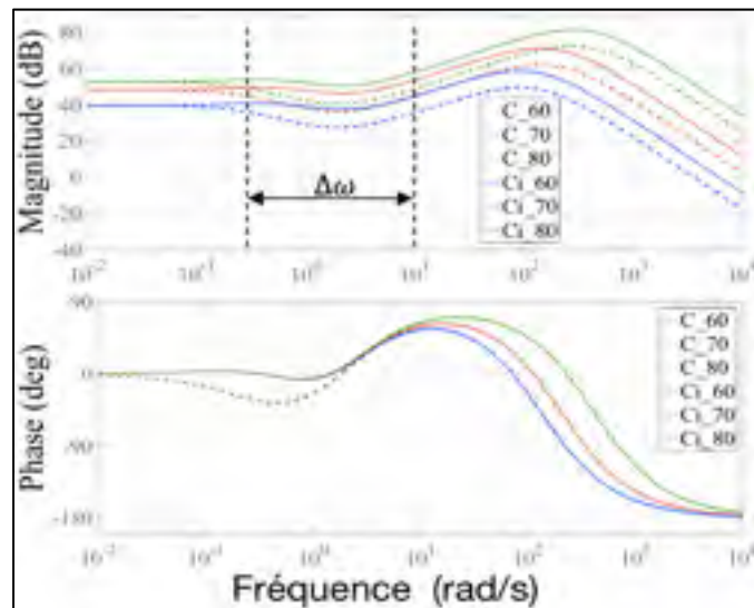
Figure 4.15 Comparaison de C(s) avec et sans F_{inter} pour trois valeurs de k_1
