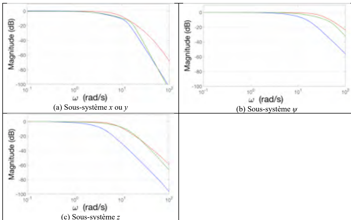
Figure 7.4 Diagramme de Bode du gain de la transmission T(s) sur les axes x ou y (a), z (c) et autour de l'angle \psi (b) avec les compensateurs B (rouge), H_2 (vert) et H_\infty (bleu)
