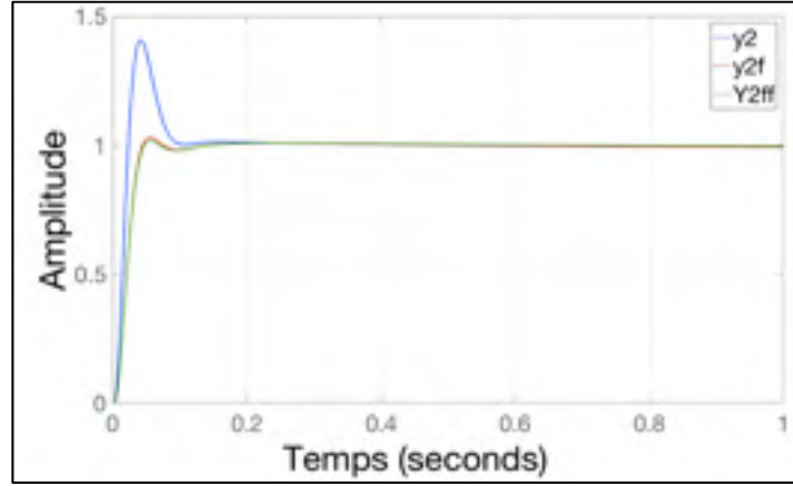
Figure 4.57 Réponse indicielle de y_2(t) , y_{2f}(t) et y_{2ff}(t)
