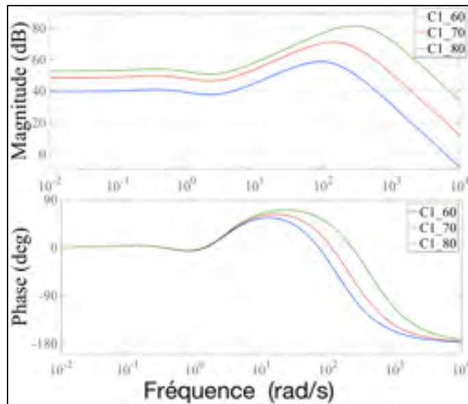
Figure 4.18 Allure de C(s) optimisé pour C_{max} = 60, 70 et 80 dB
