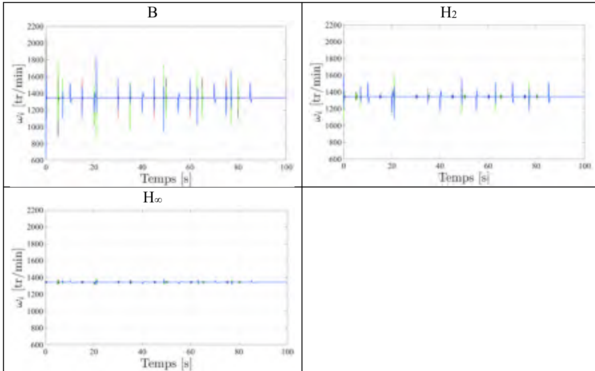
Figure 7.19 Vitesses \omega_1 (noire), \omega_2 (rouge), \omega_3 (verte), \omega_4 (bleue) pour le scénario de référence défini en (7.2), avec les compensateurs B, H_2 , H_\infty sur le processus linéaire
