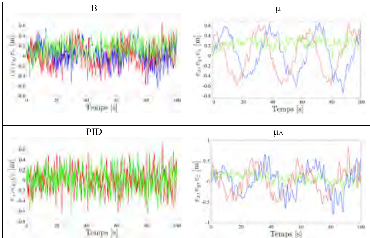
Figure 7.112 Erreurs e_x (bleue), e_y (rouge), e_z (verte) lors d'une consigne hélicoïdale définie en (7.4), en présence de perturbation en sortie pour les compensateurs B, \mu , \mu_\Delta , PID sur le processus linéaire
