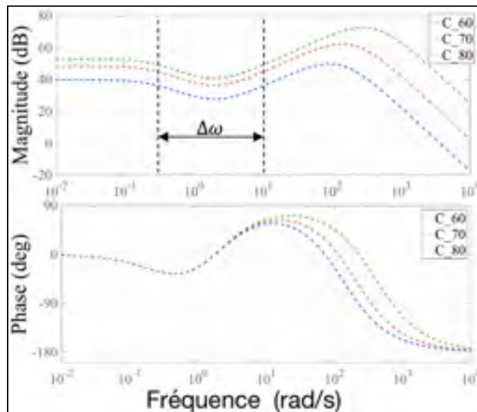
Figure 4.13 Allure du compensateur C(s) pour trois valeurs de k_1
