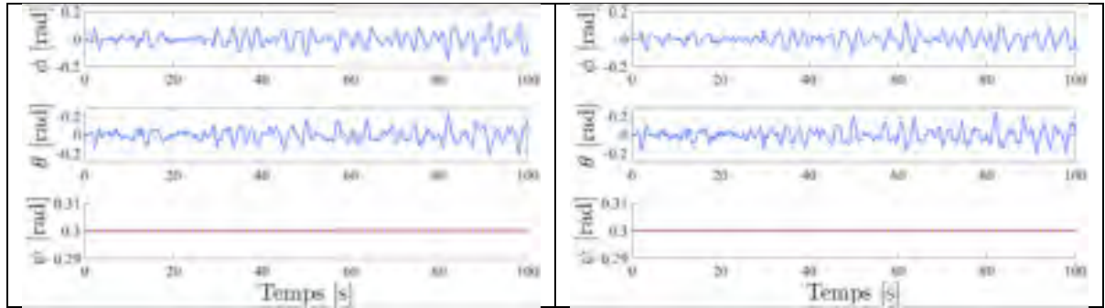
Figure 7.99 Déplacements autour des angles \phi , \theta , \psi lors d'un vol stationnaire en présence de perturbation en sortie pour les compensateurs backstepping et hiérarchique
