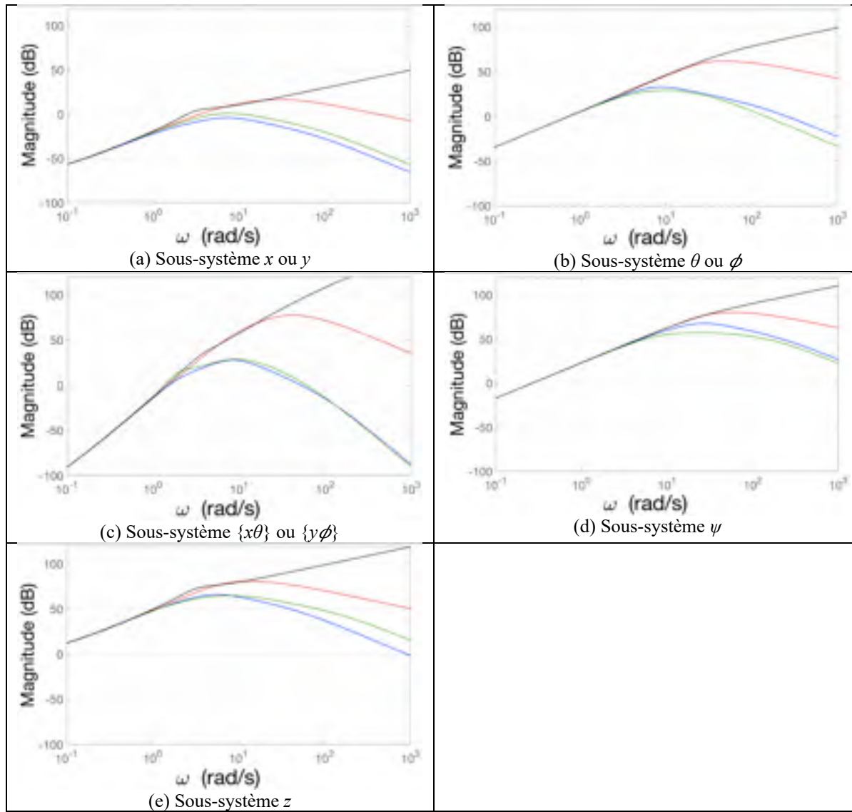
Figure 7.9 Sensibilité S_{du}(s) sur les axes x ou y (a), \{x\theta\} ou \{y\phi\} (c), z (e) et autour des angles \theta ou \phi (b), \psi (d) pour les compensateurs B (rouge), \mu (bleu), \mu_\Delta (vert) et PID (noir)
