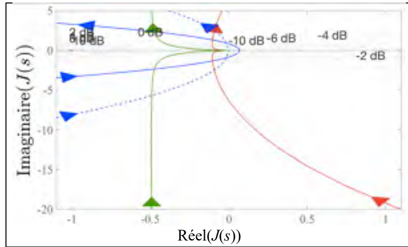
Figure 8.34 Nyquist de la boucle ouverte J(s) pour les compensateurs : PID _{\phi} (bleu) ; B (rouge) ; B amélioré (vert)
