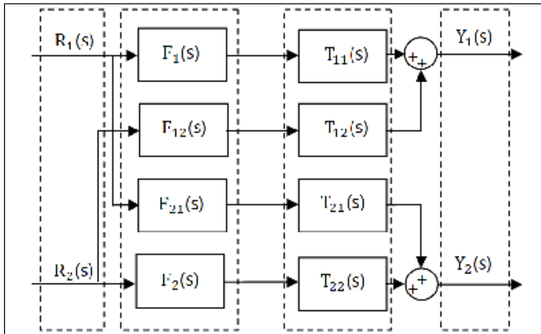
Figure 4.53 Représentation sous forme de schéma bloc du système multivariable, avec un préfiltre associé à chacune des transmittances
