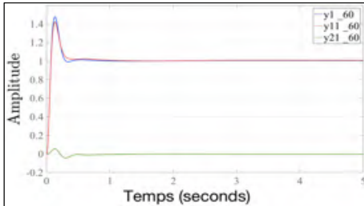
Figure 4.39 Réponse temporelle de y_1(t) , y_{11}(t) et y_{21}(t) pour C_{max} = 60 dB, dans le cas sans erreur statique
