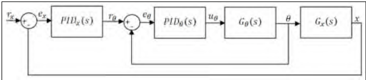
Figure 5.4 Structure PID double boucle pour la commande de \theta et x
