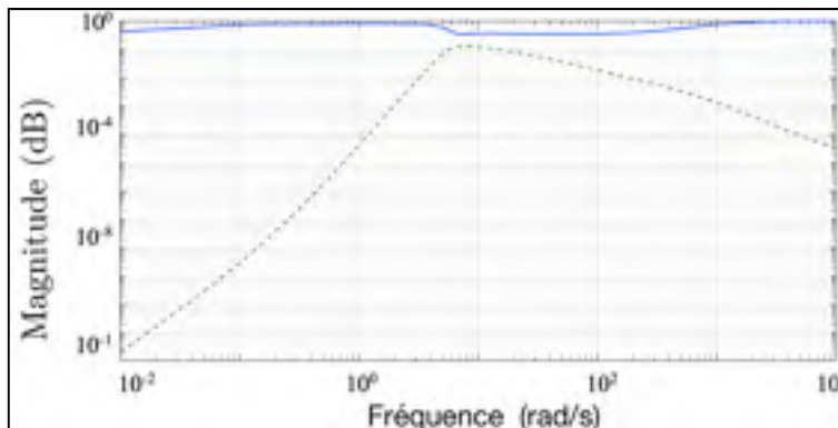
Figure 5.32 Stabilité robuste \|M_{d \rightarrow \tilde{u}}\|_{\infty} en pointillé vert et robuste performance \mu_{\tilde{Z}_p}(M(j\omega)) courbes rouge et bleue (superposées) pour les axes x - y , avec incertitudes
