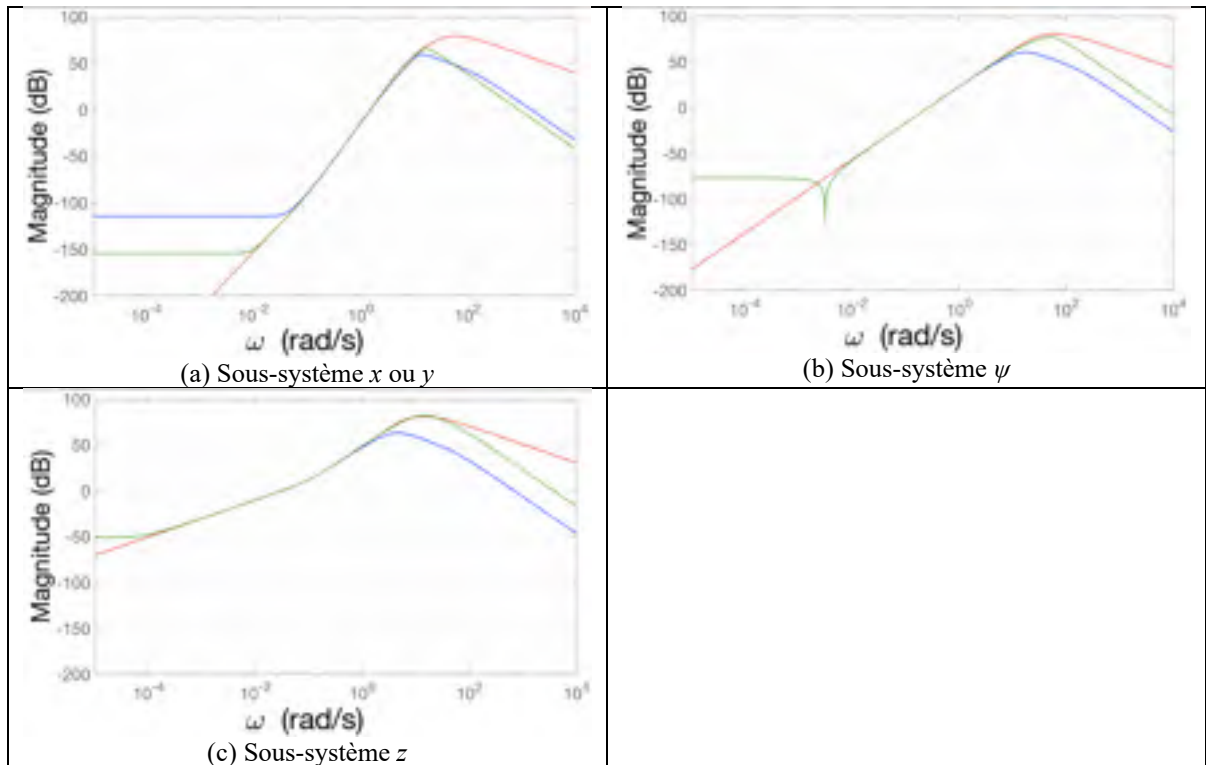
Figure 7.8 Sensibilité S_{du}(s) sur les axes x ou y (a), z (c) et autour de l'angle \psi (b) pour les compensateurs B (rouge), H_2 (vert) et H_\infty (bleu)
