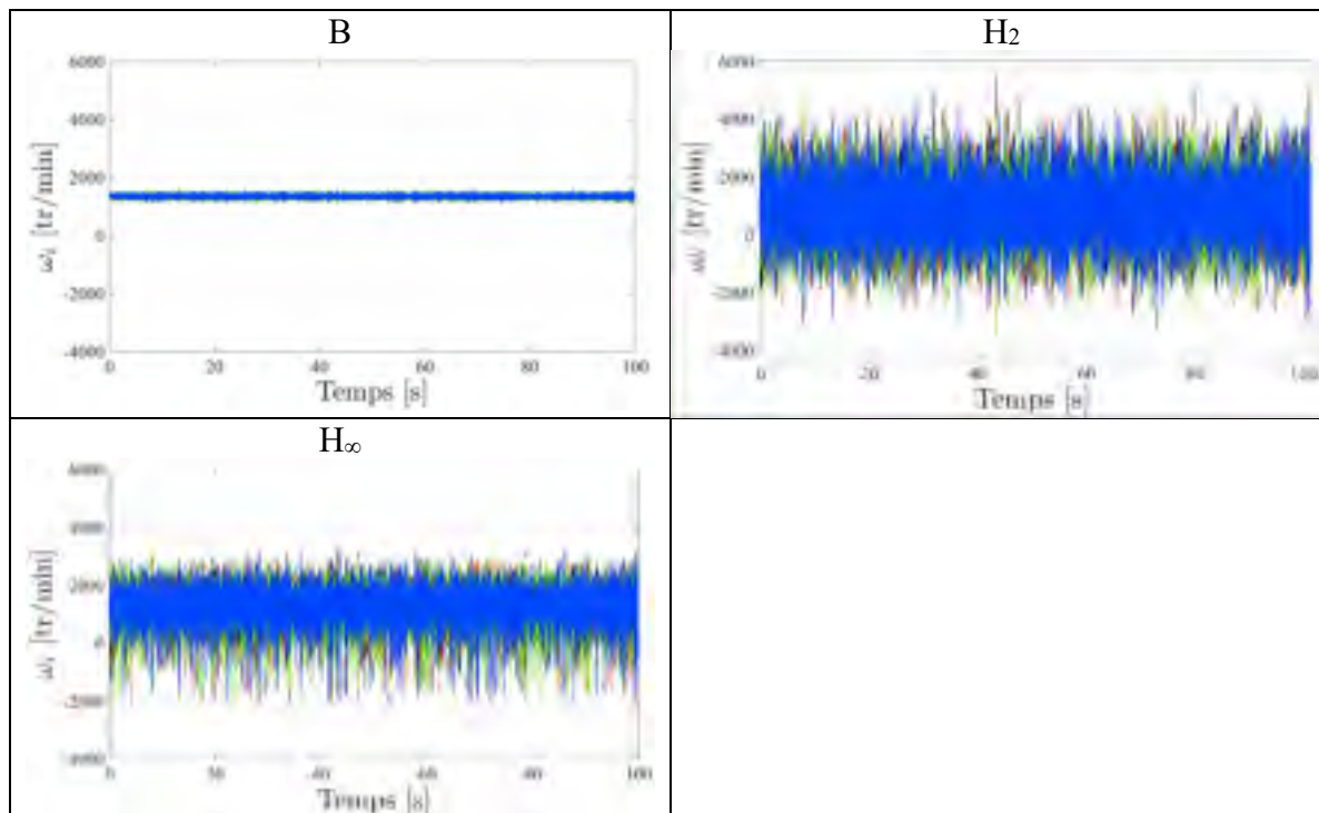
Figure 7.120 Vitesses \omega_1 (noire), \omega_2 (rouge), \omega_3 (verte), \omega_4 (bleue) lors d'une consigne hélicoïdale définie en (7.4), en présence de perturbation en sortie pour les compensateurs B, H 2 , H ∞ sur le processus non linéaire
