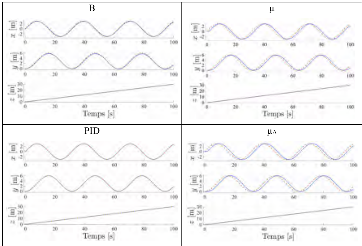
Figure 7.61 Déplacement sur x , y , z lors d'une consigne hélicoïdale définie en (7.4), pour les compensateurs : B, \mu , PID, \mu_{\Delta}
