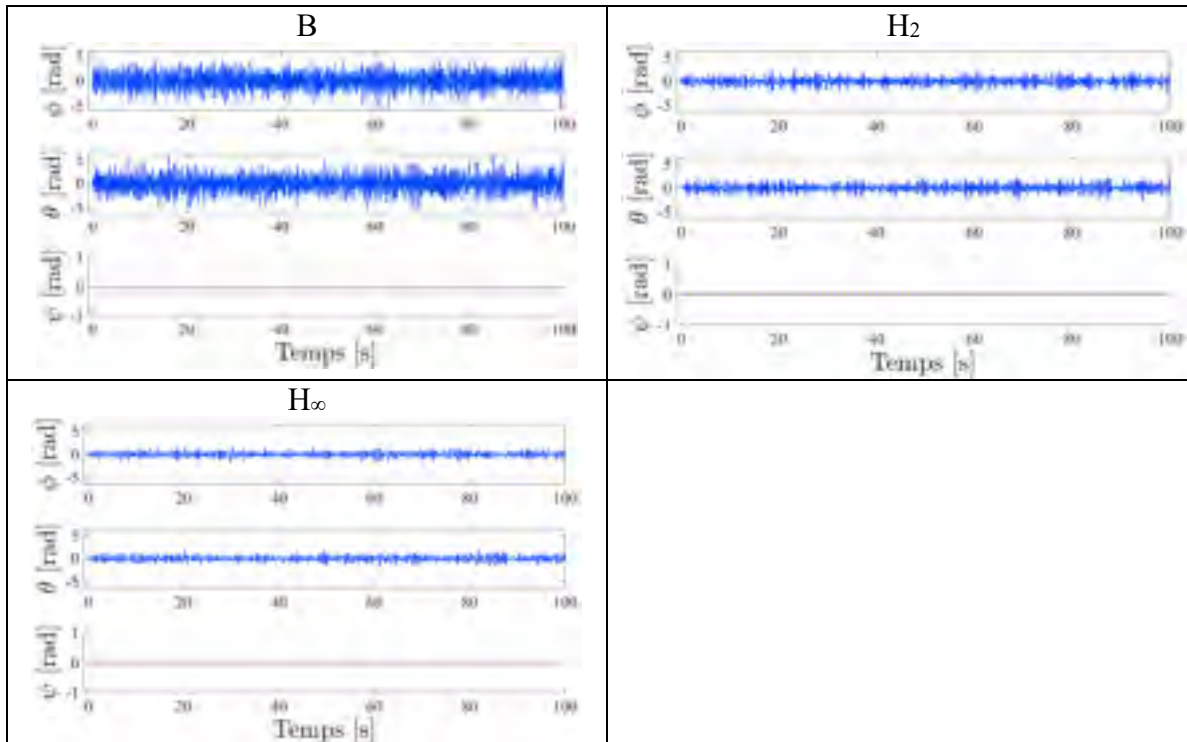
Figure 7.105 Déplacement des angles \phi, \theta, \psi lors d'une consigne hélicoïdale en pointillé rouge définie en (7.4), en présence de perturbation en sortie pour les compensateurs B, H_2 , H_\infty sur le processus linéaire
