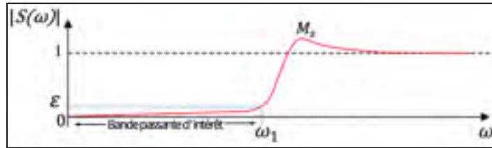
Figure 4.1 Allure fréquentielle de la sensibilité Tirée et reproduite de Garnier (2007)
