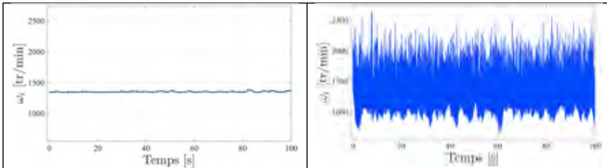
Figure 7.102 Vitesses \omega_1 (noire), \omega_2 (rouge), \omega_3 (verte), \omega_4 (bleue) lors d'un vol stationnaire en présence de perturbation en sortie pour les compensateurs backstepping et hiérarchique
