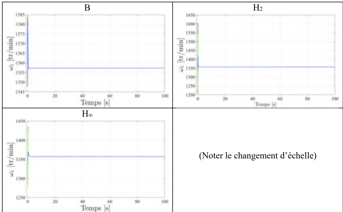
Figure 7.59 Vitesses \omega_1 (noire), \omega_2 (rouge), \omega_3 (verte), \omega_4 (bleue) lors d'une consigne hélicoïdale définie en (7.4), pour les compensateurs : B, H_2 , H_\infty
