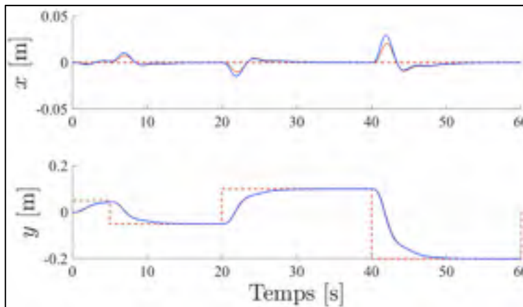
Figure 7.40 Réponses temporelles sur les axes x , y pour le scénario de référence (7.3) y_d en pointillé rouge, avec les compensateurs : backstepping (rouge) ; hiérarchique (bleu)
