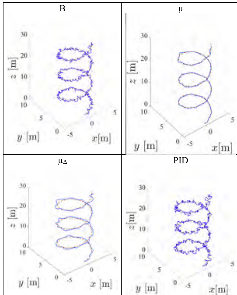
Figure 7.109 Déplacements en 3D sur les axes x , y , z lors d'une consigne hélicoïdale en pointillé rouge et définie en (7.4), en présence de perturbation en sortie pour les compensateurs B, \mu , \mu_{\Delta} , PID sur le processus linéaire
