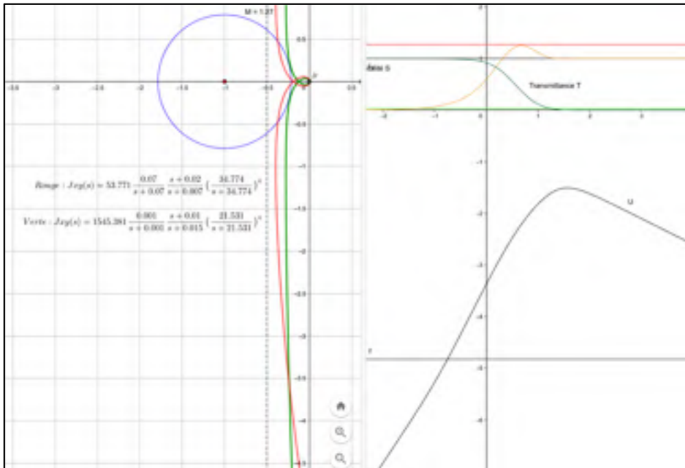
Figure 7.150 Conception de la commande B pour des axes x et y avec GeoGebra avec sur la partie de gauche : la commande B (rouge) ; la commande B_u (vert) ; Cercle de sensibilité S_{ey}(s) (bleu). À droite pour le compensateur B_u uniquement : Sensibilité S_{ey}(s) (jaune) ; Transmittance T(s) (verte foncée) ; \epsilon (vert clair) ; M_s (rouge) ; U(s) (noir)
