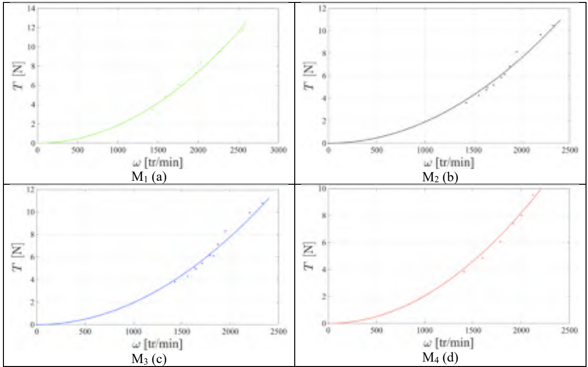
Figure 8.25 T en fonction de \omega , mesures pratiques en pointiller et fonctions approximées x\omega^2 en trait plein pour les moteurs : M 1 (a), M 2 (b), M 3 (c), M 4 (d)
