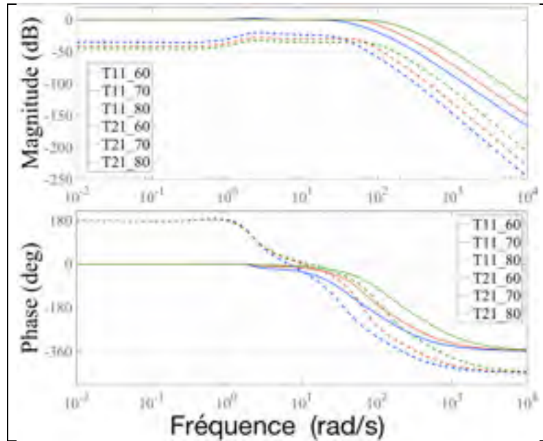
Figure 4.19 Allure de T_{11}(s) et T_{21}(s) optimisées pour C_{max} = 60, 70 et 80 dB
