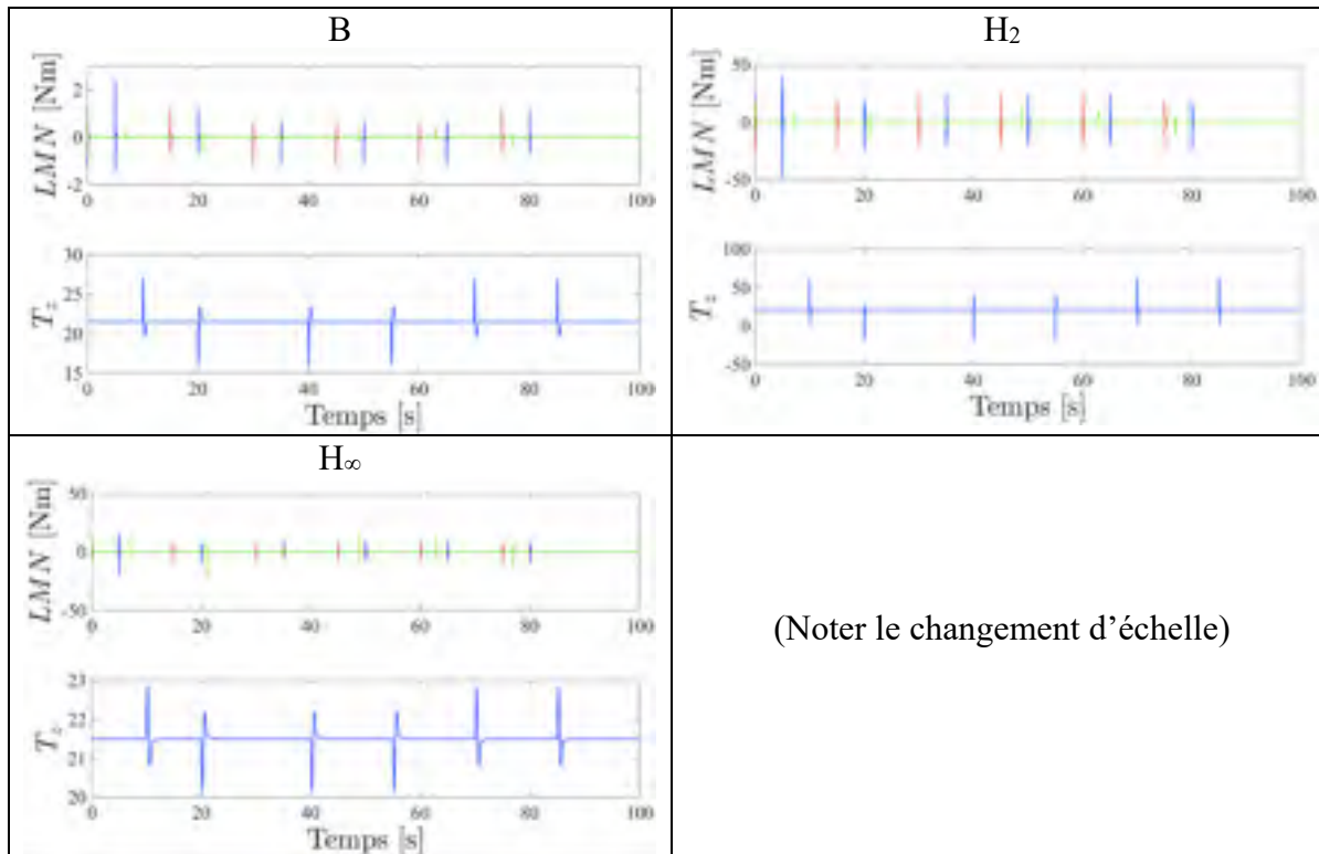
Figure 7.26 Réponses des commandes L , M , N et T_z pour le scénario de référence défini en (7.2), avec les compensateurs B, H_2 , H_\infty sur le processus non linéaire
