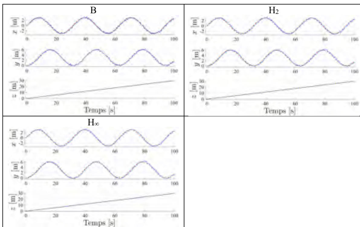
Figure 7.104 Déplacements en bleu sur les axes x , y , z lors d'une consigne hélicoïdale en pointillé rouge et définie en (7.4), en présence de perturbation en sortie pour les compensateurs B, H_2 , H_\infty sur le processus linéaire
