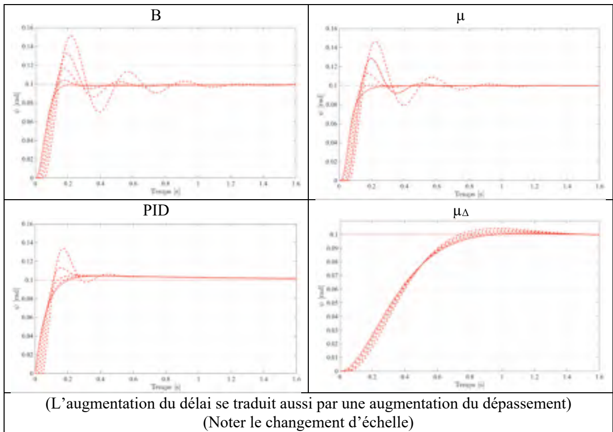
Figure 7.145 Réponses unitaires nominales en trait plein autour de l'angle \psi et en pointillés avec l'ajout de délais de mesure, pour les compensateurs : B, \mu , PID, \mu_\Delta sur le processus non linéaire
