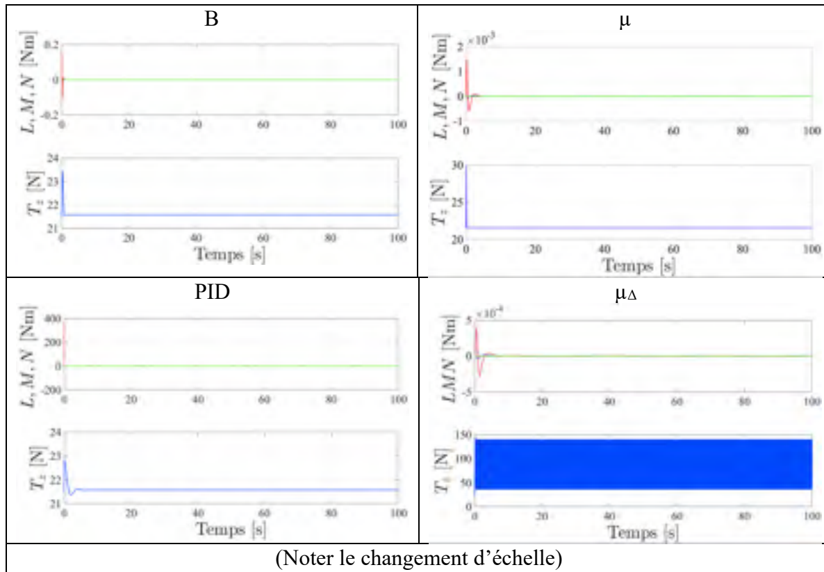
Figure 7.64 Commandes L , M , N , T_z lors d'une consigne hélicoïdale définie en (7.4), pour les compensateurs B , \mu , PID , \mu_\Delta
