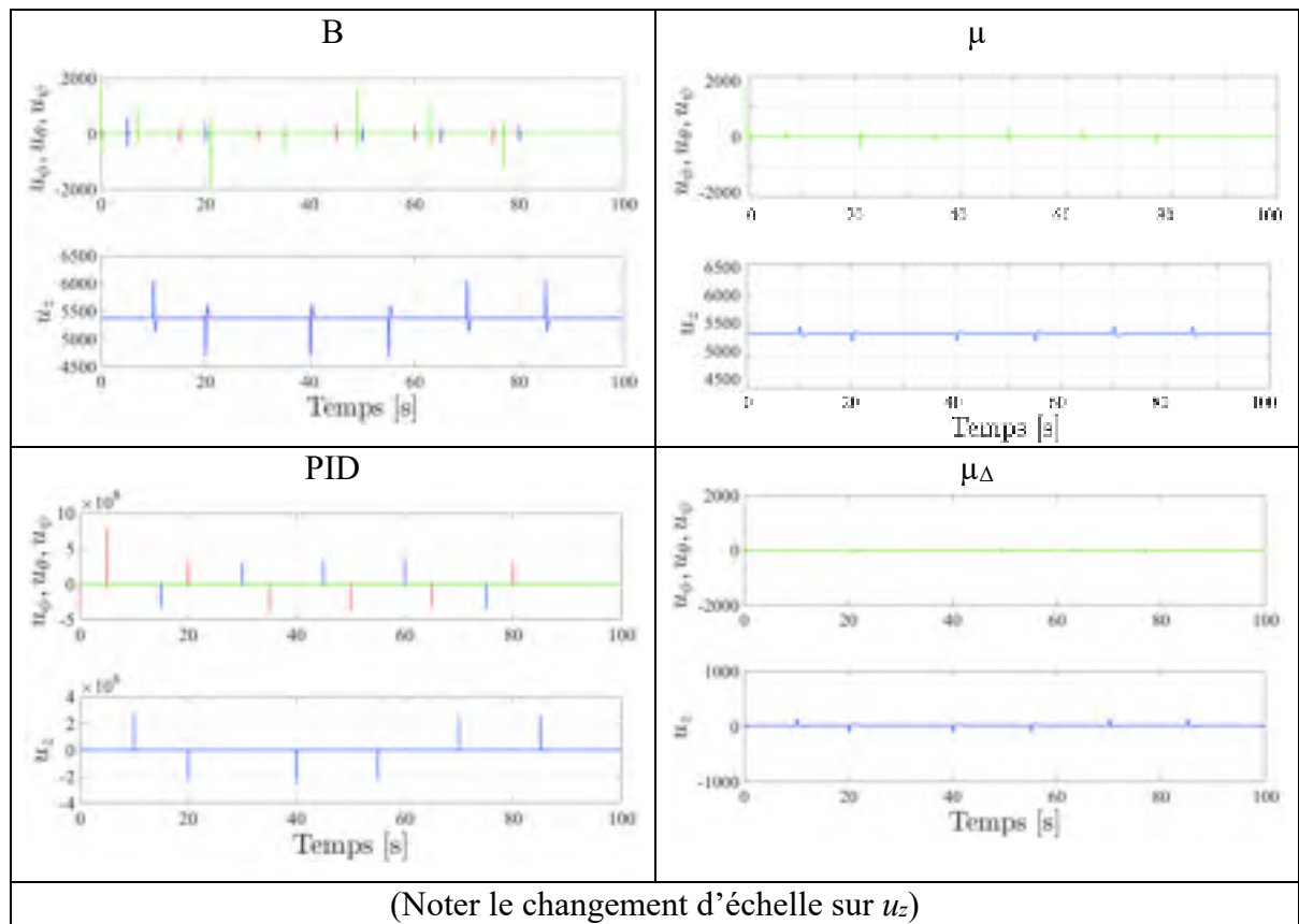
Figure 7.22 Réponses des commandes u_\phi (bleue), u_\theta (rouge), u_\psi (verte) et u_z pour le scénario de référence (7.2), avec les compensateurs B, \mu , PID, \mu_\Delta sur le processus linéaire
