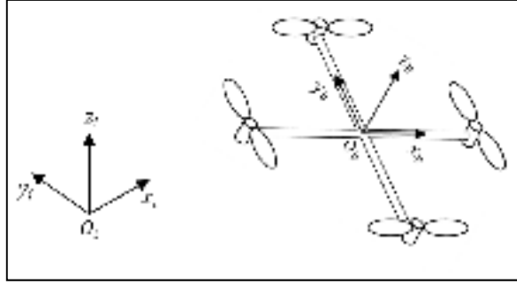
Figure 3.1 Repère inertiel F_i et repère de la base du drone F_b
