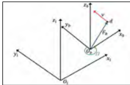
Figure 3.3 Représentation du quadricoptère en un point d
