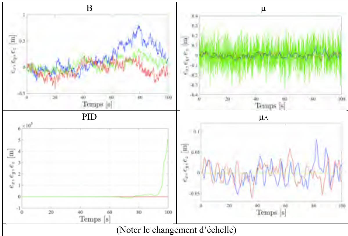
Figure 7.95 Erreurs e_x (bleue), e_y (rouge), e_z (verte) lors d'un vol stationnaire en présence de perturbation en sortie pour les compensateurs B, \mu , \mu\Delta , PID appliqués sur le modèle non linéaire de drone
