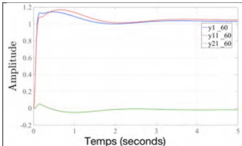
Figure 4.25 Allure de y_1(t) , y_{11}(t) et y_{21}(t) optimisées pour C_{max} = 60 dB
