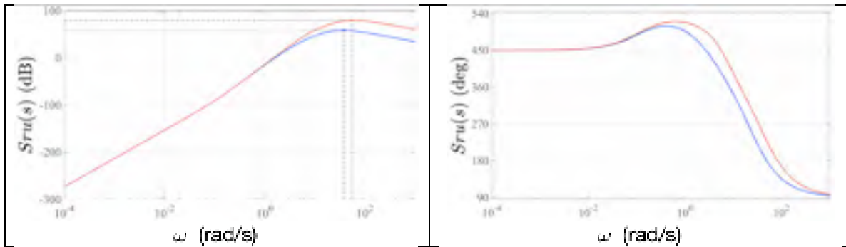
Figure 7.151 Allures de la sensibilité S_{ru}(s) sur x ou y pour le compensateur B (rouge) et le compensateur B_u (bleu). À gauche l'amplitude et à droite la phase
