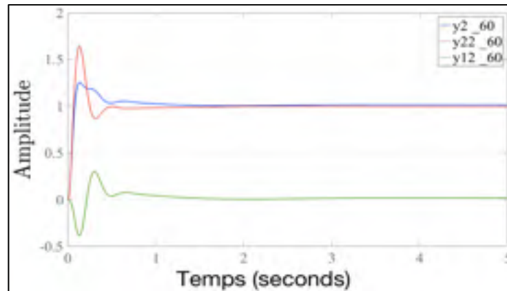
Figure 4.42 Réponse temporelle de y_2(t) , y_{22}(t) et y_{12}(t) pour C_{max} = 60 dB, dans le cas sans erreur statique
