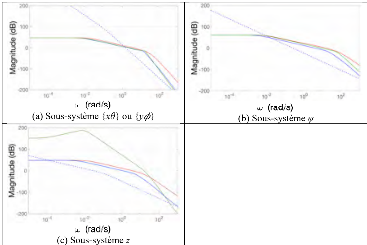
Figure 7.2 Diagramme de Bode de gain de la boucle ouverte J(s) sur les axes \{x\theta\} ou \{y\phi\} (a), z (c) et autour de l'angle \psi (b) pour le système seul (pointillés bleus) et avec compensateurs B (rouge), H_2 (vert) et H_\infty (bleu)
