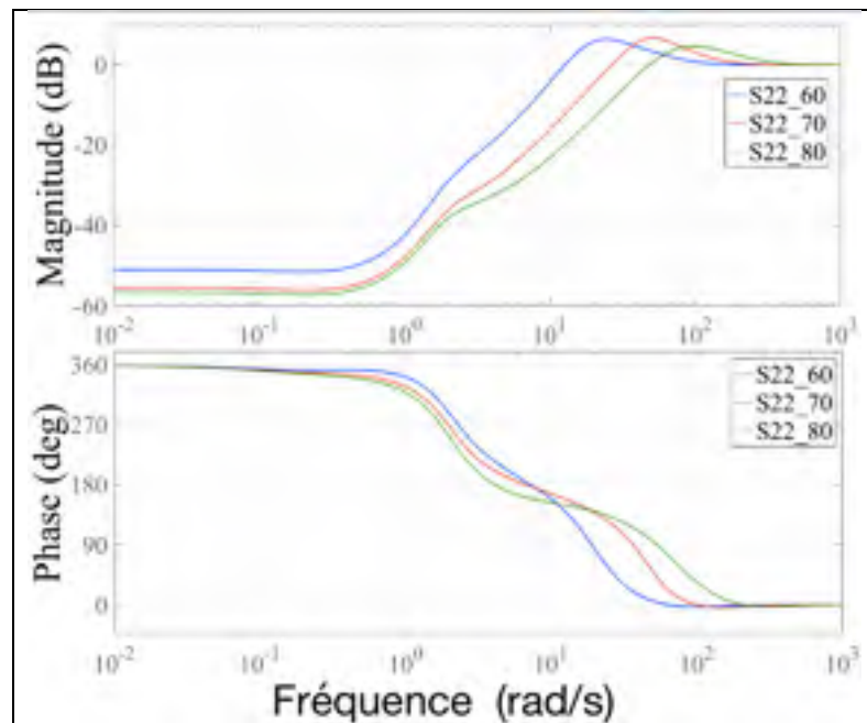
Figure 4.36 Bode de S_{22}(s) pour C_{max} = \{60, 70, 80\} dB, dans le cas sans erreur statique
