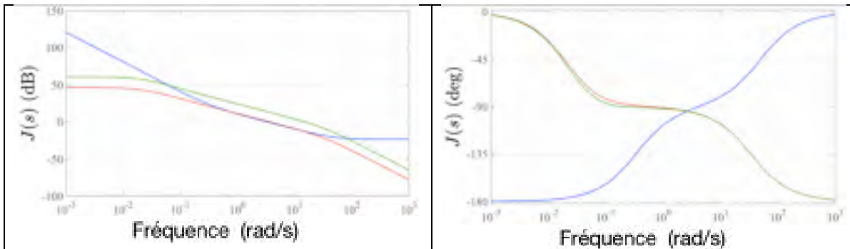
Figure 8.33 Bode de la boucle ouverte J(s) avec à gauche l'amplitude et à droite la phase pour les compensateurs : PID_{\dot{\phi}} (bleu) ; B (rouge) ; B amélioré (vert)
