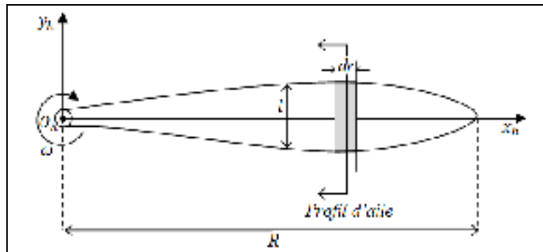
Figure 3.4 Élément infiniment petit dr sur l'hélice
