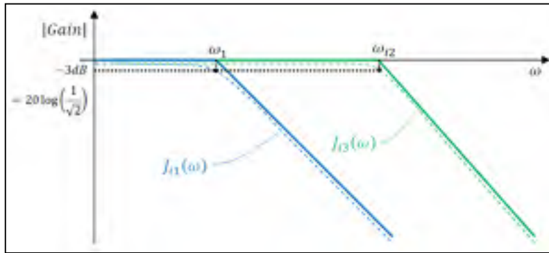
Figure 4.7 Représentation graphique de J_{i1}(\omega) et J_{i3}(\omega)
