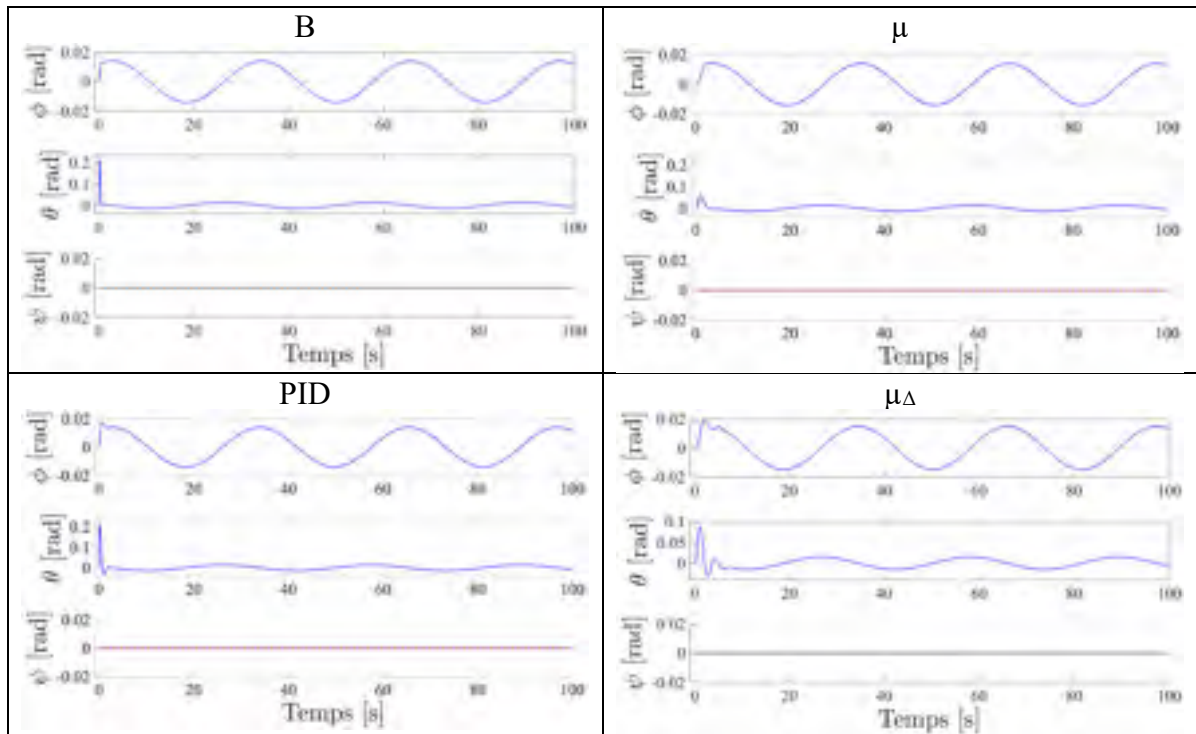
Figure 7.50 Déplacement des angles \phi , \theta , \psi lors d'une consigne hélicoïdale définie en (7.4), pour les compensateurs : B, \mu , PID, \mu_{\Delta}
