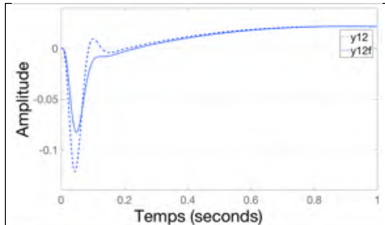
Figure 4.50 Réponse indicielle de y_{12}(t) et y_{12f}(t)
