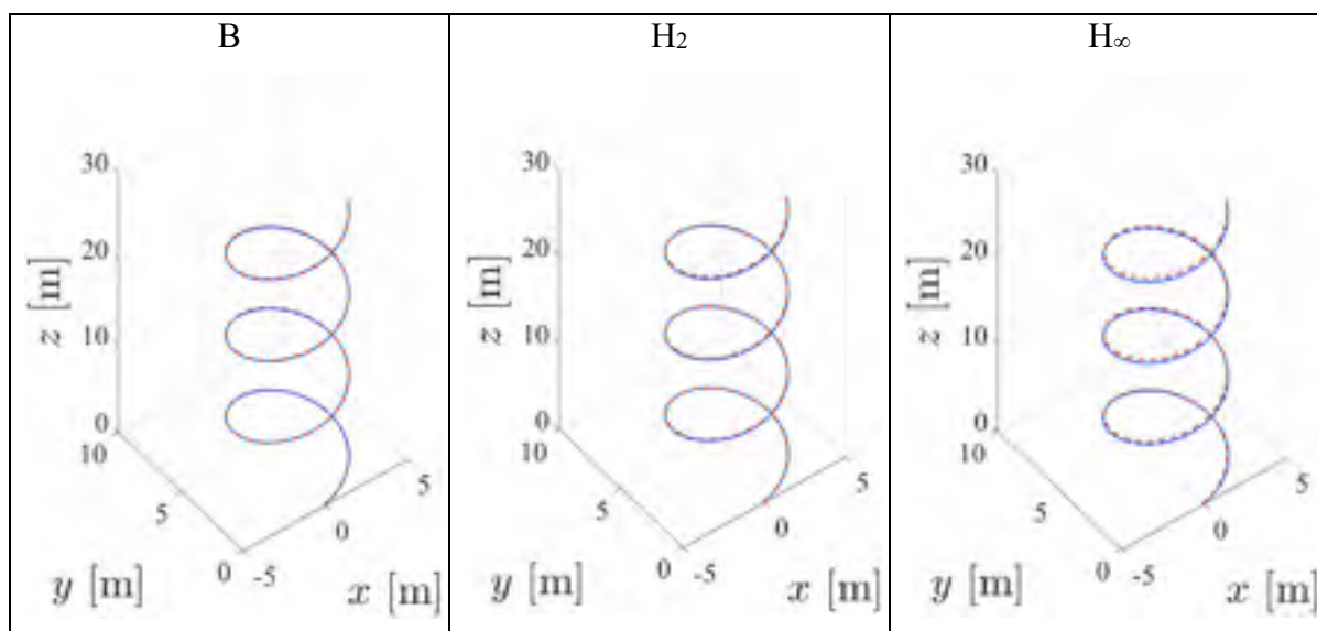
Figure 7.54 Déplacement en 3D sur x, y, z lors d'une consigne hélicoïdale définie en (7.4), pour les compensateurs : B, H_2 , H_\infty
