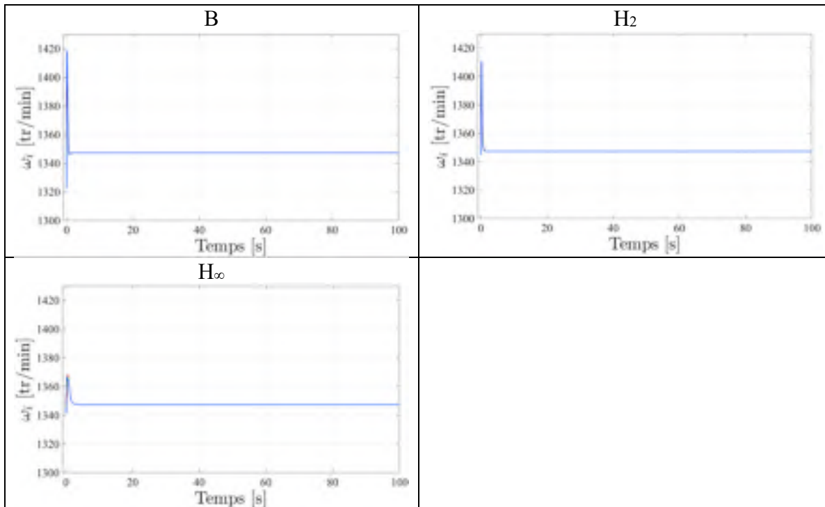
Figure 7.47 Vitesses \omega_1 (noire), \omega_2 (rouge), \omega_3 (verte), \omega_4 (bleue) lors d'une consigne hélicoïdale définie en (7.4), pour les compensateurs : B, H_2 , H_\infty
