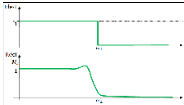
Figure 2.11 Comparaison entre l'allure de la transmittance en fonction de la fréquence, dans le cas idéal (en haut) et dans le réel (en bas)
