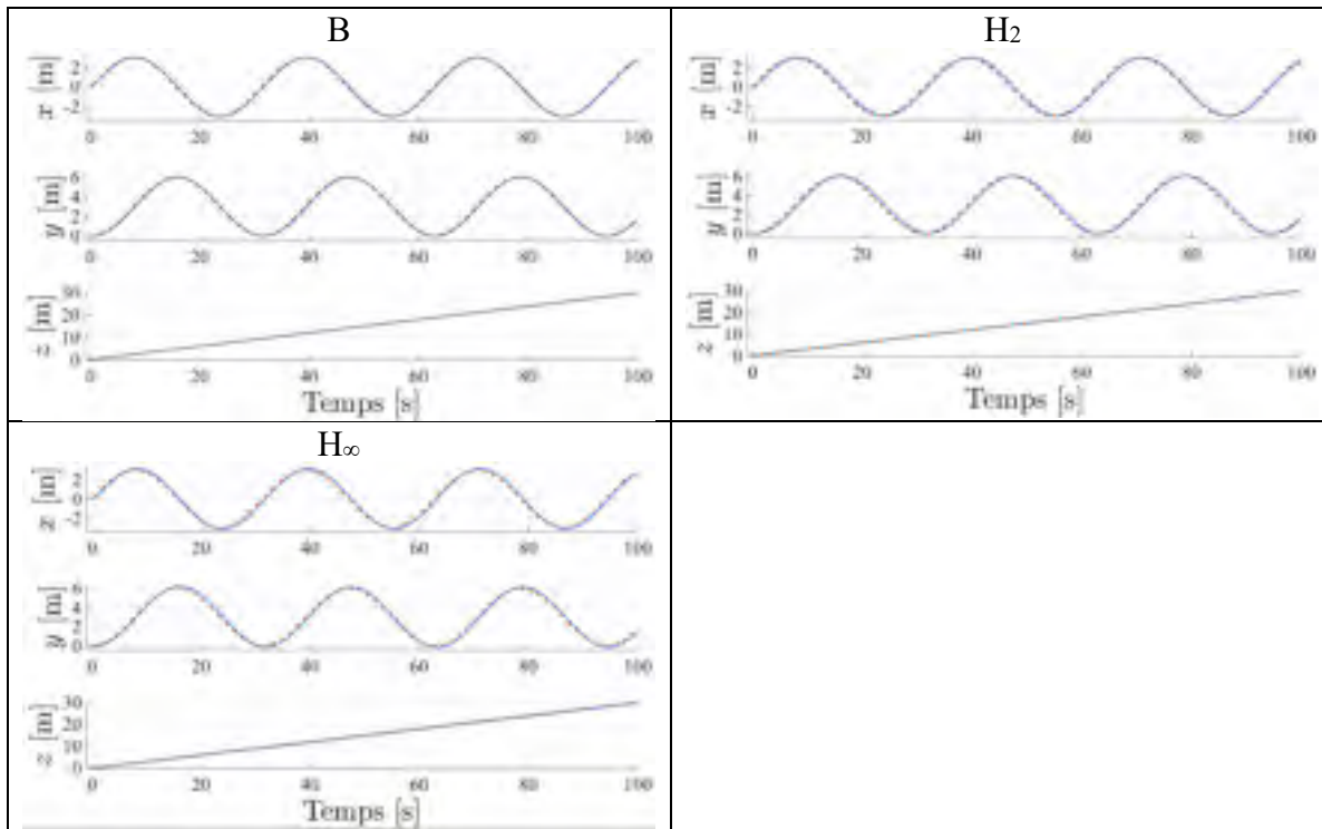
Figure 7.43 Déplacement en bleu sur x , y , z lors d'une consigne hélicoïdale en pointillé rouge et définie en (7.4), pour les compensateurs : B, H_2 , H_\infty
