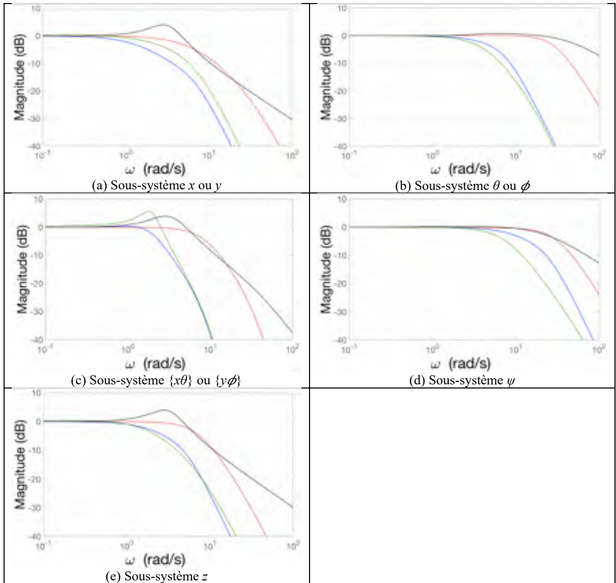
Figure 7.5 Diagramme de Bode du gain de la transmission T(s) sur les axes x ou y (a), \{x\theta\} ou \{y\phi\} (c), z (e) et autour des angles \theta ou \phi (b), \psi (d) avec les compensateurs B (rouge), \mu (bleu), \mu_\Delta (vert) et PID (noir)
