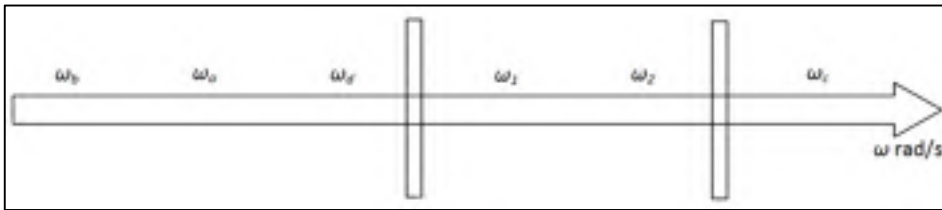
Figure 4.4 Ordre des fréquences dans la conception de la commande B
