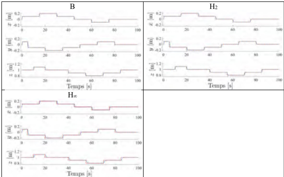
Figure 7.16 Réponses temporelles (bleue) sur les axes x , y , z pour le scénario de référence (pointillé rouge) défini en (7.2), avec les compensateurs B, H_2 , H_\infty sur le processus linéaire
