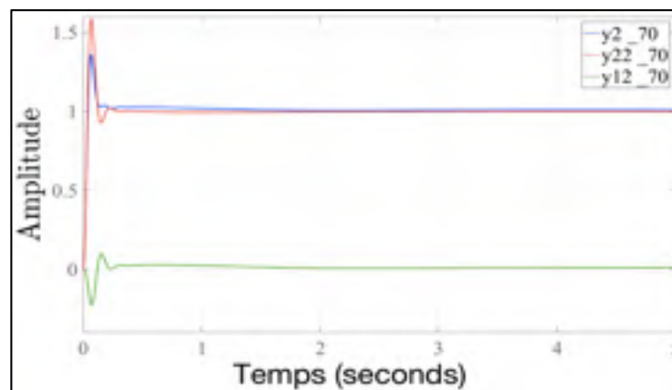
Figure 4.43 Réponse temporelle de y_2(t) , y_{22}(t) et y_{12}(t) pour C_{max} = 70 dB, dans le cas sans erreur statique
