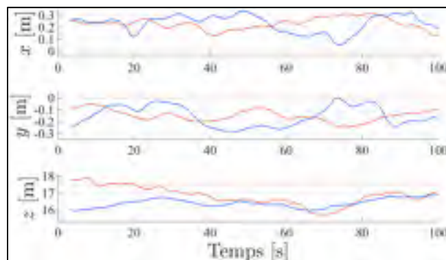
Figure 8.41 Mesures expérimentales avec le drone F450J des déplacements sur x, y, z lors d'un vol stationnaire pour les compensateurs : \text{PID}_{\phi} (bleu) ; B (rouge)
