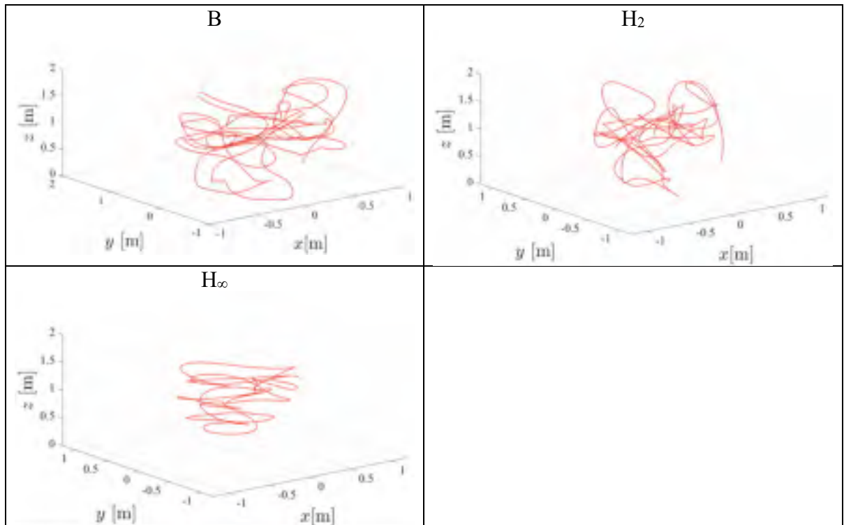
Figure 7.73 Déplacements sur les axes x, y, z lors d'un vol stationnaire en présence de perturbation sur la sortie pour les compensateurs B, H 2 , H ∞ appliqués sur le modèle linéaire de drone
