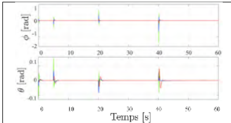
Figure 7.37 Réponses temporelles sur les angles \phi , \theta et l'axe x pour le scénario de référence y_d défini en (7.3), avec les compensateurs : B (rouge), H_2 (verte), H_\infty (bleue)
