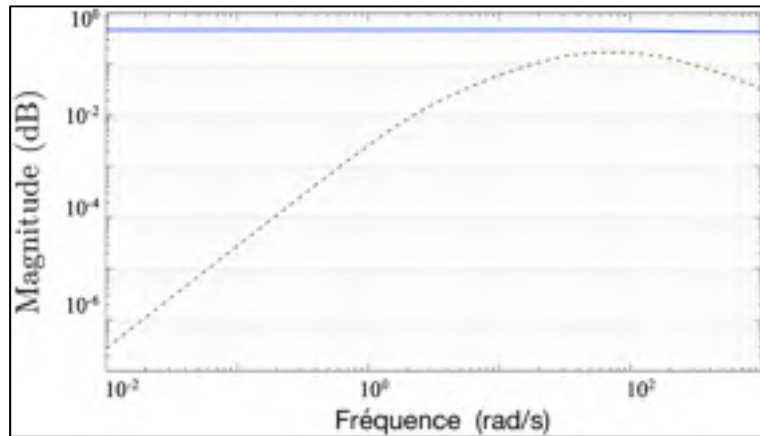
Figure 5.33 Stabilité robuste \|M_{\tilde{a} \rightarrow \tilde{u}}\|_{\infty} en pointillé vert et robuste performance \mu_{\tilde{\Delta}_p}(M(j\omega)) courbes rouge et bleue (superposées) autour de l'angle \psi , sans incertitudes
