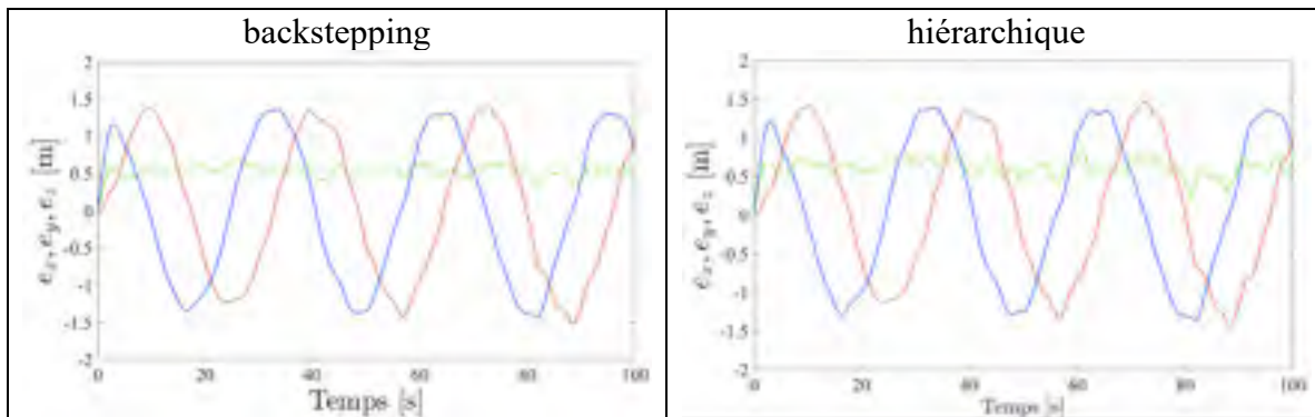
Figure 7.130 Erreurs e_x (bleue), e_y (rouge), e_z (verte) pour une consigne hélicoïdale définie en (7.4), avec perturbation en sortie pour les compensateurs backstepping et hiérarchique
