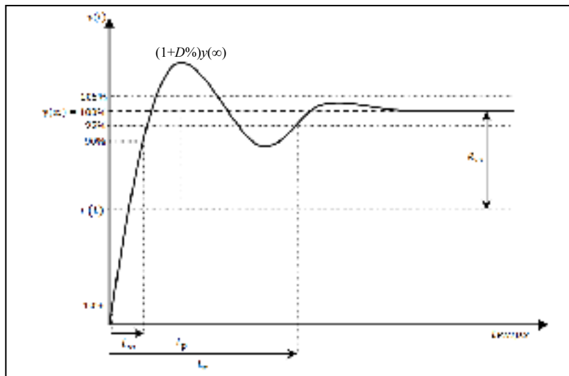
Figure 2.8 Exemple de réponse unitaire
