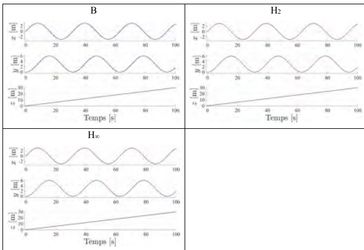
Figure 7.55 Déplacements sur x, y, z lors d'une consigne hélicoïdale définie en (7.4), pour les compensateurs : B, H_2 , H_\infty
