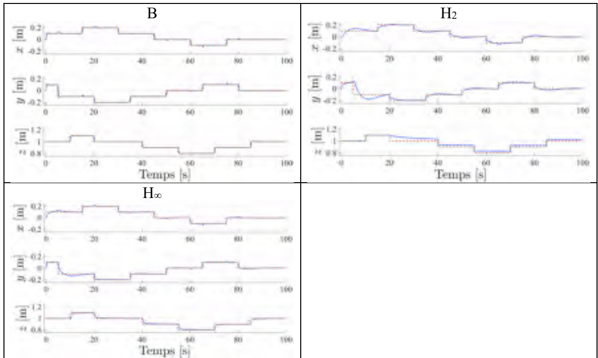
Figure 7.24 Réponses temporelles sur les axes x , y , z pour le scénario de référence en pointillé rouge (7.2), avec les compensateurs B, H_2 , H_\infty sur le processus non linéaire
