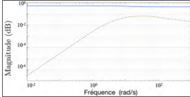
Figure 5.35 Stabilité robuste \|M_{\tilde{d} \rightarrow \tilde{u}}\|_{\infty} en pointillé vert et robuste performance \mu_{\tilde{d}_p}(M(j\omega)) courbes rouge et bleue (superposées) autour de l'angle \psi , avec incertitude
