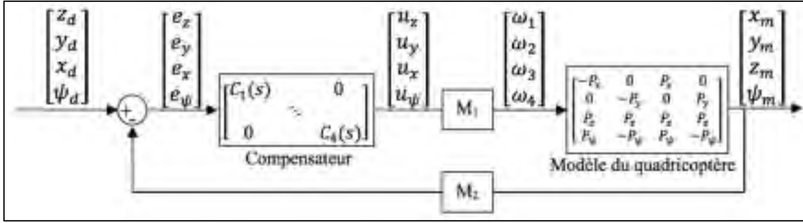
Figure 3.11 Boucle fermée avec le processus non diagonal linéarisé pour une commande en translation et de rotation en cascade
