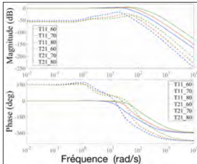
Figure 4.33 Bode de T_{11}(s) et T_{21}(s) pour C_{max} = \{60, 70, 80\} dB, dans le cas sans erreur statique
