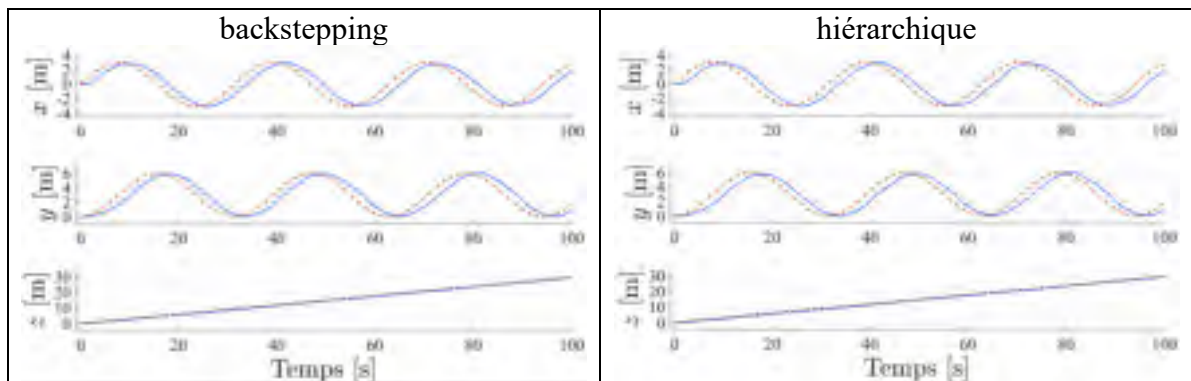
Figure 7.128 Variations sur x, y, z lors d'une consigne hélicoïdale en pointillé rouge définie en (7.4), avec perturbation en sortie pour les compensateurs backstepping et hiérarchique
