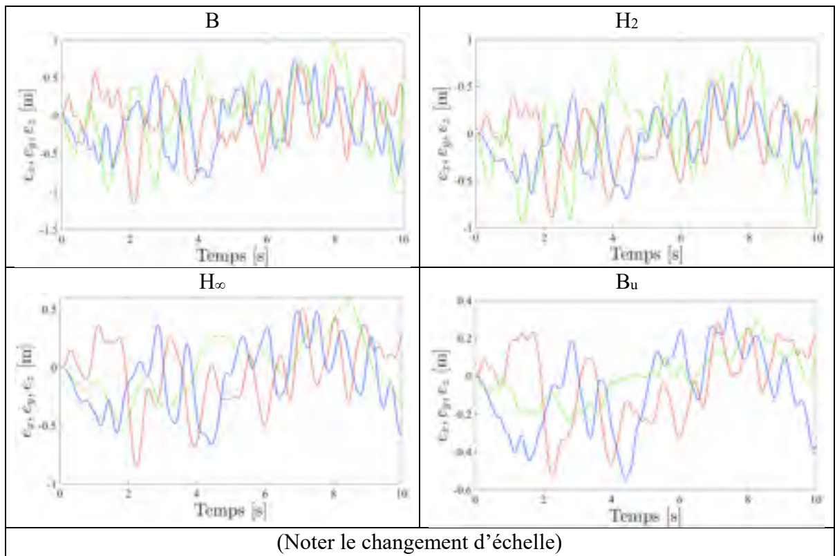
Figure 7.159 Erreurs e_x (bleue), e_y (rouge), e_z (verte) lors d'un vol stationnaire en présence de perturbation en sortie pour les compensateurs B, H_2 , H_\infty , B_u appliqués sur le modèle linéaire de drone
