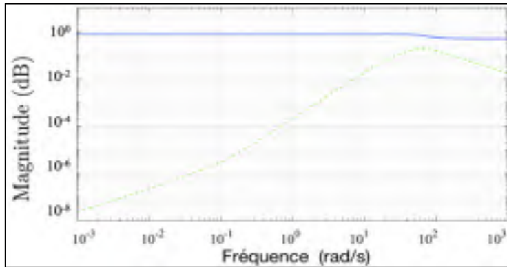
Figure 5.26 Stabilité robuste \|M_{\tilde{d} \rightarrow \tilde{u}}\|_\infty en pointillé vert et robuste performance \mu_{\tilde{A}_p}(M(j\omega)) courbes rouge et bleue (superposées) pour l'axe z , sans incertitudes
