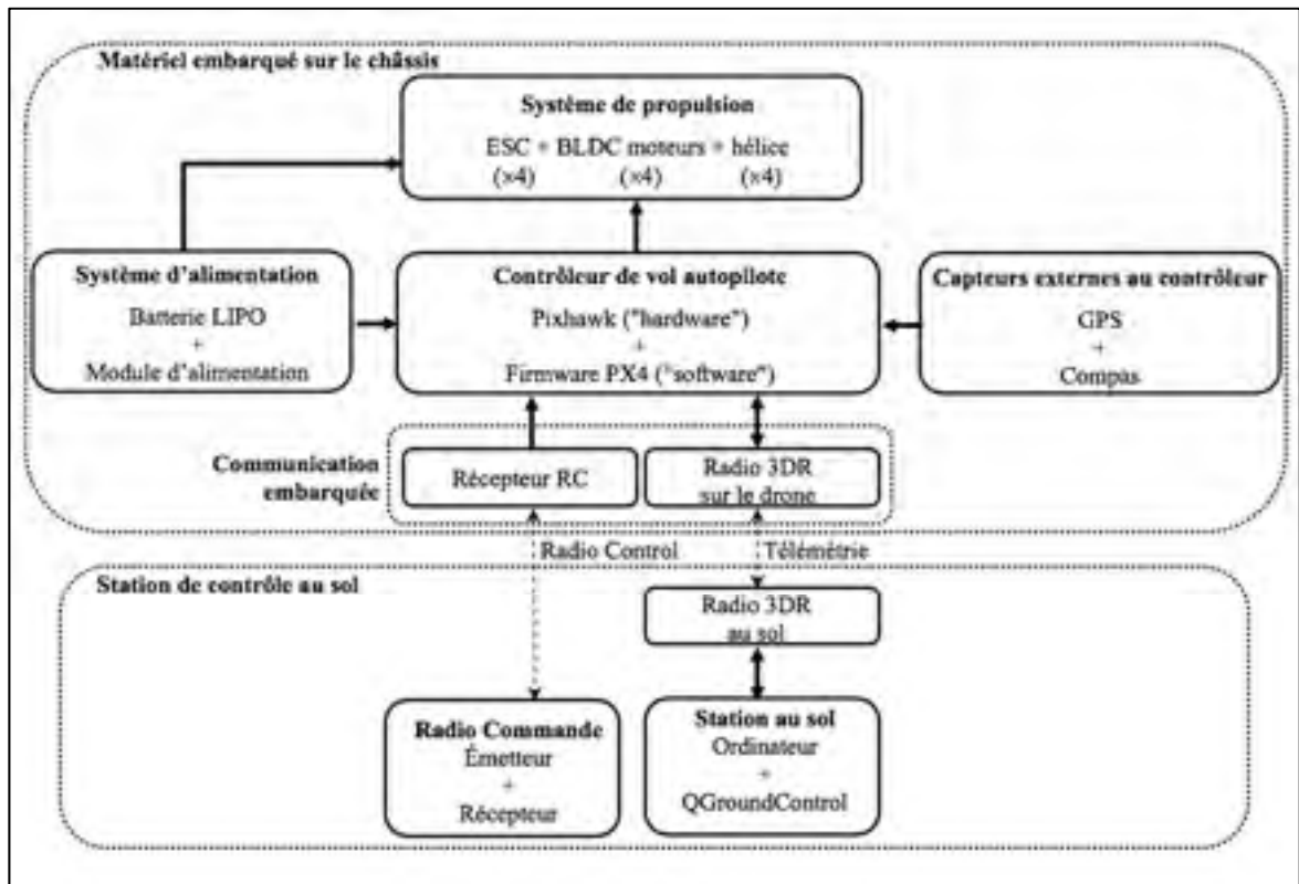
Figure 8.1 Configuration matérielle du quadricoptère F450J basée sur l'autopilote PX4
