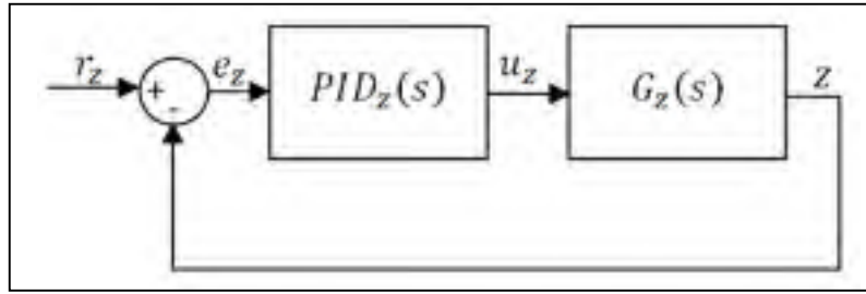
Figure 5.3 Chaîne d'altitude avec le compensateur PID_z(s)
