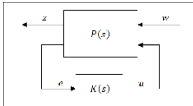
Figure 5.14 Représentation de la forme standard soumise à des perturbations exogènes
