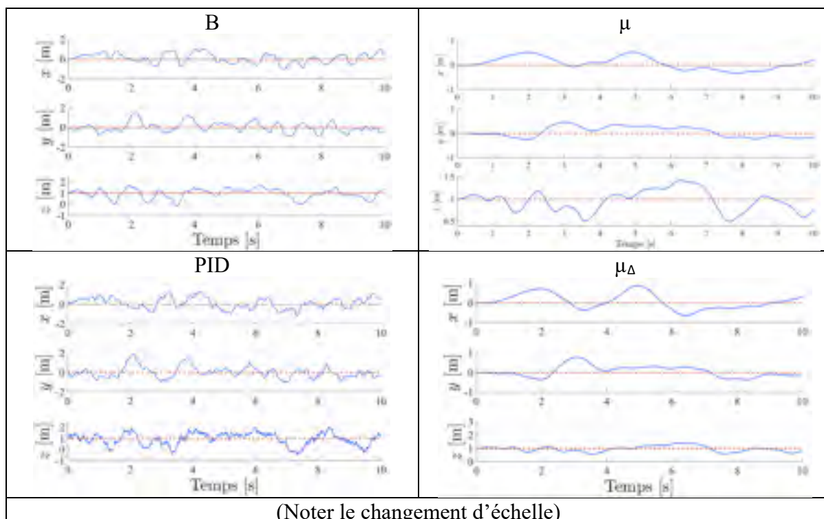
Figure 7.79 Variations des axes x , y , z lors d'un vol stationnaire en présence de perturbation sur la sortie pour les compensateurs B , \mu , \mu_{\Delta} , PID appliqués sur le modèle linéaire de drone
