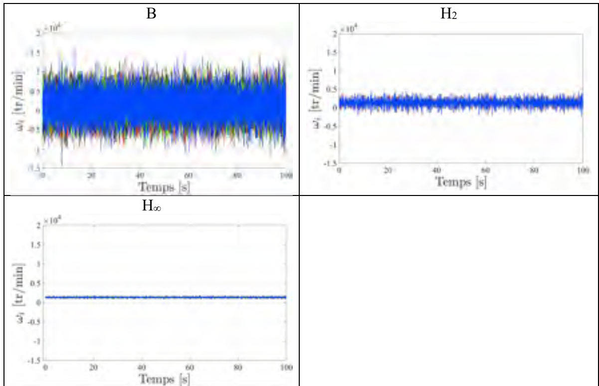
Figure 7.108 Vitesses \omega_1 (noire), \omega_2 (rouge), \omega_3 (verte), \omega_4 (bleue) lors d'une consigne hélicoïdale en pointillé rouge et définie en (7.4), en présence de perturbation en sortie pour les compensateurs B, H 2 , H ∞ sur le processus linéaire
