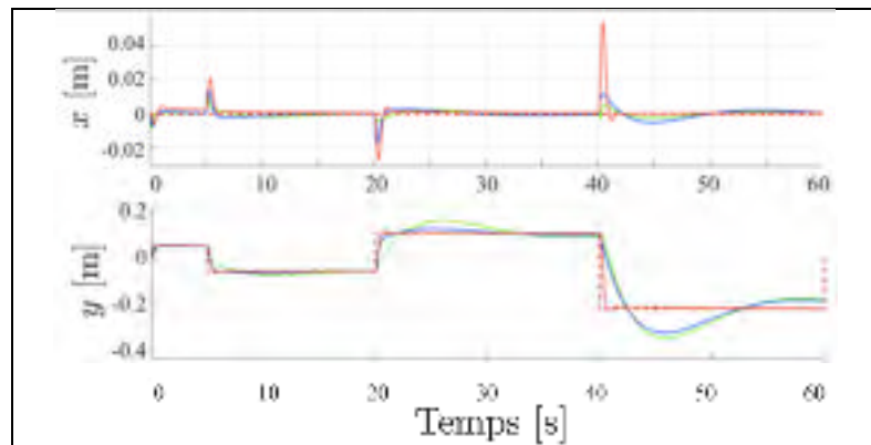
Figure 7.36 Réponses temporelles sur x , y pour le scénario de référence y_d en pointillé rouge défini en (7.3), avec les compensateurs : B (rouge), H_2 (vert), H_\infty (bleu)
