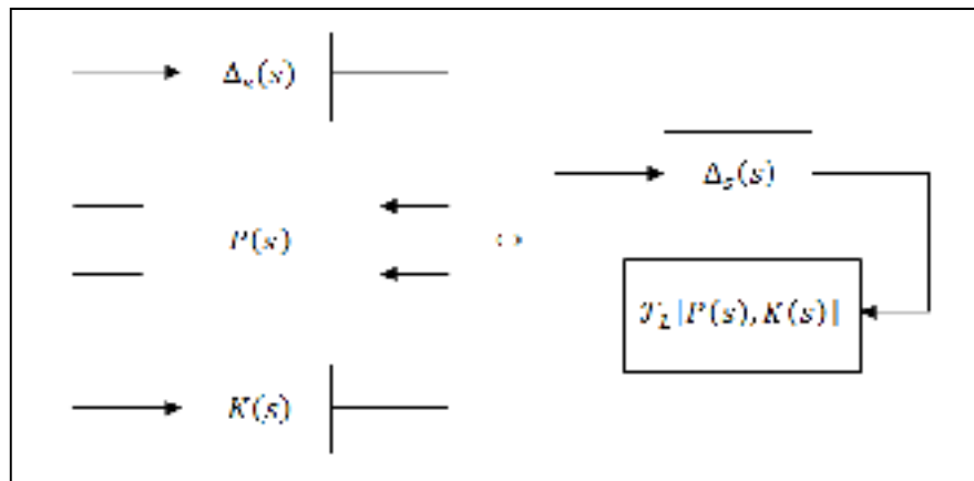
Figure 5.13 P(s) et K(s) associés à des incertitudes structurées \Delta_s(s)
