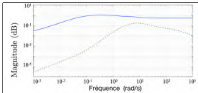
Figure 5.28 Stabilité robuste \|M_{\tilde{d} \rightarrow \tilde{u}}\|_{\infty} en pointillé vert et robuste performance \mu_{\tilde{Z}_p}(M(j\omega)) courbes rouge et bleue (superposées) pour l'axe z , avec incertitudes
