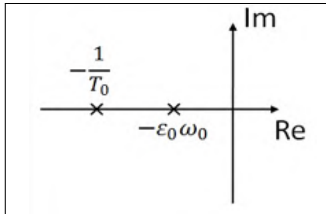
Figure 5.2 Emplacement des pôles de la boucle fermée T(s) dans le cas d'un compensateur PID(s) associé à un second ordre G(s)
