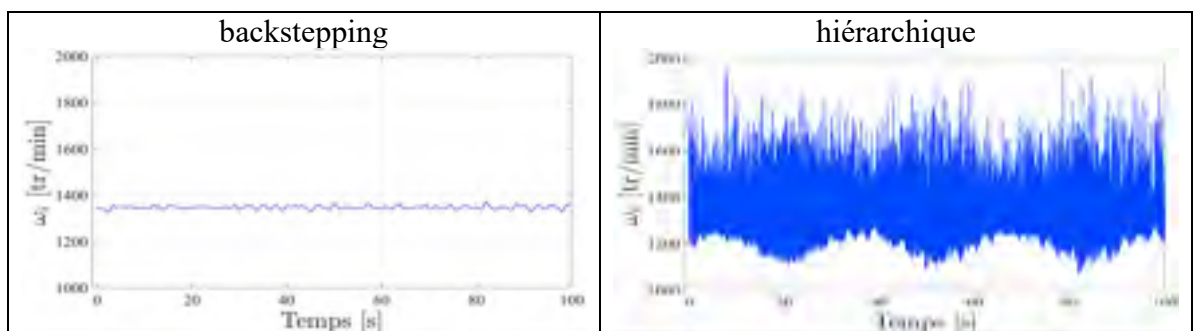
Figure 7.132 Vitesses \omega_1 (noire), \omega_2 (rouge), \omega_3 (verte), \omega_4 (bleue) lors d'une consigne hélicoïdale, avec perturbation en sortie pour les compensateurs backstepping et hiérarchique
