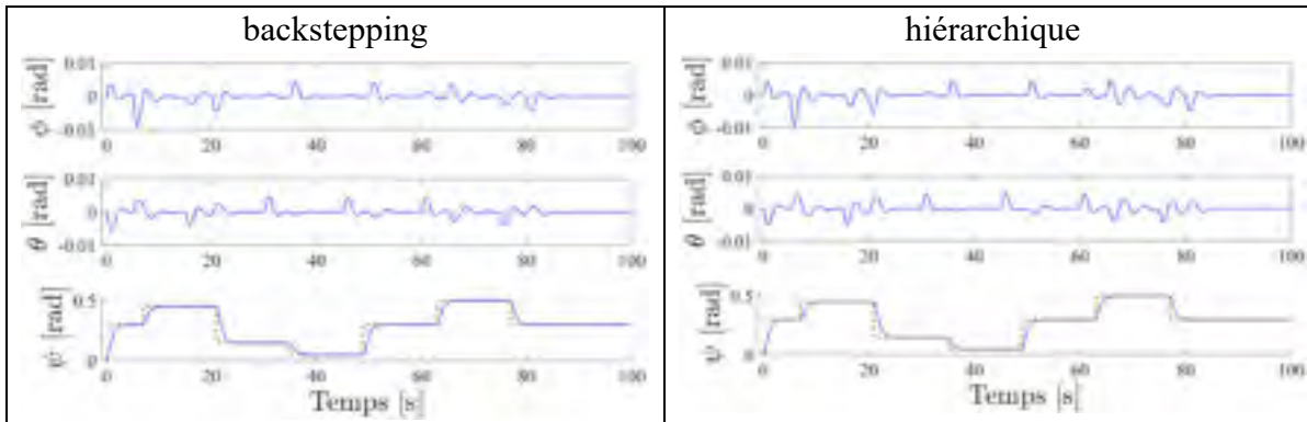
Figure 7.33 Réponses temporelles des angles \phi , \theta , \psi pour le scénario de référence en pointillé rouge et défini en (7.2), avec les compensateurs backstepping et hiérarchique
