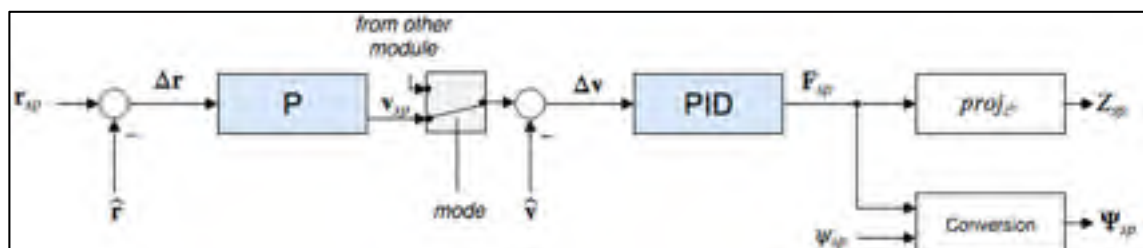
Figure 8.20 Contrôleur de position et vitesse linéaire PX4 31
