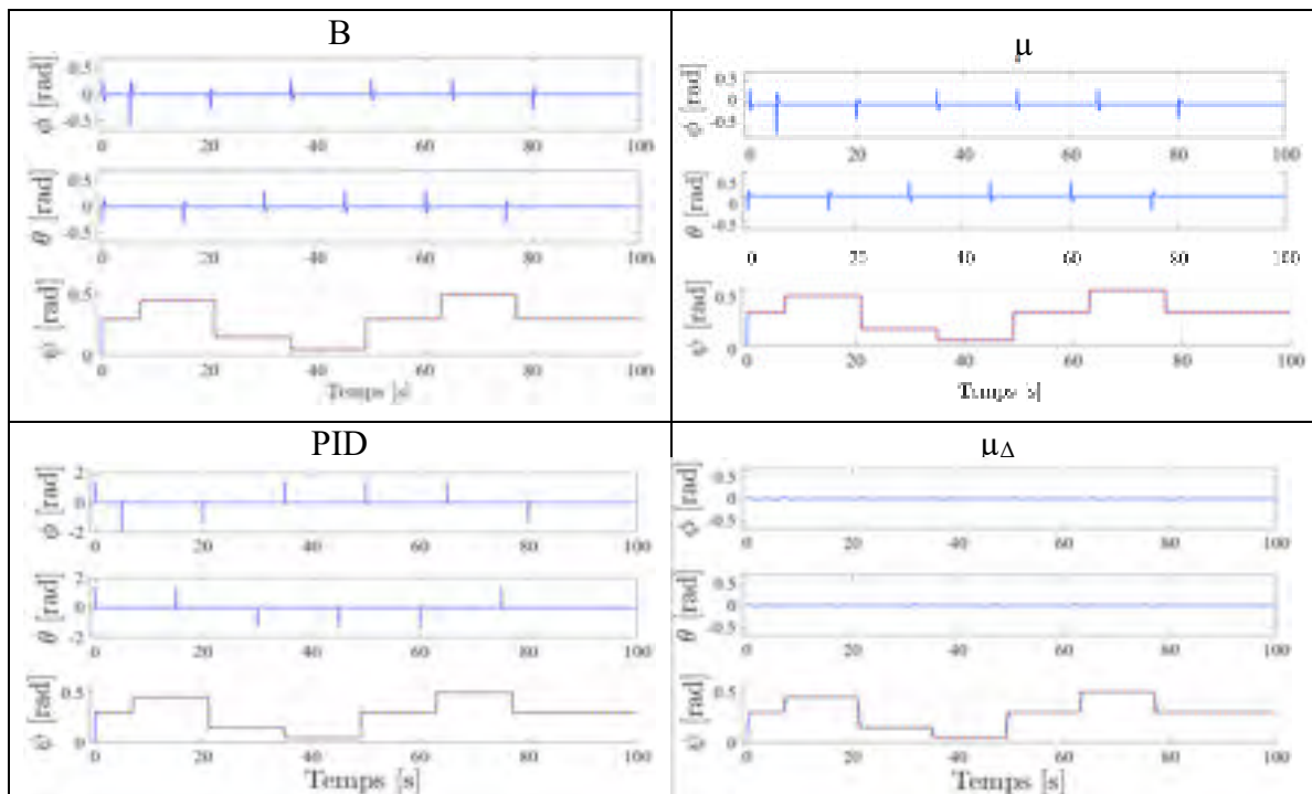
Figure 7.21 Réponses temporelles des angles \phi , \theta , \psi pour le scénario de référence en pointillé rouge défini en (7.2), avec les compensateurs B , \mu , PID, \mu_{\Delta} sur le processus linéaire
