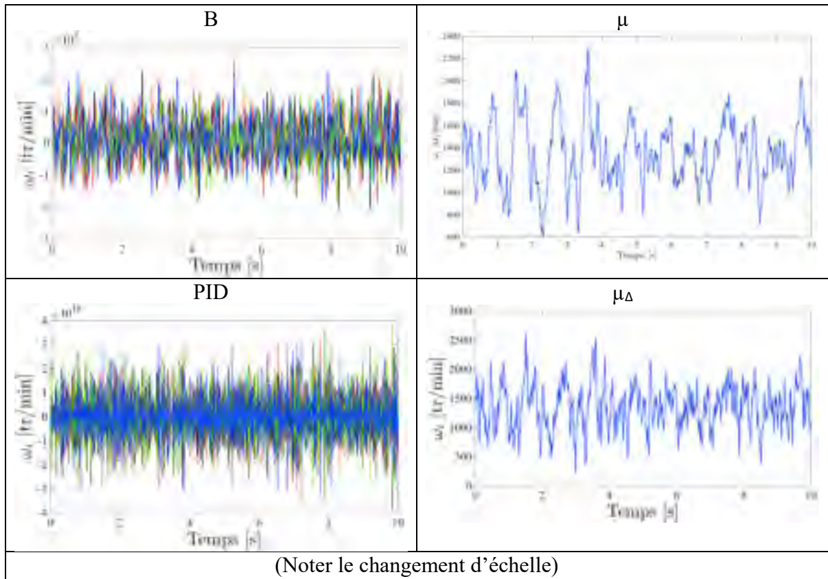
Figure 7.84 Vitesses \omega_1 (noire), \omega_2 (rouge), \omega_3 (verte), \omega_4 (bleue) lors d'un vol stationnaire en présence de perturbation en sortie pour les compensateurs B, \mu , \mu_\Delta , PID appliqués sur le modèle linéaire de drone
