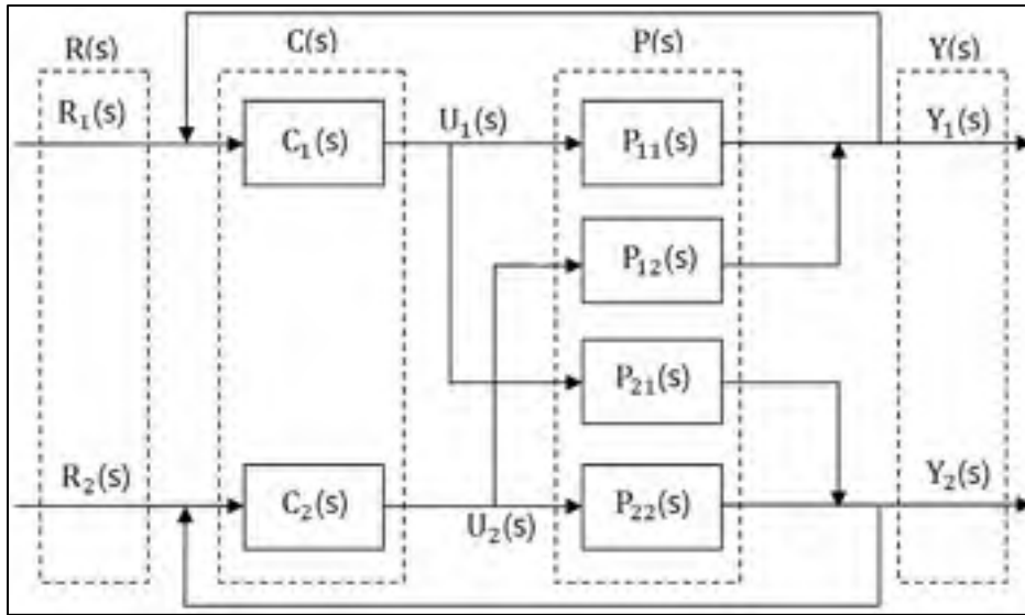
Figure 4.8 Représentation sous forme de schéma bloc du système multivariable P(s) et de son compensateur C(s)
