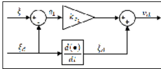
Figure 6.1 Schéma bloc de la commande virtuelle en vitesse v_d
