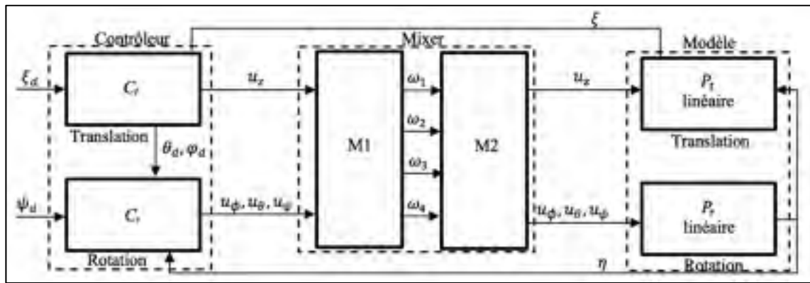
Figure 3.12 Boucle fermée avec le processus linéarisé pour une commande en translation et rotation séparées
