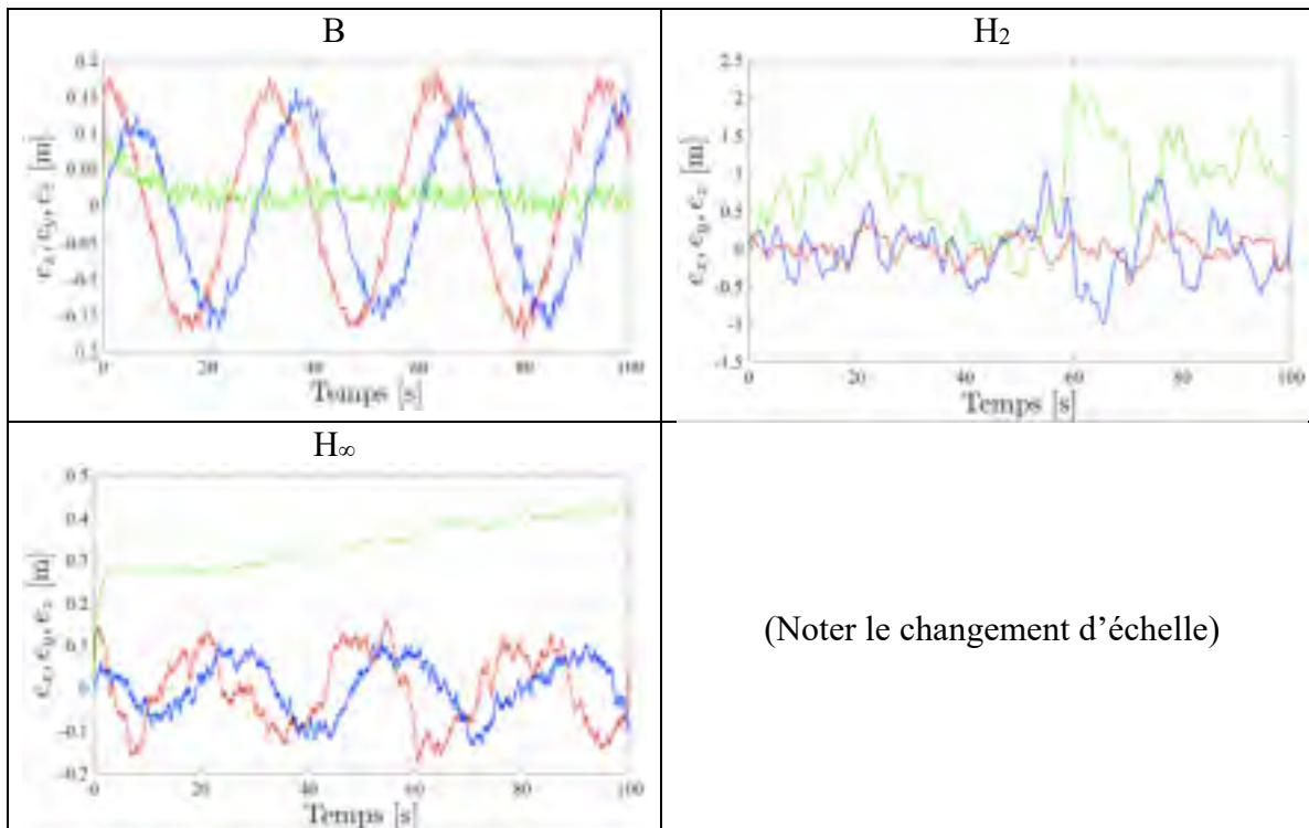
Figure 7.118 Erreurs e_x (bleue), e_y (rouge), e_z (verte) lors d'une consigne hélicoïdale définie en (7.4), en présence de perturbation en sortie pour les compensateurs B, H_2 , H_\infty sur le processus non linéaire
