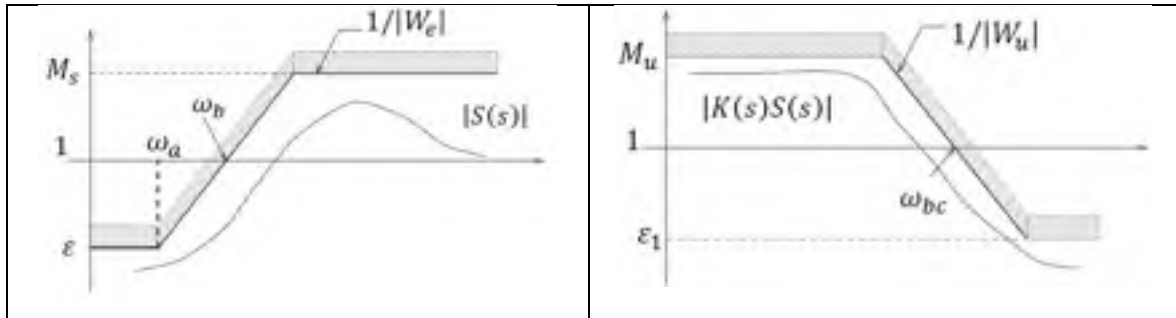
Figure 5.7 a Sensibilité et pondération S(s) et 1/W_e(s) Extrait et adapté de Zhou & Doyle (1998)
