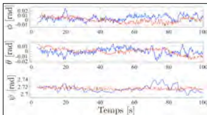
Figure 8.42 Mesures expérimentales avec le drone F450J des orientations angulaires \phi , \theta , \psi lors d'un vol stationnaire pour les compensateurs : PID _{\phi} (bleu) ; B (rouge)
