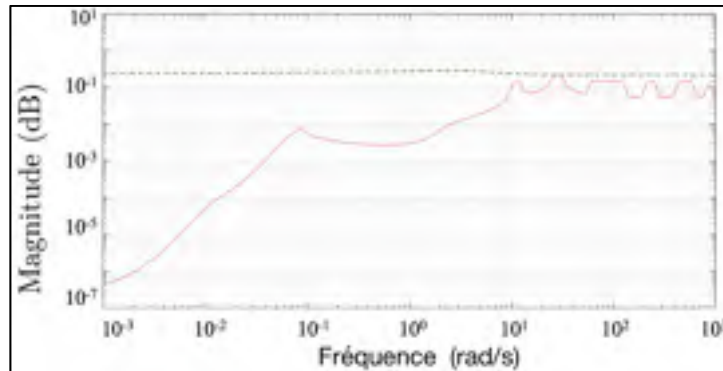
Figure 5.27 \mu_{\Delta s} et \|\mathcal{F}_l(P(j\omega), K(j\omega))\|_{\infty} pour l'axe z avec incertitude
