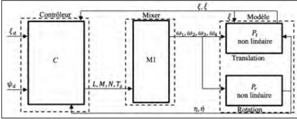
Figure 3.13 Boucle fermée avec le processus non linéaire pour une commande en translation et de rotation en cascade
