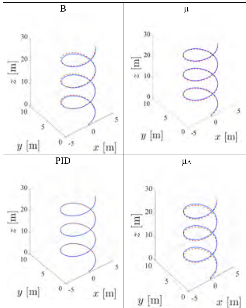
Figure 7.60 Déplacement en 3D sur x , y , z lors d'une consigne hélicoïdale définie en (7.4), pour les compensateurs : B , \mu , PID, \mu\Delta
