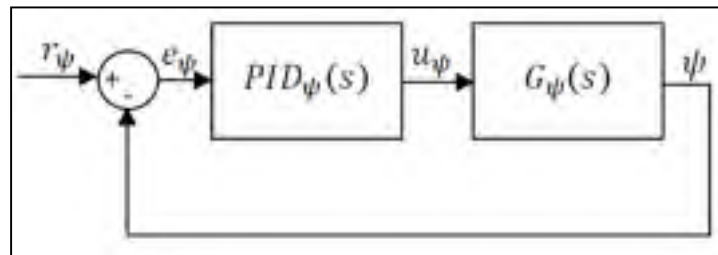
Figure 5.5 Chaîne de commande autour de l'angle \psi avec le compensateur PID_\psi(s)
