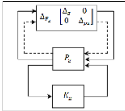
Figure 5.23 Insertion du critère de performance \Delta_{pz}
