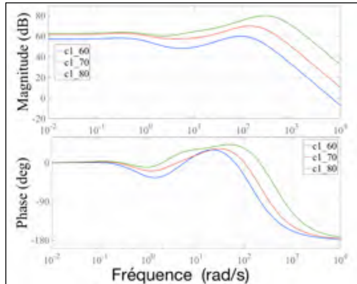
Figure 4.32 Bode de C(s) pour C_{max} = \{60, 70, 80\} dB, dans le cas sans erreur statique
