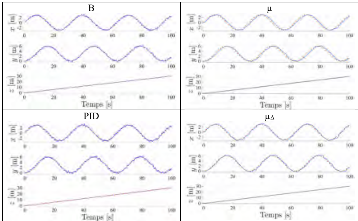
Figure 7.110 Déplacements sur les axes x , y , z en fonction du temps lors d'une consigne hélicoïdale en pointillé rouge et définie en (7.4), en présence de perturbation en sortie pour les compensateurs B , \mu , \mu_{\Delta} , PID sur le processus linéaire
