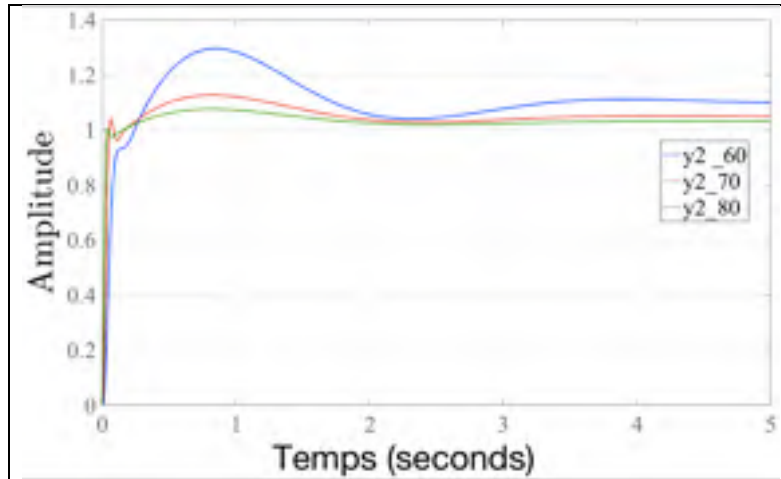
Figure 4.24 Allure de y_2(t) optimisé pour C_{max} = 60, 70 et 80 dB
