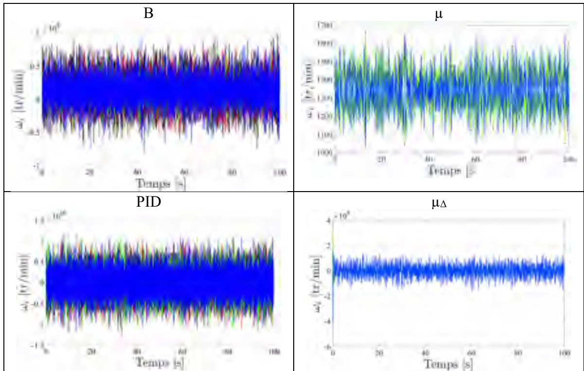
Figure 7.114 Vitesses \omega_1 (noire), \omega_2 (rouge), \omega_3 (verte), \omega_4 (bleue) lors d'une consigne hélicoïdale définie en (7.4), en présence de perturbation en sortie pour les compensateurs B, \mu , \mu\Delta , PID sur le processus linéaire
