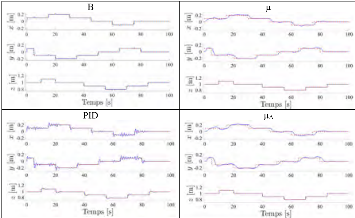
Figure 7.28 Réponses temporelles sur les axes x , y , z pour le scénario de référence en pointillé rouge et défini en (7.2), avec les compensateurs B, \mu , PID, \mu_{\Delta} sur le processus non linéaire
