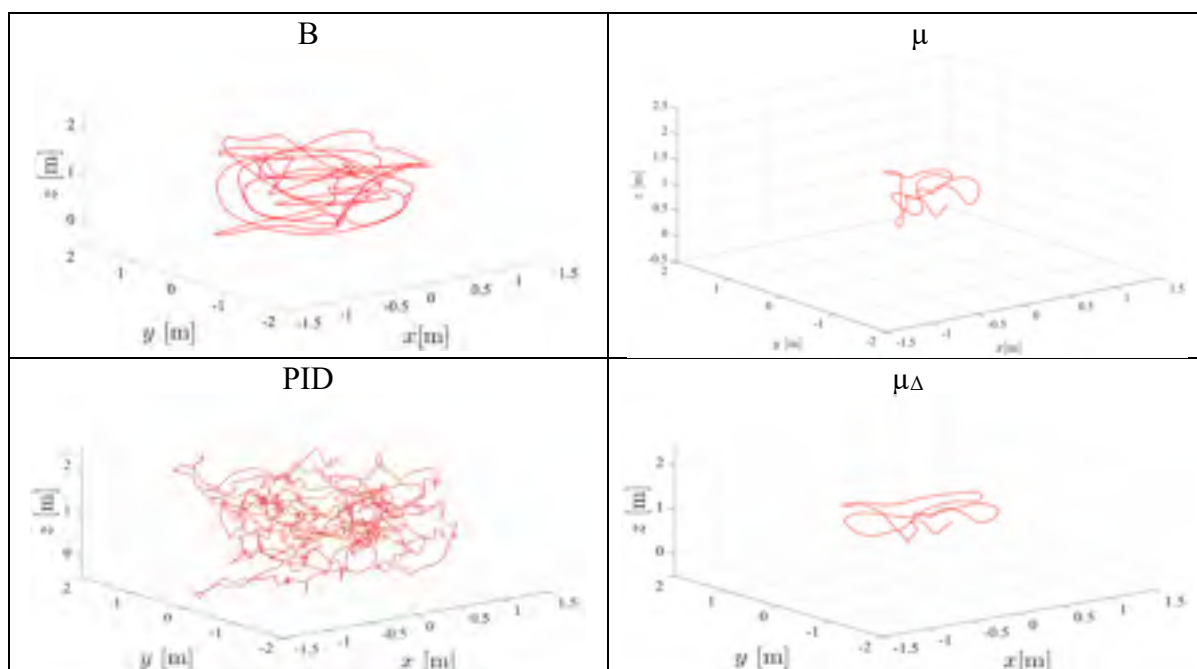
Figure 7.79 Variations des axes x , y , z lors d'un vol stationnaire en présence de perturbation sur la sortie pour les compensateurs B , \mu , \mu_{\Delta} , PID appliqués sur le modèle linéaire de drone
