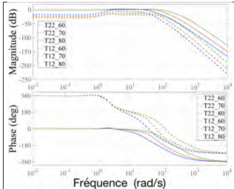
Figure 4.20 Allure de T_{22}(s) et T_{12}(s) optimisées pour C_{max} = 60, 70 et 80 dB
