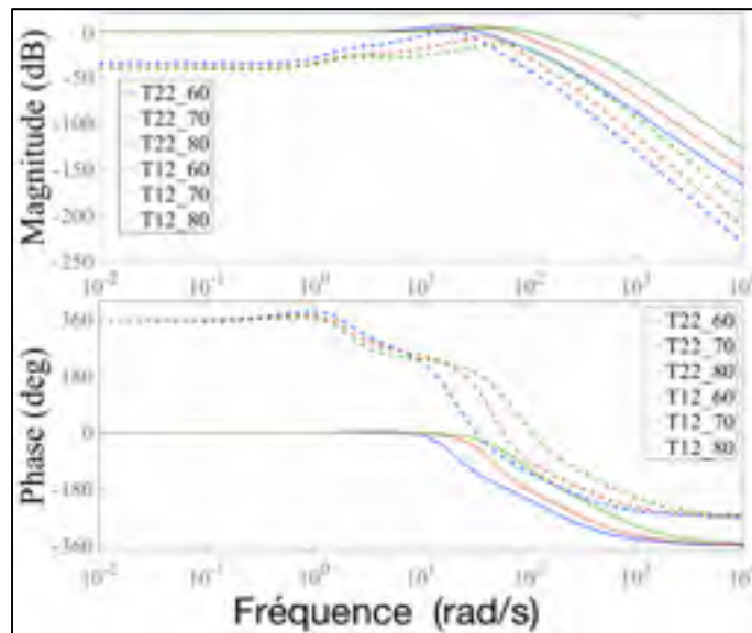
Figure 4.34 Bode de T_{22}(s) et T_{12}(s) pour C_{max} = \{60, 70, 80\} dB, dans le cas sans erreur statique
