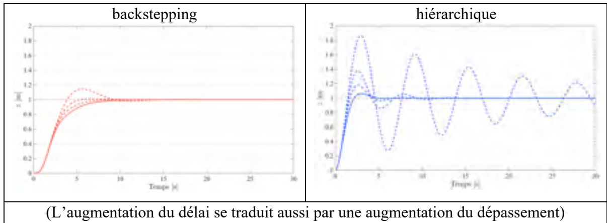
Figure 7.147 Réponses unitaires nominales en trait plein sur l'axe z et en pointillés avec ajout de délais de mesure, pour les compensateurs : backstepping (rouge), hiérarchique (bleu)
