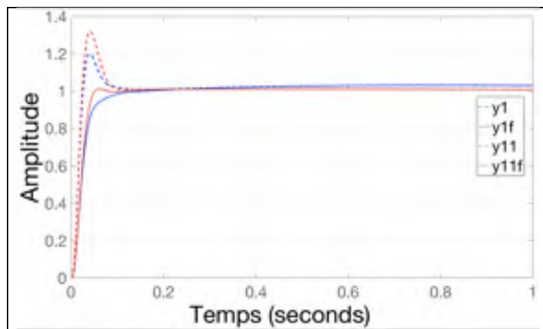
Figure 4.49 Réponse indicielle de y_1(t) , y_{1f}(t) , y_{11}(t) et y_{11f}(t)
