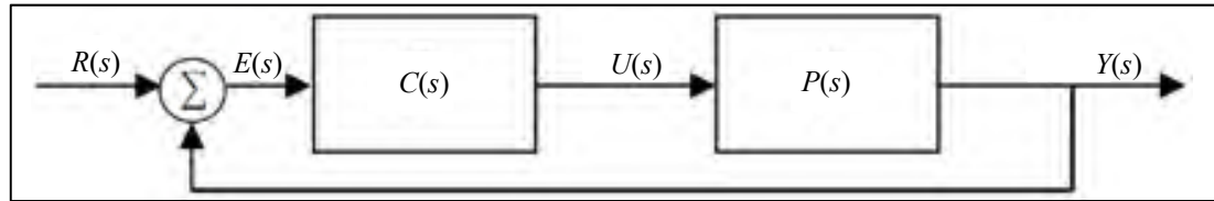
Figure 2.5 Schéma bloc d'une commande en boucle fermée
