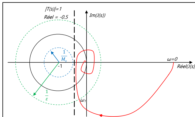
Figure 2.12 Diagramme de Nyquist de J(s) Tirée et reproduite de Houimdi (2015)
