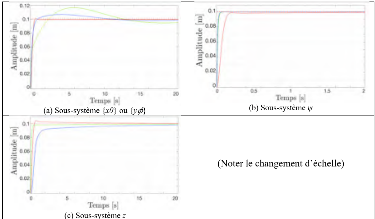
Figure 7.13 Réponse unitaire y(t) pour les compensateurs B (rouge), H_2 (vert) et H_\infty (bleu) sur le processus non linéaire
