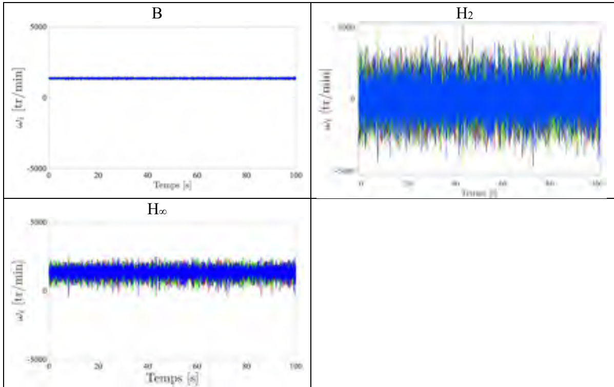
Figure 7.90 Vitesses \omega_1 (noire), \omega_2 (rouge), \omega_3 (verte), \omega_4 (bleue) lors d'un vol stationnaire en présence de perturbation en sortie pour les compensateurs B, H_2 , H_\infty appliqués sur le modèle non linéaire de drone
