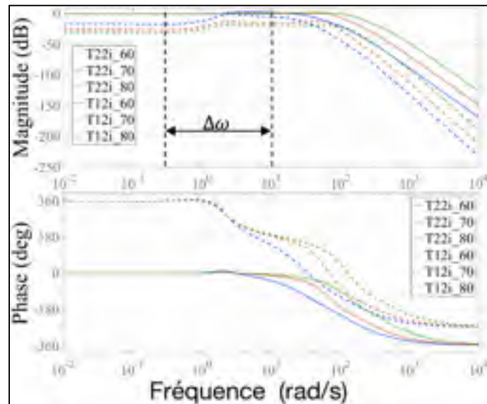
Figure 4.17 Bode de T_{22i}(s) et T_{12i}(s)
