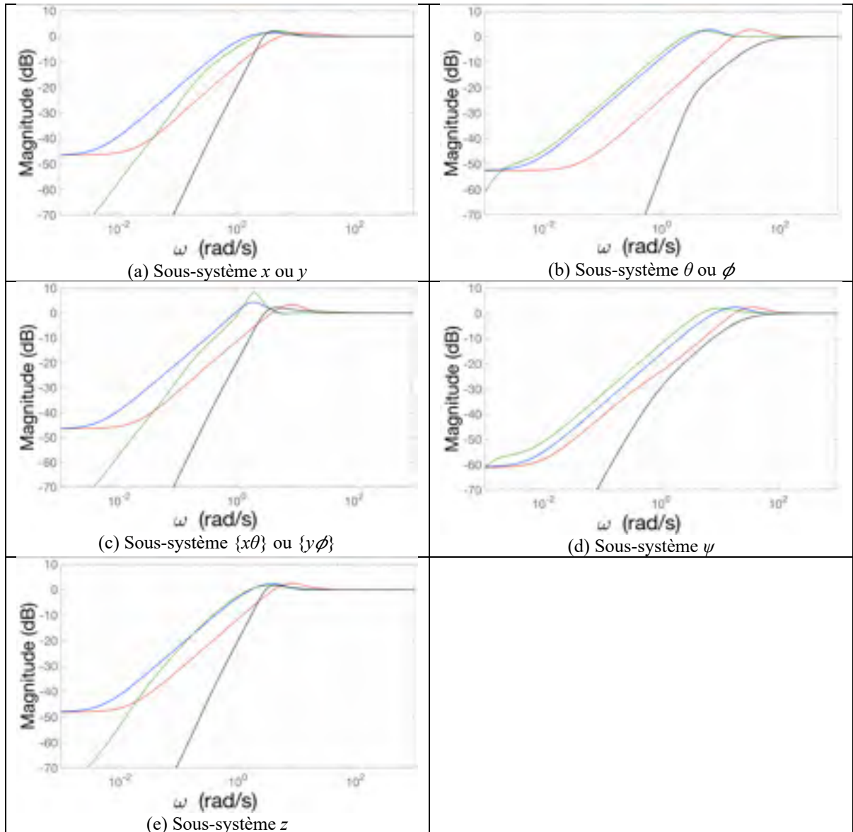
Figure 7.7 Diagramme de Bode du gain de la sensibilité S_{ey}(s) sur les axes x ou y (a), \{x\theta\} ou \{y\phi\} (c), z (e) et autour des angles \theta ou \phi (b), \psi (d) avec les compensateurs B (rouge), \mu (bleu), \mu_\Delta (vert) et PID (noir)
