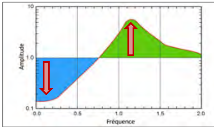
Figure 2.9 Image illustrant le comportement de la sensibilité en HF lors d'une augmentation de gain pour minimiser la sensibilité en BF
