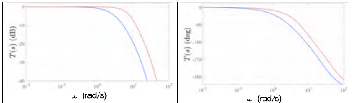
Figure 7.153 Transmissions T(s) sur x ou y pour le compensateur B (rouge) et le compensateur B_u (bleu). À gauche l'amplitude et à droite la phase
