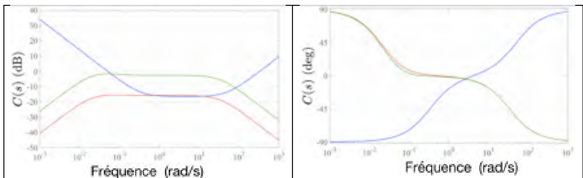
Figure 8.35 Bode des compensateurs (gains à gauche et phases à droite) : PID _{\phi} (bleu) ; B (rouge) ; B amélioré (vert)
