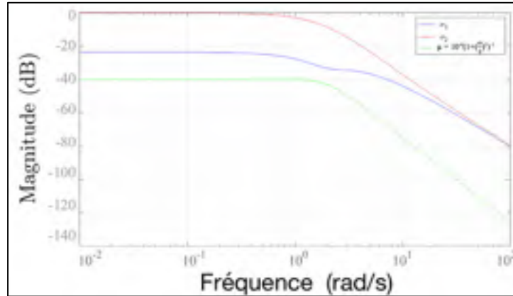
Figure 4.9 Valeurs singulières de P(j\omega)
