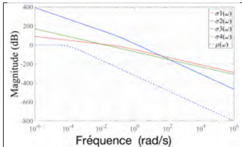
Figure 4.58 Valeurs singulières de P(j\omega) , \sigma_1(\omega) en noir (derrière la courbe rouge) et \sigma_2(\omega) en rouge, \sigma_3(\omega) en bleu et \sigma_4(\omega) en vert, \mu(\omega) en pointillé bleu.
