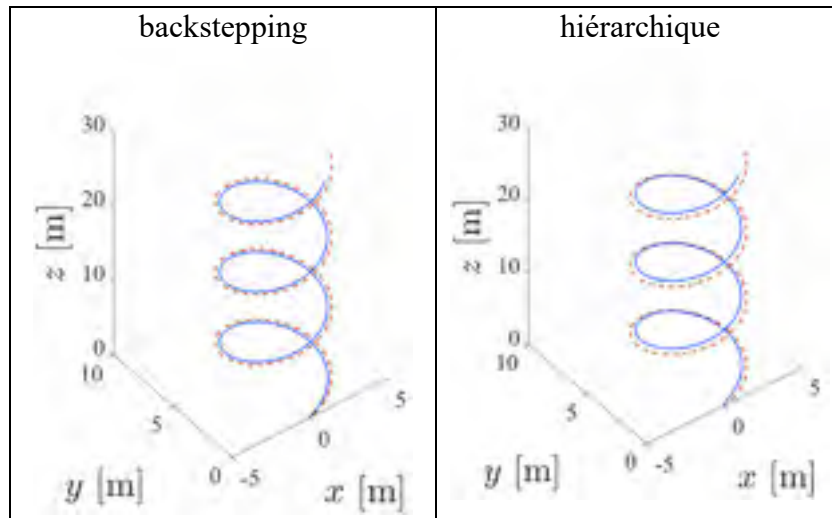
Figure 7.66 Déplacement en 3D sur x , y , z lors d'une consigne hélicoïdale définie en (7.4), pour les compensateurs backstepping et hiérarchique
