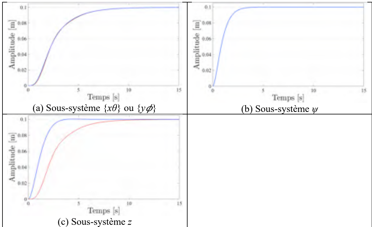
Figure 7.15 Réponse unitaire y(t) pour les compensateurs backstepping (rouge) et hiérarchique (bleu)
