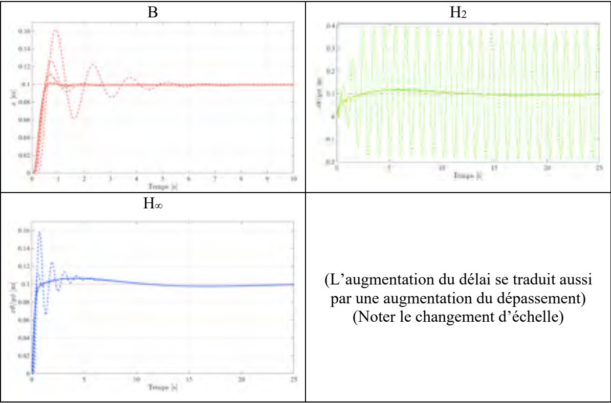
Figure 7.140 Réponses unitaires nominales en trait plein sur les axes \{x\theta\} ou \{y\phi\} et en pointillés avec l'ajout de délais de mesure, pour les compensateurs : B (rouge), H 2 (vert), H ∞ (bleu) pour le processus non linéaire
