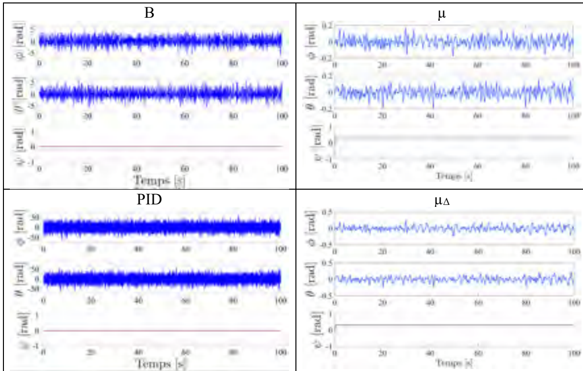
Figure 7.111 Déplacements des angles \phi, \theta, \psi lors d'une consigne hélicoïdale définie en (7.4), en présence de perturbation en sortie pour les compensateurs B, \mu , \mu_\Delta , PID sur le processus linéaire
