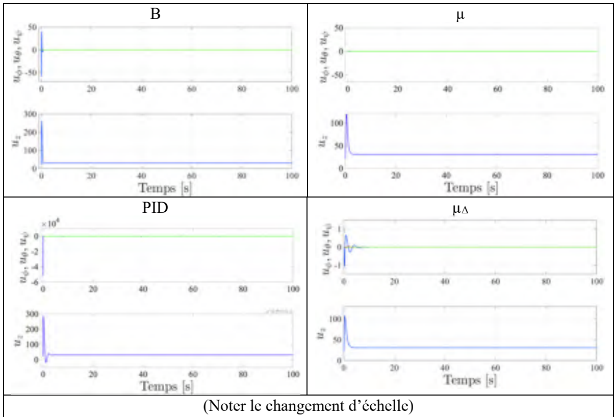
Figure 7.52 Commandes u_\phi (bleue), u_\theta (rouge), u_\psi (verte), u_z lors d'une consigne hélicoïdale définie en (7.4), pour les compensateurs : B, \mu , PID, \mu_\Delta
