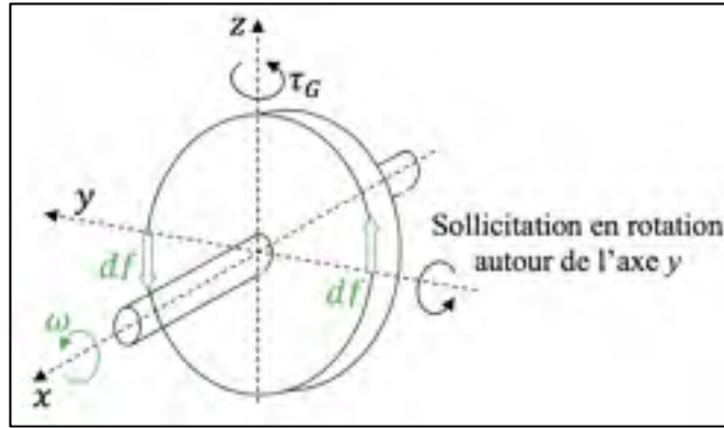
Figure 3.8 Représentation du couple gyroscopique
