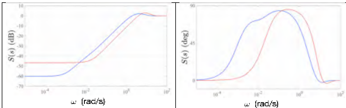
Figure 7.152 Allures de la sensibilité S_{ey}(s) sur x ou y pour le compensateur B (rouge) et le compensateur B_u (bleu). À gauche l'amplitude et à droite la phase
