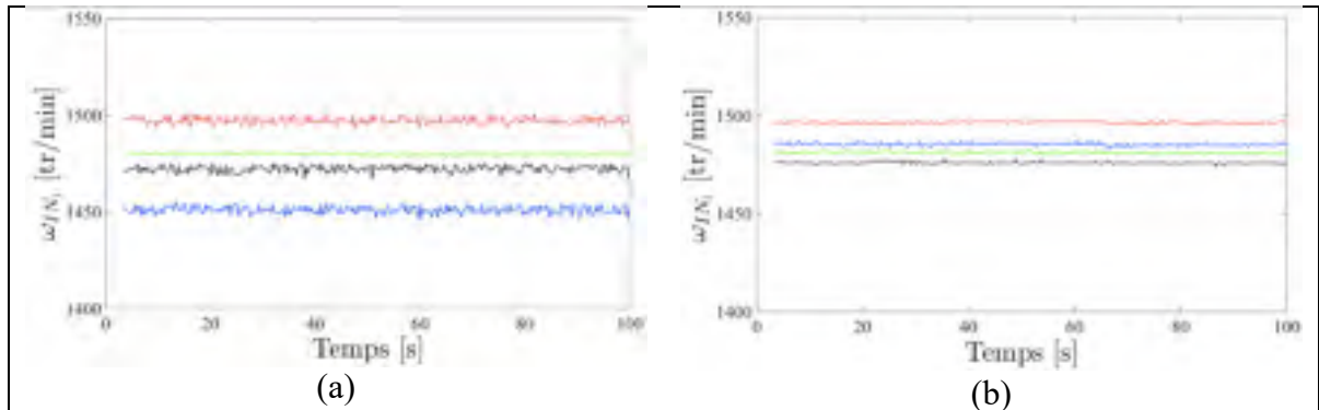
Figure 8.43 Commandes expérimentales avec le drone F450J en vitesse \omega_1, \omega_2, \omega_3, \omega_4 envoyées au drone pour les compensateurs : PID _{\phi} (a) ; B (b)
