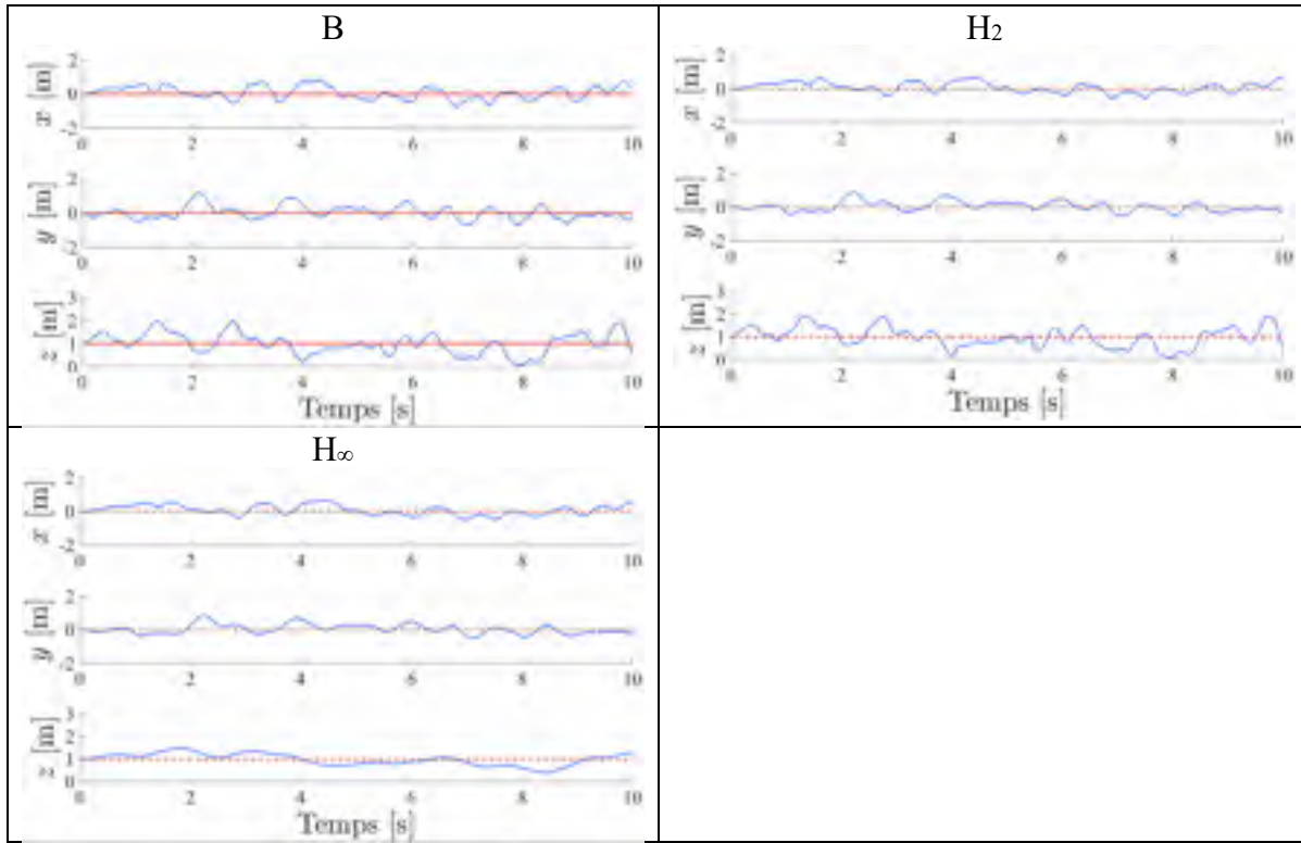
Figure 7.74 Variations des axes x , y , z lors d'un vol stationnaire en présence de perturbation sur la sortie pour les compensateurs B , H_2 , H_\infty appliqués sur le modèle linéaire de drone
