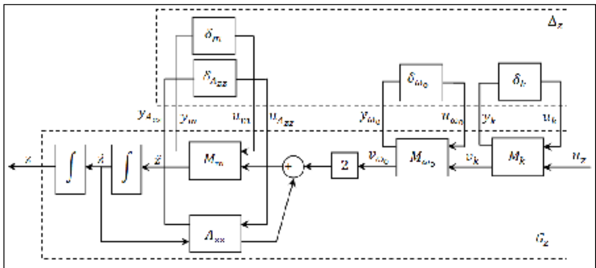
Figure 5.20 Structure de la chaîne d'élévation pour faire apparaître le contenu \Delta_z et G_z
