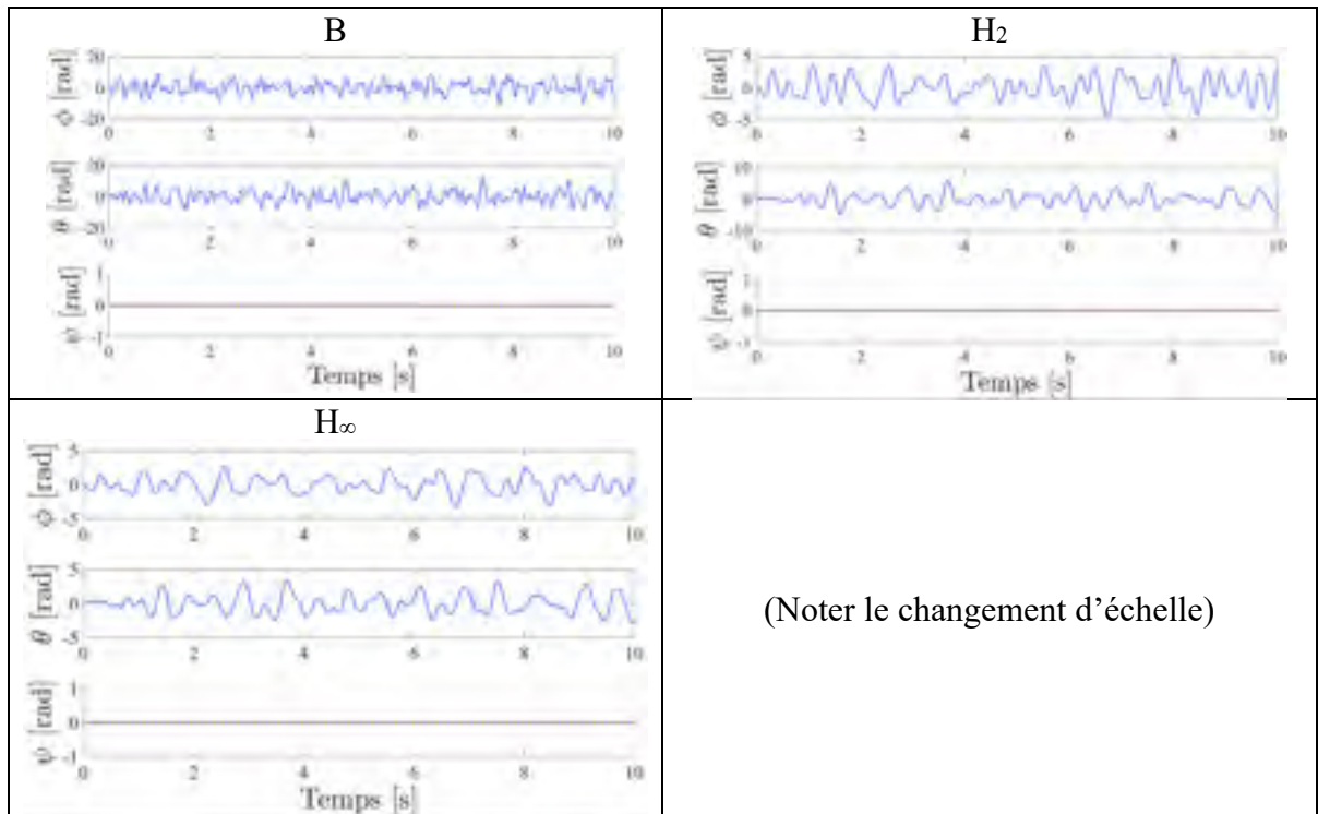
Figure 7.75 Déplacement autour des angles \phi , \theta , \psi lors d'un vol stationnaire en présence de perturbation sur la sortie pour les compensateurs B, H_2 , H_\infty appliqués sur le modèle linéaire de drone
