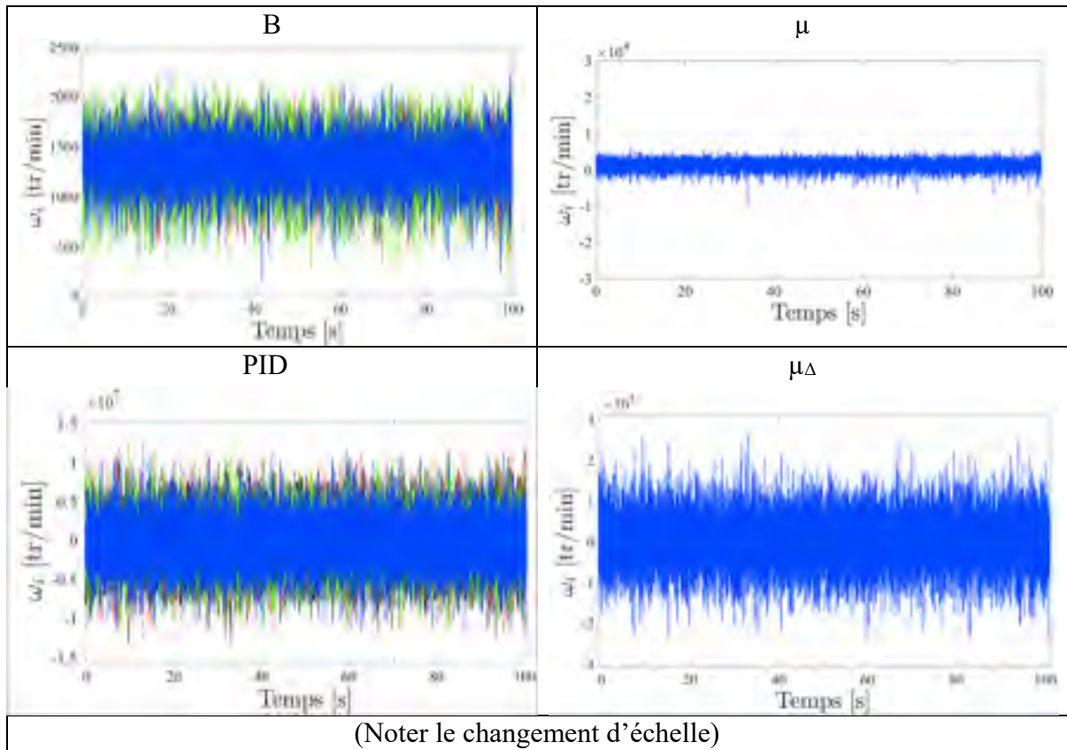
Figure 7.96 Vitesses \omega_1 (noire), \omega_2 (rouge), \omega_3 (verte), \omega_4 (bleue) lors d'un vol stationnaire en présence de perturbation en sortie pour les compensateurs B, \mu , \mu_\Delta , PID appliqués sur le modèle non linéaire de drone
