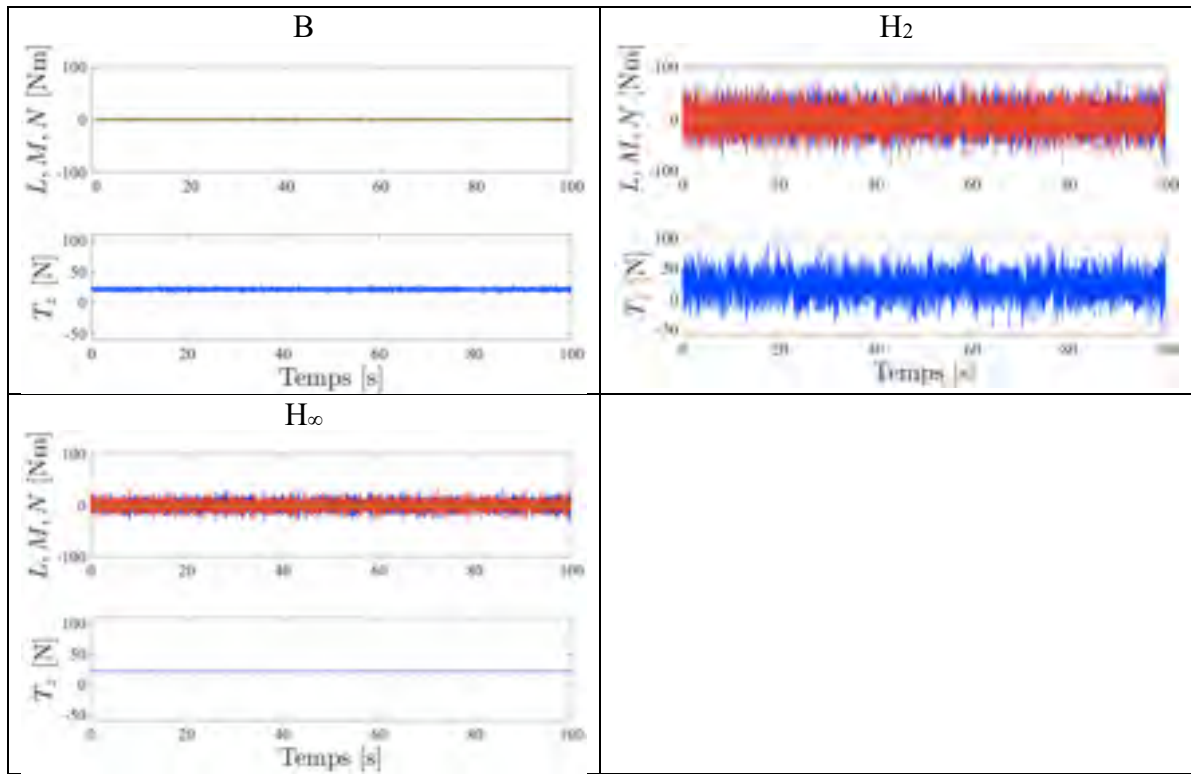
Figure 7.119 Commandes L (bleue), M (rouge), N (verte), T_z lors d'une consigne hélicoïdale définie en (7.4), présence de perturbation en sortie pour les compensateurs B, H 2 , H ∞ sur le processus non linéaire
