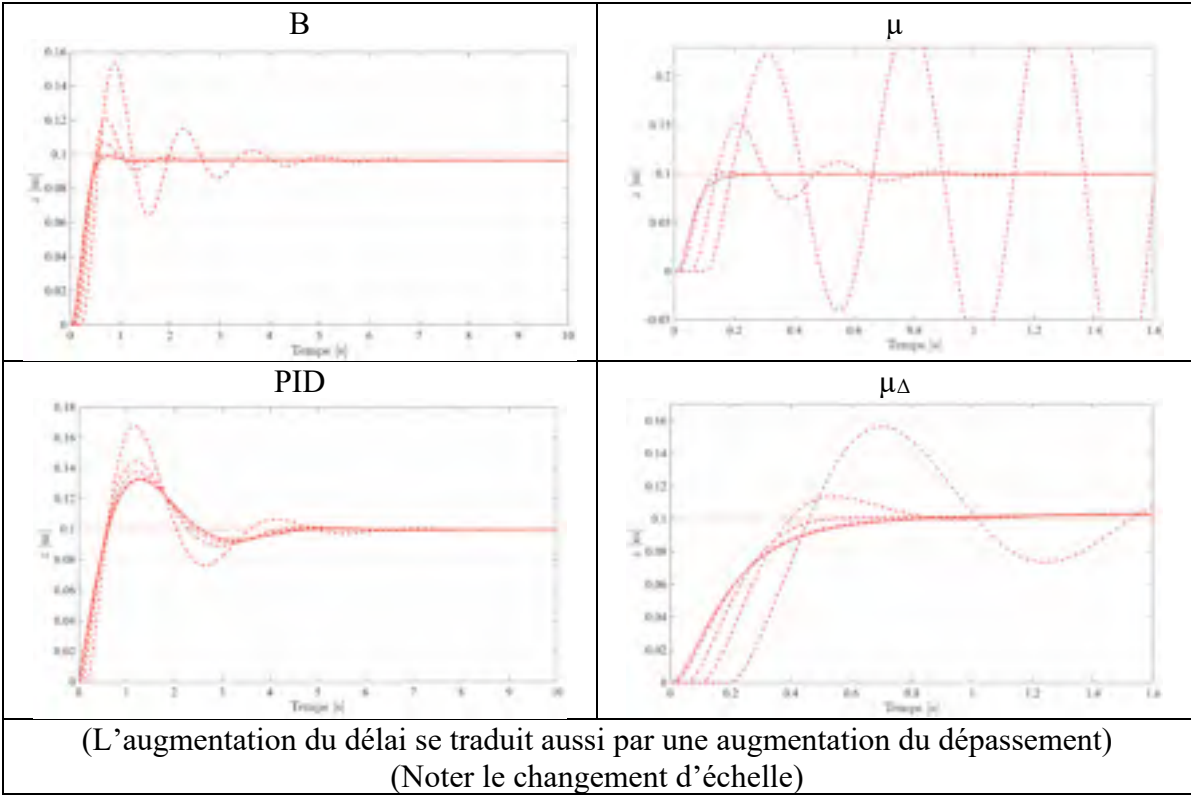
Figure 7.144 Réponses unitaires nominales en trait plein sur z et en pointillés avec l’ajout de délais de mesure, pour les compensateurs : B, \mu , PID, \mu_\Delta sur le processus non linéaire
