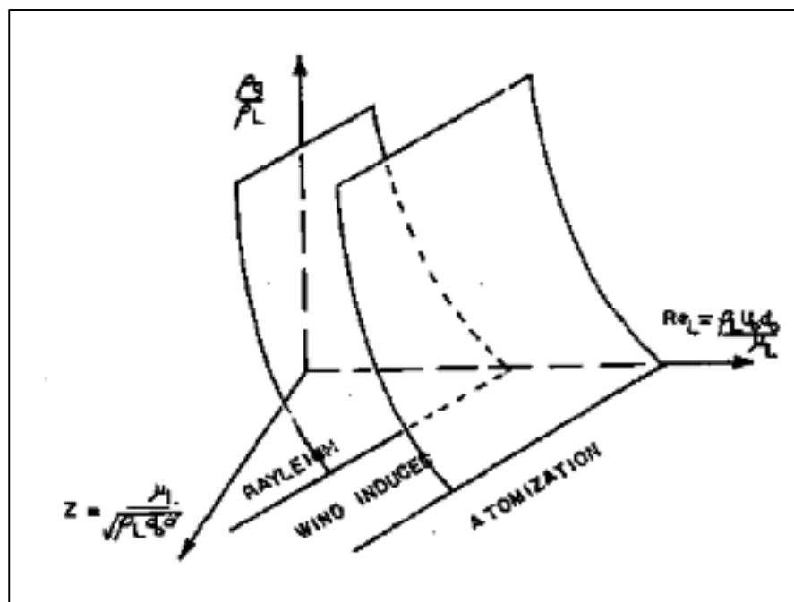
Figure-A I-2 Régions délimitant les mécanismes d'atomisation tiré de (Reitz, 1977).
