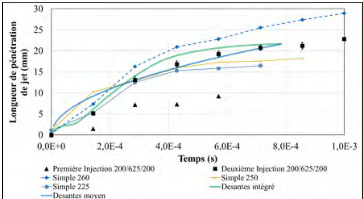
Figure 6.10 Comparaison des différentes méthodes de prédiction proposées à une seconde injection espacée de 625µs de la première (Pression d'injection de 900 bar et contrepression de 15 bar)
