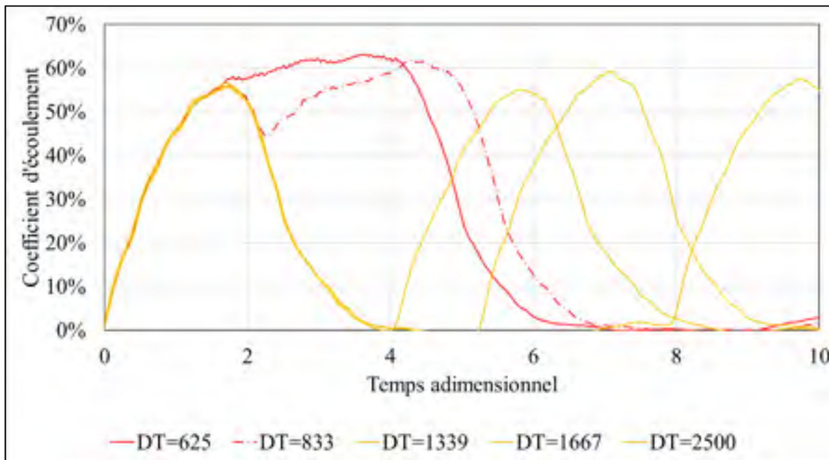
Figure 4.15 Profils de débits d'injections coupées d'un temps d'énergisation de 500 \mu\text{s} à une pression d'injection de 900 bar et contrepression de 30 bar
