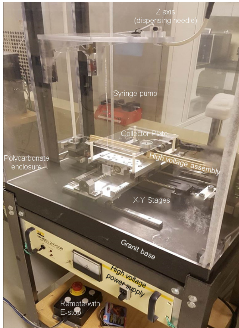
Figure 2.8 : Actual test bench
