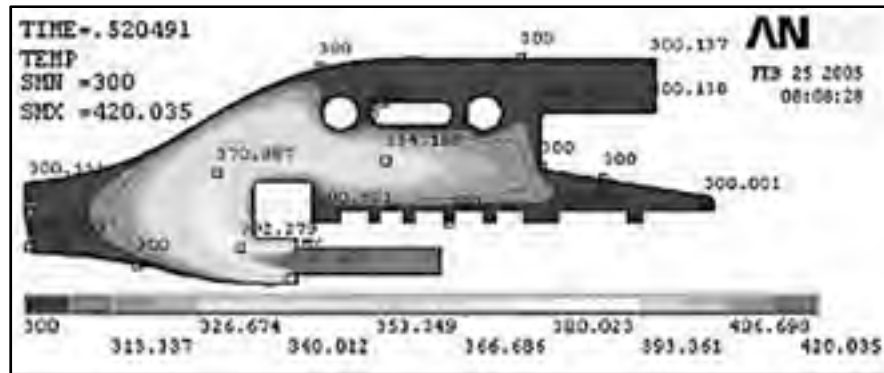
Figure 1.9 Distribution de la température à la fin de l'injection (Z. Zheng & Qu, 2006)
