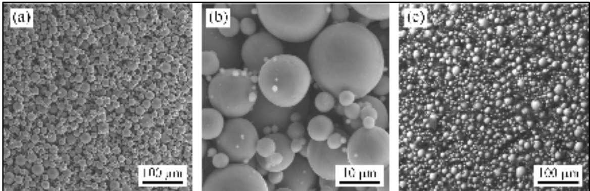
Figure 3.3 Observations au MEB de la poudre de titane selon différents grossissements: (a) \times 200 et (b) \times 2000 et (c) distribution de la poudre et du liant dans le mélange à un grossissement \times 200
