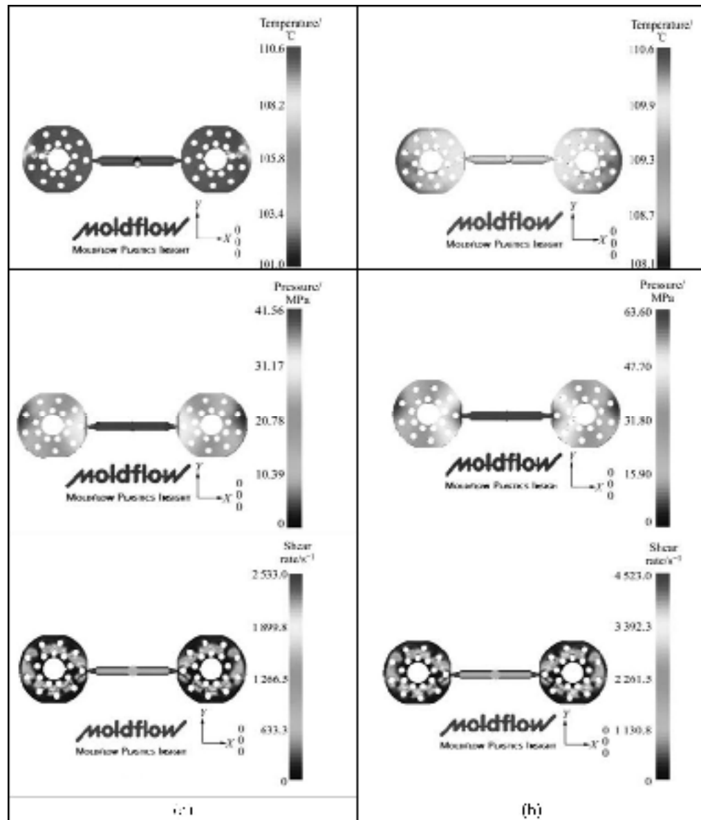
Figure 1.15 Visualisation de l'effet de variation du débit d'injection sur la température, la pression et le taux de cisaillement : (a) Débit = 10 \text{ cm}^3/\text{s} et (b) Débit = 20 \text{ cm}^3/\text{s} (Z.-X. Zheng et al., 2008)
