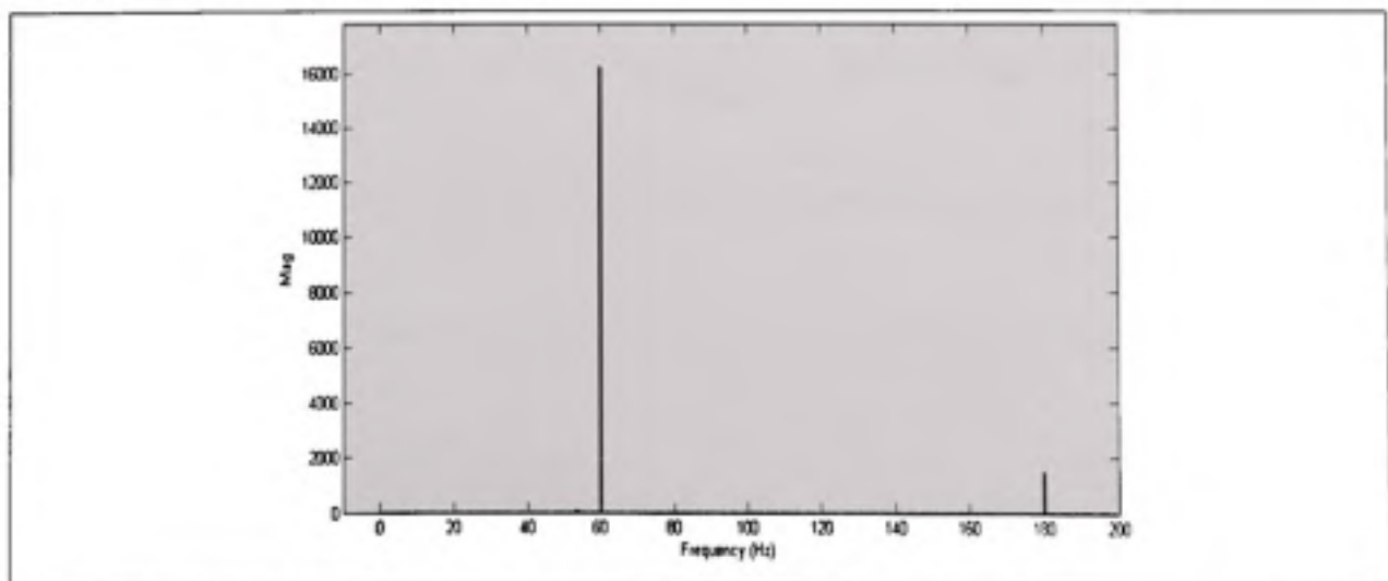
Figure 5-30 FFT de la tension aux bornes du compensateur défaut quatre cycles.
