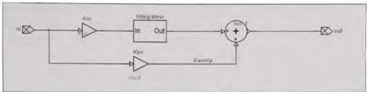
Figure 3-8 Schéma régulateur PI du compensateur.
