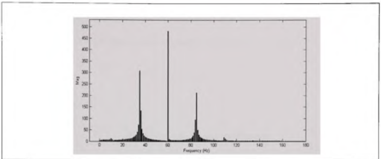
Figure 5-18 Transformée de Fourier discrète du courant dans la ligne.
