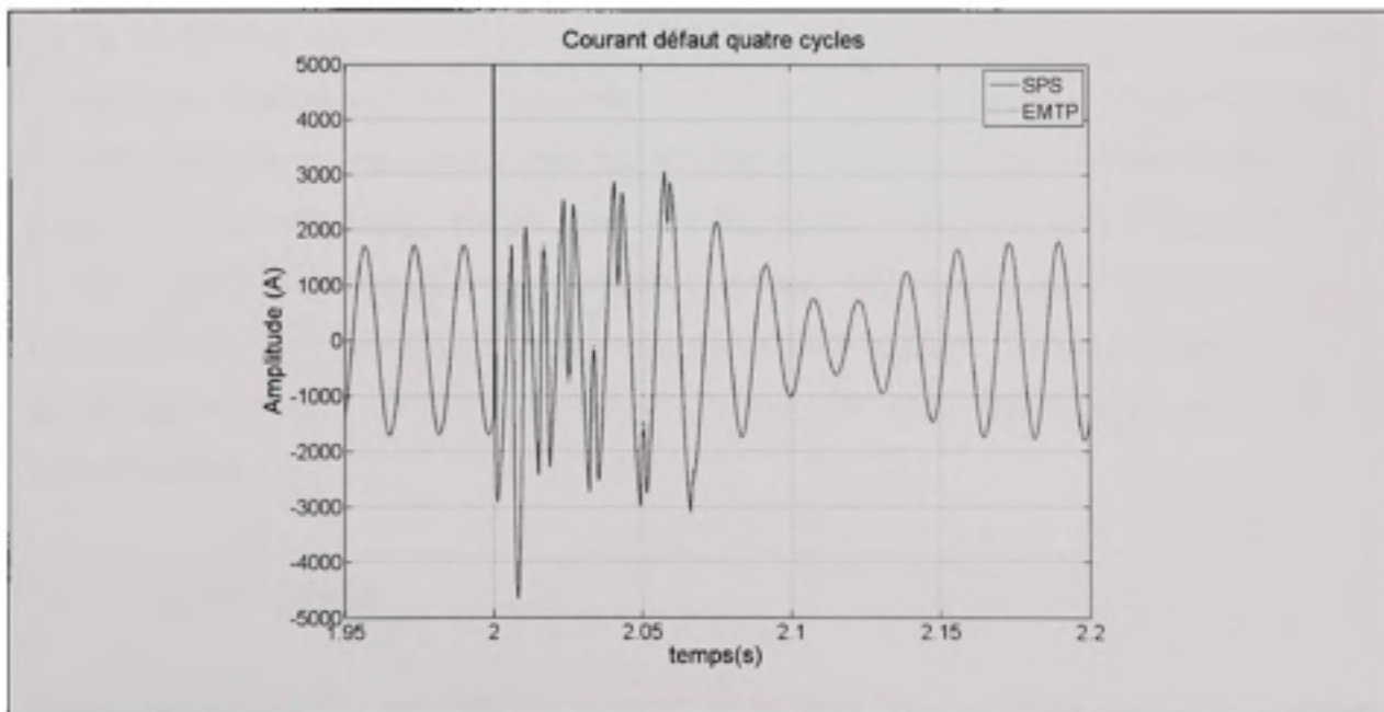
Figure 4-23 Forme du courant de ligne avec défaut monophasé.
