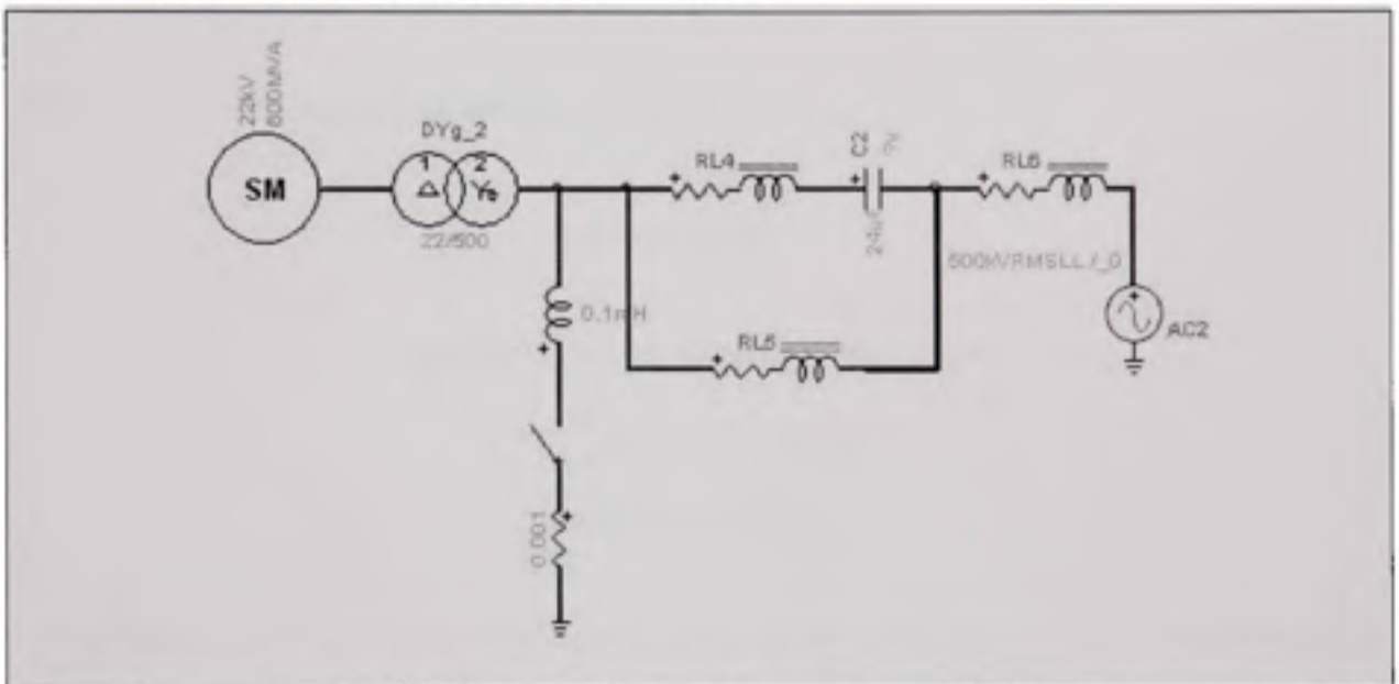
FigureAnnexe I.1 Modèle du second banc d'essai
