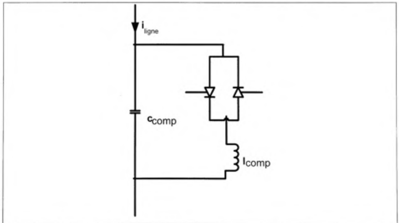
Figure 3-2 Schéma du compensateur série variable.
