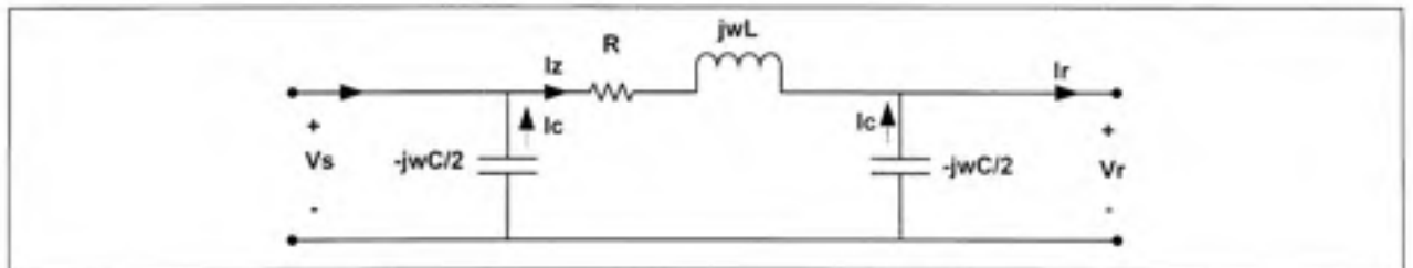
Figure 2-4 Modèle de la ligne moyenne avec pertes.
