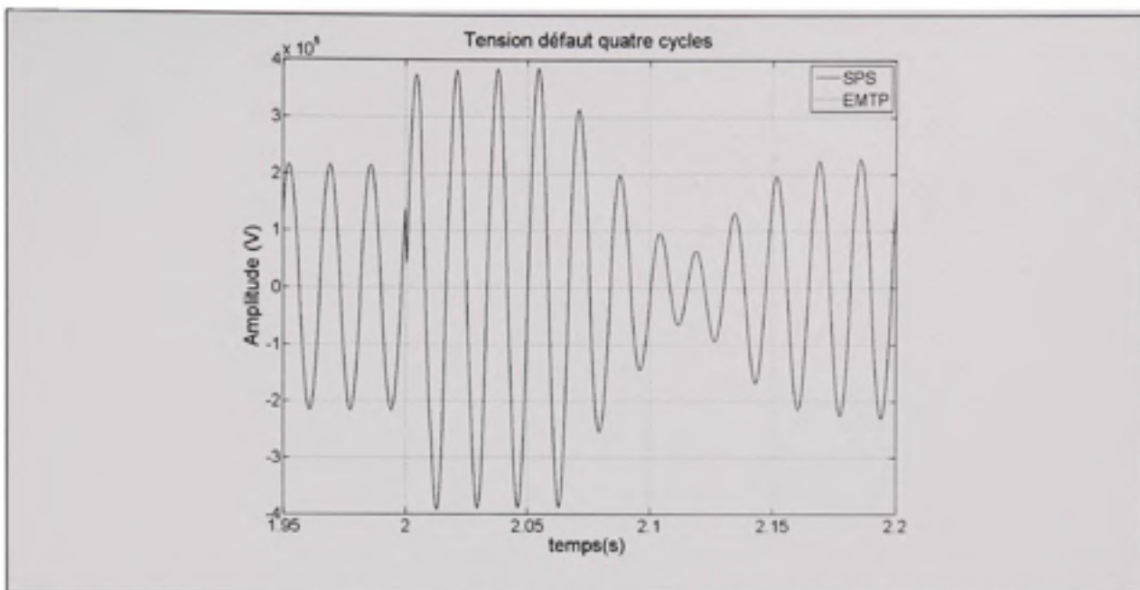
Figure 4-22 Tension aux bornes du compensateur avec défaut.
