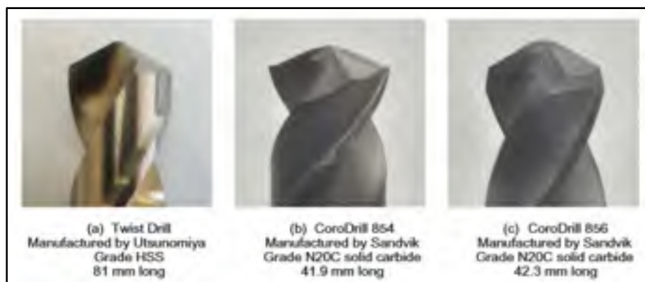
Figure 1.7 Les trois forets utilisés dans le perçage des FFRP (Rezghi Maleki et al., 2018)
