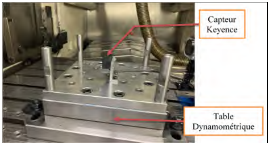
Figure-A III-1 Capteur de déplacement monté sur la table dynamométrique
