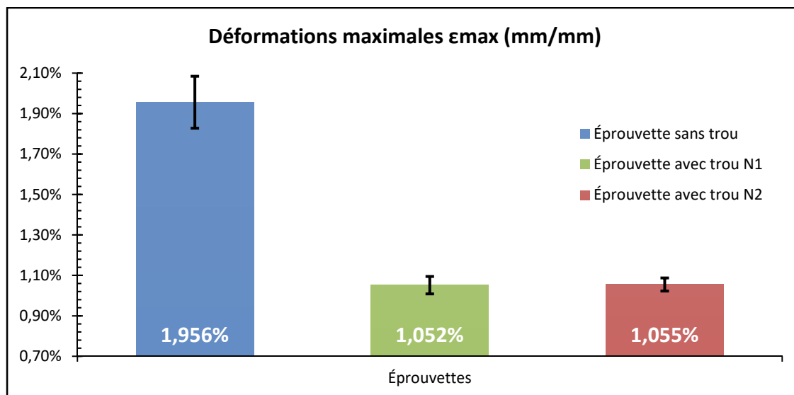
Figure 4.6 Déformations maximales des éprouvettes
