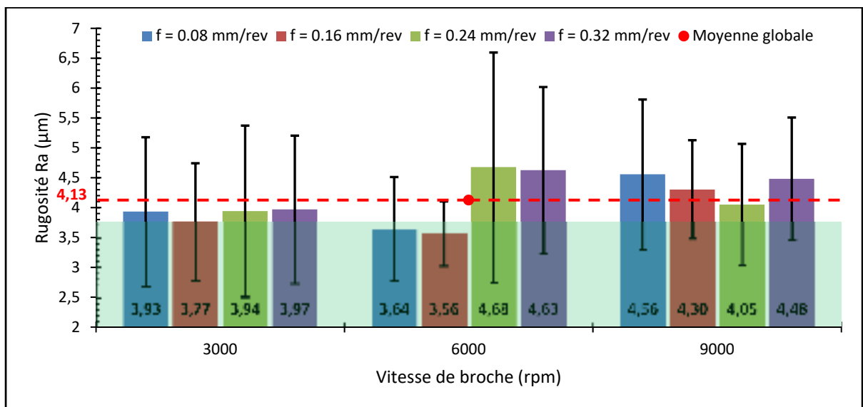
Figure 3.6 Rugosité en fonction des conditions de coupe - \overline{M(Ra)} = 4.13 \mu\text{m}
