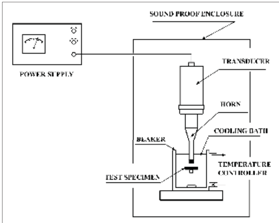
Figure 3.2 Représentation schématique du dispositif de test par cavitation vibratoire. Tirée et adaptée de ASTM (2016).
