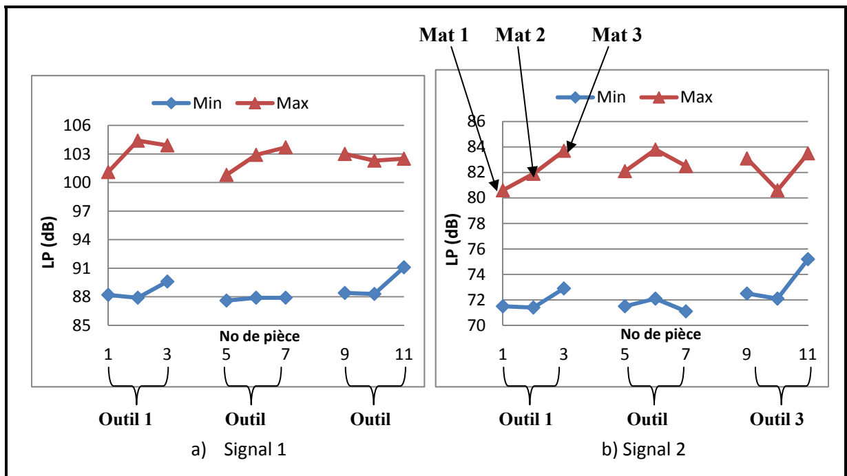
Figure 3.31 Zone de variation du niveau de pression acoustique en fonction des outils de coupe, des signaux et des conditions de coupe.
