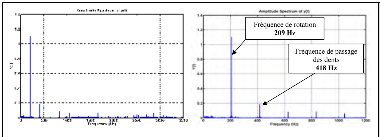
Figure 3.47 Représentation fréquentielle du signal avec V_c = 750\text{ m/min} A = 0,1\text{ mm/dent} Prof= 2 mm Mat : Al 2024 Revêt TiCN.
