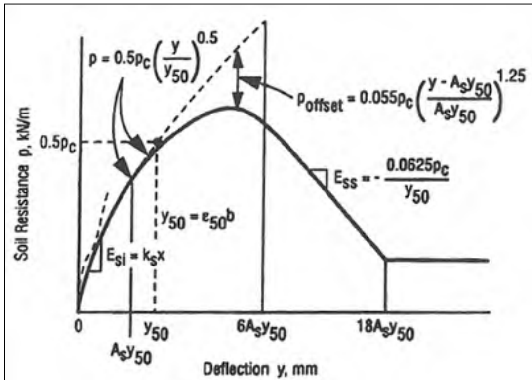
Figure 2.18 Courbes p - y caractéristique pour argiles raides submergées (chargement statique). Tiré de Reese et al.(2004)
