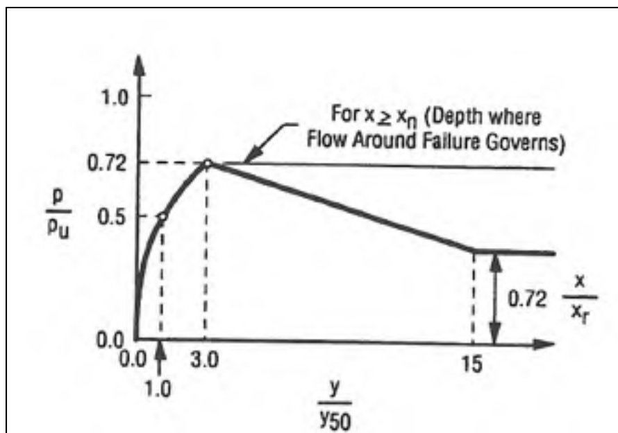
Figure 2.17 Courbe p - y caractéristique pour des argiles molles submergées (chargement cyclique). Tiré de Reese et al. (2004)
