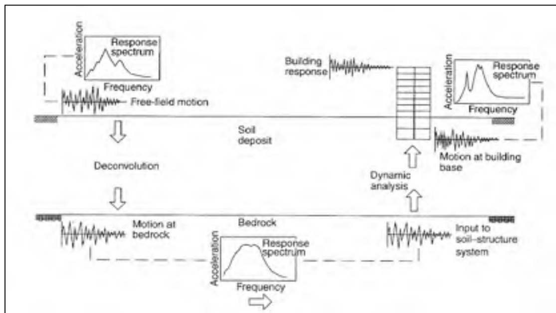
Figure 1.1 Schéma de la méthode globale pour prendre en compte les effets de l'ISS. Tiré de Villaverde (2009)
