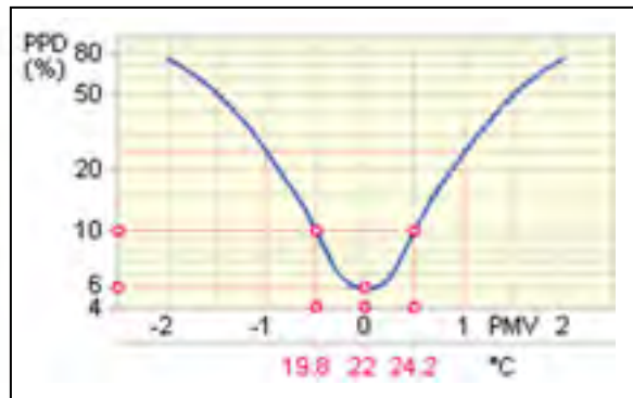
Figure 2.8 Illustration : PMV-PPD Tirée de Louvain (2011)
