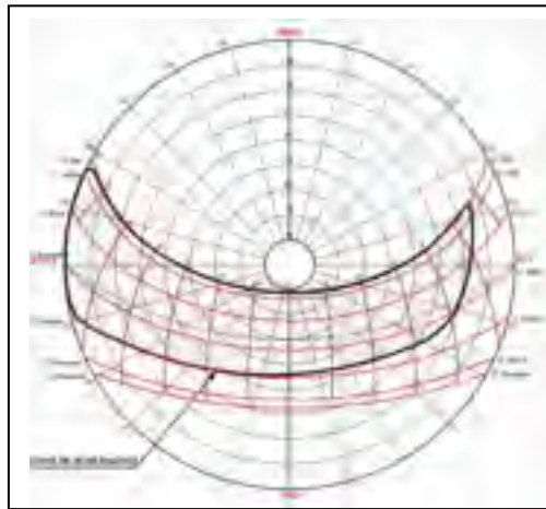
Figure 3.6 Diagramme polaire de Biskra (présentation de la zone de surchauffe en noir)
