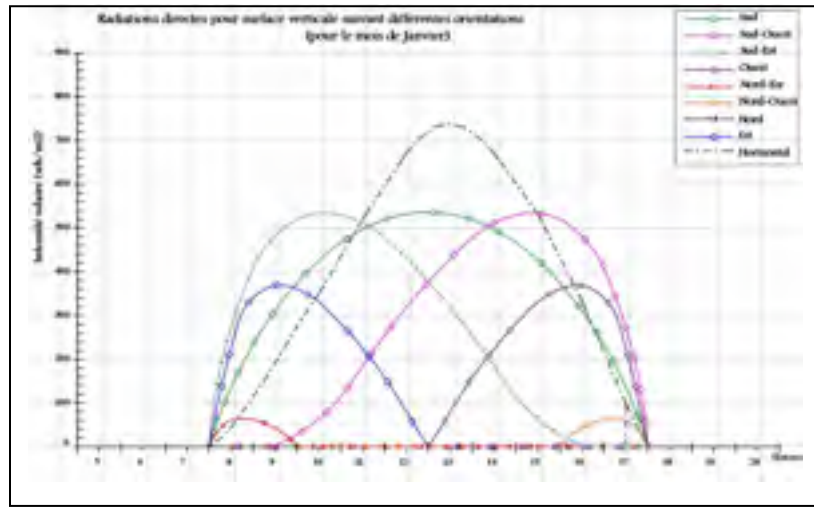
Figure 3.12 Diagramme de radiations solaires de Biskra mois de janvier Adaptée de Capderou (1985, pp. 140-149)
