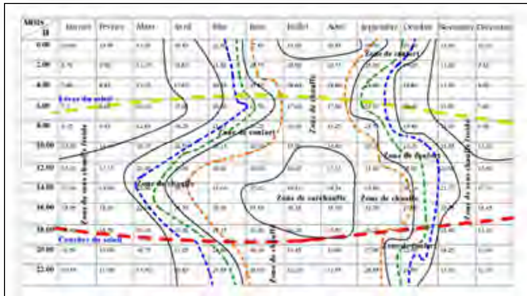
Figure 2.11 Courbes d'égalité de température (isoplèthes) par mois et en heures de Biskra
