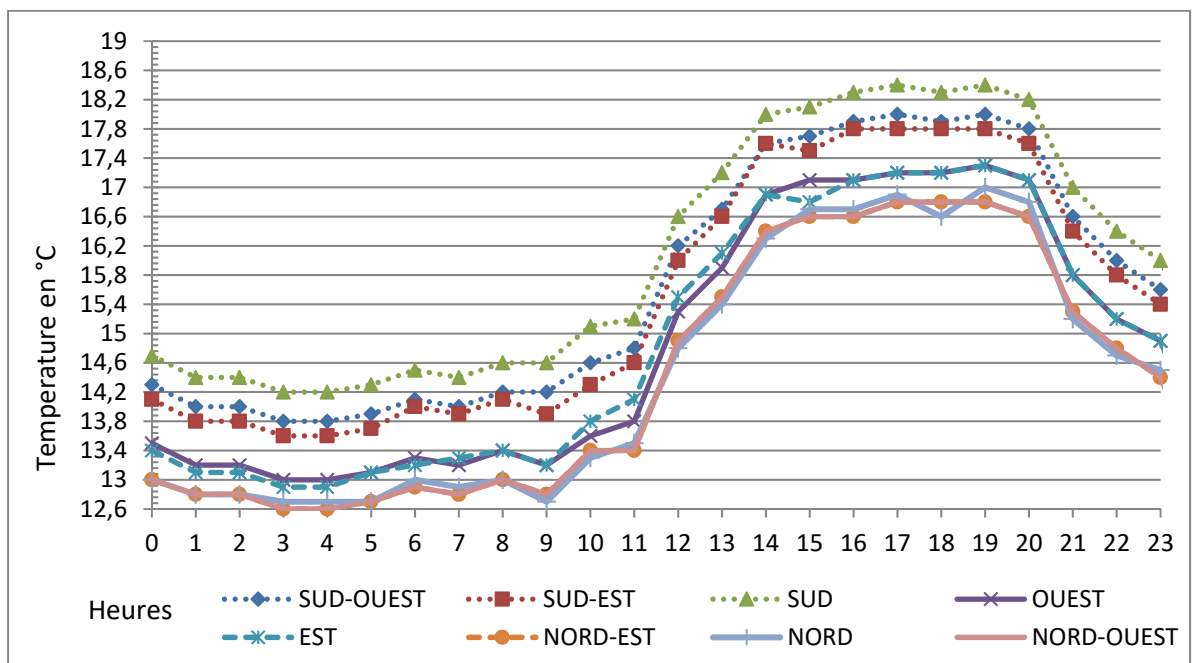
Figure 5.8 Comparaison des températures intérieures simulées des différentes orientations pendant la période d'hiver
