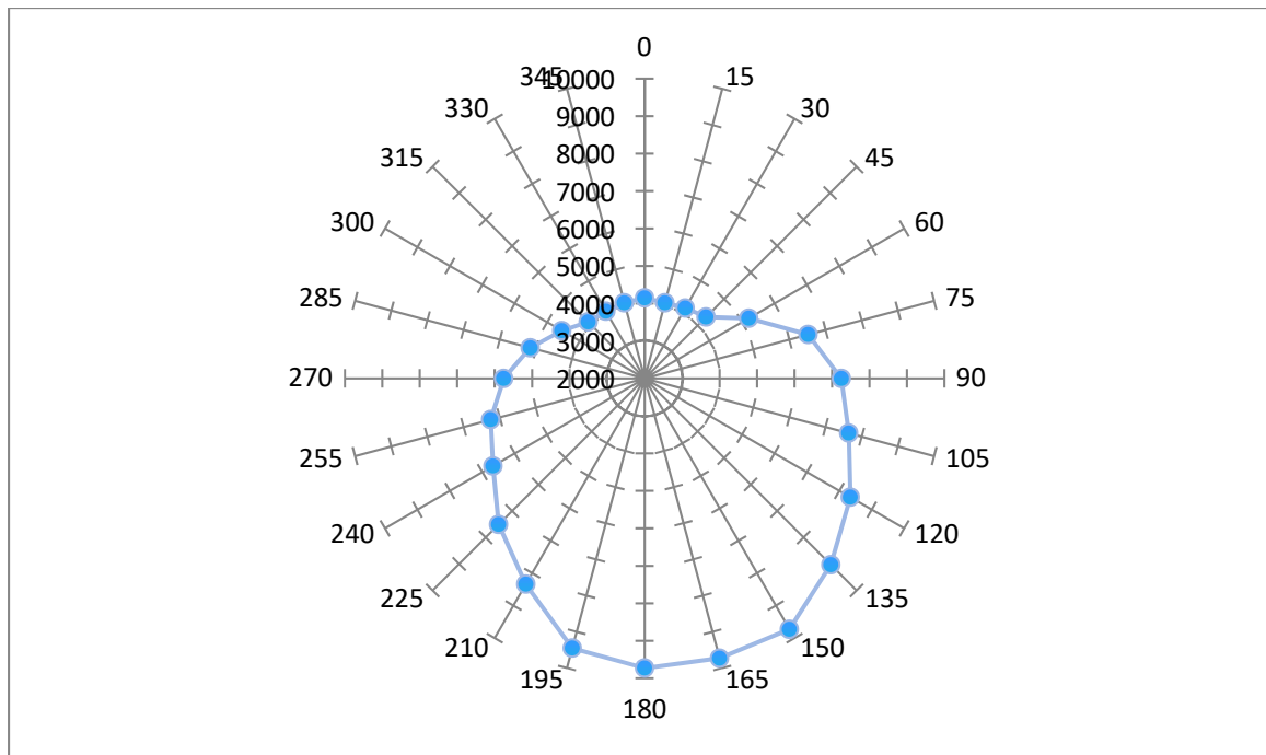
Figure 5.10 Total des radiations solaires absorbées en W/m^2 suivant l'orientation par le mur extérieur pendant la période hivernale
