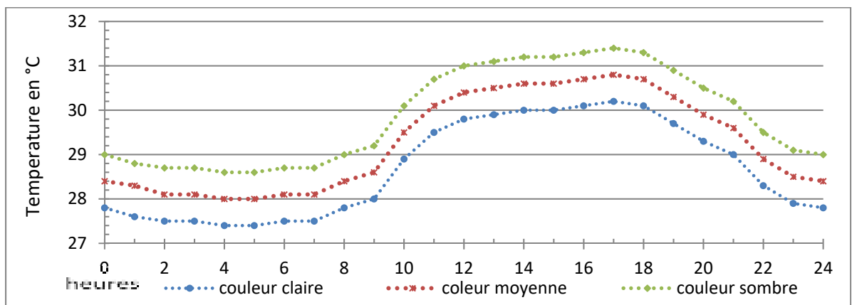
Figure 5.13 Effet de la couleur sur la température intérieure orientation Est
