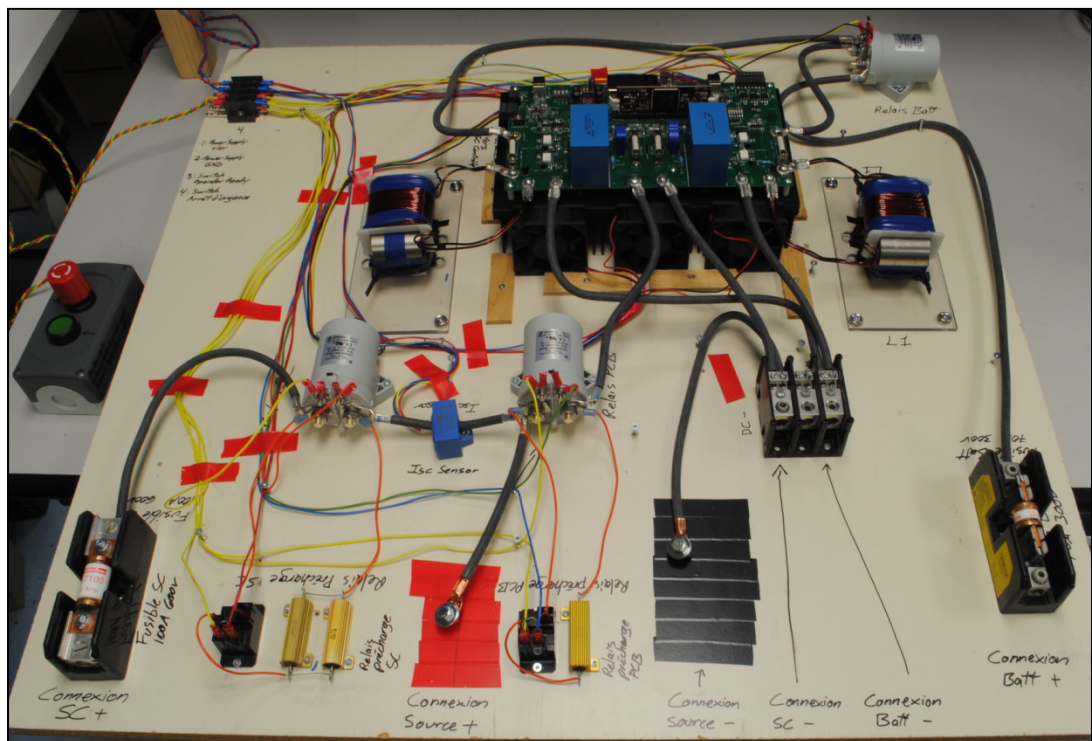
Figure 4.6 Convertisseur expérimental
