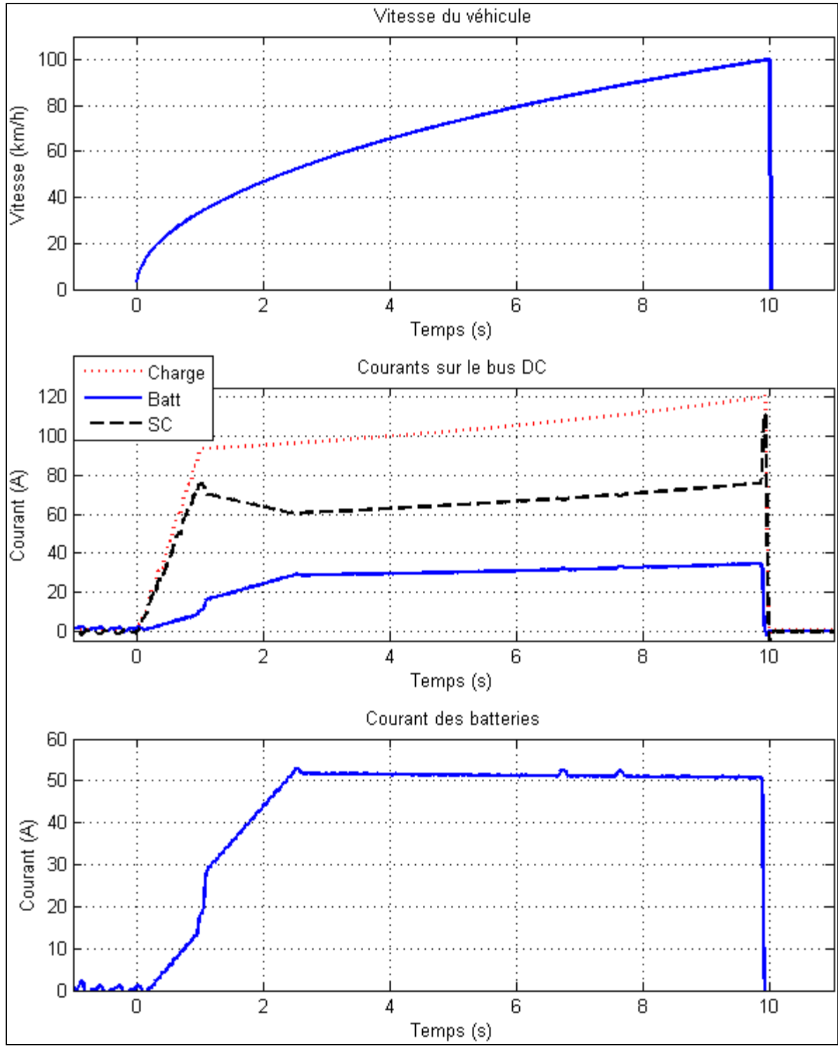
Figure 4.17 Courants expérimentaux du test d'accélération maximale
