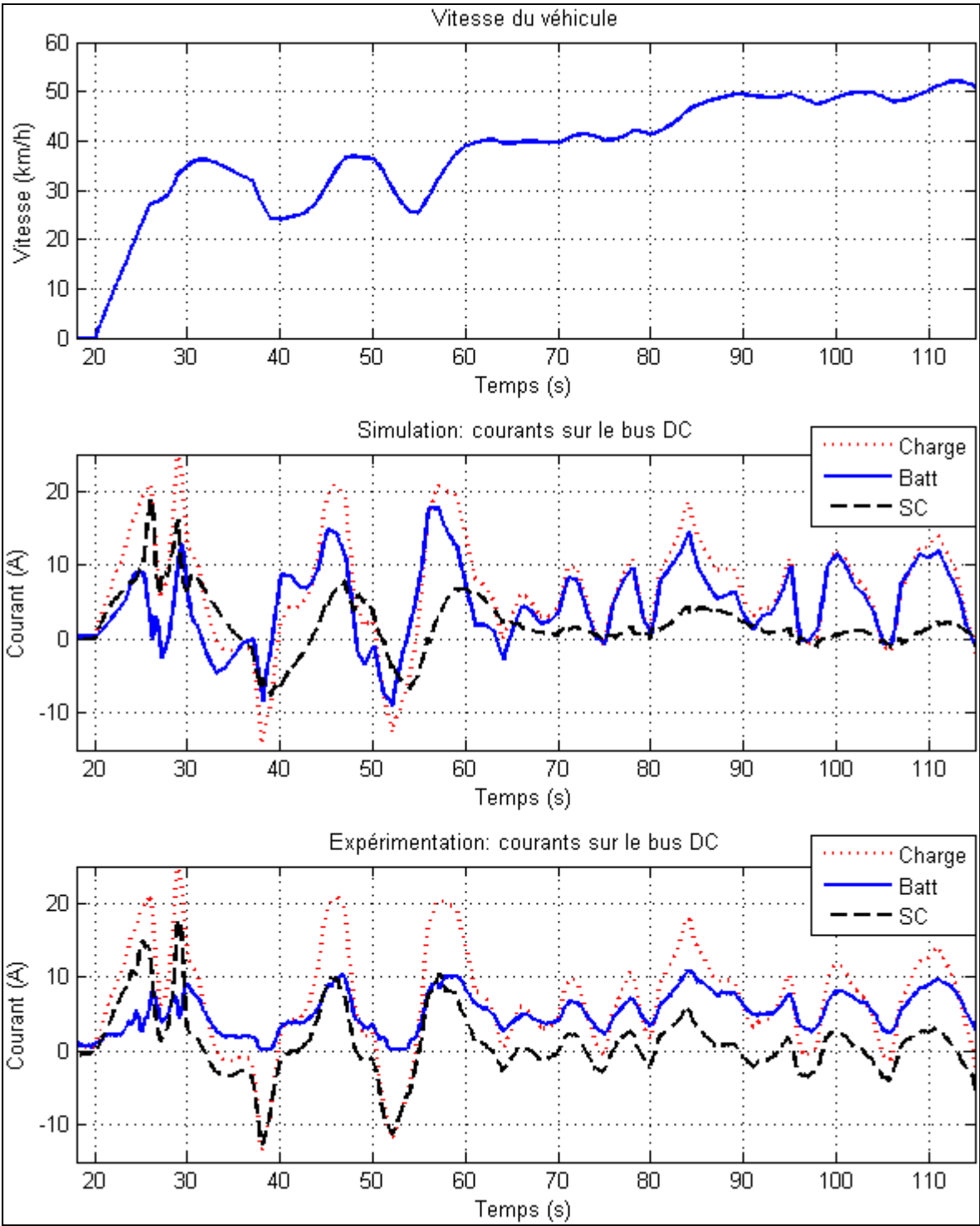
Figure 4.18 Courants simulés et expérimentaux démontrant la répartition des puissances
