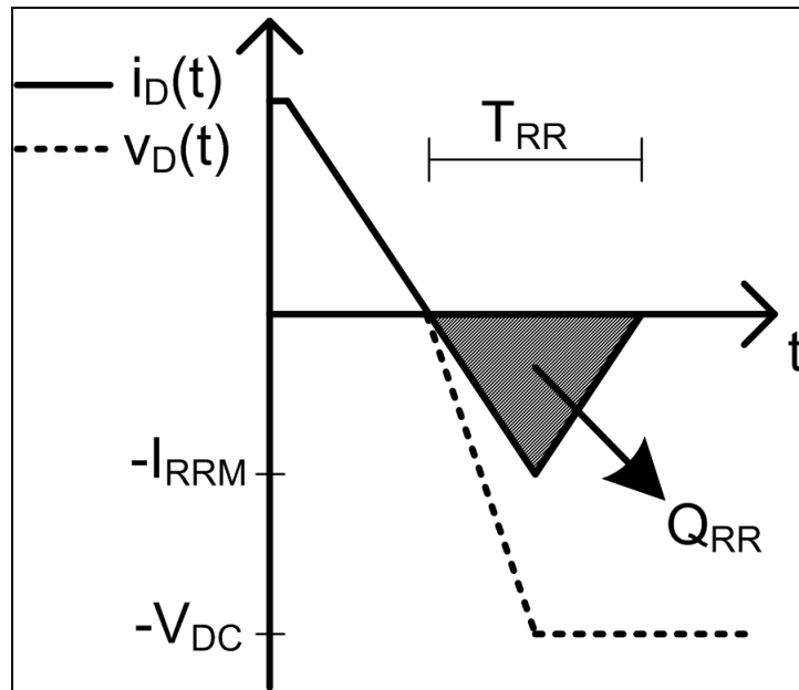
Figure 3.11 Évolution simplifiée du recouvrement inverse
