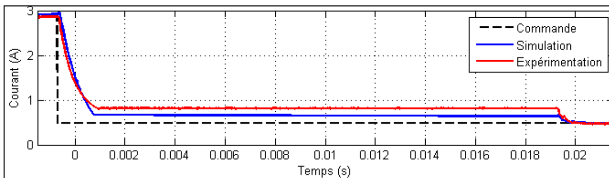
Figure 4.13 Courant HV moyen simulé et expérimental lors d'une transition du mode de conduction continue à discontinue
