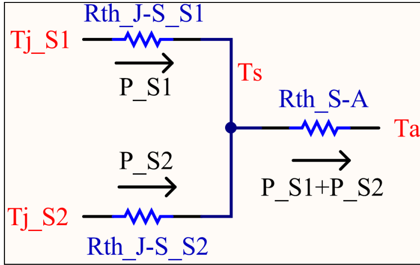
Figure 3.12 Modèle thermique du système interrupteurs-radiateur
