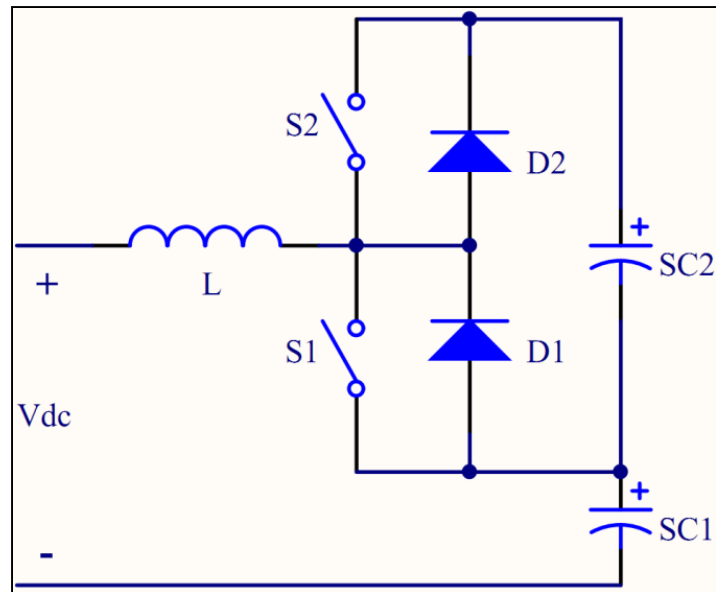
Figure 1.19 Convertisseur en cascade demi-contrôlé
