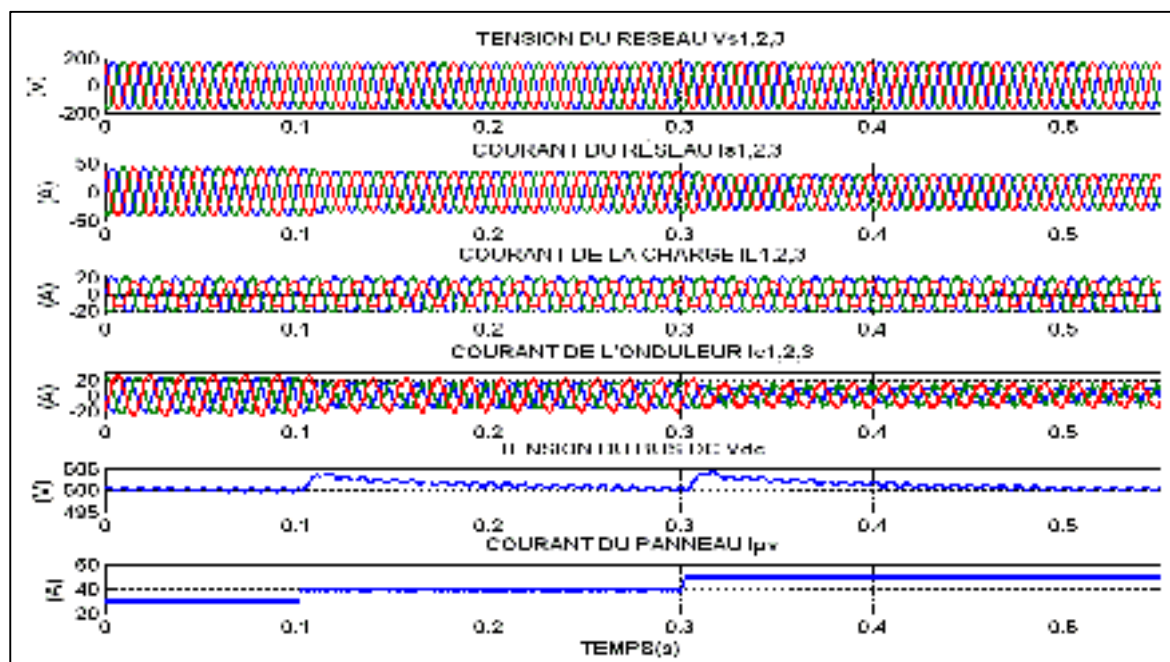
Figure 4.29 Réponse en régime dynamique avec variation de l'ensoleillement
