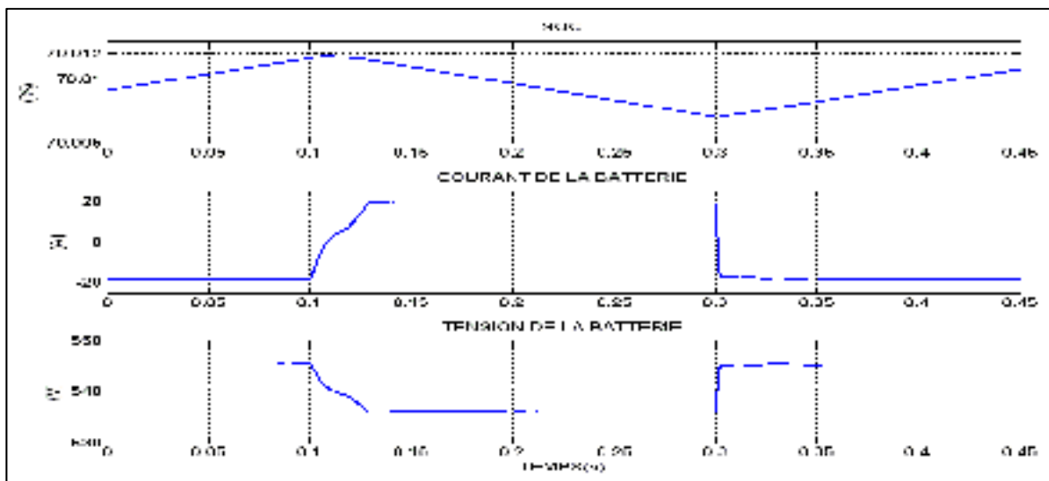
Figure 4.36 État de charge de la batterie
