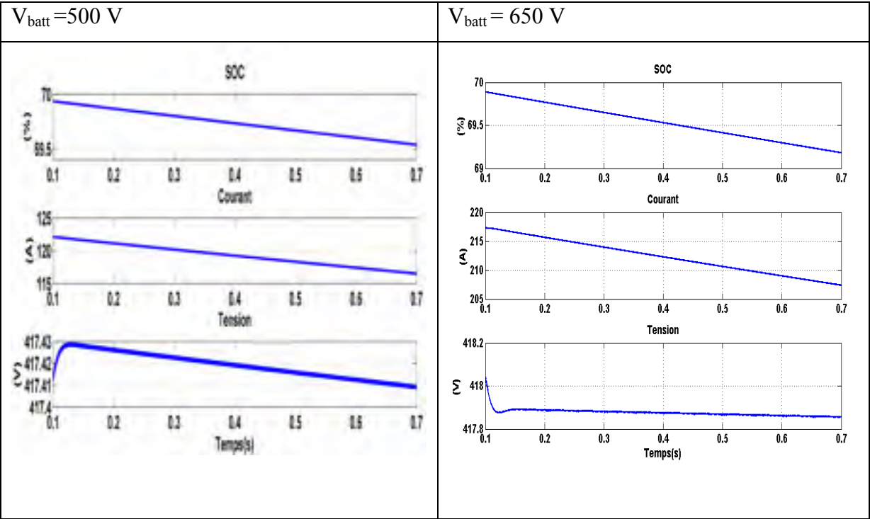
Figure 2.24 Résultat de simulation avec Buck-Boost pour V_{batt}=500 et 650\text{V}
