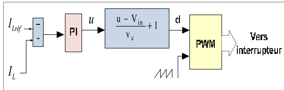
Figure 4.3 Schéma de la commande du convertisseur Boost
