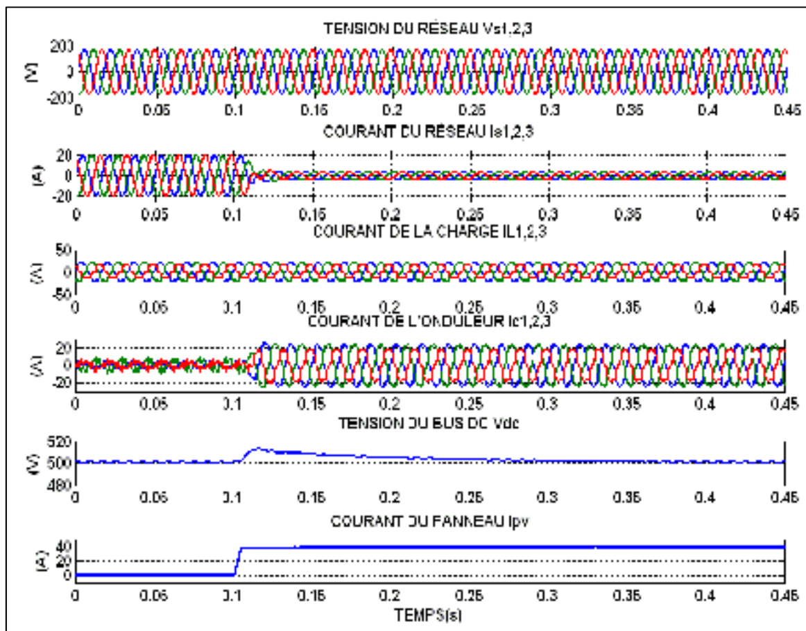
Figure 4.21 Réponse en régime dynamique avec ensoleillement G=800W/m^2
