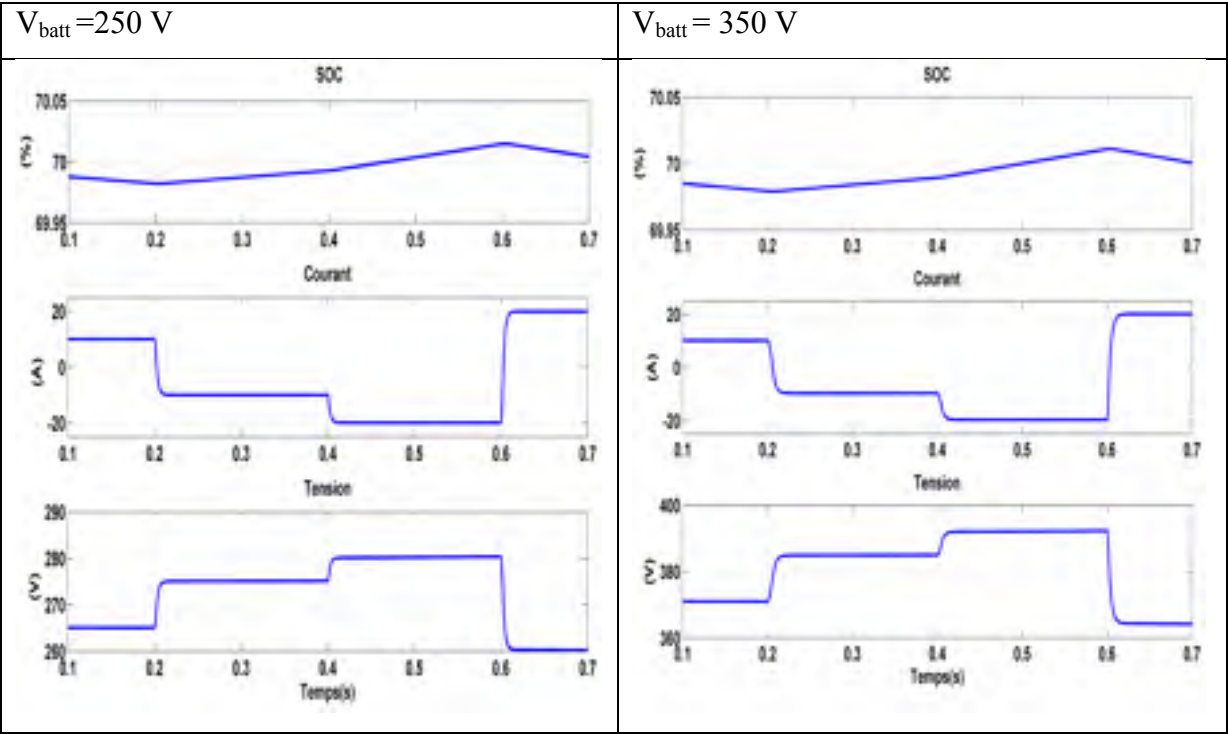
Figure 2.23 Résultat de simulation avec Buck-Boost pour V_{batt}=250 et 350\text{V}
