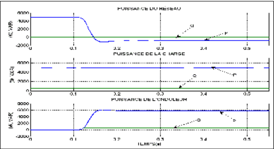
Figure 4.43 Écoulement de puissance avec ensoleillement G=800W/m^2
