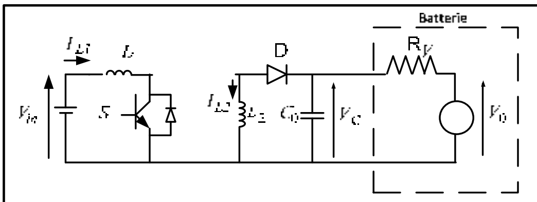
Figure 2.14 Schéma du montage du convertisseur Sepic lorsque l'interrupteur est passant
