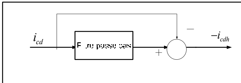
Figure 4.6 Schéma du principe d'extraction des courants harmoniques
