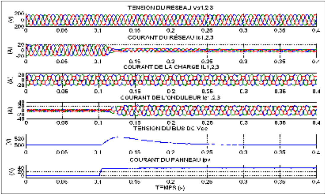
Figure 4.42 Réponse dynamique avec ensoleillement G=800W/m^2
