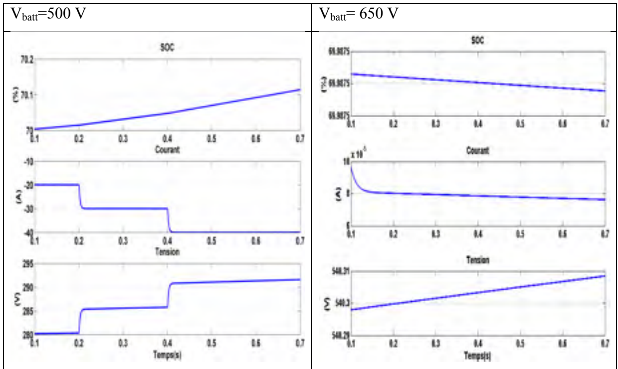
Figure 2.12 Résultat de simulation avec Buck pour V_{batt}=500 et 650 \text{ V}
