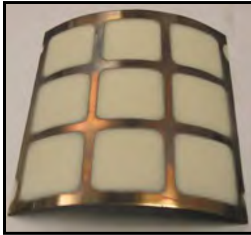
Figure 2.12 Capteurs piézoélectriques
