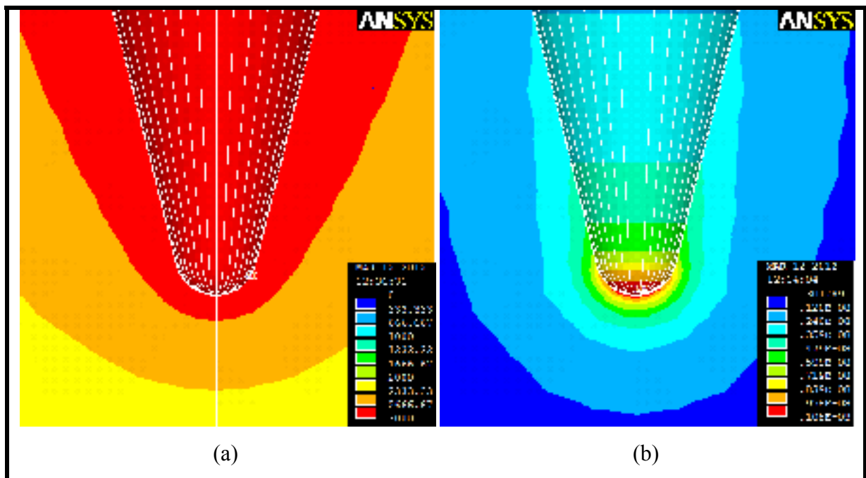
Figure 4.5 Profil du potentiel (a) et du champ électrique (b) dans l'air pour V_a = 3 \text{ kV}
