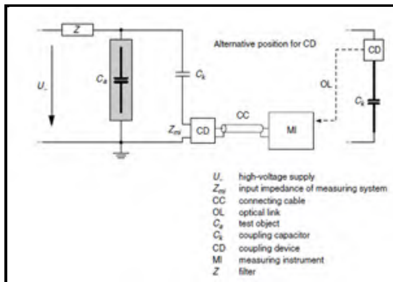
Figure 2.4 Diagramme conventionnel de mesure de DP par la méthode couplage capacitif Tirée de Power & Energy Society (2009, p.32)
