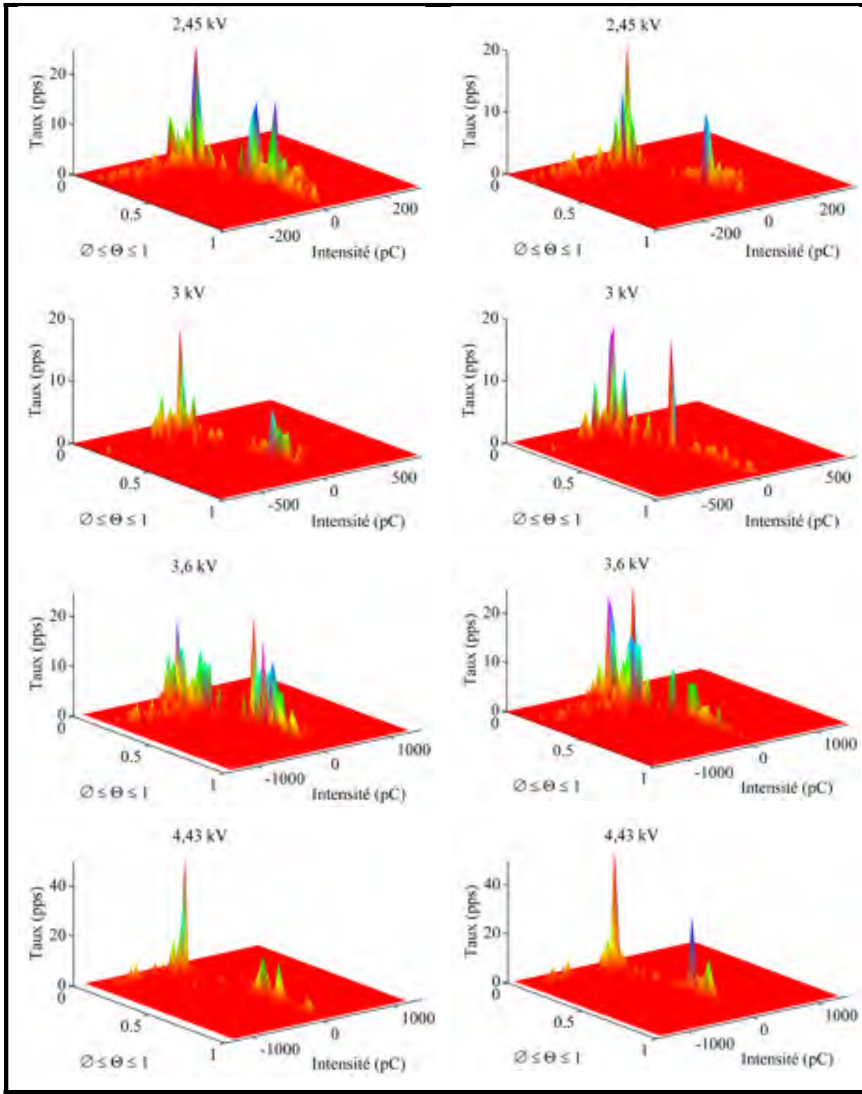
(a) (b) Figure 5.8 DRPDP 3D a) Piézoélectrique BIT/PZT b) Coupleur capacitif
