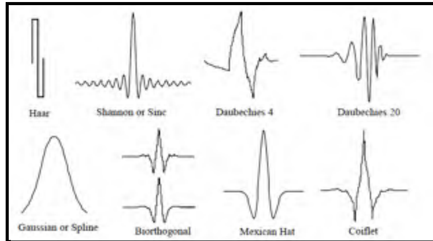
Figure 4.13 Quelques ondelettes mères (Fugal, 2009)
