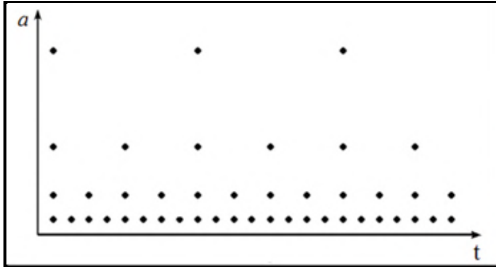
Figure 4.17 Espace temps-échelle sur une grille dyadique
