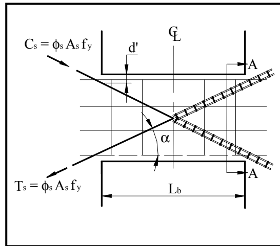
Figure 1.7 Poutres de couplage - disposition diagonale de l'armature principale
