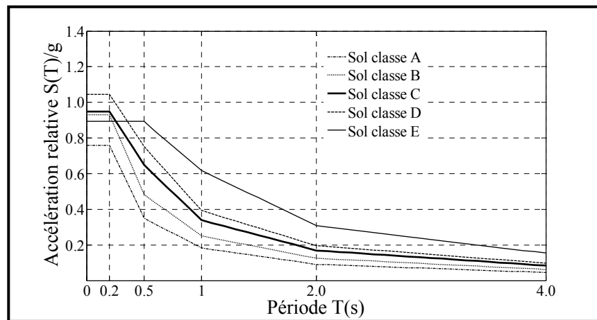
Figure 1.5 Spectres de dimensionnement de la ville de Vancouver
