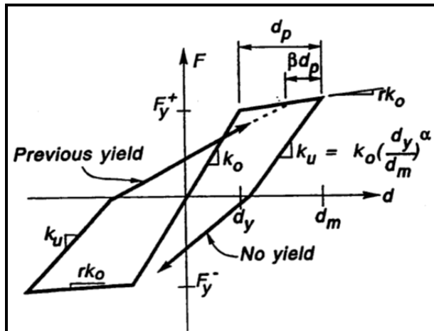
Figure 5.1 Loi de comportement hystérétique - Takeda modifiée (S. Otani, 1974)
