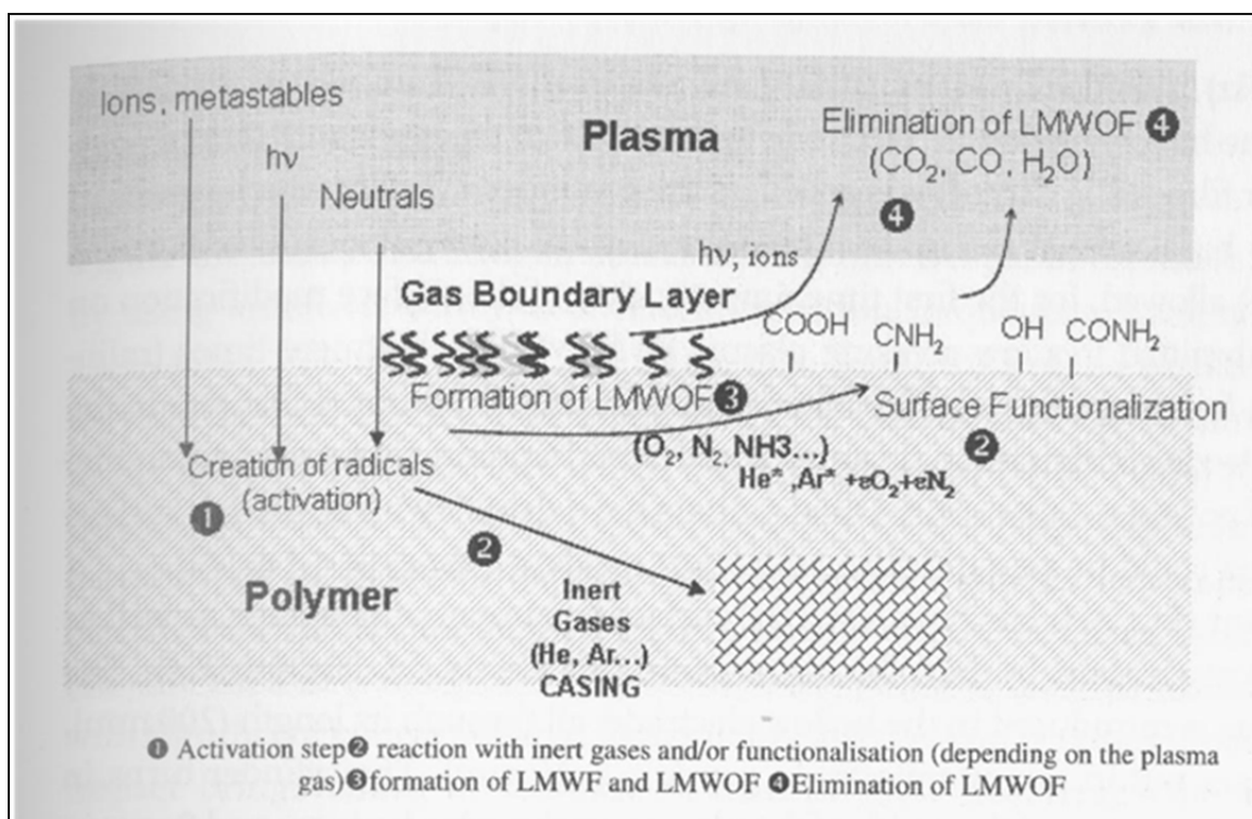
Figure 1.11 Interactions plasma-polymère dans un traitement de surface des polymères : 1, étape d'activation; 2, réaction avec les gaz inertes et/ou fonctionnalisation (dépendamment du gaz plasma utilisé); 3, formation de fragments de faible poids moléculaire (LMWF) et de fragments oxydés de faible poids moléculaire (LMWOF) ; 4, élimination des LMWOF (Arefi-Khonsari et Tatoulian, 2008)
