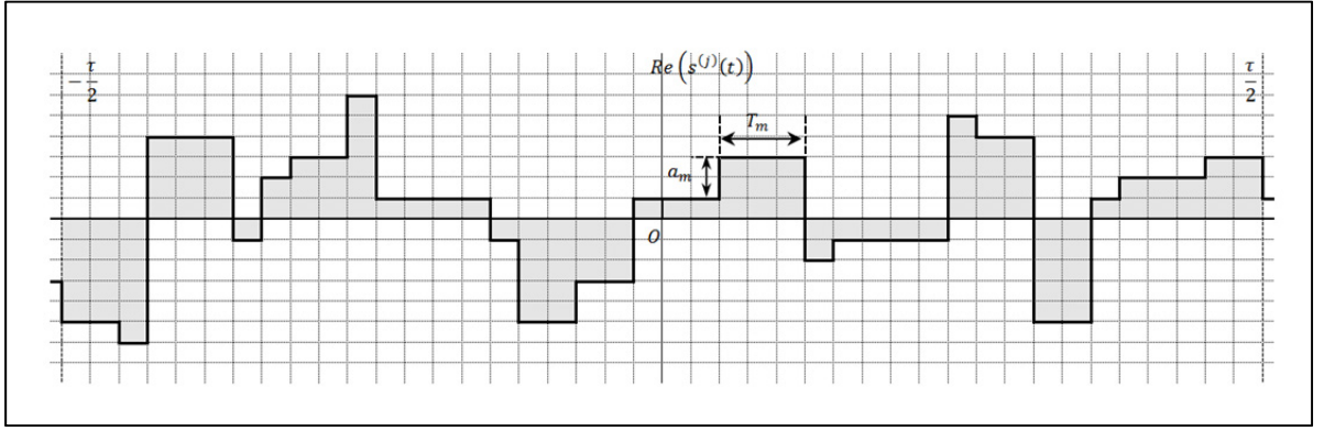
Figure 4.1 Signal à modulation d'amplitude à durée d'impulsion aléatoire
