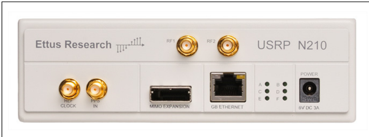
Figure 5.3 Vue de face du périphérique USRP N210
