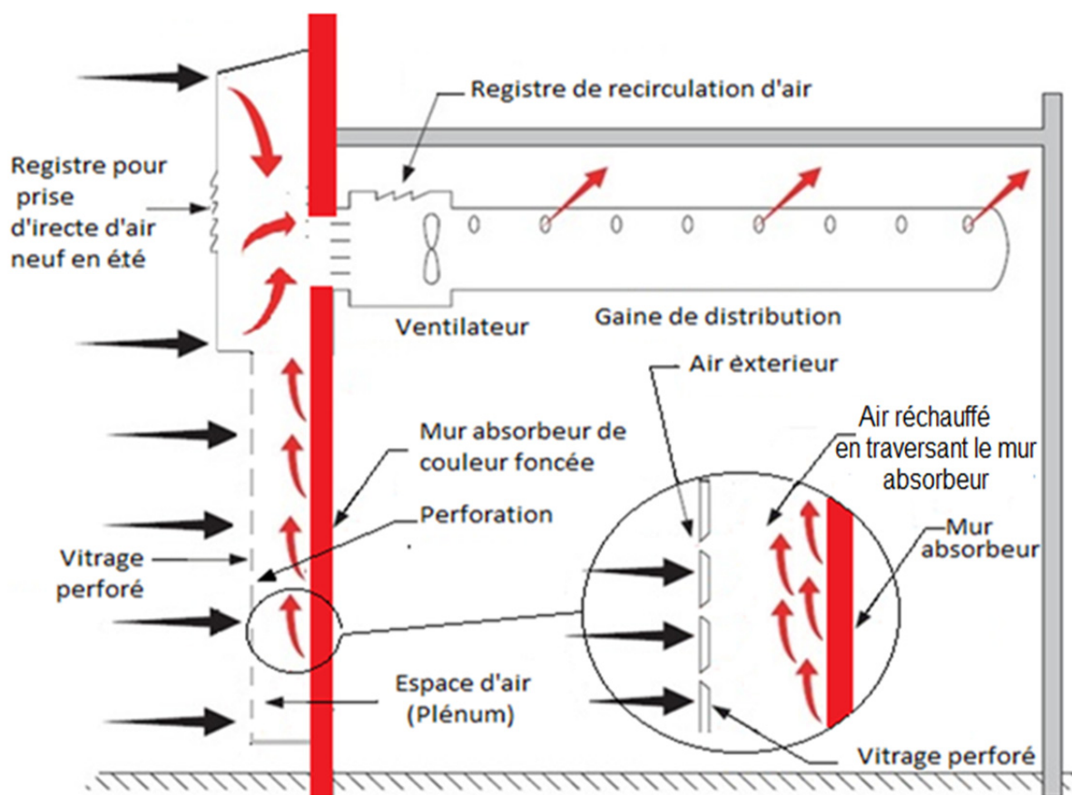
Figure 0.4 Schéma d'un SCSA à vitrage polymère perforé.
