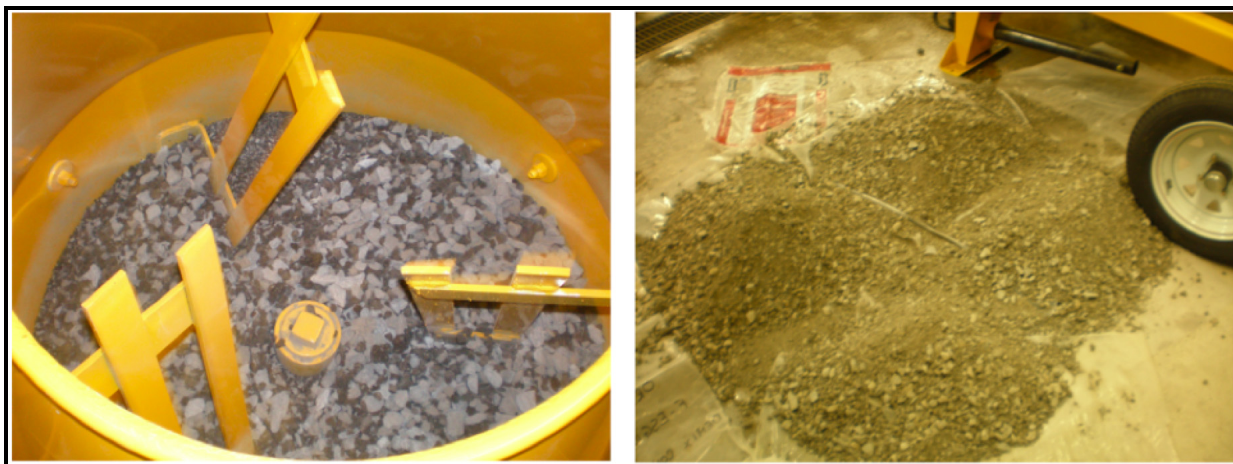
Figure 2.3 Malaxage et séparation du MR-5
