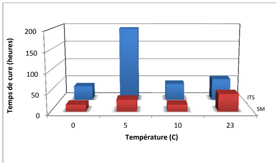
Figure 4.9 Temps pour atteindre le 75% de la résistance pour les deux méthodes d'essai
