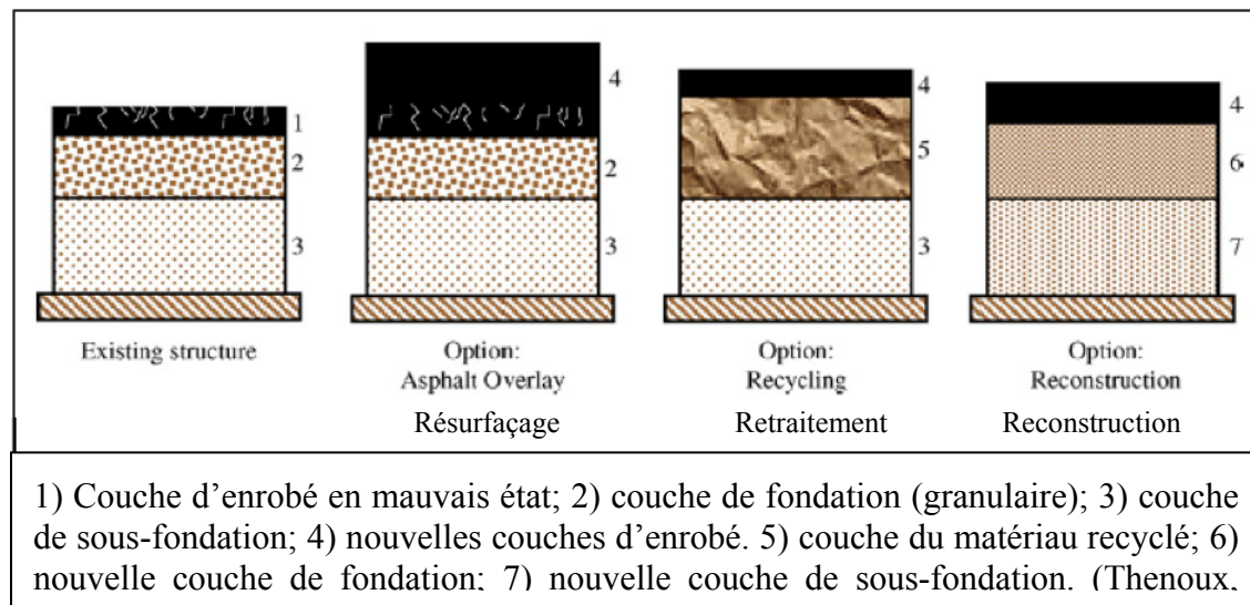
Figure 1.2 Schéma d'une chaussée existante et des techniques de réhabilitation éventuelle Tirée de (Thenoux, Gonzalez et Dowling, 2007).
