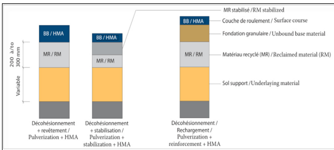
Figure 1.4 Principes techniques pour le décohesionnement (Bergeron, 2006b)
