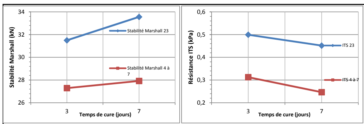
Figure 4.19 Résistances à 3 et 7 jours pour deux températures de cure
