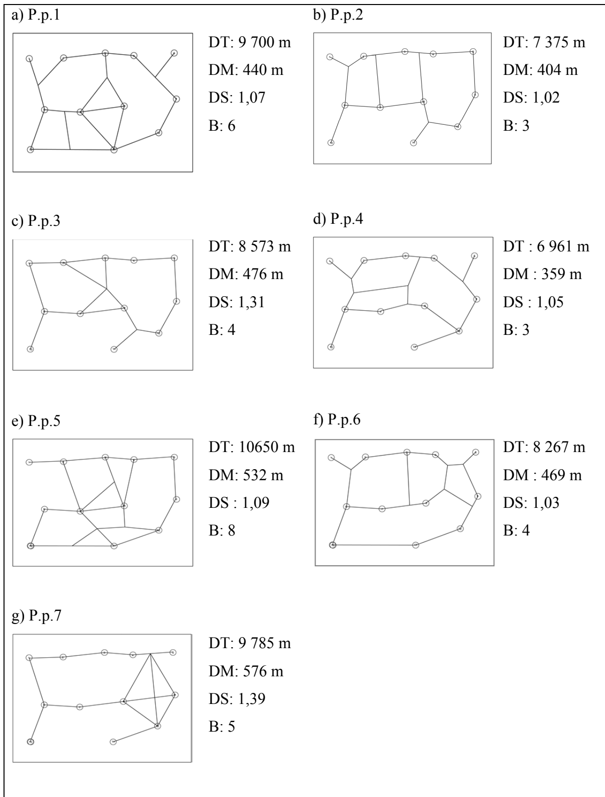
Figure 3.1 a) à g) Configurations des réseaux obtenus à l'aide du modèle biologique
