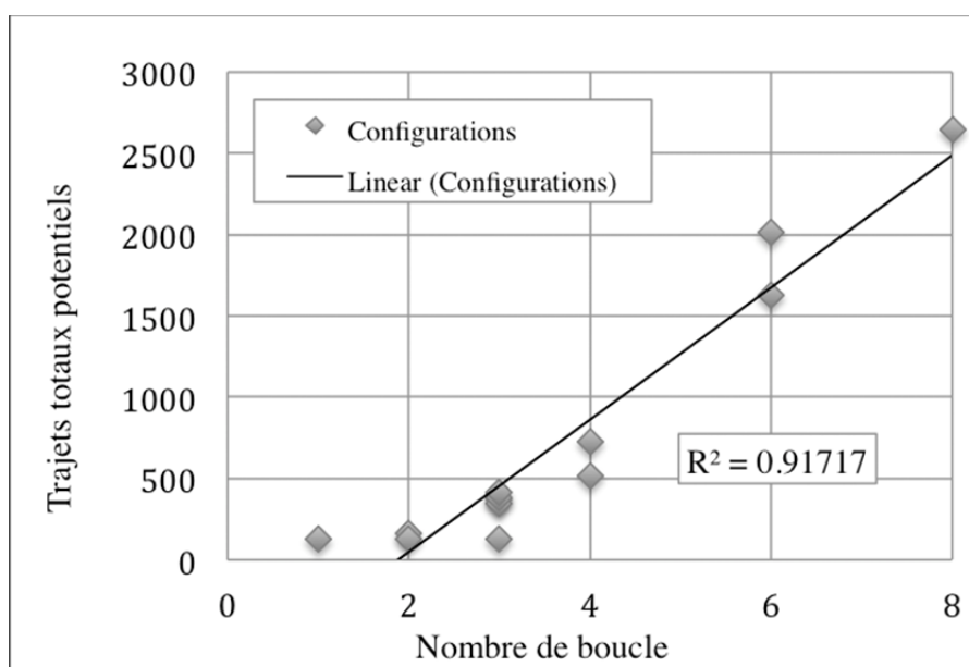
Figure 3.4 Trajet totaux potentiels selon le nombre de boucle pour toutes les configurations excluant l'AMS.
