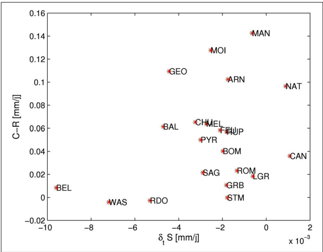
Figure-A I-5 Relation entre l'erreur de fermeture (C-R) et de la variation du réservoir sol ( \delta_t S ) en mm/j pour les 21 bassins versants du Québec
