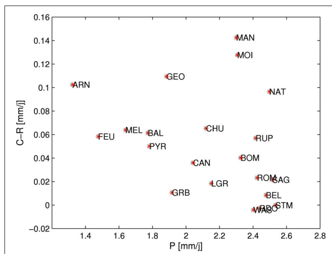
Figure-A I-2 Relation entre l'erreur de fermeture (C-R) et des précipitations (P) en mm/j pour les 21 bassins versants du Québec
