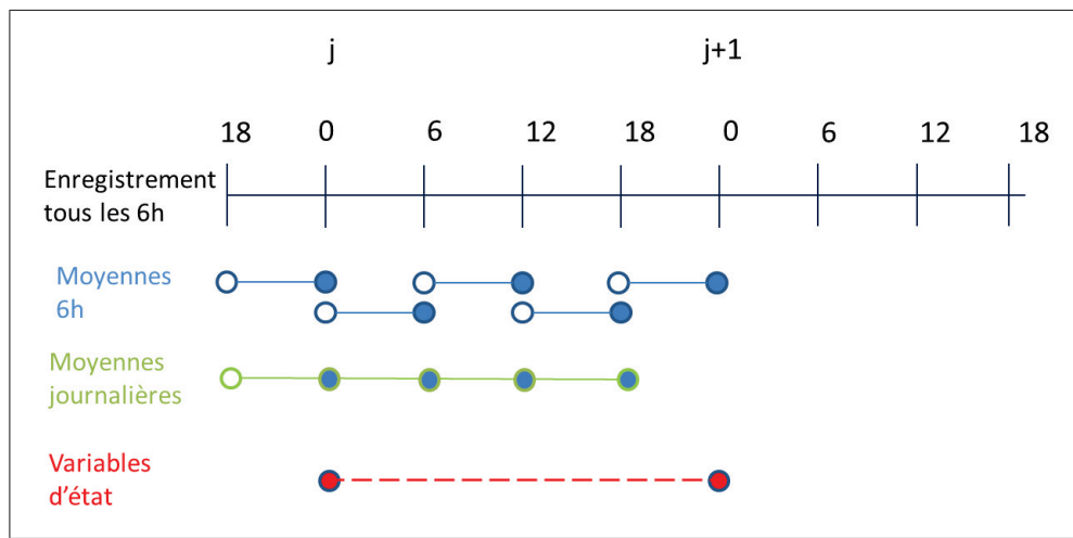
Figure 4.4 Représentation du schéma numérique et d'enregistrement du MRCC
