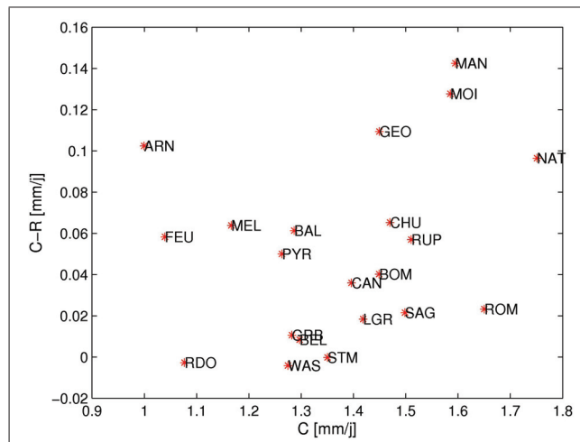
Figure-A I-1 Relation entre l'erreur de fermeture (C-R) et la convergence (C) en mm/j pour les 21 bassins versants du Québec.
