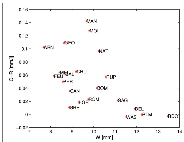
Figure-A I-4 Relation entre l'erreur de fermeture (C-R) et du contenu en eau du réservoir atmosphérique (W) en mm/j pour les 21 bassins versants du Québec
