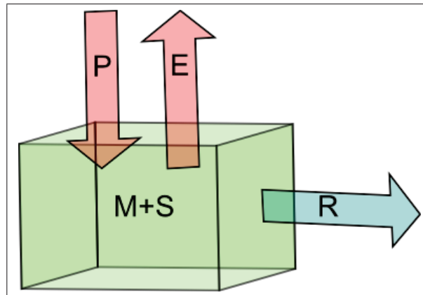
Figure 1.2 Schéma du bilan hydrologique sur une colonne terrestre
