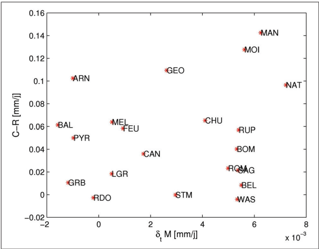
Figure-A I-6 Relation entre l'erreur de fermeture (C-R) et de la variation du couvert de neige ( \delta_t M ) en mm/j pour les 21 bassins versants du Québec
