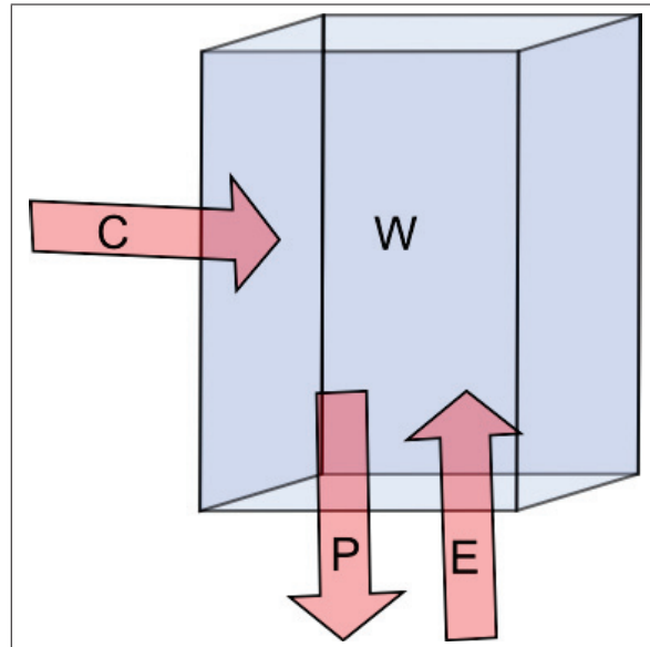
Figure 1.4 Schéma du bilan hydrologique sur une colonne atmosphérique
