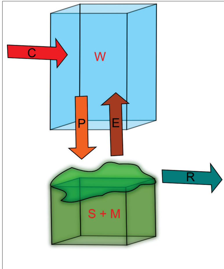
Figure 1.5 Schéma du bilan hydrologique sur une colonne terre-atmosphère
