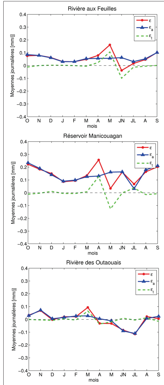
Figure 3.6 Cycle annuel moyen des erreurs totale ( \epsilon ), atmosphérique ( \epsilon_a ) et terrestre ( \epsilon_t )
