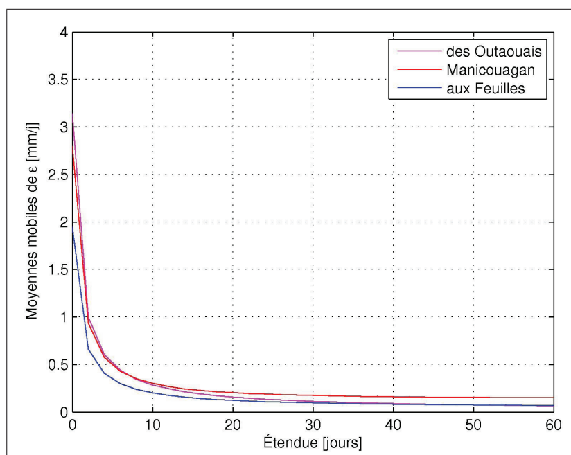
Figure 3.15 Moyenne de l'erreur dans le bilan hydrique en fonction de l'étendue des moyennes mobiles 1961-2000
