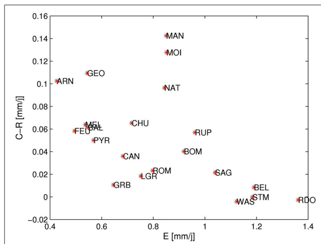
Figure-A I-3 Relation entre l'erreur de fermeture (C-R) et de l'évaporation (E) en mm/j pour les 21 bassins versants du Québec
