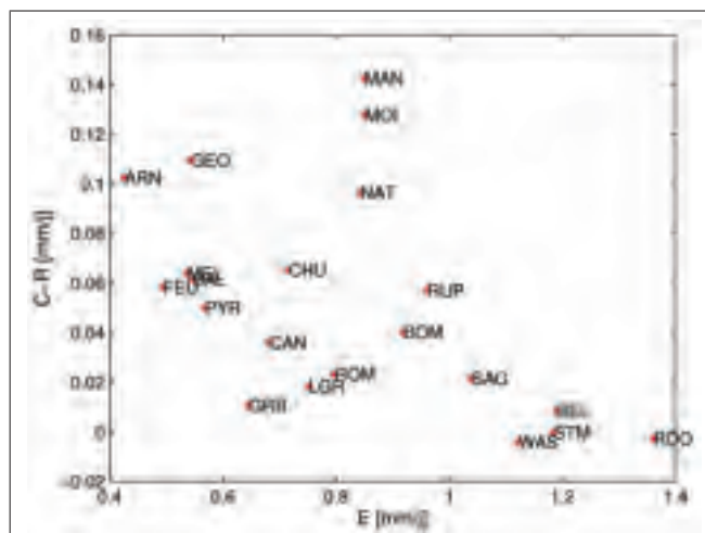
Figure-A I-3 Relation entre l'erreur de fermeture (C-R) et de l'évaporation (E) en mm/j pour les 21 bassins versants du Québec
