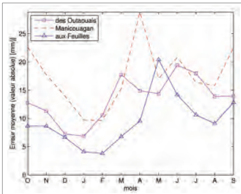
Figure 3.13 Cycle annuel de l'erreur en valeur absolue
