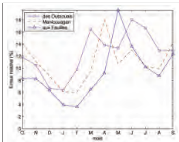
Figure 4.3 Erreur relative à l'échelle mensuelle cycle annuel moyen 1961-2000
