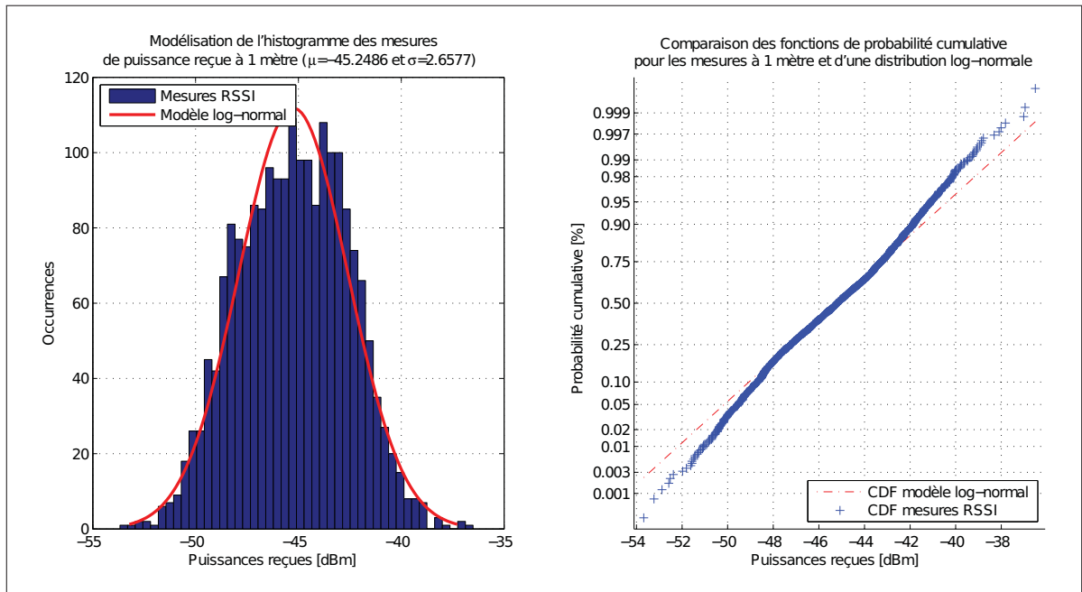
Figure 4.7 Modélisation de l'historgramme des moyennes linéaires de puissances reçues par une loi log-normale à 1 mètre (droite) et une comparaison visuelle entre la fonction de probabilité cumulative du modèle log-normal et celle des données (gauche).
