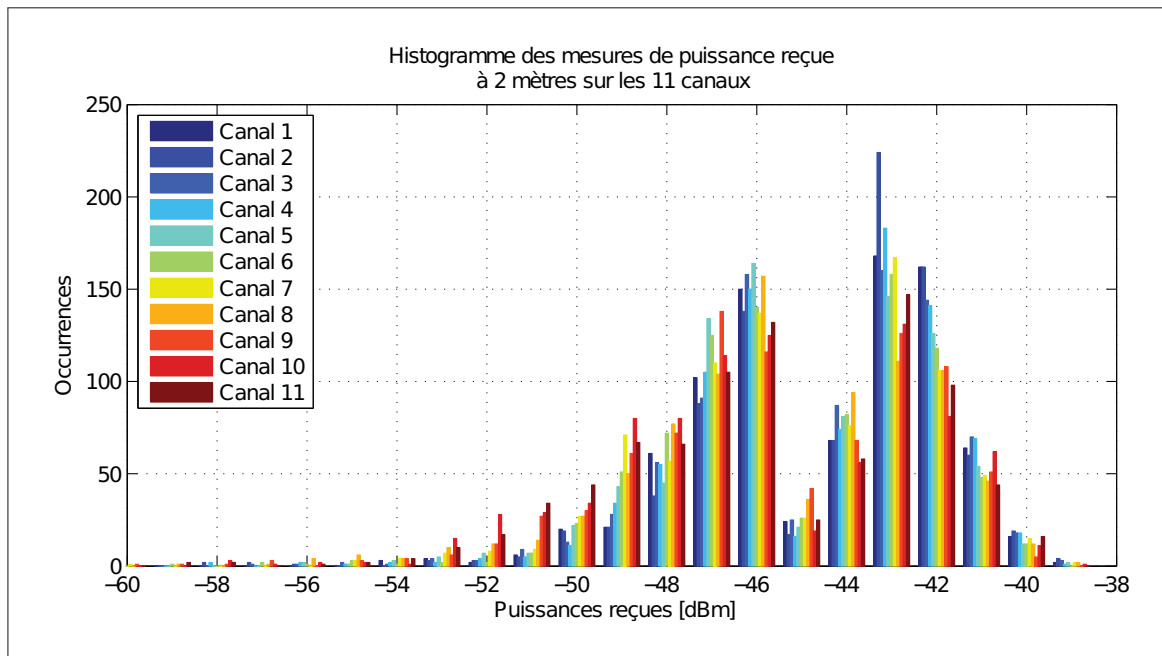
Figure 4.5 Histogramme des mesures de puissance reçue à 2 m dans les 11 canaux du tableau 3.1 avec un incrément de 1 dBm par colonne.
