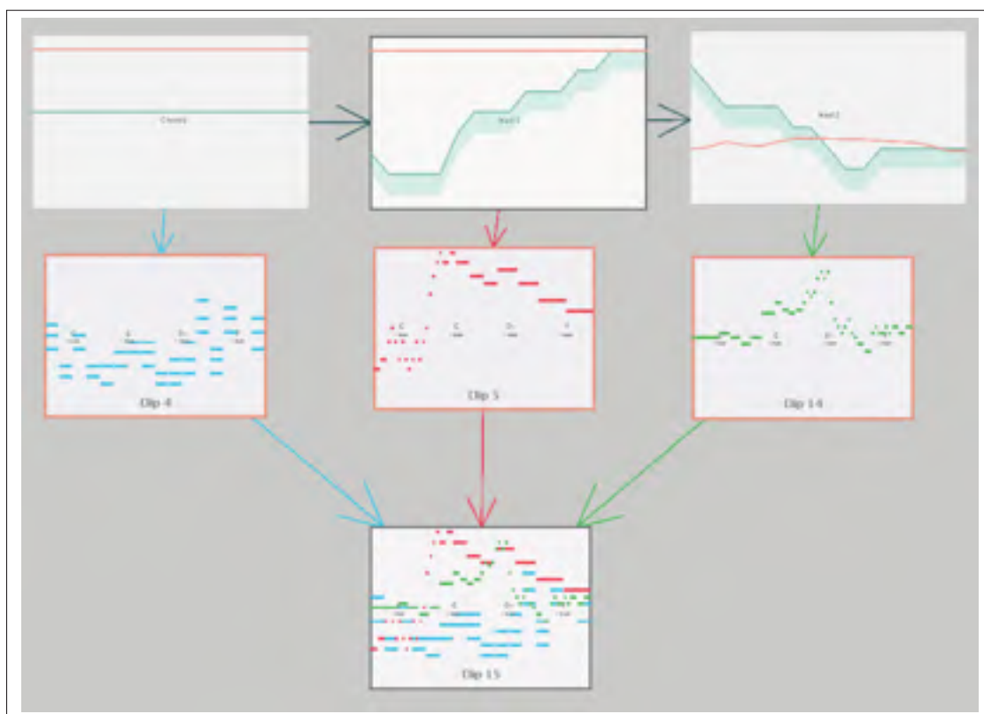
Figure 3.8 Exemple de fusion des voix Imprime-écran de GenSession
