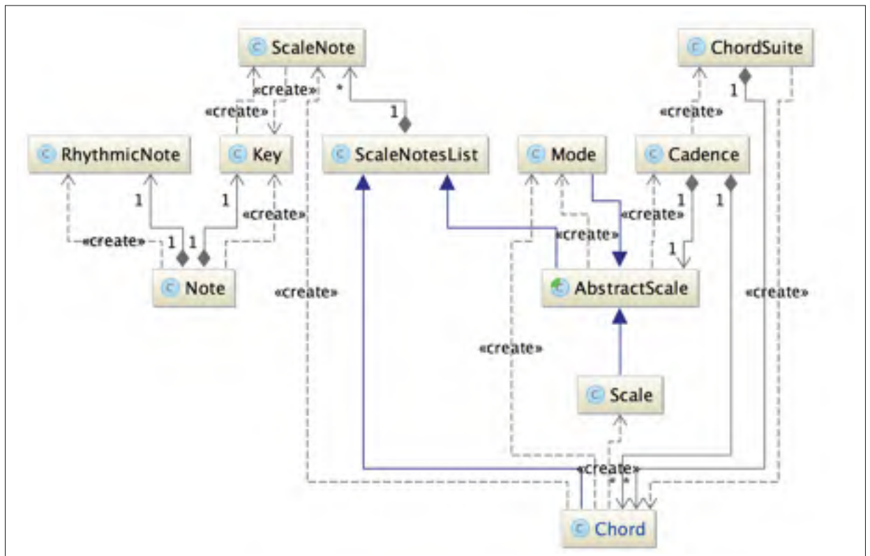
Figure 3.17 Diagramme de classe représentant l'architecture du module de théorie musicale du prototype
