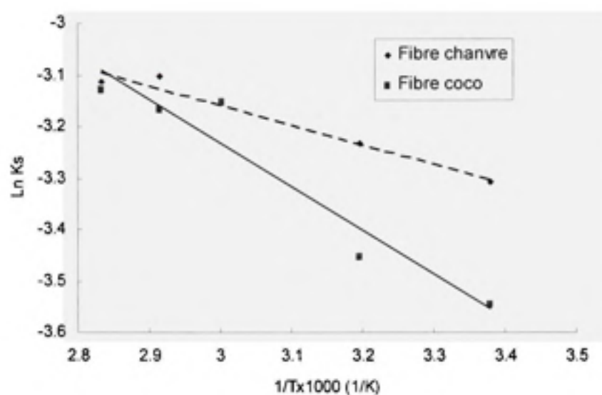
Figure 52 Graphique de \ln K_s versus l'inverse de la température
