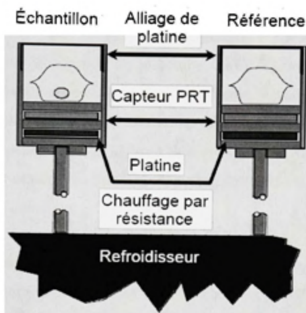
Figure 23 Schéma de fonctionnement du calorimètre différentiel à balayage [111]
