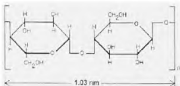
Figure 3 Formule chimique d'une unité répétitive constituant la cellulose
