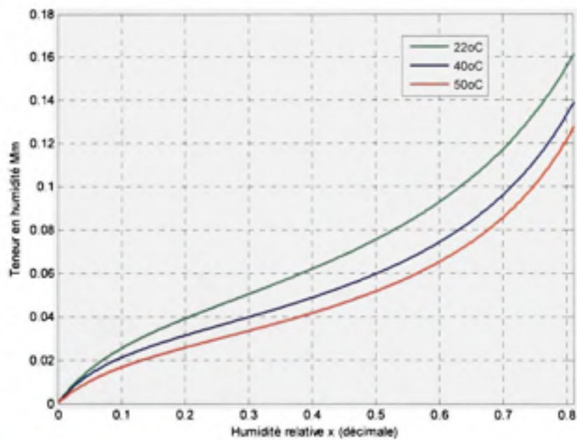
Figure 45 Isotherme de sorption d'humidité aux différentes températures des fibres de coco selon le modèle de GAB
