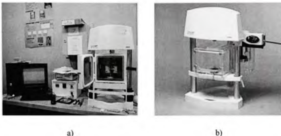
Figure 26 Machine à traction : a) avec la chambre thermique, b) avec bain de saline
