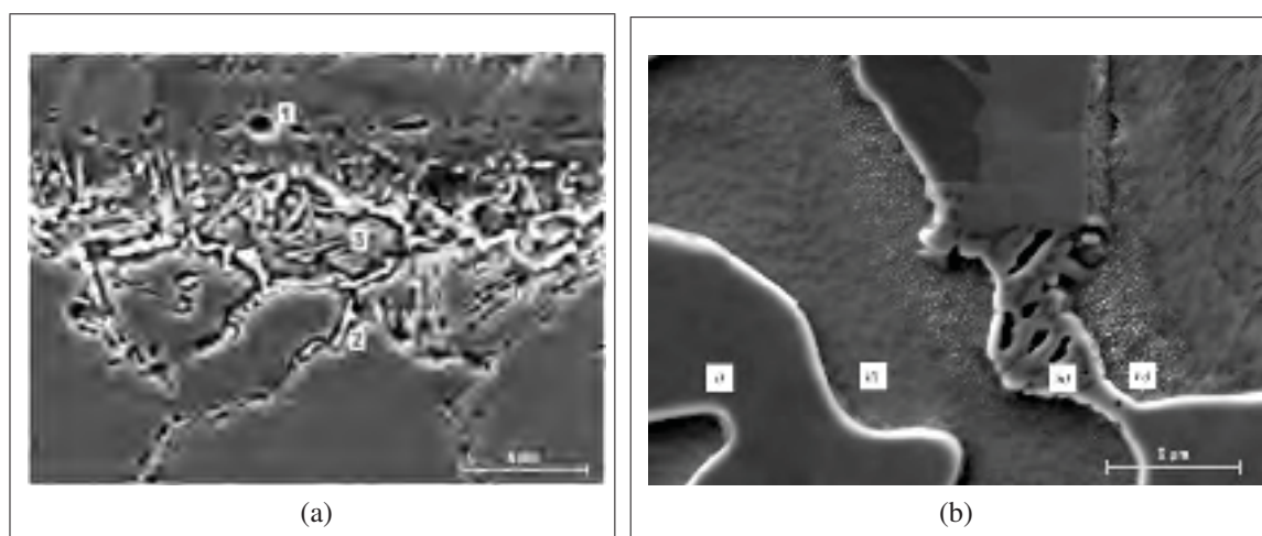
Figure 5.8 a) Détail de la zone BDPL et la couche X sur l'échantillon plaqué 42 \mu\text{m} . b) Détail de la zone CBL et les fin précipités de Si sur l'échantillon plaqué 19 \mu\text{m} .
