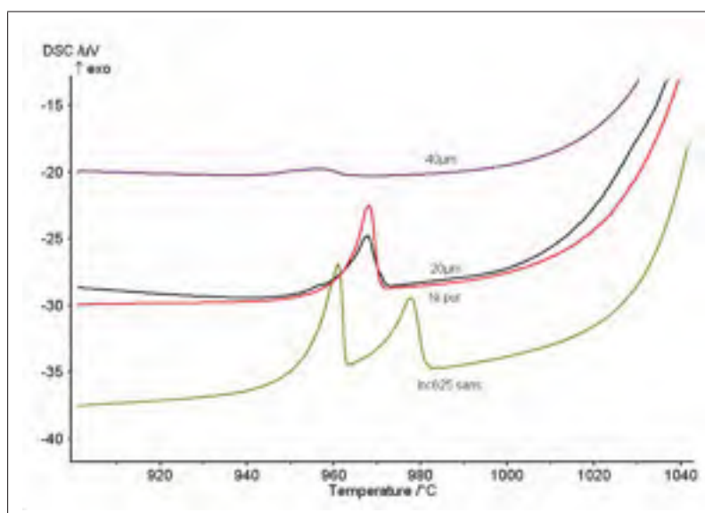
Figure 5.3 Pics DTA au refroidissement des échantillons brasés de IN625, IN625 plaqué 19 \mu\text{m} , IN625 plaqué 42 \mu\text{m} et Ni pur avec du BNi-2 (chauffage et refroidissement à 25 K/min, température maximale 1050 °C ).
