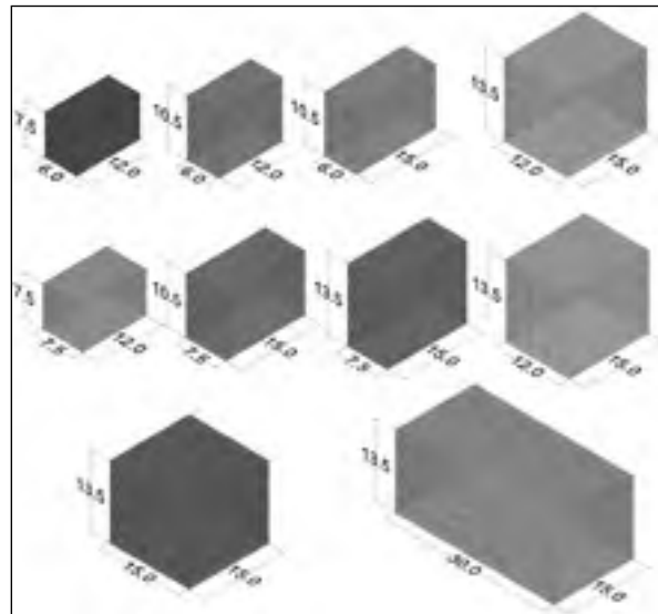
Figure 2.5 Bâtiments types du modèle Tirée de Beckers (2012)
