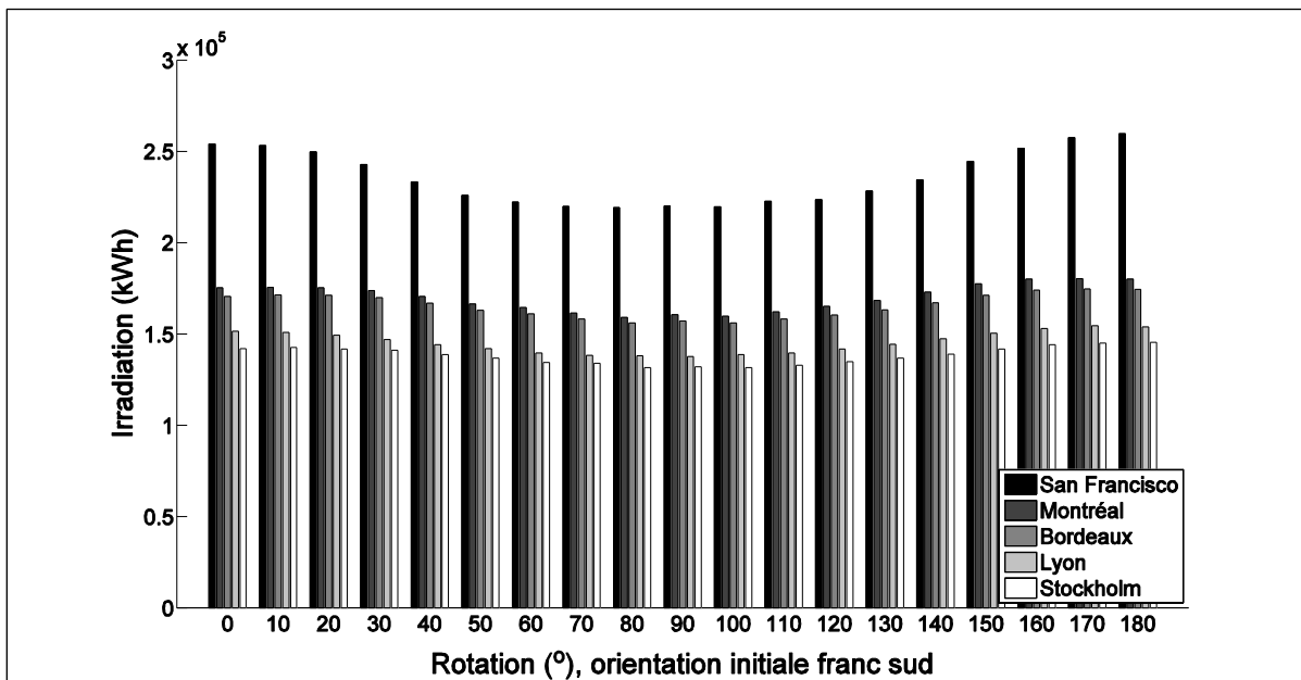
Figure 3.4 Irradiation totale sur la surface vitrée du quartier d'étalement, un étage supplémentaire, pour des fenêtres de 1 m 2 par rapport son orientation, selon la ville à l'étude et leur période de chauffe respective
