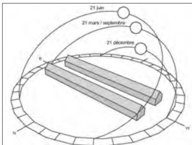
Figure 1.13 Uniformité du canyon urbain selon l'étude de van Esch Adaptée de van Esch, Looman et Bruin Hordjik (2012)
