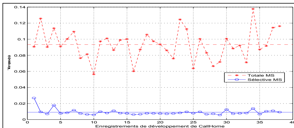
Figure 8.6 Comparaison du temps d'exécution (en secondes) des deux stratégies, totale (STR) et sélective (SSR), de l'algorithme de Mean Shift.
