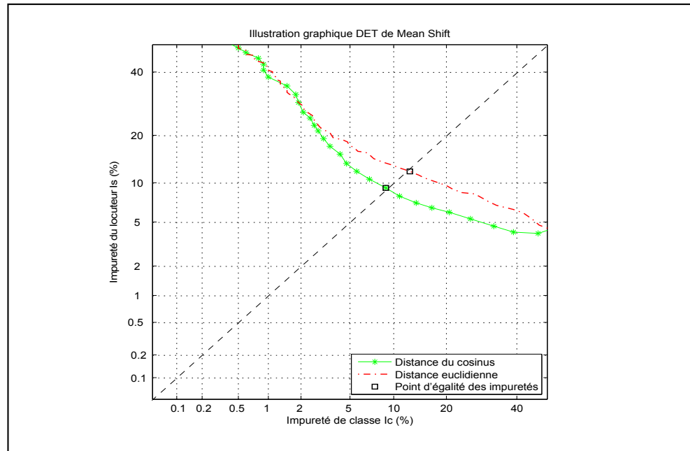
Figure 7.1 Illustration graphique DET des performances de l'algorithme de Mean Shift à base de la distance euclidienne et de celui à base de la distance angulaire du cosinus testés sur la tâche du regroupement en locuteurs de l'ensemble des données SRE 2008 de NIST.
