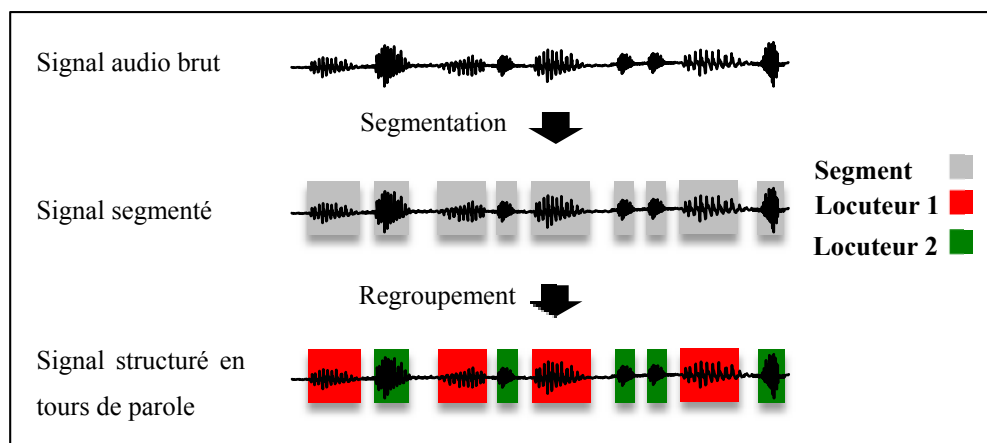
Figure 1.6 Structuration en locuteurs d'un flux audio contenant deux locuteurs.
