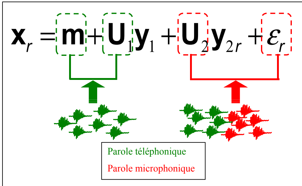
Figure 4.4 Procédure d'entraînement des paramètres du modèle PLDA destiné à la réduction de la dimensionnalité.
