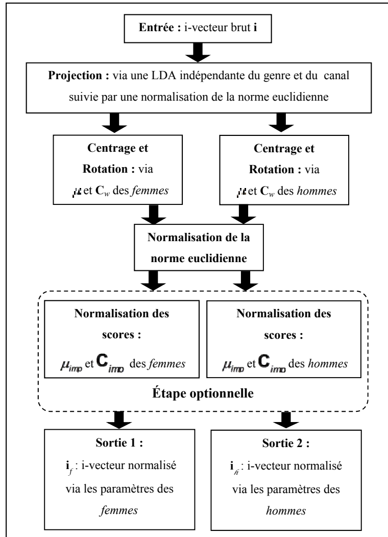
Figure 5.2 Représentation graphique du processus de la normalisation indépendante du genre d'un i-vecteur \mathbf{i} dans le cadre d'un classificateur à base de la similarité angulaire du cosinus.
