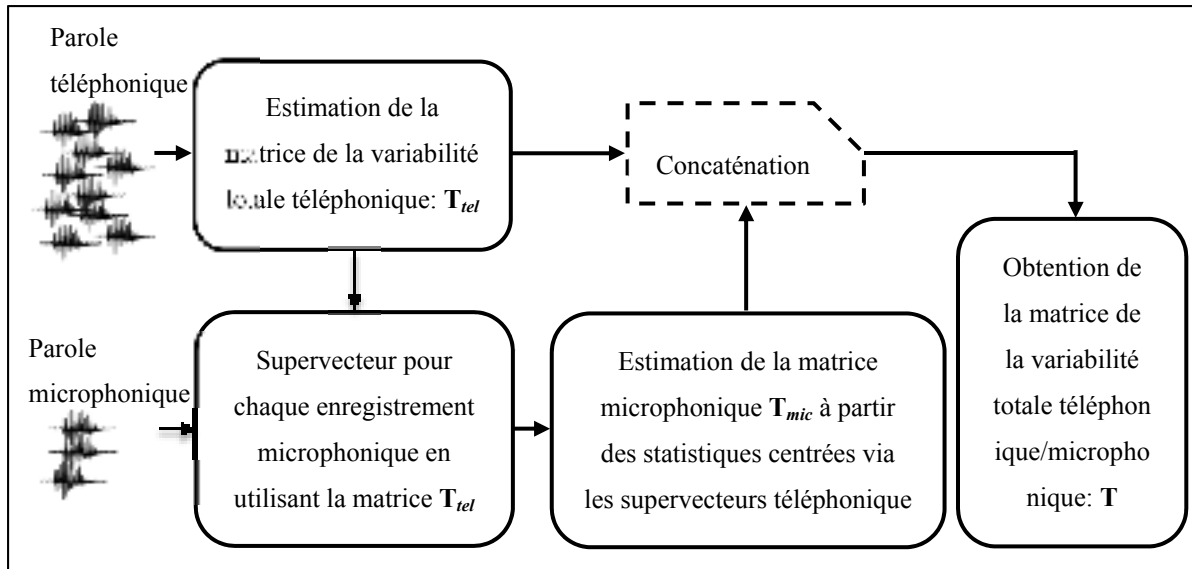
Figure 4.2 La procédure d'estimation par concaténation de la matrice de la variabilité totale indépendante du canal (téléphonique/microphonique).
