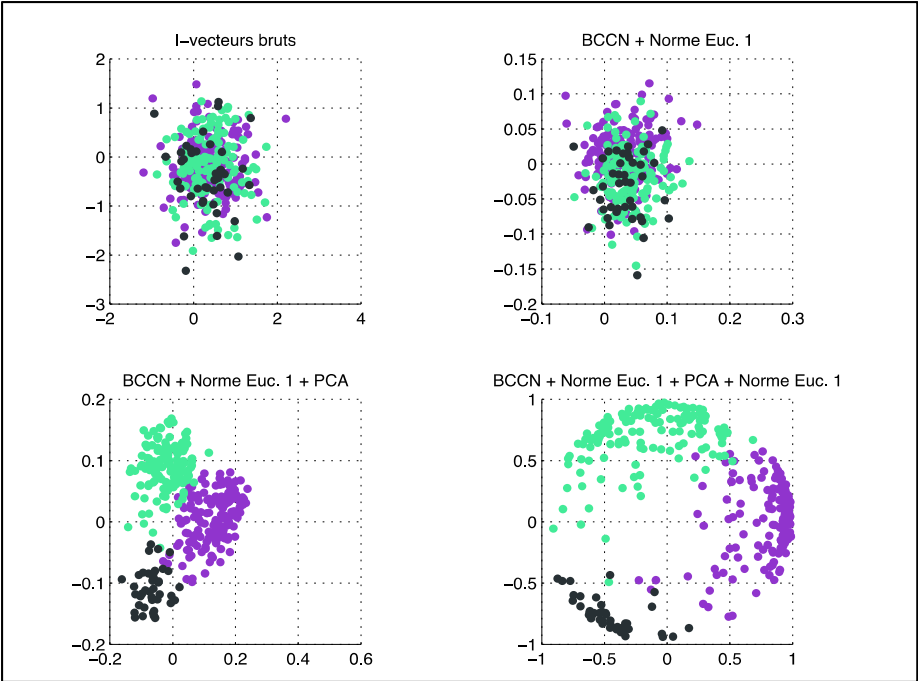
Figure II.2 Effets de la normalisation des i-vecteurs de la conversation iabi
