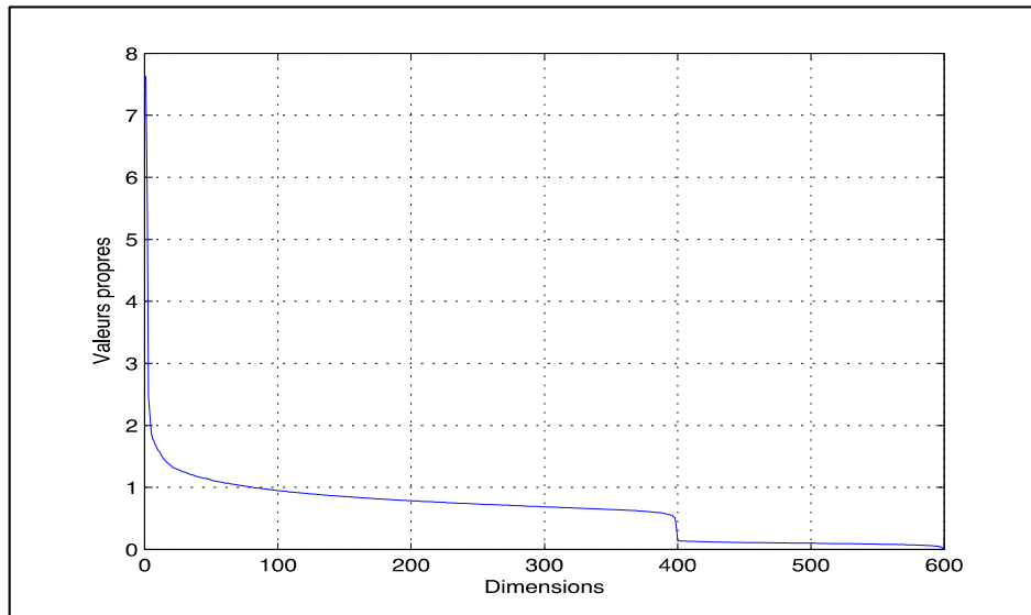
Figure 4.3 Graphe des valeurs propres de la matrice de covariance des i-vecteurs (obtenus par la concaténation des matrices de la variabilité totale) des données d’entraînement de NIST.
