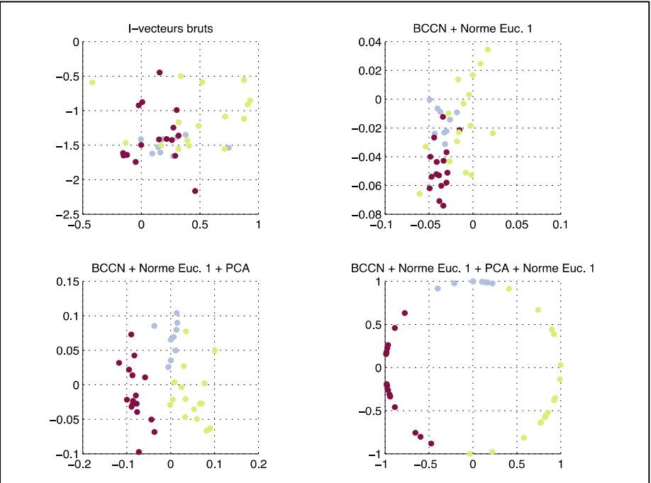
Figure II.3 Effets de la normalisation des i-vecteurs de la conversation iaab
