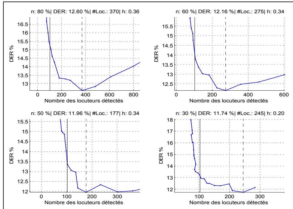
Figure 8.3 Résultats (DER/nombre des locuteurs estimés) de la stratégie totale de regroupement (STR) obtenus à partir de l'ensemble de développement en utilisant la normalisation des i-vecteurs via la PCA. Le minimum de DER, sa bande passante fixe correspondante ( h ) ainsi que son nombre de locuteurs estimés correspondant ( \#Loc. ) sont également fournis pour chaque facteur \eta = 80, 60, 50 et 30 de la PCA.
