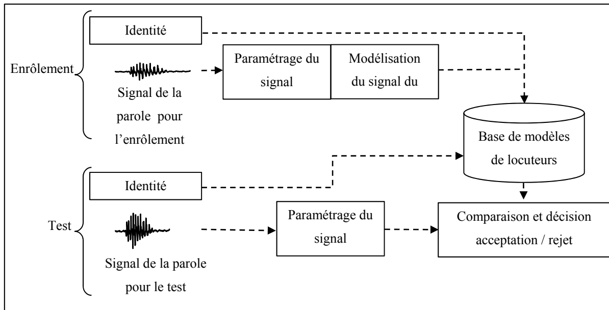
Figure 1.2 Schéma typique d'un système de vérification du locuteur : phase d'enrôlement et phase de test.
