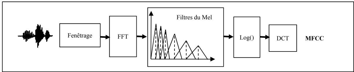
Figure 2.1 Procédure d'extraction des vecteurs caractéristiques à court terme MFCC.
