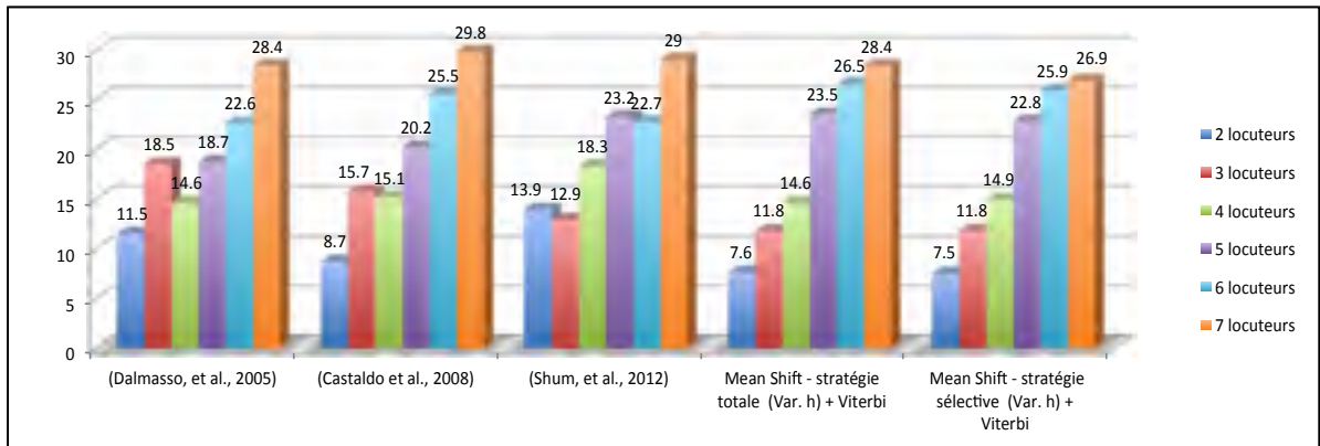
Figure 8.5 Comparaison des résultats (DER % en ordonnée) des deux versions, totale (STR) et sélective (SSR), de l’algorithme de Mean Shift avec les résultats de l’état de l’art obtenus à partir des mêmes données du test du corpus CallHome.
