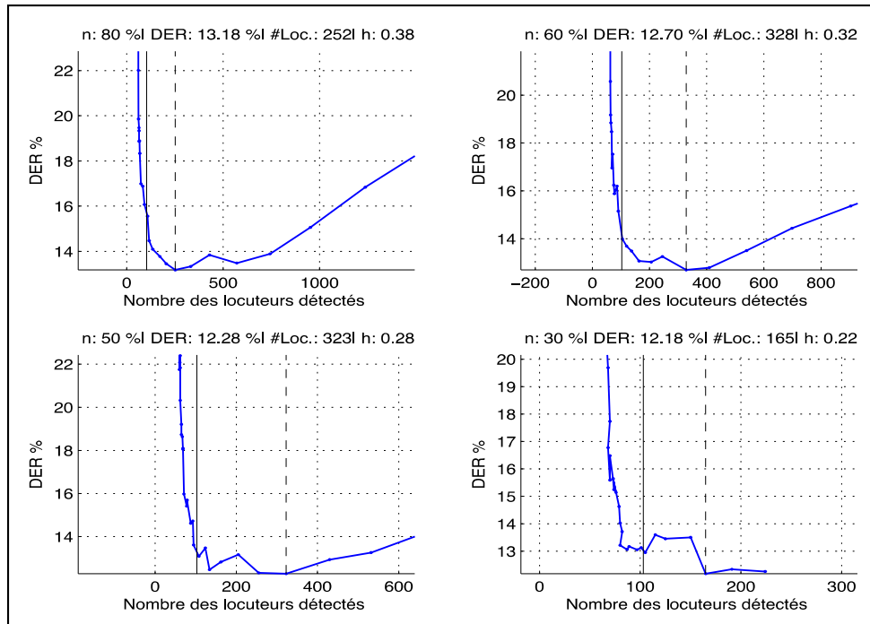
Figure 8.4 Résultats (DER/nombre des locuteurs estimés) de la stratégie sélective de regroupement (SSR) obtenus à partir de l'ensemble de développement en utilisant la normalisation des i-vecteurs via la PCA. Le minimum de DER, sa bande passante fixe correspondante ( h ) ainsi que son nombre de locuteurs estimés correspondant ( \#Loc. ) sont également fournis pour chaque facteur \eta = 80, 60, 50 et 30 de la PCA.
