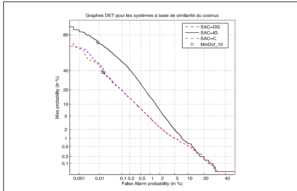
Figure 5.3 Courbes DET des systèmes à base de la SAC testés sur les listes téléphoniques de NIST (det5).
