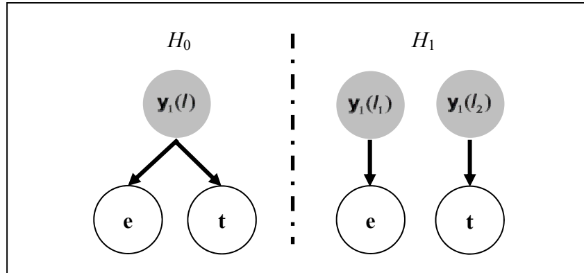
Figure 3.2 Graphe décrivant, dans le cadre du modèle PLDA, les deux hypothèses ( H_0 , H_1 ) utilisées pour calculer le score de vérification en présence d'un i-vecteur d'enrôlement e et d'un autre i-vecteur pour le test t .
