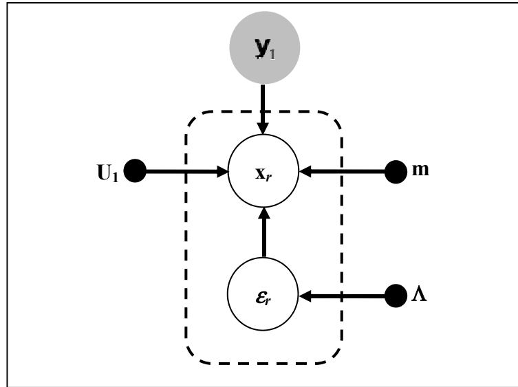
Figure 3.1 Graphe probabiliste du modèle PLDA donné par l'équation (3.3). Les points noirs représentent les paramètres du modèle, le cercle plein (arrière-plan gris) représente le vecteur caché, les deux cercles vides représentent respectivement un i-vecteur et un vecteur de bruit résiduel et enfin le cadre discontinu représente la répétition de la partie encadrée R fois.
