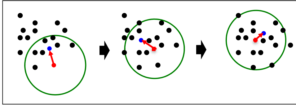
Figure 6.1 Évolution du processus de recherche du mode d'une distribution de probabilité via l'algorithme de Décalage de la moyenne . Le cercle vert représente le noyau centré sur le point d'intérêt (point rouge), la flèche rouge représente le vecteur de Mean Shift et finalement le point bleu représente la moyenne des points qui se trouvent dans le cercle de noyau.
