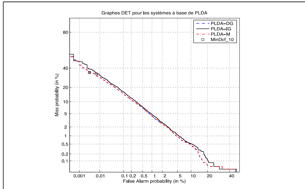
Figure 5.1 Courbes DET des systèmes à base de PLDA testés sur les listes téléphoniques de NIST (det5).
