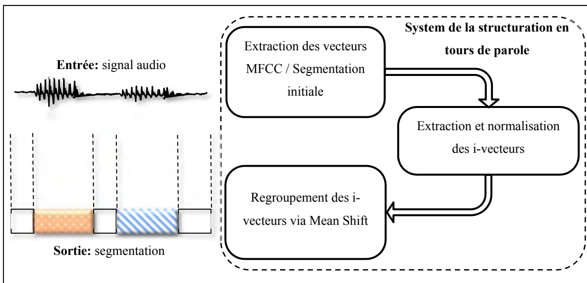
Figure 8.1 Illustration graphique de la structure générale d'un système de segmentation en tours de parole à base de la représentation en i-vecteurs et de regroupement via l'algorithme de Mean Shift.
