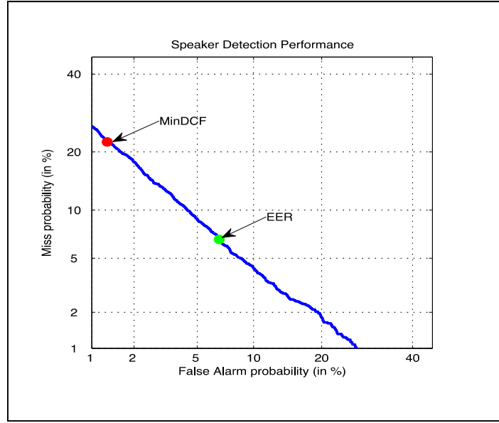
Figure 1.4 Illustration graphique DET de NIST sur laquelle l'ERR et le minimum DCF sont respectivement représentés par le point vert et le point rouge.
