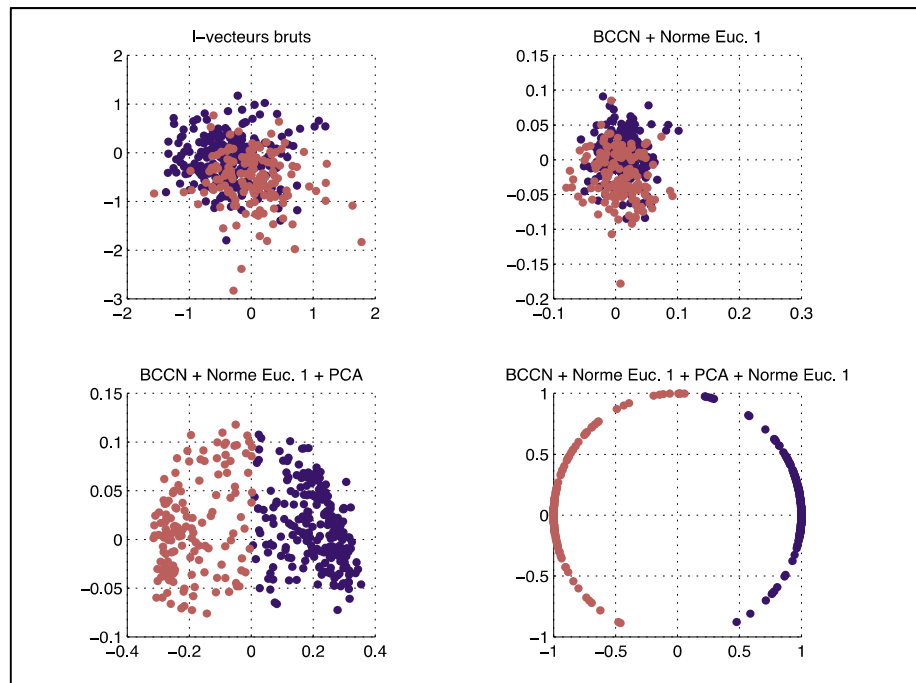
Figure II.1 Effets de la normalisation des i-vecteurs de la conversation iahb
