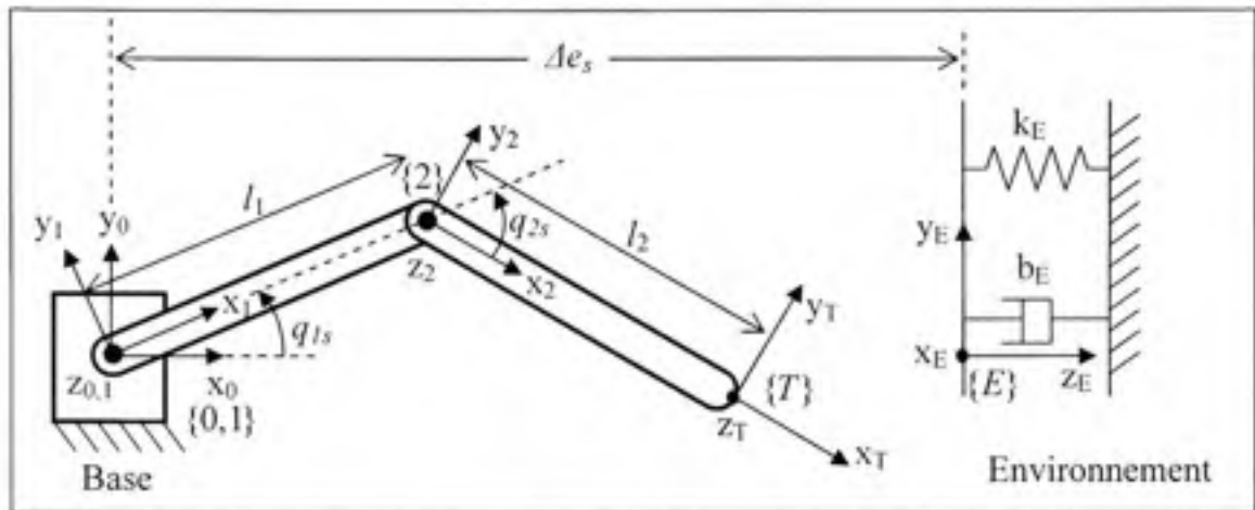
Figure 2.2 Schéma du robot virtuel.
