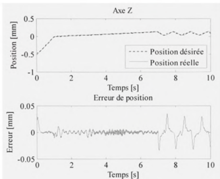
Figure 5.18 Position du robot réel (axe Z) de la simulation sans application de la contrainte (PID).
