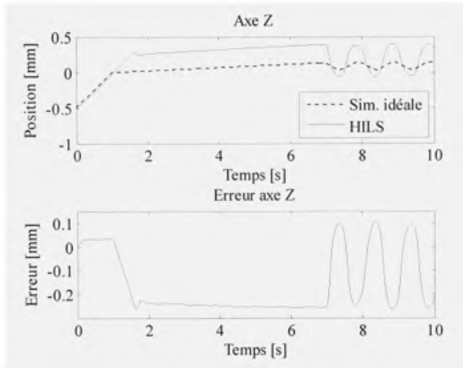
Figure 5.16 Position du robot virtuel (axe Z) de la simulation sans application de la contrainte (PD).
