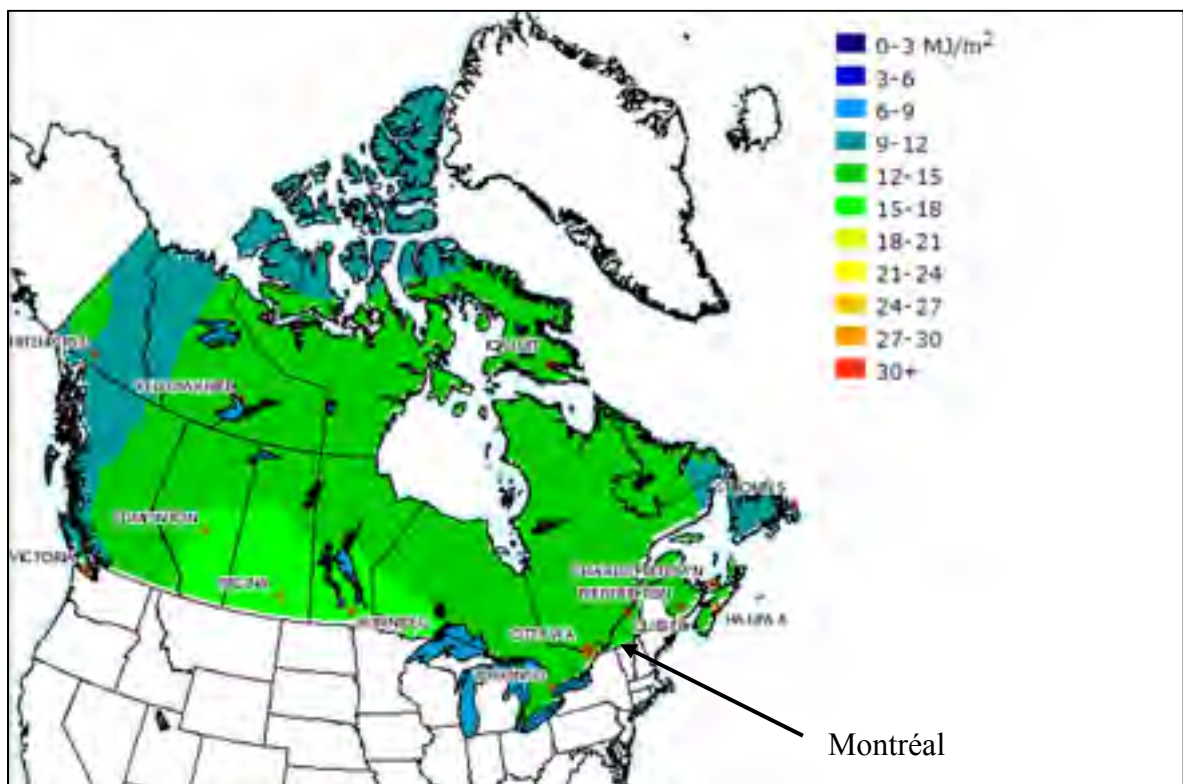
Figure 2.3 Ensoleillement global quotidien moyen sur une base annuelle (MJ/m 2 ) pour une surface orientée vers le sud avec inclinaison = latitude + 15° Canada, 2013c
