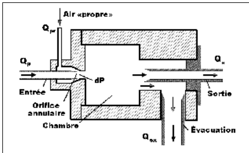
Figure 1.18 Croquis d'un diluteur à injection PALAS Adaptée de www.palas.com consultée le 28/02/2014
