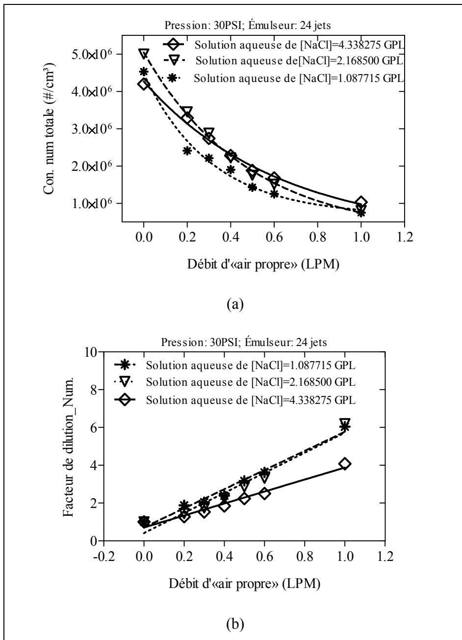
Figure 2.17 Graphiques à différentes concentrations de solutions aqueuses de NaCl : (a) concentration des aérosols NaCl, (b) facteur de dilution
