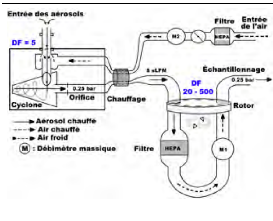
Figure 1.23 Diluteur à rotor CAMBUSTION-DMS 500 Tirée de www.cambustion.com consulté le 28/02/2014
