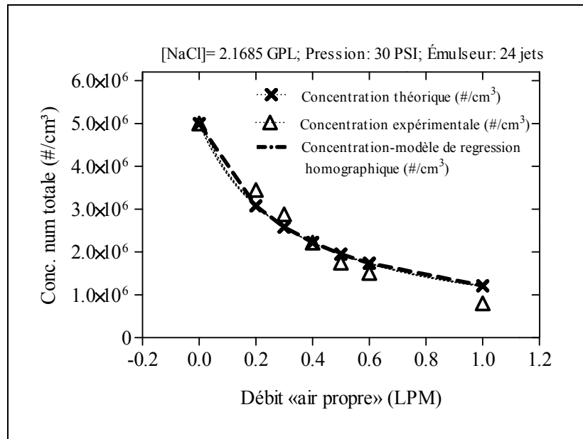
Figure 2.12 Graphiques de la concentration expérimentale et du modèle de régression homographique
