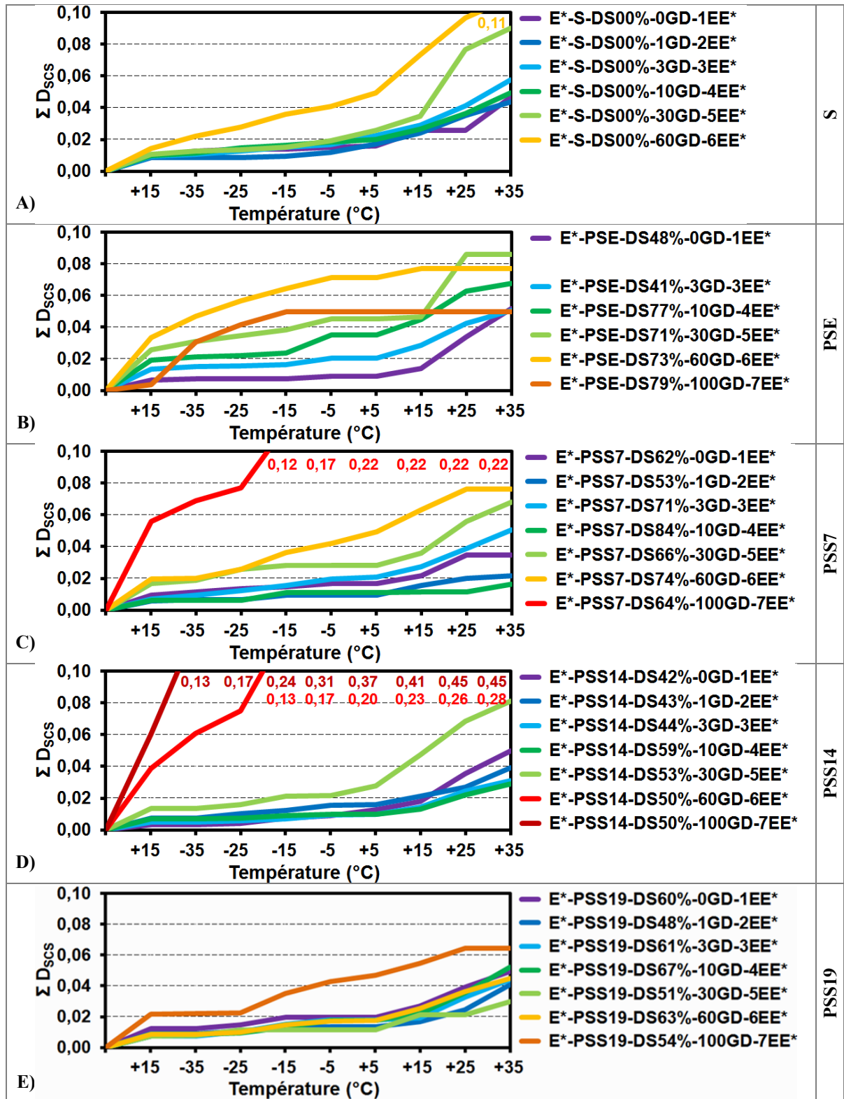
Figure 4.53 Dommage cumulatif g n r  par les s quences de cyclage de sollicitation ( \Sigma D_{scs} ) lors d'un essai de module complexe ( EE^* )
