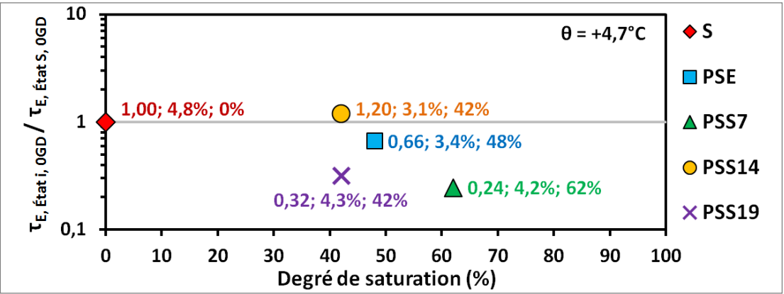
Figure 4.40 Valeurs de tau des enrobés à une température de +4,7^\circ\text{C} , aux états étudiés et à 0 GD, en fonction du DS et normalisées en référence à celle de l'enrobé à l'état S (valeurs du rapport, teneur en vides et degré de saturation indiquées)
