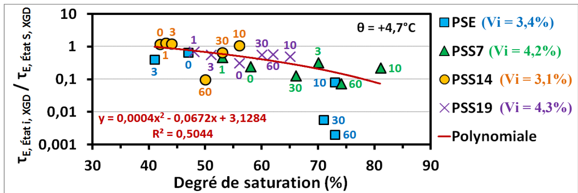
Figure 4.43 Normalisation de la valeur de \tau de l'enrobé à une température de +4,7^\circ\text{C} , à l'état i et à X GD par rapport à celle obtenue pour l'enrobé à cette même température à l'état sec ( S ) et à X GD (paramètres fixés, #CGD en étiquette)
