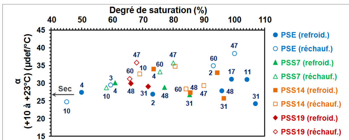
Figure 3.14 Coefficients de dilatation linéique ( \alpha ) des éprouvettes lors du refroidissement ( \downarrow T ) et lors du réchauffement ( \uparrow T ) entre +10 et +23^{\circ}\text{C} en fonction du degré de saturation (le numéro du cycle de GD près de cette plage de température est mis en étiquette)
