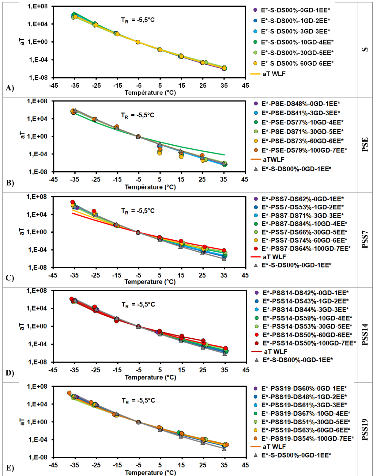
Figure 4.30 Évolution d' a_T avec la température pour les cinq états étudiés avec des paramètres fixés pour 2S2P1D et WLF (références : \theta de -5,5^{\circ}C et E^*-S-DS00\%-0GD-1EE^* )
