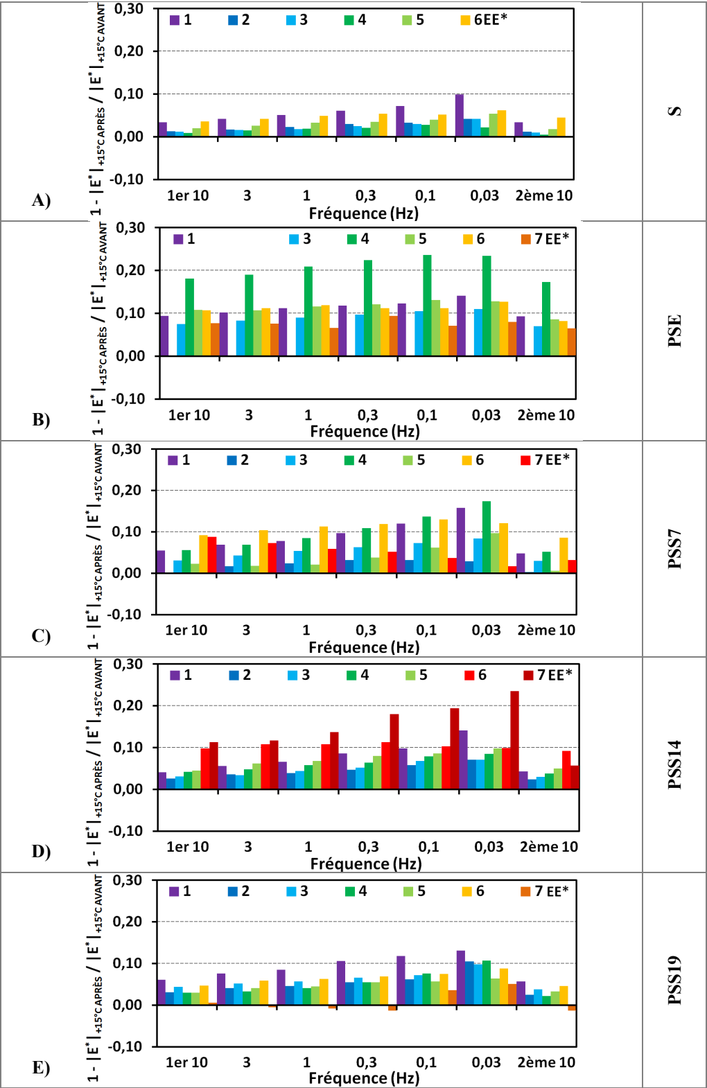
Figure 4.51 Évolution du dommage établi à partir de la comparaison des valeurs de |E^*| à +15^\circ\text{C} AVANT et +15^\circ\text{C} APRES en fonction de la fréquence
