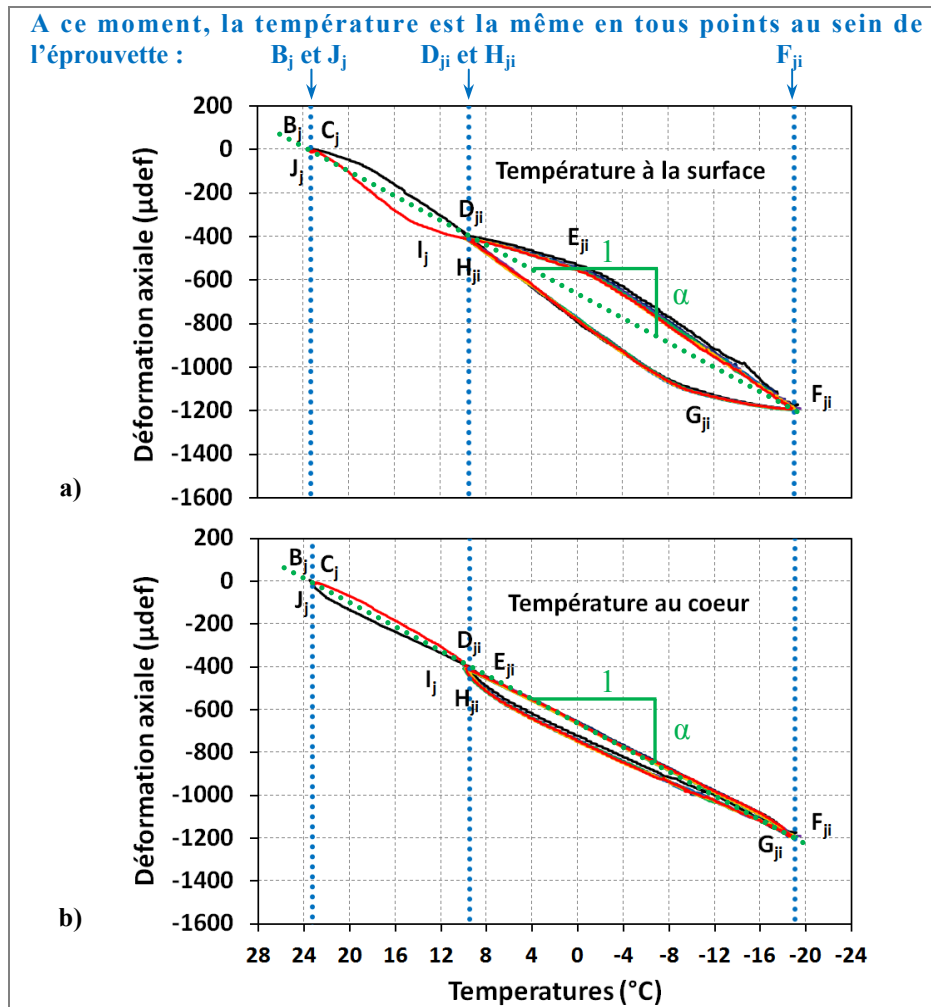
Figure 3.13 a) \epsilon_{\text{axiale}} vs T_{\text{surface}} , b) \epsilon_{\text{axiale}} vs T_{\text{cœur}} pour l'éprouvette PSS7 ( 58 \leq \text{DS} \leq 61\% ; B_j à J_j définis à la Figure 2.9 ; j = 3 ; 4 \leq i \leq 10 )
