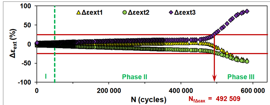
Figure 1.15 Écart de déformation et détermination de N_{f\Delta\epsilon ax}
