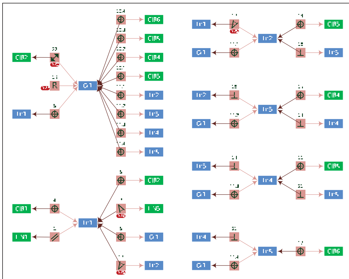
Figure A II-45 Cinquième cas de figure : Schémas originaux de contraintes relatives aux éléments de forme auxiliaires à transposer
