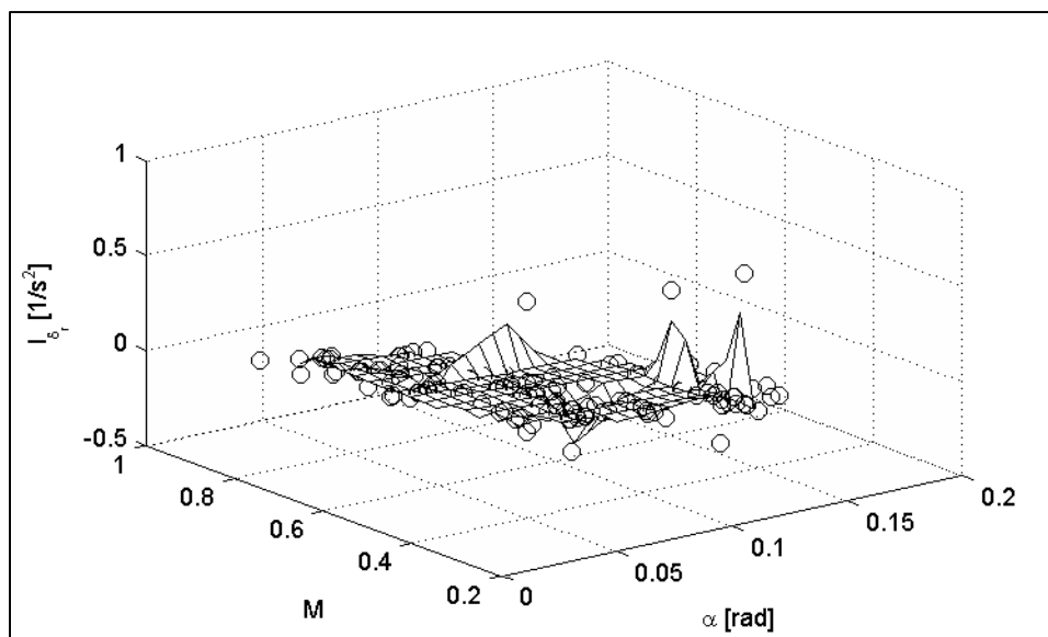
Figure-A IV-32 – Variation de l_{\delta_r} en fonction de \alpha et M
