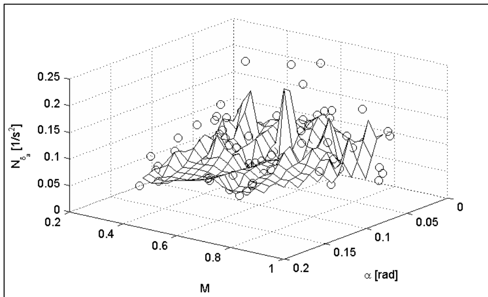
Figure-A V-23 – Variation de N_{\delta_a} en fonction de \alpha et M
