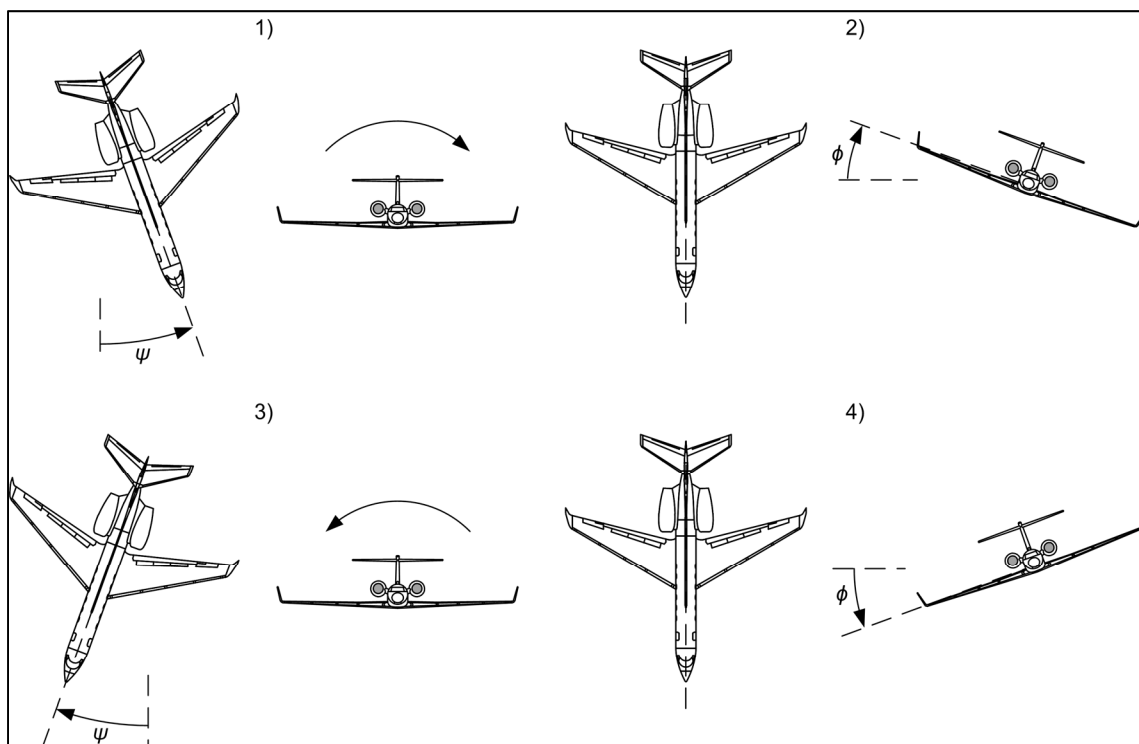
Figure 2.12 – Schéma de l'oscillation du mode du roulis hollandais
