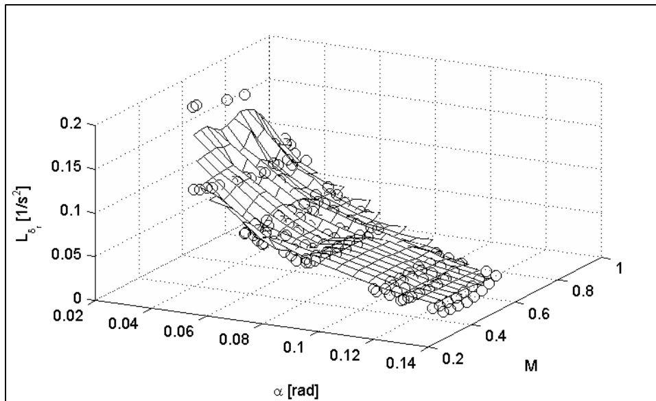
Figure-A V-22 – Variation de L_{\delta_t} en fonction de \alpha et M
