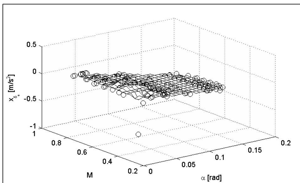
Figure-A IV-5 – Variation de x_{\delta_\theta} en fonction de \alpha et M
