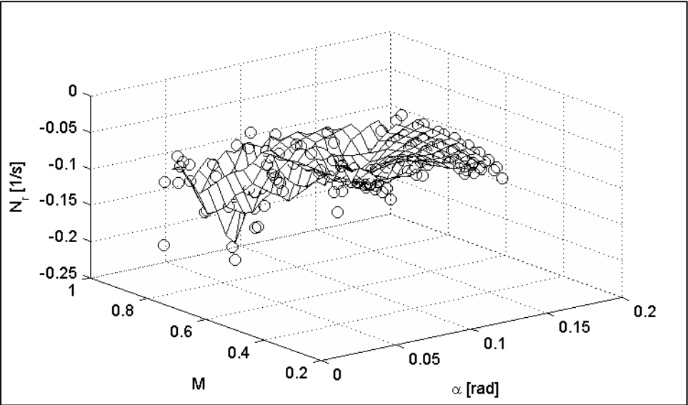
Figure-A V-19 – Variation de N_r en fonction de \alpha et M
