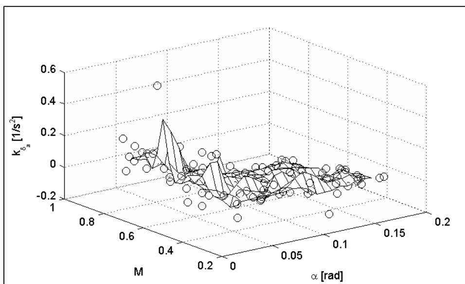
Figure-A IV-43 – Variation de k_{\delta_\alpha} en fonction de \alpha et M
