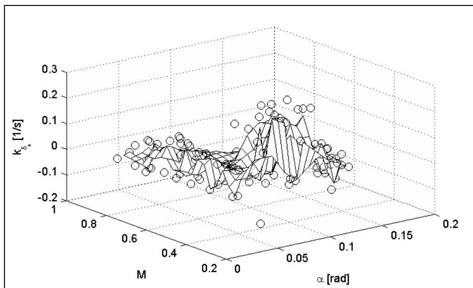
Figure-A IV-20 – Variation de k_{\delta_e} en fonction de \alpha et M
