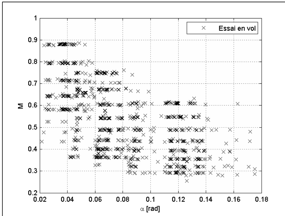
Figure 2.23 – Plan (\alpha, M) des essais en vol réalisés
