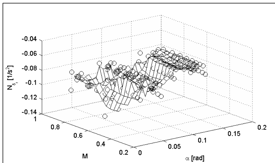
Figure-A V-24 – Variation de N_{\delta} , en fonction de \alpha et M
