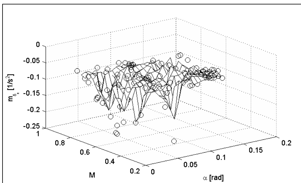
Figure-A IV-15 – Variation de m_{\delta_e} en fonction de \alpha et M
