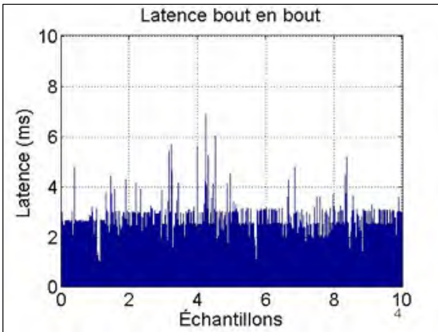
Figure 3.10 Test de latence avec intergiciel DDS par réception asynchrone
