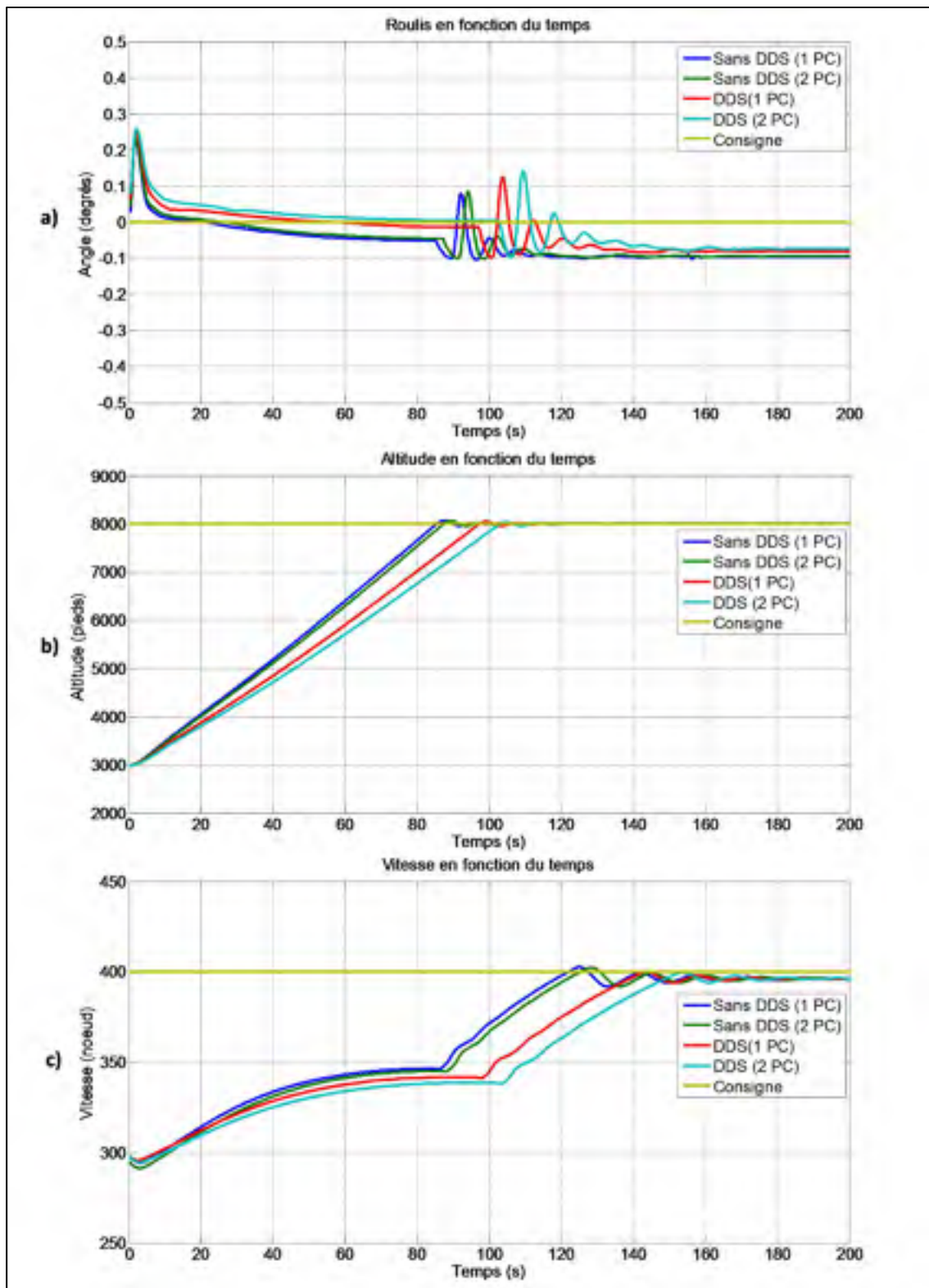
Figure 4.18 Résultats des scénarios de tests avec intergiciel DDS a) roulis, b) altitude, c) vitesse
