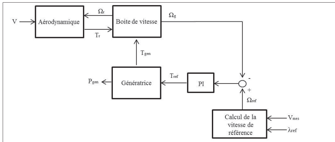
Figure 3.7 Schéma de la boucle de controle
