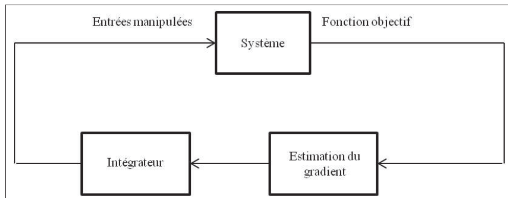
Figure 1.6 Principe de fonctionnement des méthodes de commande extrême
