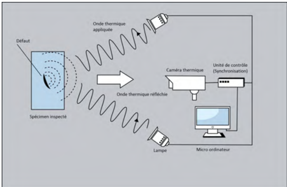
Figure 1-4 Montage expérimental pour la thermographie modulée
