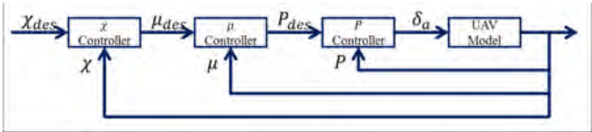
Figure 3.8 Schéma bloc Angle de cap
