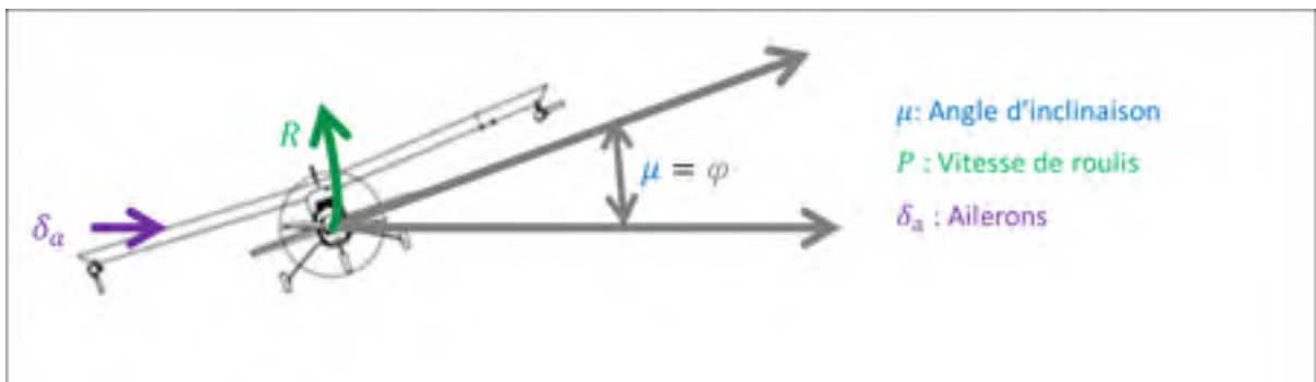
Figure 3.10 Angle d'inclinaison
