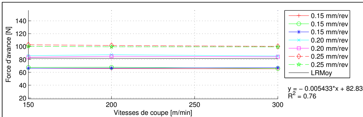
Figure 3.53 Effort d'avance moyen en fonction de la vitesse de coupe de l'OP50P6 -45° CR10 Y
