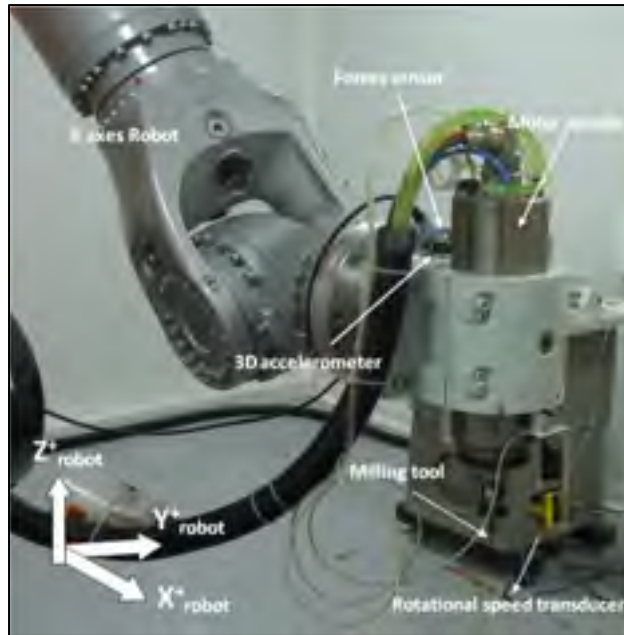
Figure 1.11 Montage expérimental Tirée de (Claudiu et al., 2012)
