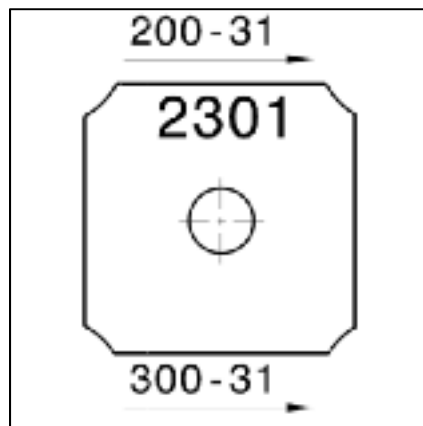
Figure 2.6 Identification des échantillons de CFRP détouré et de leurs conditions de coupe
