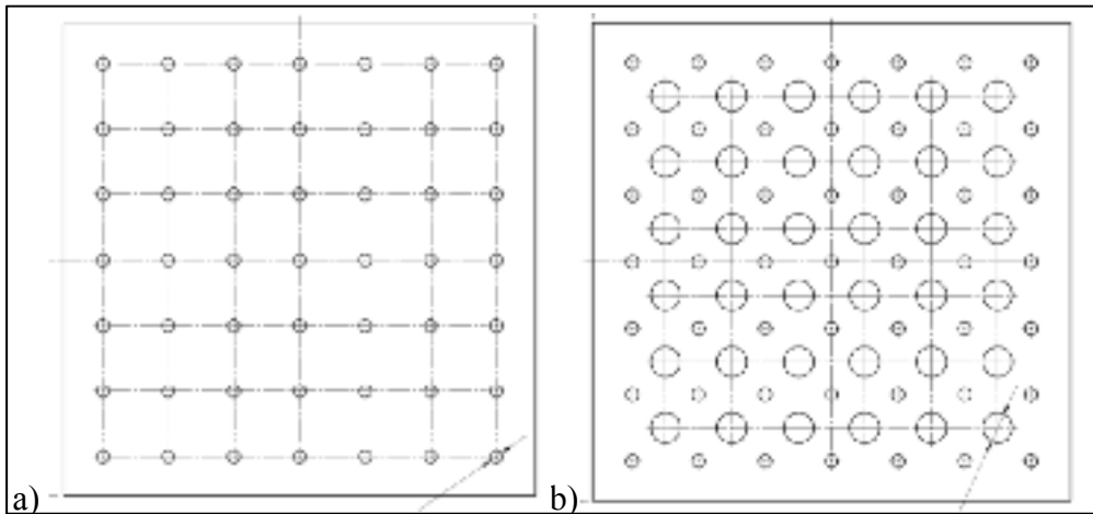
Figure 2.9 Schéma de la plaque CFRP percée, a) 49 trous de fixation pour des vis ¼-20UNC, b) 36 trous de dégagement d'un diamètre de ¾ de pouce
