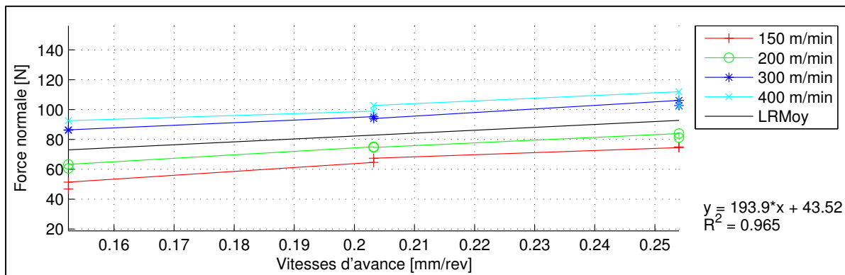
Figure 3.30 Effort normal moyen en fonction de la vitesse d'avance de l'OP30P3 45° CR20 X
