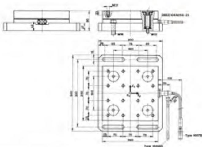
Fig. 1: Dimensions de dynamomètre de type 9255B
