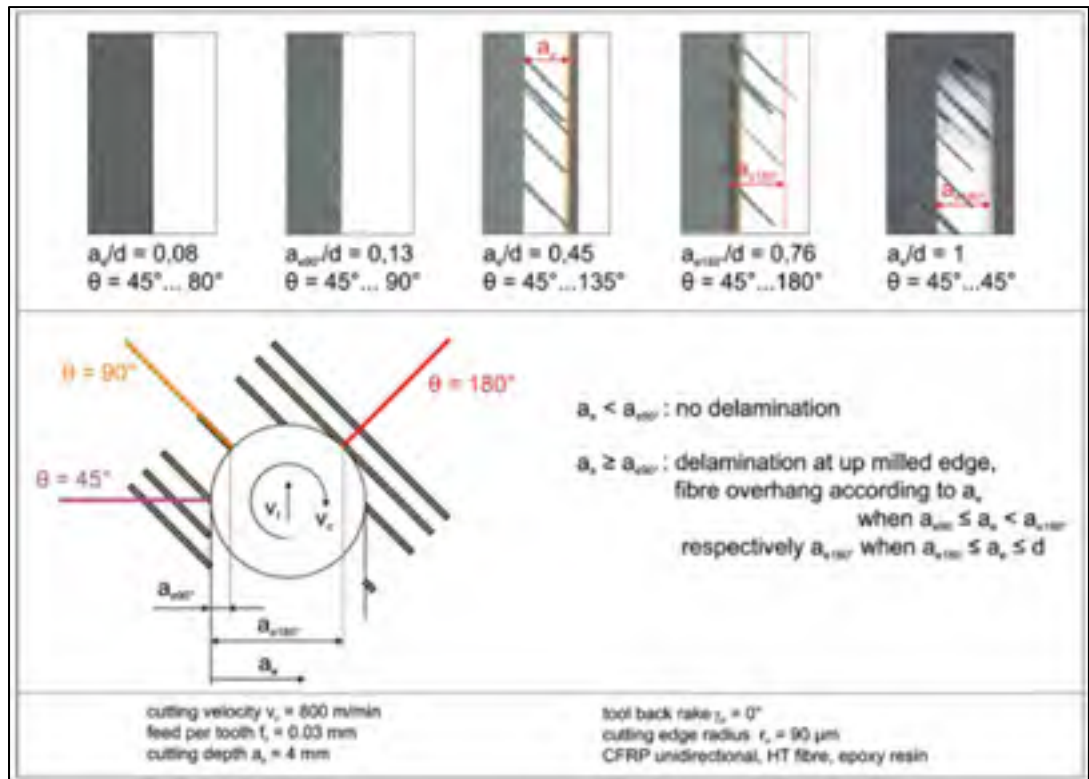
Figure 1.8 Délamination en fonction de la largeur d'usinage sur le diamètre de l'outil pour une orientation du pli de surface de -45^\circ Tirée de (Hintze, Hartmann et Schutte, 2011)
