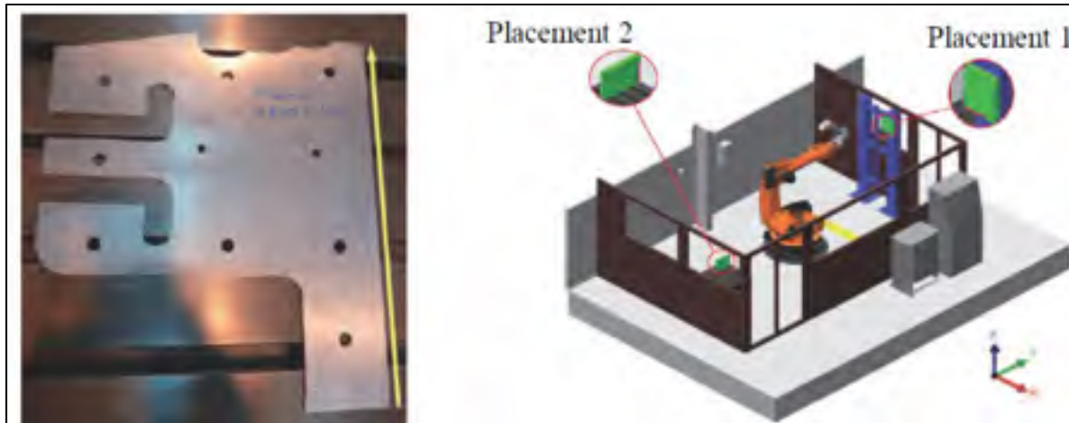
Figure 1.13 Une pièce d'essai et les deux positions de détourage Tirée de (Dumas et al., 2012)
