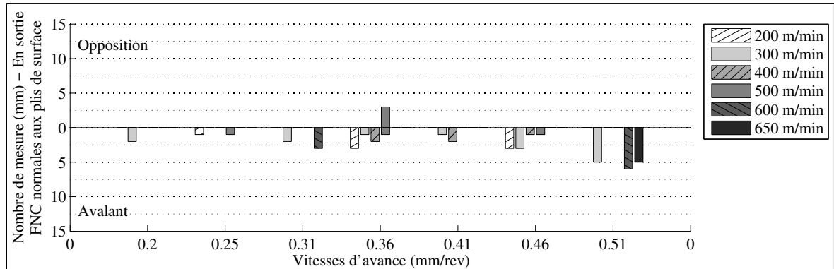
Figure 3.131 NM de FNC normales au pli supérieur en sortie, OP10P4 45° CR10 Y
