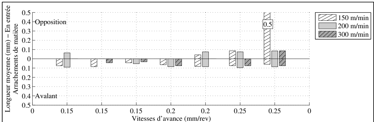
Figure 3.237 LM de l'ARM du pli supérieur en entrée de l'OP50P5 -45° CR20 Y
