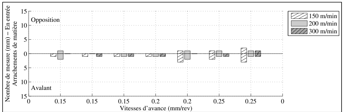
Figure 3.238 NM de l'ARM du pli supérieur en entrée de l'OP50P5 -45° CR20 Y
