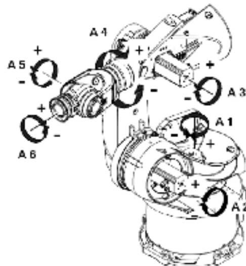
1-3 Drehachsen und Drehinn beim Verfahren des Roboters Rotational axes and directions of rotation in motion of the robot Axes de rotation du robot et sens de rotation lors du déplacement des axes
