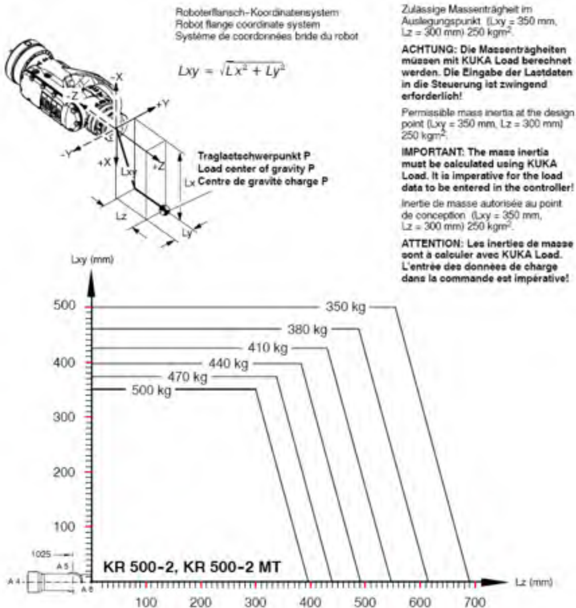
3-6 Traglastschwerpunkt P und Belastungskurven für KR 500-2, KR 500-2 MT Load center of gravity P and loading curves for KR 500-2, KR 500-2 MT Centre de gravité de la charge P et courbes de charge pour KR 500-2, KR 500-2 MT
