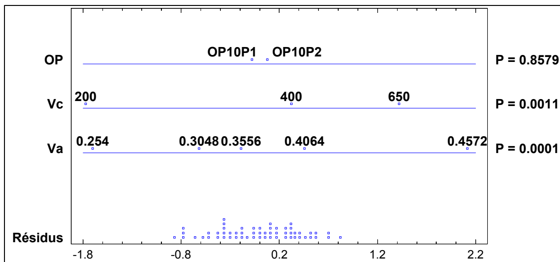
Figure 4.13 ANOVA graphique pour Ra et une orientation du pli à -45^\circ , OP10P1 CR10 et OP10P2 sur centre d'usinage
