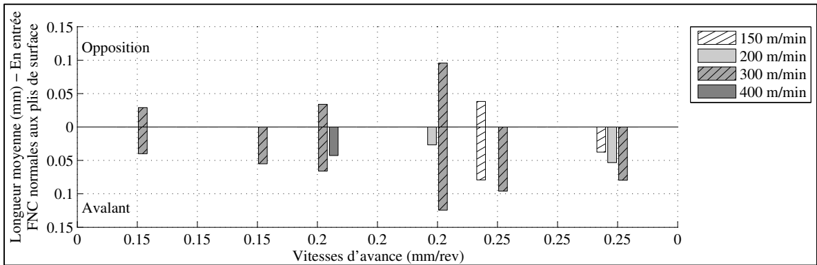
Figure 3.151 LM de FNC normales au pli supérieur en entrée, OP30P3 45° CR20 X
