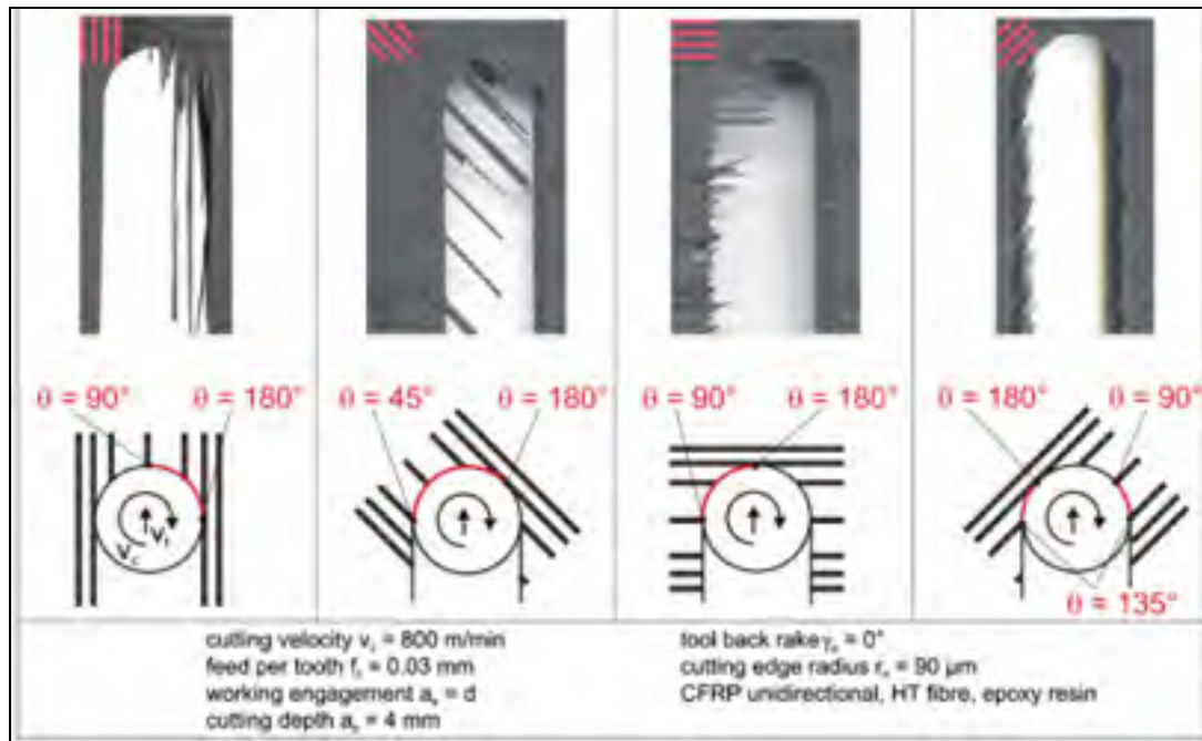
Figure 1.7 Délamination en fonction de l'angle de coupe de fibre critique \theta Tirée de (Hintze, Hartmann et Schutte, 2011)
