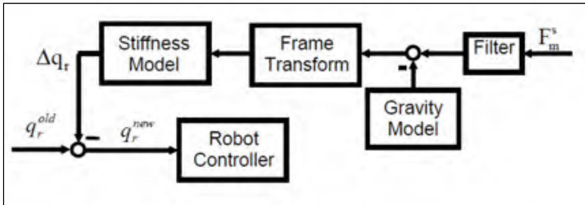
Figure 1.21 Compensation de la déformation en temps réel à l'aide d'un modèle de rigidité et d'un capteur de force Tirée de (Zhang et al., 2005)
