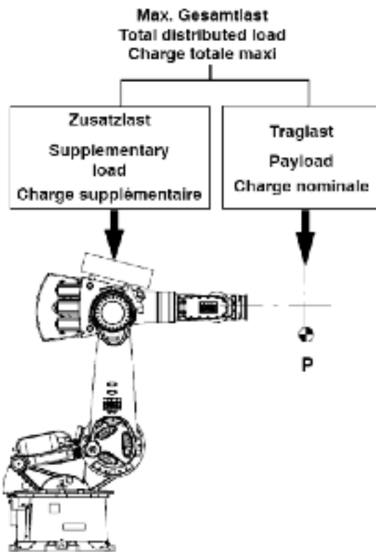
3-1 Lastverteilung Distribution of the total load Distribution de la charge
