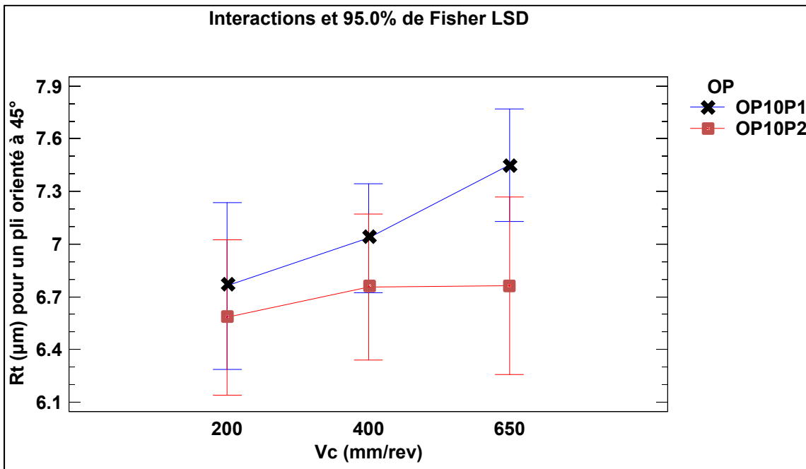
Figure 4.21 Interaction entre la vitesse de coupe ( V_c ) et les opérations pour des valeurs moyennes de R_t mesurées sur un pli orienté à 45^\circ
