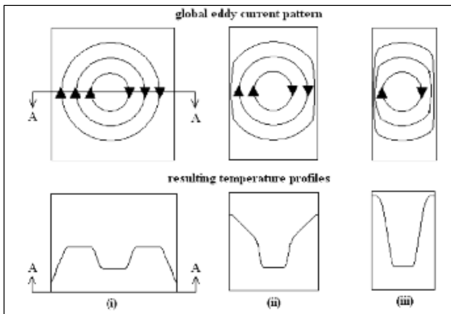
Figure 1-26 Exemples d'effets de bord en fonction de la géométrie de la pièce induite
