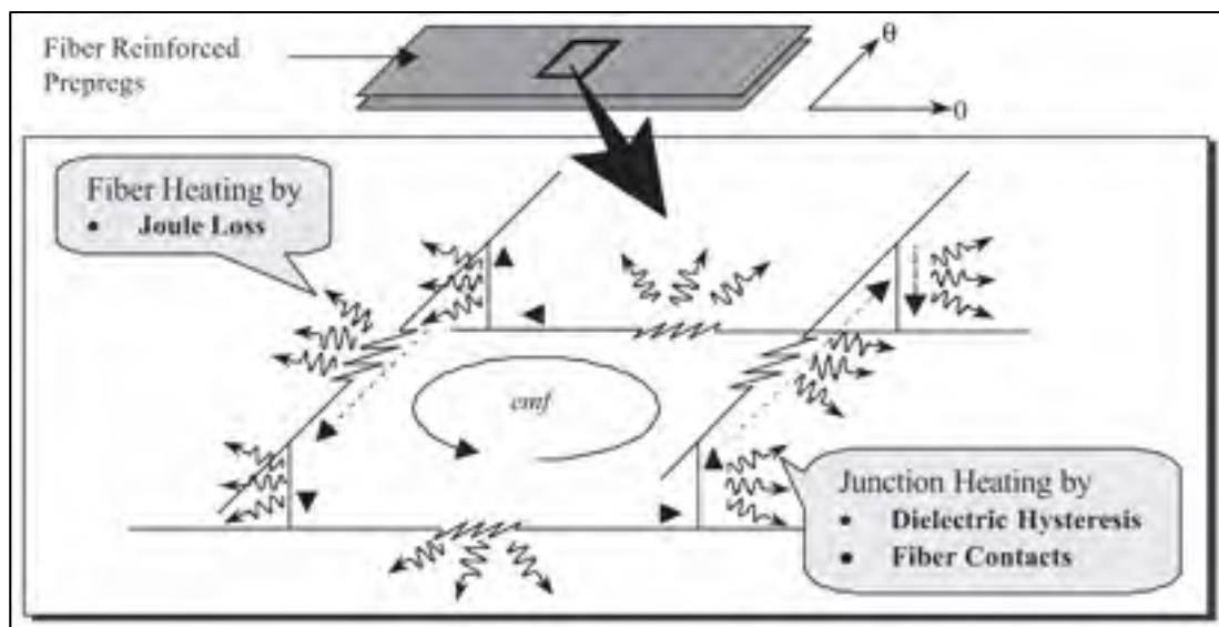
Figure 1-20 Mécanismes de chauffe observables dans un composite à fibres conductrices électriques chauffé par induction Tirée de (Yarlagadda et al., 2002)
