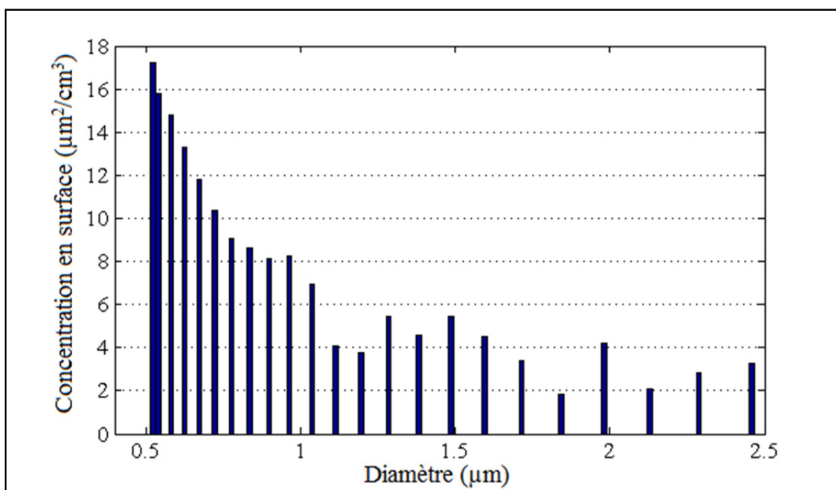
Figure 3-7 Dispersion de la concentration en surface des particules ( PM_{2,5} ) pour le détournage
