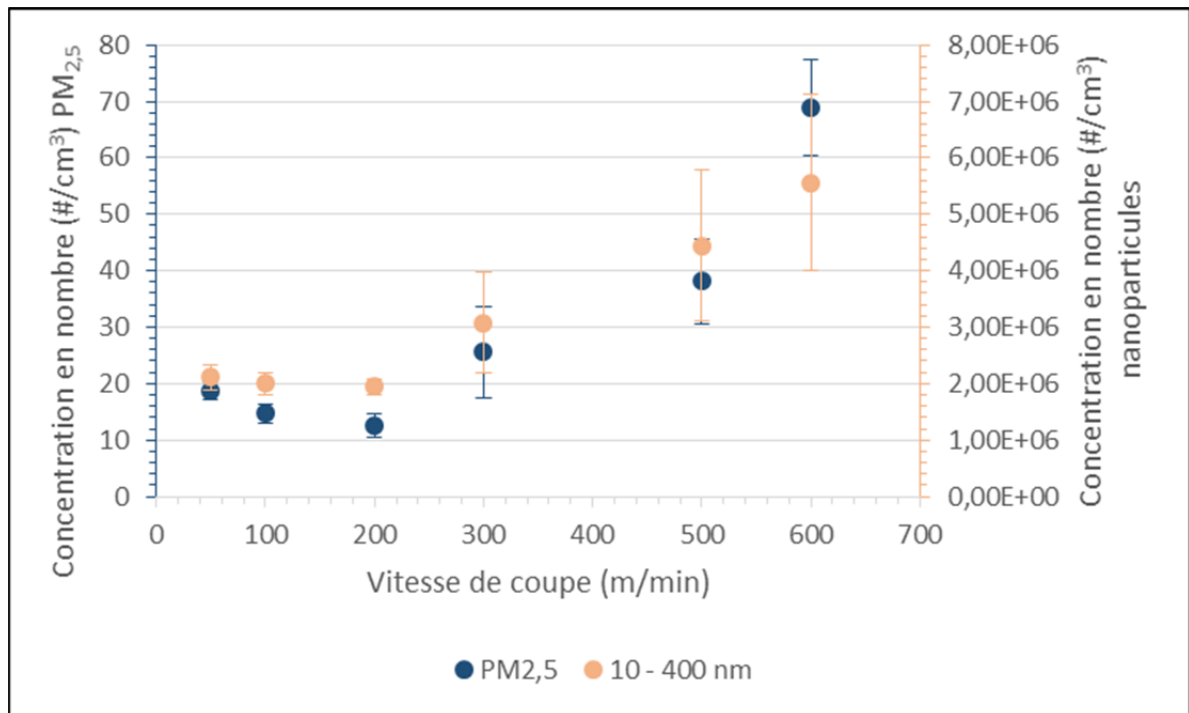
Figure 3-3 Concentration en nombre de particules en fonction de la vitesse de coupe pour le détournage
