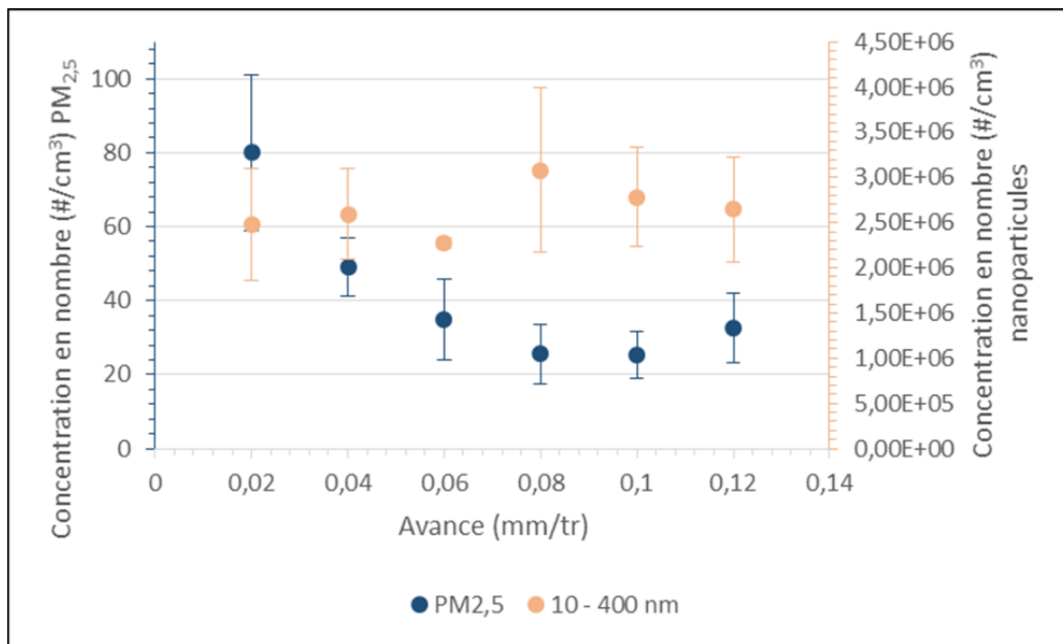
Figure 3-2 Concentration en nombre de particules en fonction de l'outil pour le détournage
