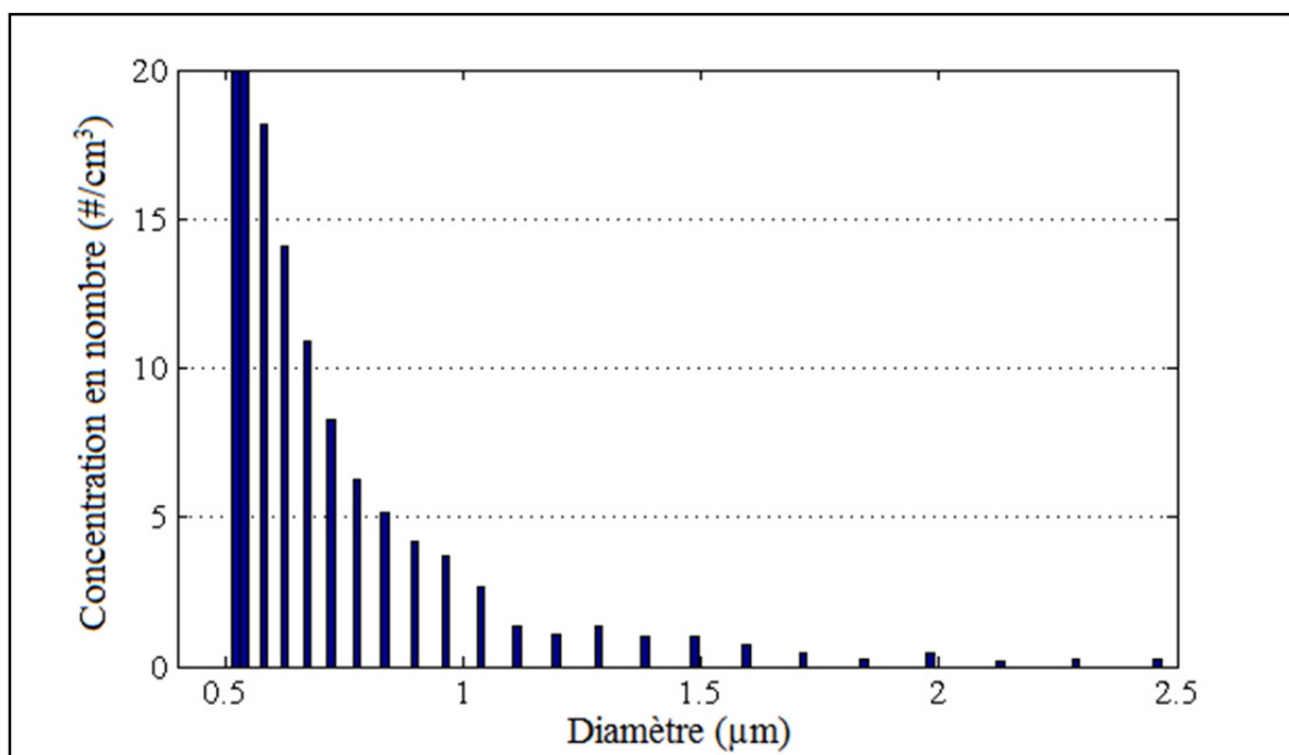
Figure 3-5 Dispersion de la concentration en nombre de particules ( PM_{2,5} ) pour le détourage
