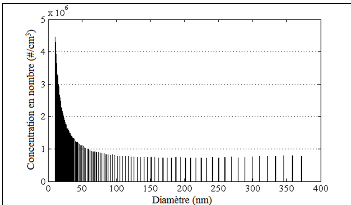
Figure 3-6 Dispersion de la concentration en nombre de particules (10 – 400 nm) pour le détourage
