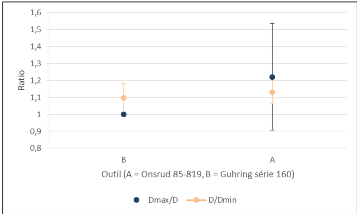
Figure 5-16 Défauts de coupe en fonction de l'outil pour le perçage
