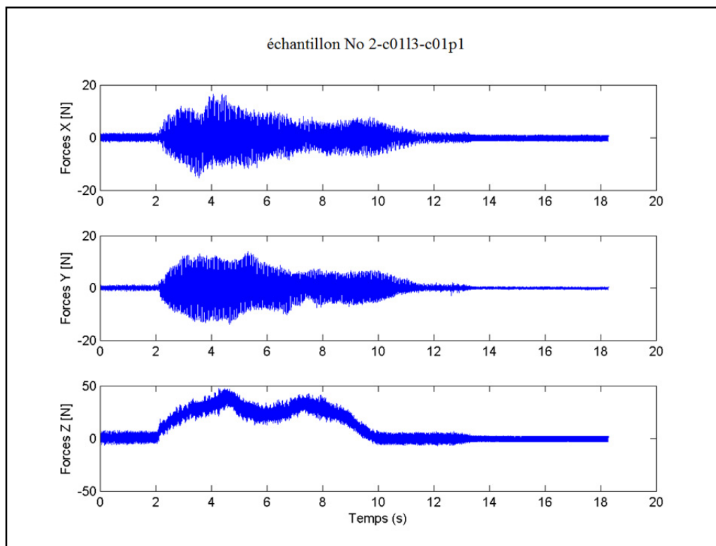
Figure 5-2 Graphique des forces de coupe lors du perçage
