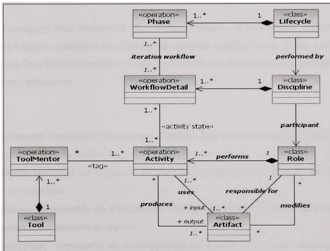
Figure 3.2 Représentation partielle du méta-modèle de RUP.
