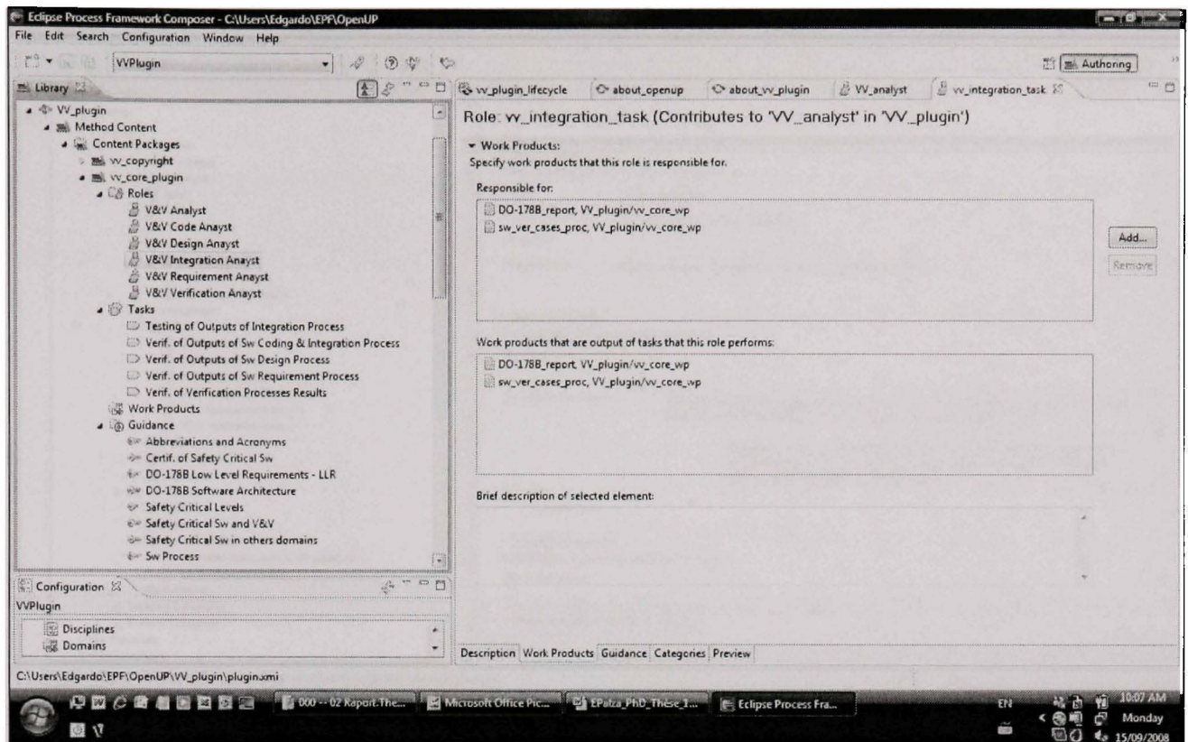
Figure 8.2 Les rôles dans le plugiciel de la V&V.
