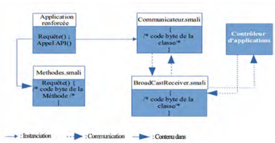
Figure 3.7 Mécanisme de communication contrôleur-applications réécrites
