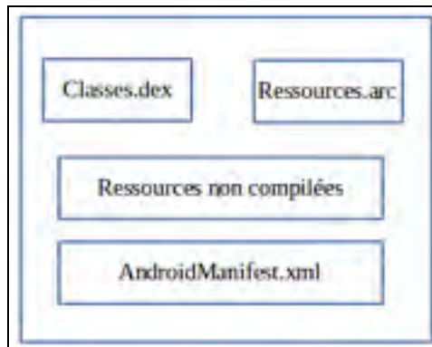
Figure 1.3 Composition d'un fichier APK
