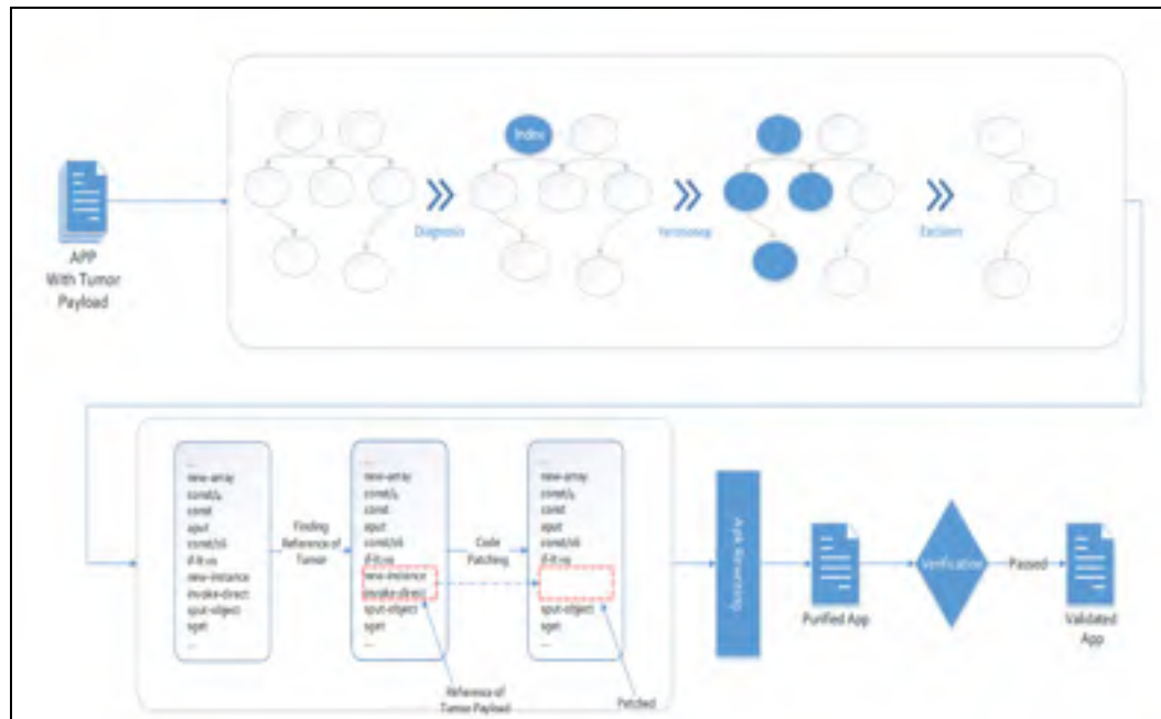
Figure 2.13 Processus de purification de l'apk. Tirée de (Yang et al., 2014)
