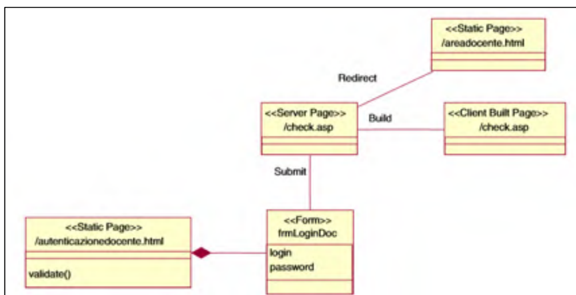
Figure 1.4 WARE, diagramme de classe Tirée de (Di Lucca, Fasolino et al. 2004)
