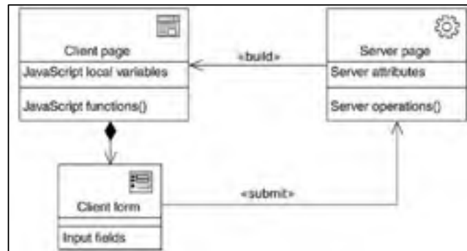
Figure-A VI-2 association « build » Tirée de (Conallen 2003)
