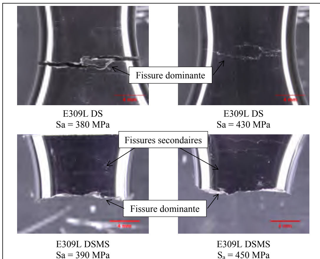
Figure 4.28 - Amorces à la surface d'éprouvettes après essais de fatigue
