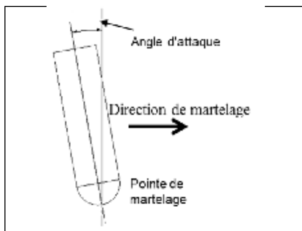
Figure 3.6 Paramètres de déplacement de l'outil de martelage
