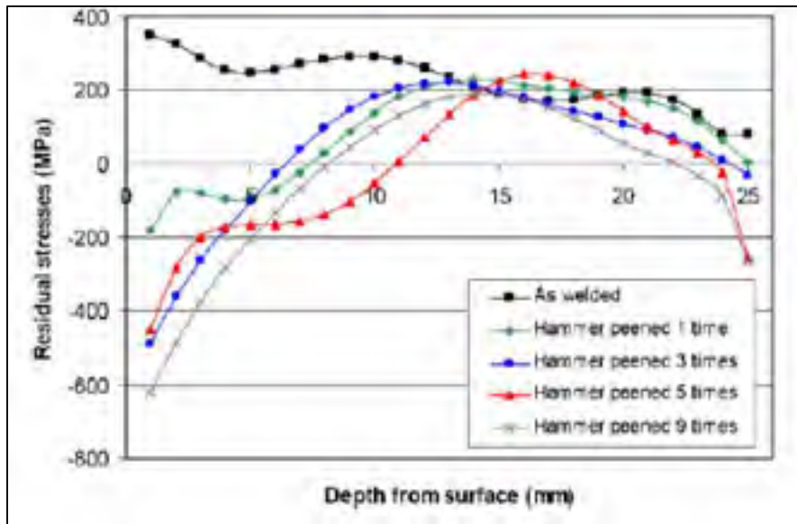
Figure 1.18 Profondeur des contraintes de compressions induites selon le nombre de passes de martelage (Hacini, Lê et Bocher, 2008b)
