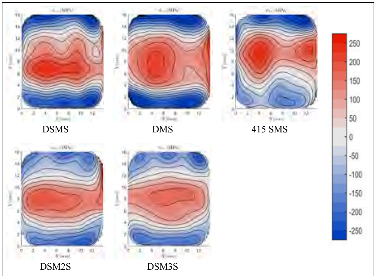
Figure 4.18 Distribution des contraintes résiduelles longitudinales dans les éprouvettes au niveau de la section critique
