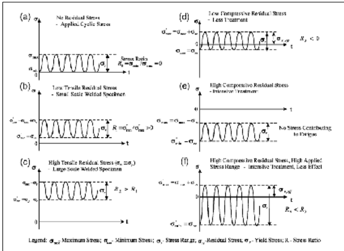
Figure 1.4 Influence des contraintes résiduelles sur un chargement cyclique R > 0 (Cheng et al., 2003)
