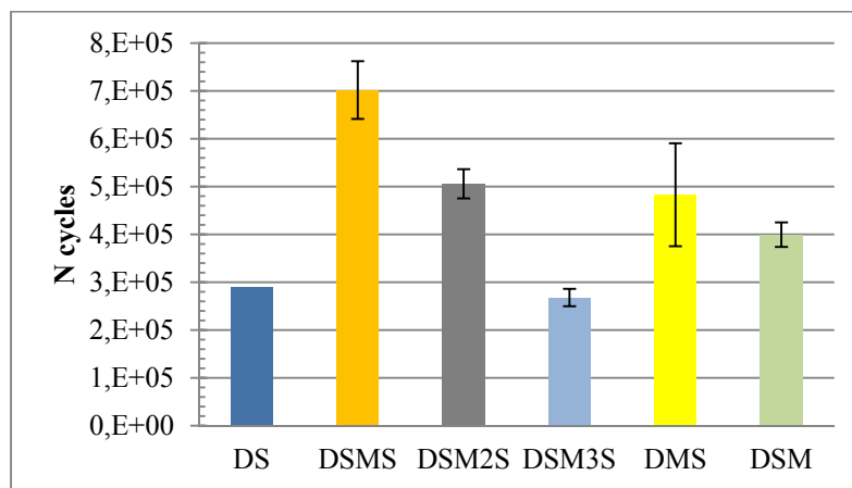
Figure 4.26 Endurance E309L à S_a = 390 MPa
