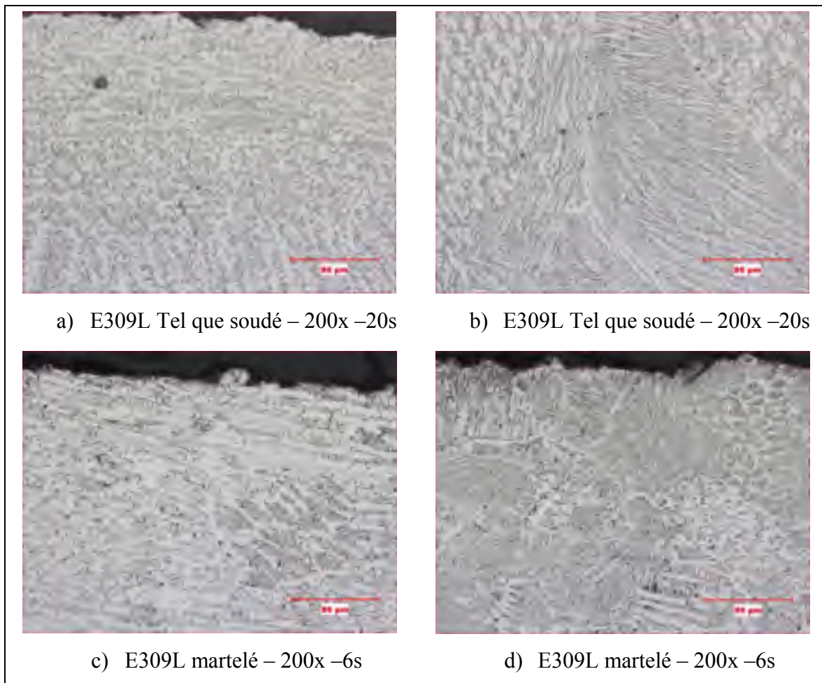
Figure 3.17 Structure de l'acier E309L observée en surface avec une attaque à l'acide oxalique, grossissement 200x a) Tel que soudé attaque 20s b) Tel que soudé attaque 20s c) martelé attaque 6s d) martelé attaque 6s
