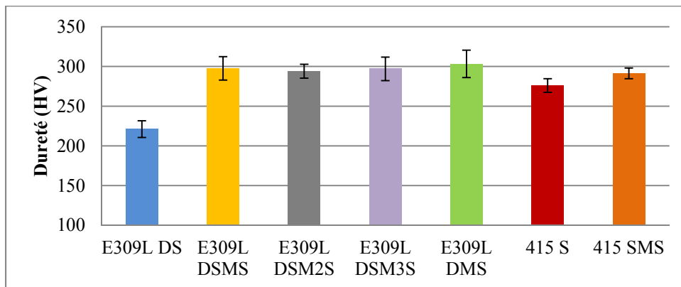
Figure 4.20 Dureté HV à la surface du dépôt selon la séquence d'opérations (mesure 300gF, 10 s)
