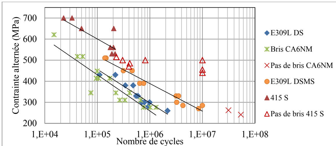
Figure 4.25 Résultats de fatigue du E309L DS, E309L DSMS et 415 S comparé aux résultats du CA6NM en traction R=-1
