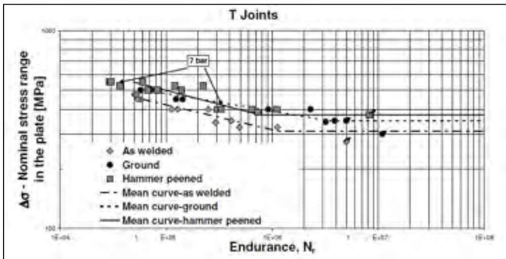
Figure 1.19 Courbes S-N des joints en T tel que soudés, ayant subi un meulage du raccordement ou ayant été martelés. Flexion 3 point, R=0,1 , acier 52-3 (Branco, Infante et Baptista, 2004)
