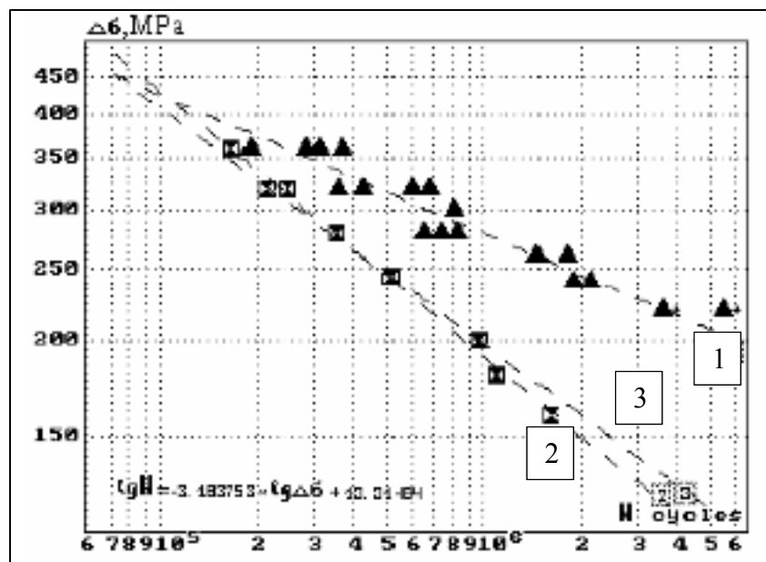
Figure 1.6 Courbe S-N de joints d'acier à faible carbone soudés bout à bout sans contraintes résiduelles (1) et avec contraintes résiduelles élevées réelles (2) ou simulées (3) adapté de (Trufyakov, Mikheev et Kudryavtsev, 1995)
