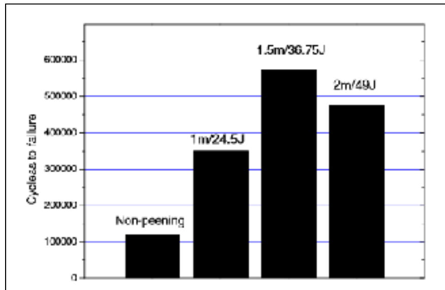
Figure 1.22 Vie en fatigue d'échantillons d'alliage d'aluminium 2A12-T4 martelés avec trois énergies différentes (Liu et al., 2009)
