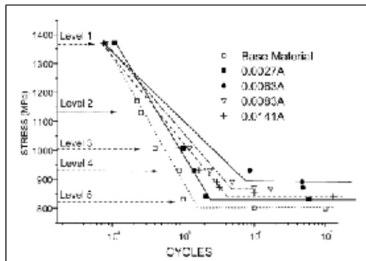
Figure 1.14 Effet de l'intensité de grenaillage sur l'endurance de l'acier 4130 (Torres et Voorwald, 2002)
