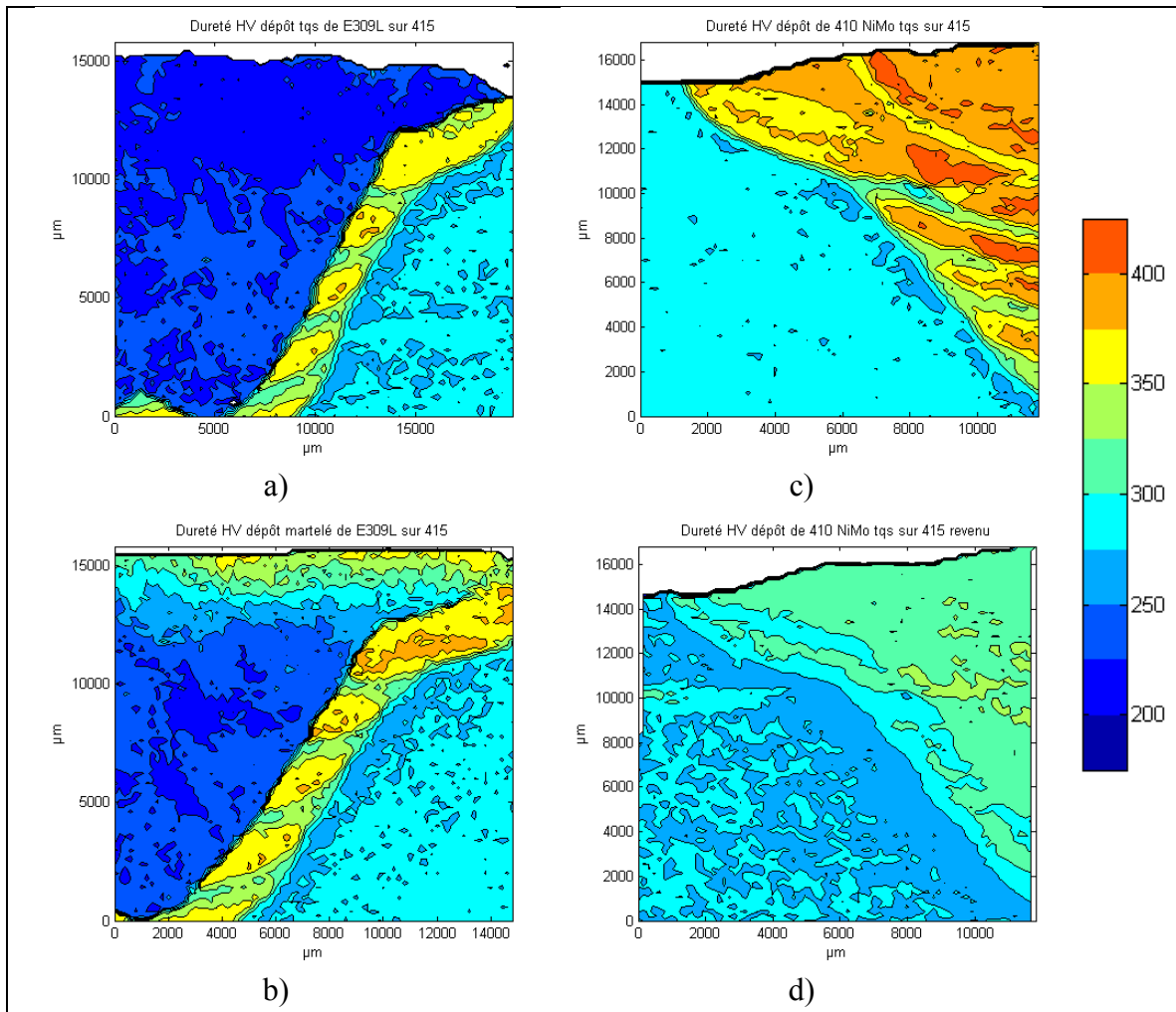
Figure 3.16 - Microdureté HV mesurée avec 300 gF de a) Dépôt de E309L sur 415 b) Dépôt de E309L martelé sur 415 c) Dépôt de 410 NiMo sur 415 d) Dépôt de 410 NiMo sur 415 après revenu de 2h à 620°C
