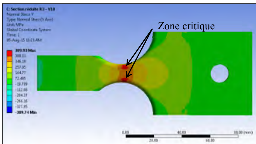
Figure 4.10 - Contrainte normale longitudinale calculée par la méthode des éléments finis pour une force de 3,5 kN
