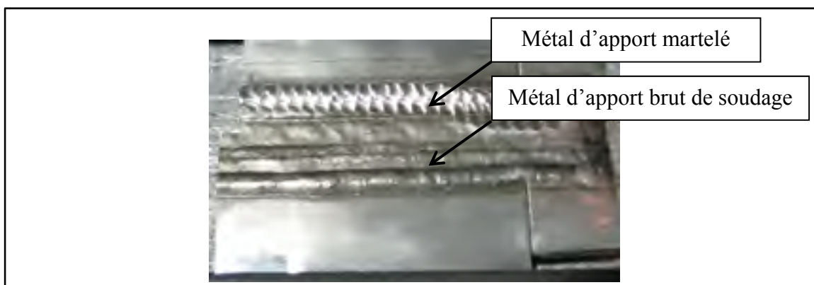
Figure 4.2 Plaque en cours de martelage brut de soudage
