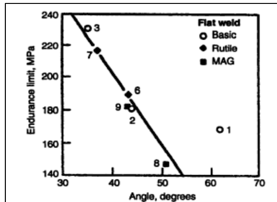
Figure 1.12 Influence de l'angle \theta sur la limite d'endurance d'un joint soudé avec différents types de métaux d'apport (Lampman, 1997)
