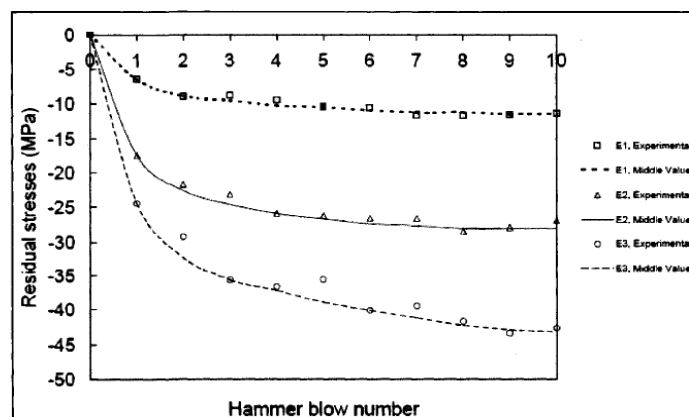
Figure 1.16 Contrainte résiduelle mesurée à 12,5 mm de l'impact sur une plaque d'acier initialement non contrainte (Hacini et Lê, 2009)
