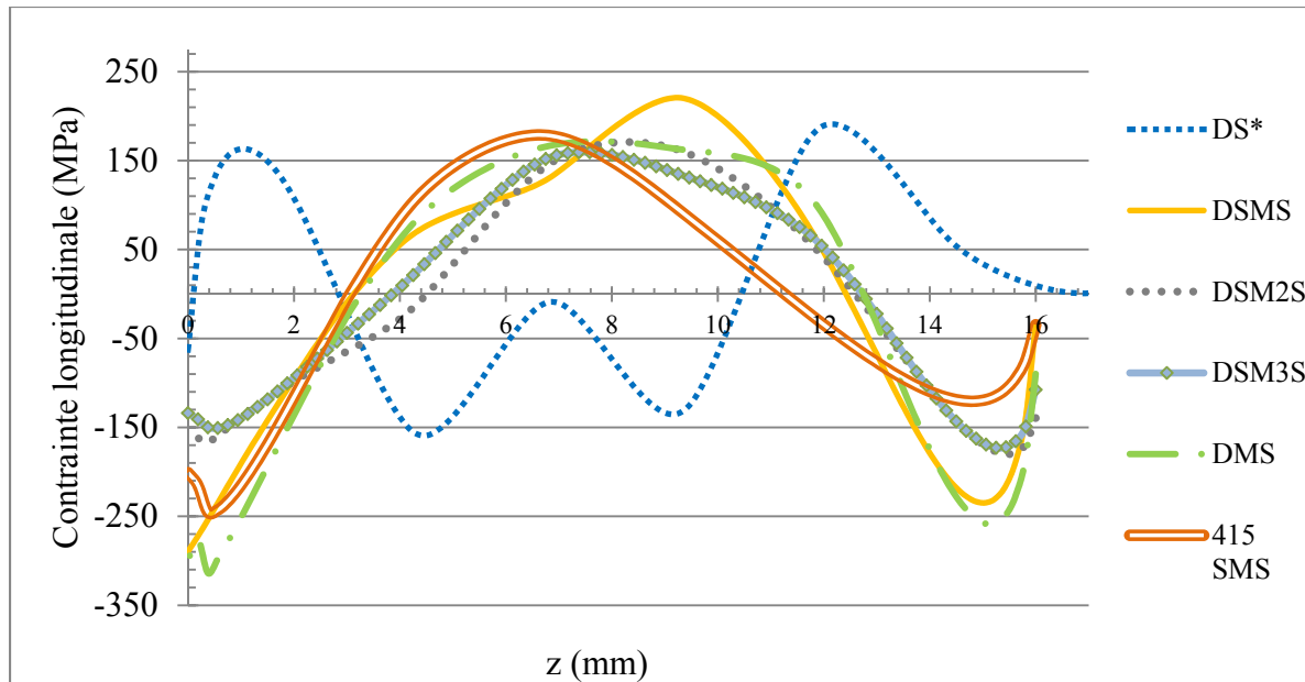
Figure 4.19 Profil des contraintes résiduelles longitudinales moyennes sous la surface des éprouvettes *DS est calculé à partir de l'éprouvette Figure 4.17-a
