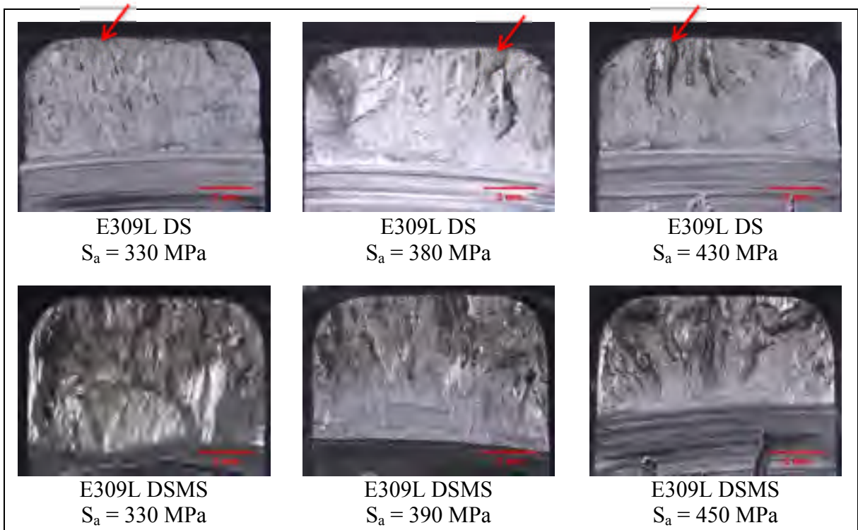
Figure 4.29 - Faciès de rupture des éprouvettes de E309L DS et DSMS avec site d'amorce identifié lorsque possible (flèche rouge)
