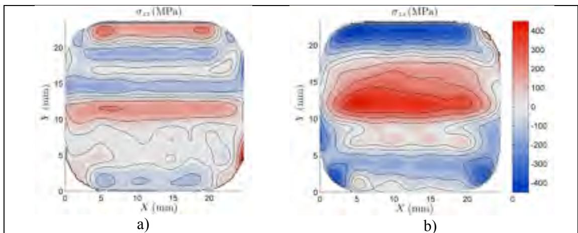
Figure 4.17 Contraintes résiduelles à la section critique dans une éprouvette de a) E309L DS b) E309L DMS
