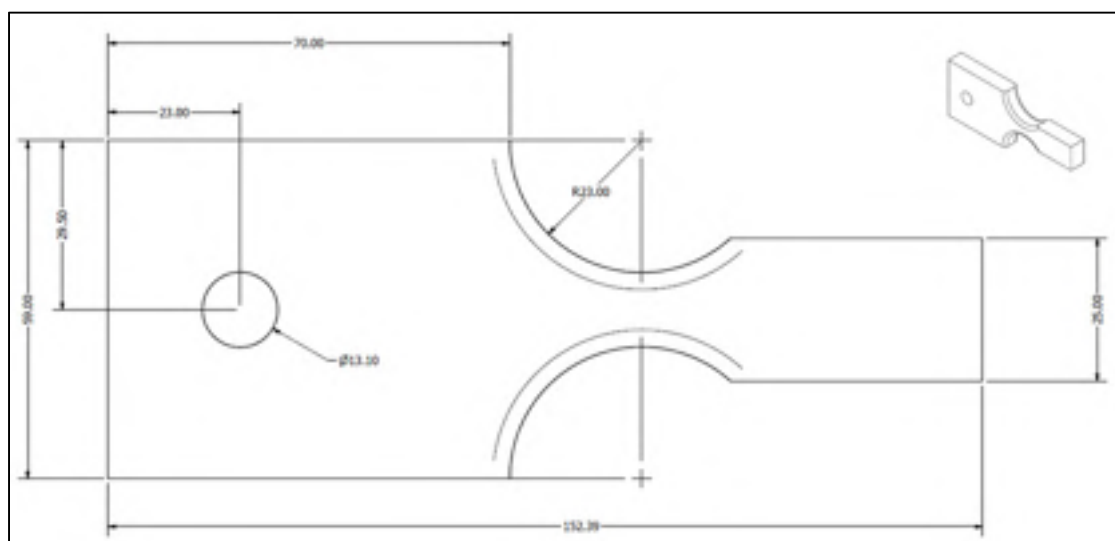
Figure 4.8 - Géométrie de l'éprouvette utilisée lors des essais de fatigue en flexion alternée (dimensions en millimètres)
