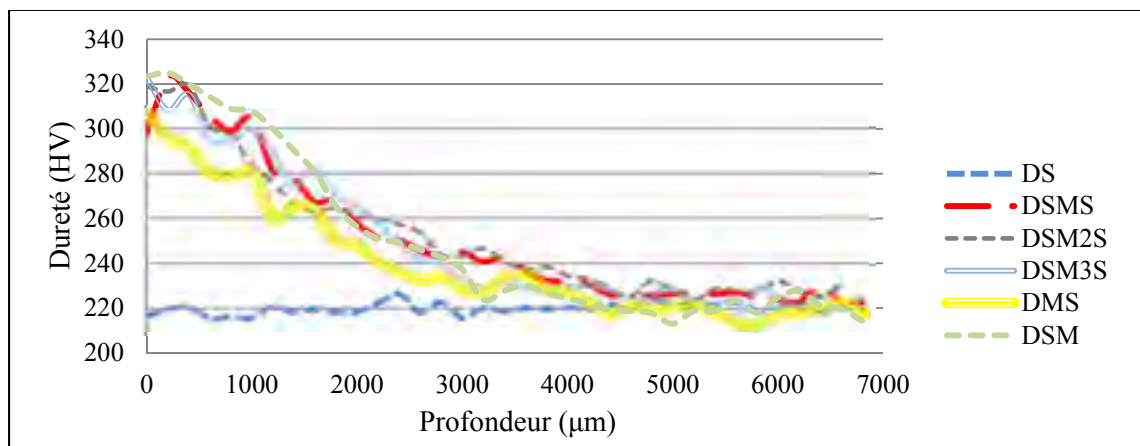
Figure 4.21 Dureté HV dans l'épaisseur des échantillons de E309L selon le traitement de surface (mesure 300 gF, 10 s)
