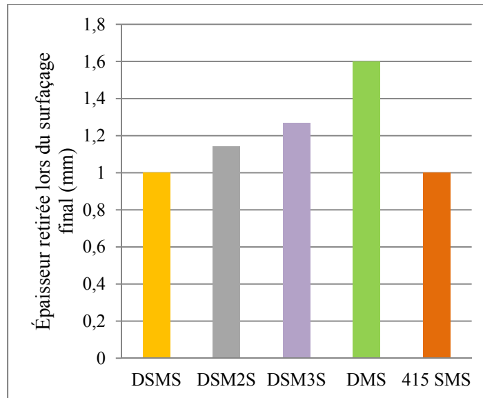
Figure 4.16 Épaisseur de métal retiré lors de l'étape de surfacage postmartelage
