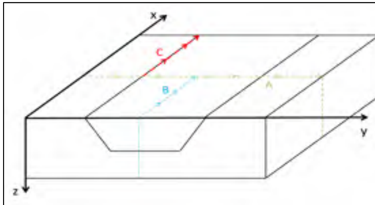
Figure 3.9 Schéma montrant les différentes coupes effectuées pour l'application de la méthode du contour
