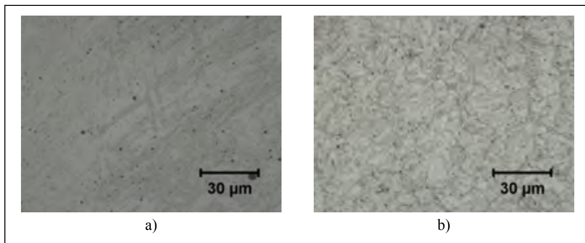
Figure 3.18 - Microstructure du 410 NiMo 500x - Villellas 20s, a) tel que déposé - Villellas 30s b) revenu 2h à 620°C
