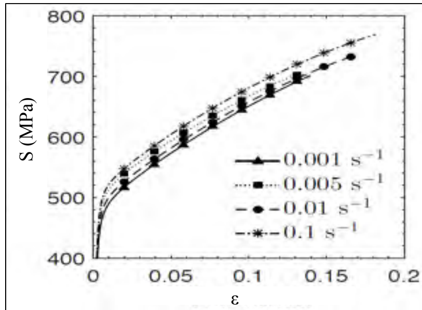
Figure 3.3 - Courbe de traction transversale aux dépôts E309L (Luk-Cyr, J., Courriel envoyé à Jean-Loup Curtat, déc. 2015. Reproduit avec l'autorisation de Jacques Luk-Cyr)
