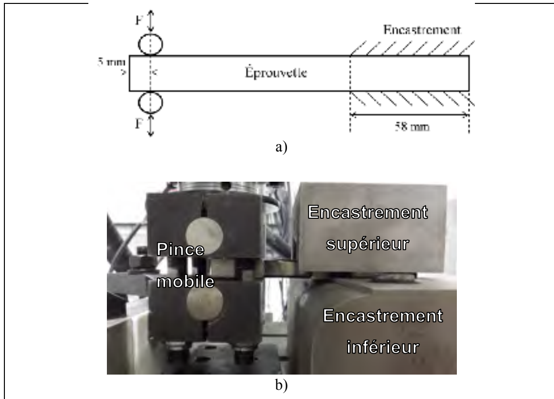
Figure 4.9 - Montage expérimental utilisé pour les essais de fatigue en flexion alternée a) montage schématique b) montage réel
