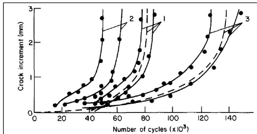
Figure 1.24 - Propagation de fissure pour un échantillon: 1) non martelé; 2) martelé pression d'outil 0,3 MPa; 3) Martelé pression d'outil 0,5 MPa (Kopsov, 1991)
