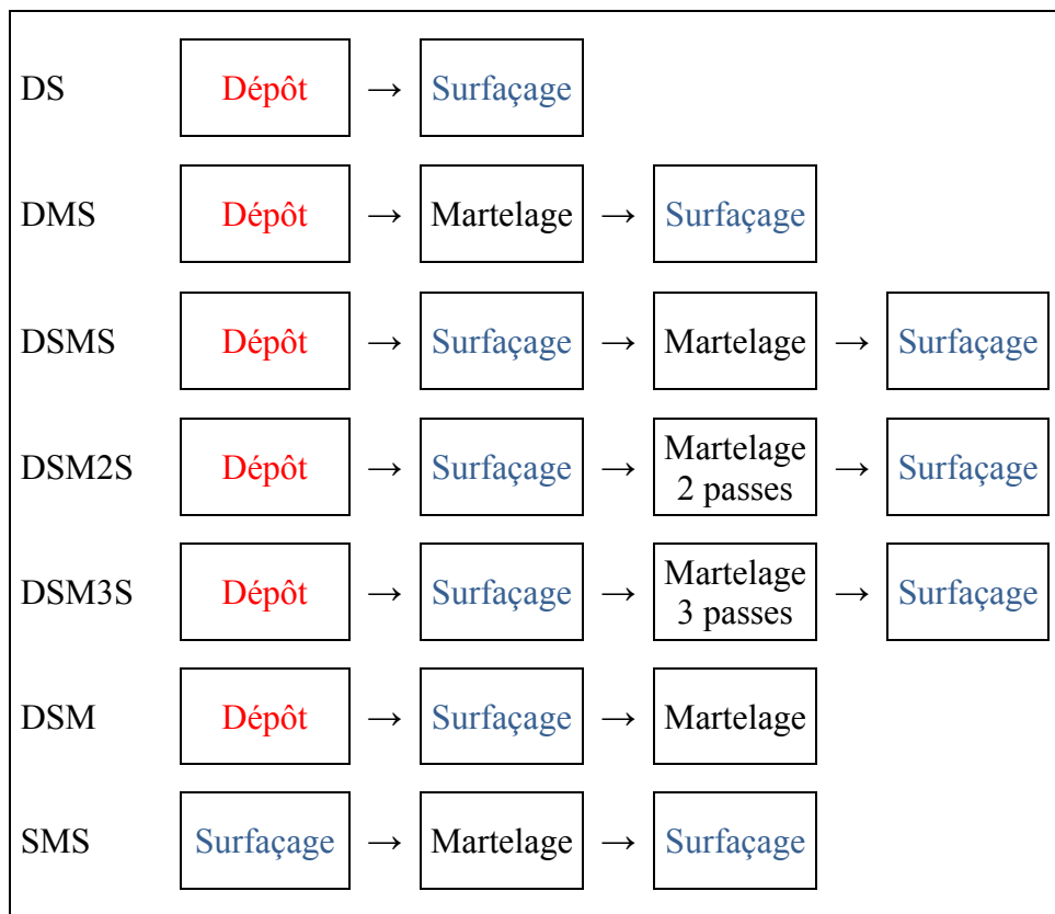
Figure 4.5 Procédures de réparation étudiées
