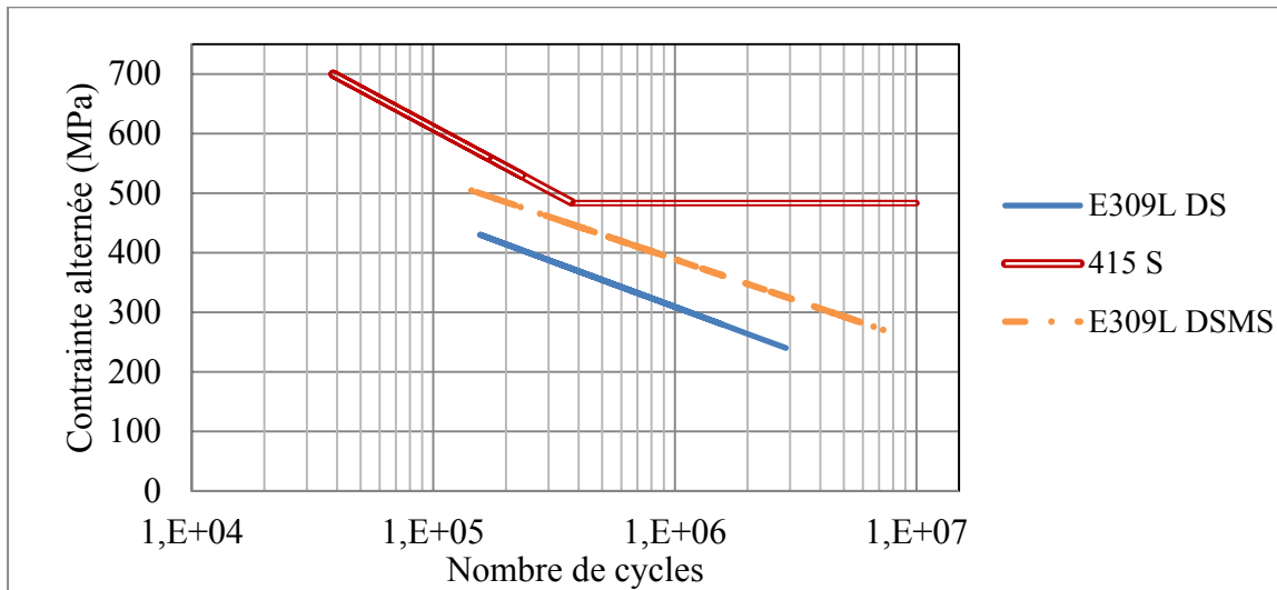
Figure 4.24 Courbes S-N du E309L DS, E309L DSMS et 415 S pour une probabilité de bris de 50%
