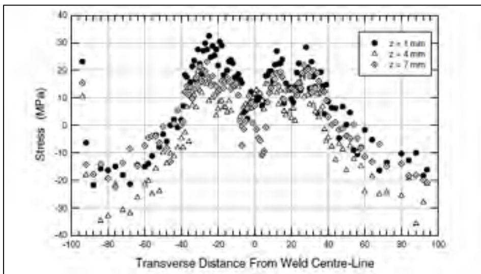
Figure 1.2 Contrainte longitudinale le long de la soudure selon la distance par rapport au cordon de soudage (James et al., 2007)
