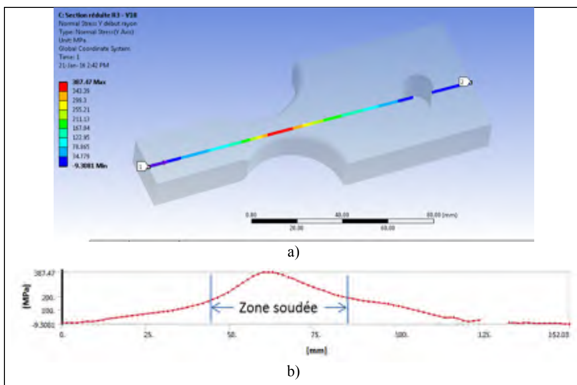
Figure 4.11 a) Trajectoire parallèle à l'axe de l'éprouvette et passant dans la zone critique b) Variation de la contrainte longitudinale le long de cette trajectoire
