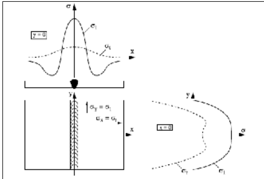
Figure 1.1 Contraintes résiduelles longitudinales et transversales dues au soudage d'une plaque (Kaplan et Murry, 2010)
