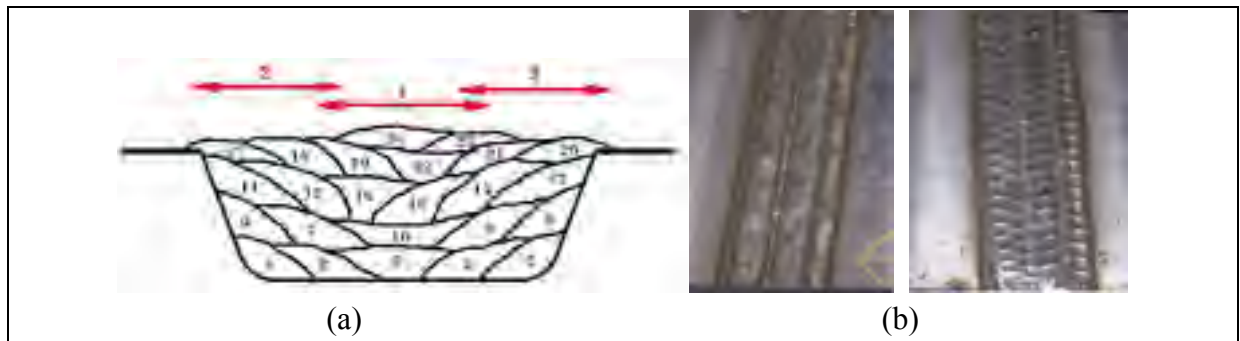
Figure 3.8 (a) Disposition des trois bandes de martelage et (b) aspect du dépôt avant (gauche) et après martelage (droite)
