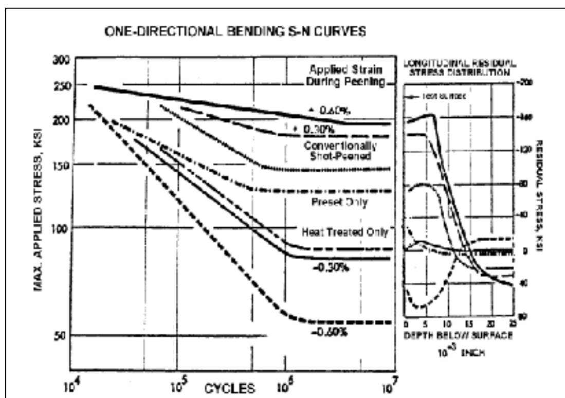
Figure 1.7 Courbes S-N et contraintes résiduelles à la surface d'échantillons grenaillés sous déformation imposée (Mattson et Roberts, 1959)
