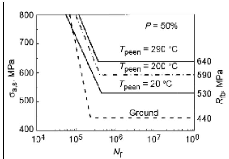
Figure 1.10 Courbes S-N à probabilité de bris P=50\% de l'acier 4140 trempé, revenu et grenaillé à différentes températures (Wick, Schulze et Vöhringer, 2000)
