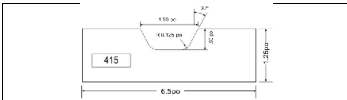
Figure 3.1 Géométrie de la préparation de soudage usinée dans les plaques d'acier 415
