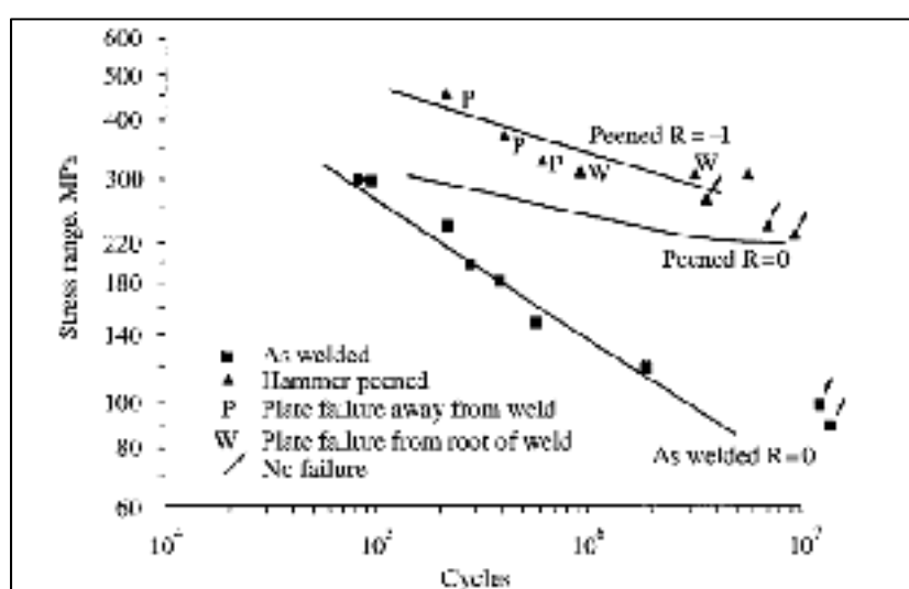
Figure 1.20 Amélioration de la vie en fatigue due au martelage de joints soudés en acier (Booth, 1977)
