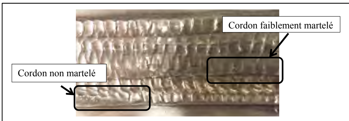
Figure 4.3 Surface irrégulière avec défauts de martelage
