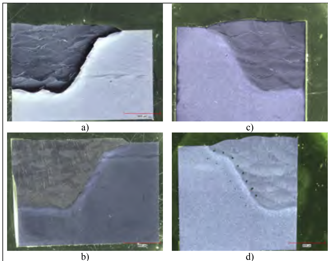
Figure 3.15 - Échantillons métallographiques de a) Dépôt de E309L sur 415 b) Dépôt de E309L martelé sur 415 c) Dépôt de 410 NiMo sur 415 d ) Dépôt de 410 NiMo sur 415 après revenu de 2h à 620°C
