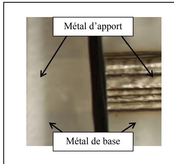
Figure 4.1 Métal d'apport surfacé (gauche) et tel que soudé (droite)
