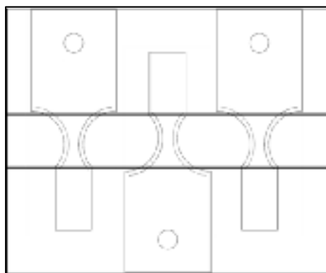
Figure 4.7 - Schéma de prélèvement des éprouvettes de fatigue
