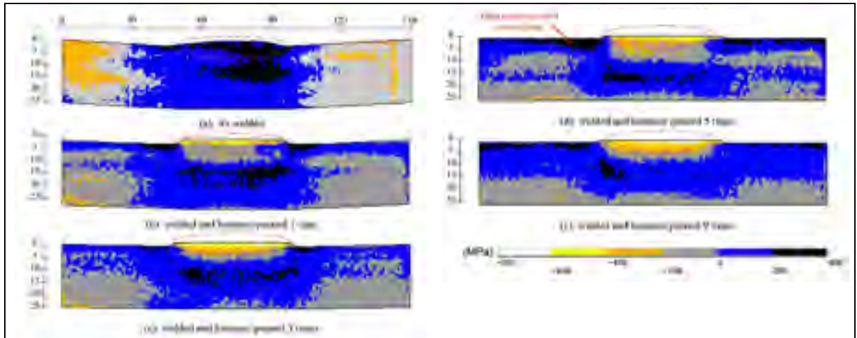
Figure 1.17 Contraintes résiduelles longitudinales dans un joint de E308L déposé sur du 304. État a) tel que soudé b) 1 passe de martelage c) 3 passes de martelage d) 5 passes de martelage f) 9 passes de martelage (Hacini, Lê et Bocher, 2008b)
