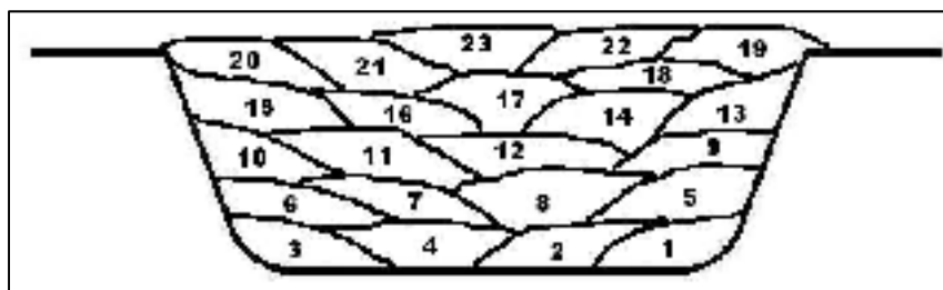
Figure 3.2 Séquence typique des cordons de soudure déposés sur les plaques d'acier 415
