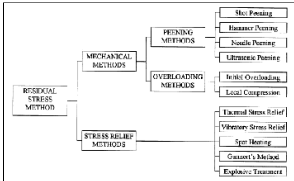
Figure 1.13 Méthodes d'amélioration de la vie en fatigue d'un joint soudé reposant sur la modification du champ de contraintes (Haagensen, 1985)
