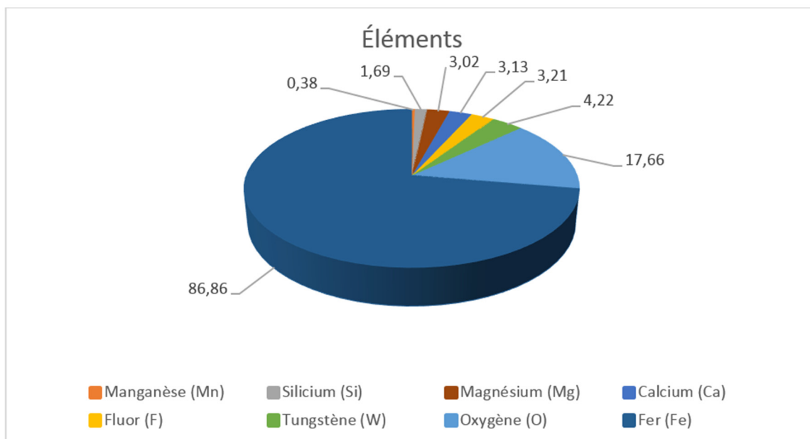
Figure 3.16 Répartition moyenne des divers éléments chimiques retrouvés sur les coupons (T03, T06, T20, T23, T28 et T50)
