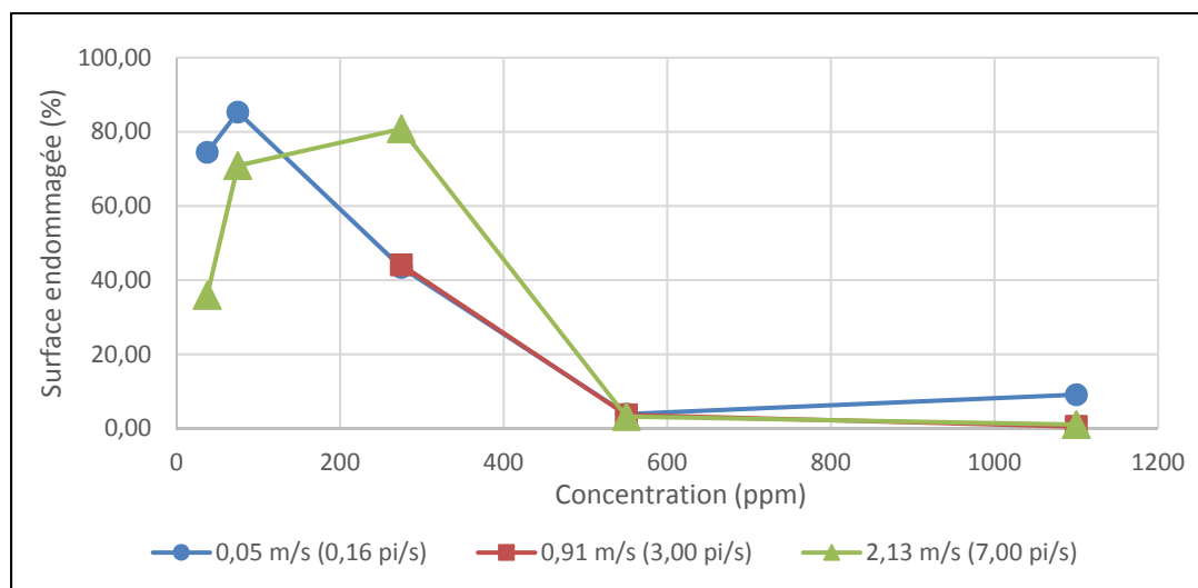
Figure 3.8 Variation de la surface relative endommagée des coupons en fonction de la concentration de tanins pour chaque vitesse d'écoulement
