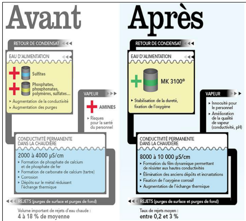
Figure 1.1 Différence de performance entre les produits conventionnels (avant) et le tanin TG3106 (après) (Technologies propres TGWT, 2013)
