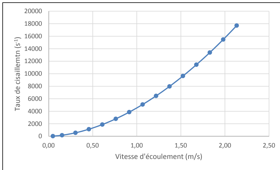
Figure 3.1 Taux de cisaillement dans le montage expérimental pour un fluide newtonien
