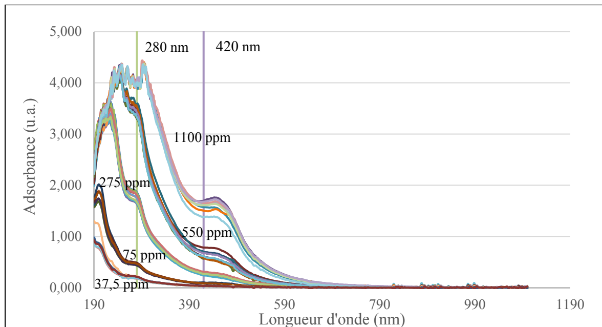
Figure 3.17 Absorbance du TG 3304 en fonction de la longueur d'onde pour différentes concentrations de tanins (Spectroquant Pharo 300)
