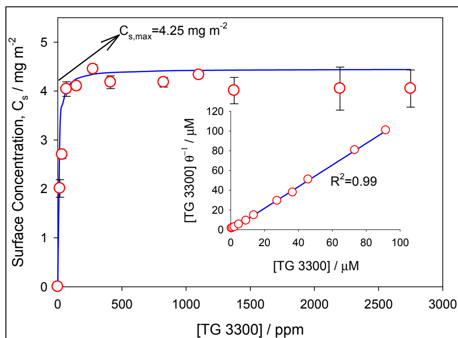
Figure 1.3 Isotherme d'adsorption des tanins purifiés (TG3300) sur l'acier doux à pH 10,50 et température de la pièce (Dargahi et al., 2015)
