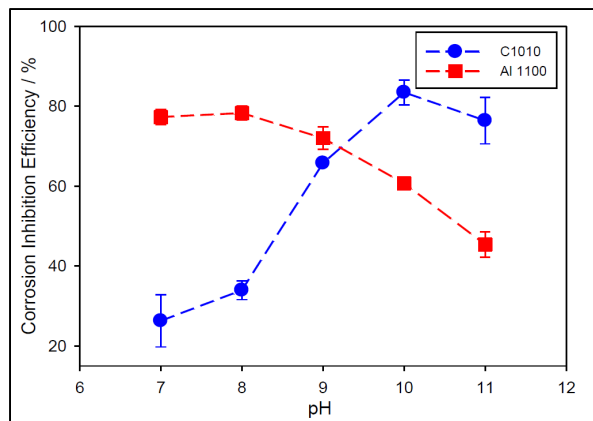
Figure 1.5 Efficacité d'inhibition de la corrosion sur l'acier 1010 et l'aluminium Al 100 à l'aide du TG3300 (Gaudreault et al., 2013)
