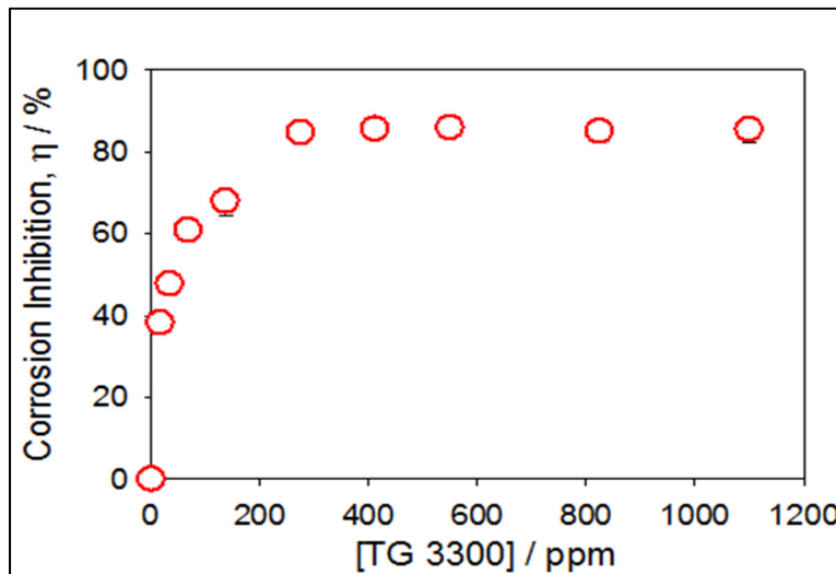
Figure 1.4 Efficacité d'inhibition de la corrosion de l'acier doux en fonction de la concentration de tanins purifiés (TG 3300) (Dargahi et al., 2015)
