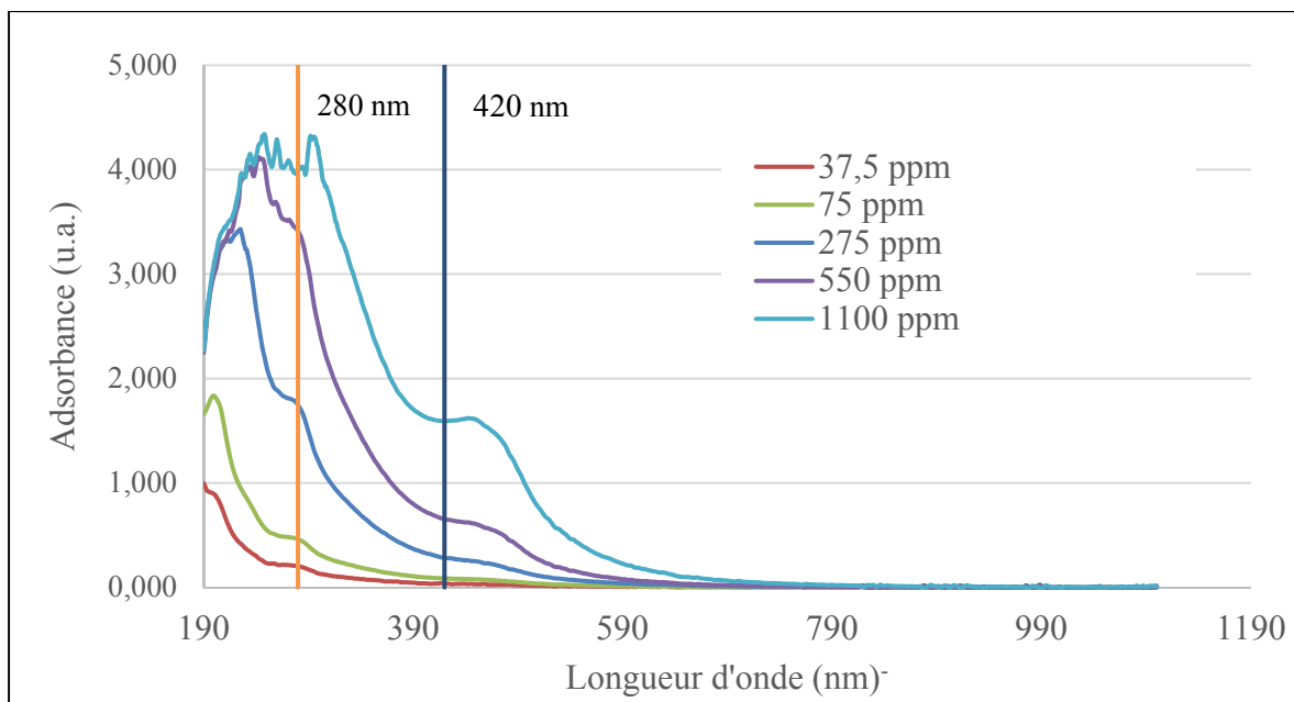
Figure 3.18 Absorbance moyenne du TG 3304 en fonction de la longueur d'onde pour différentes concentrations de tanins (Spectroquant Pharo 300)
