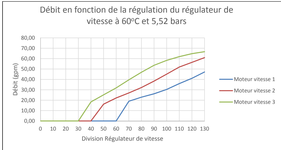
Figure A I-1 Courbe de performance de la pompe de recirculation
