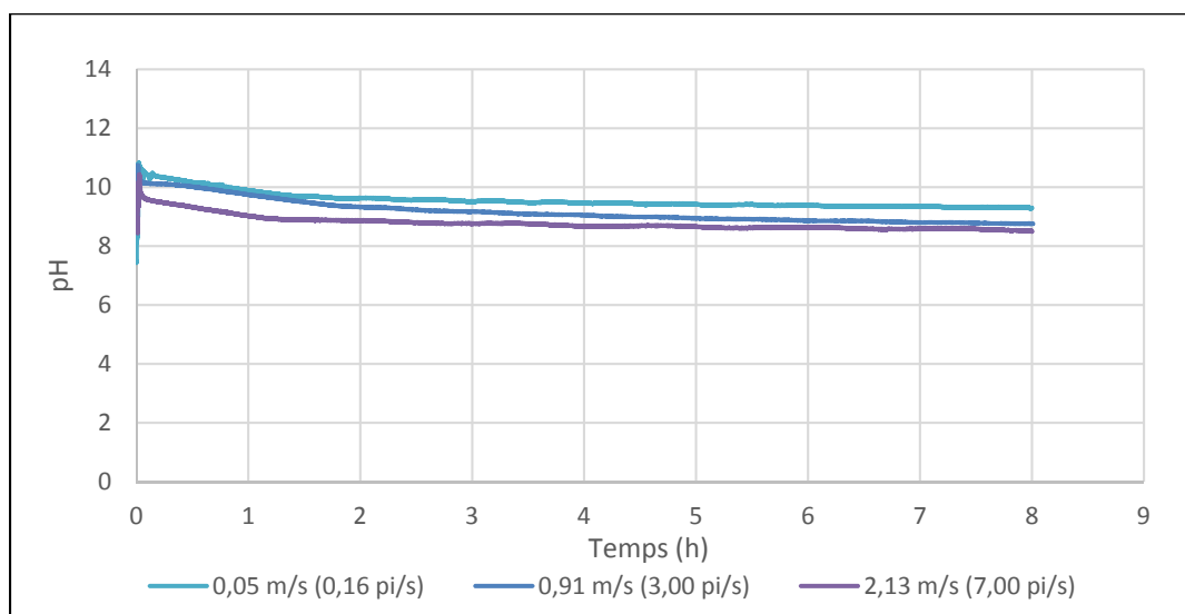
Figure 3.6 Variation du pH pour différentes vitesses à une concentration de tanins de 275 ppm
