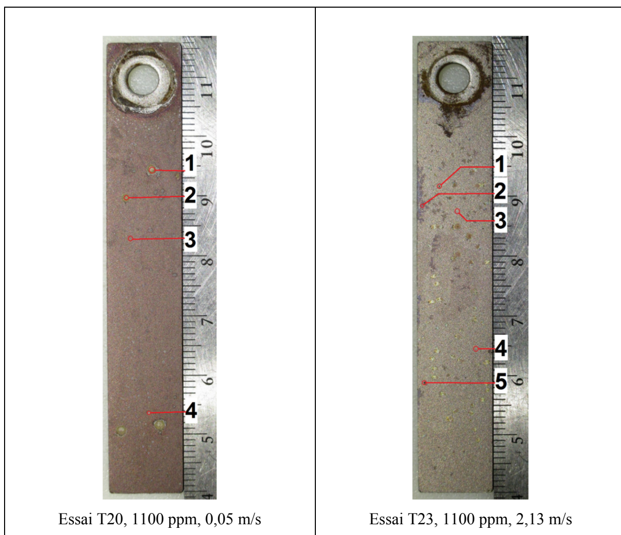
Figure 3.15 Coupons en acier doux- Essai T20 et T23 analysés par diffraction rayon X
