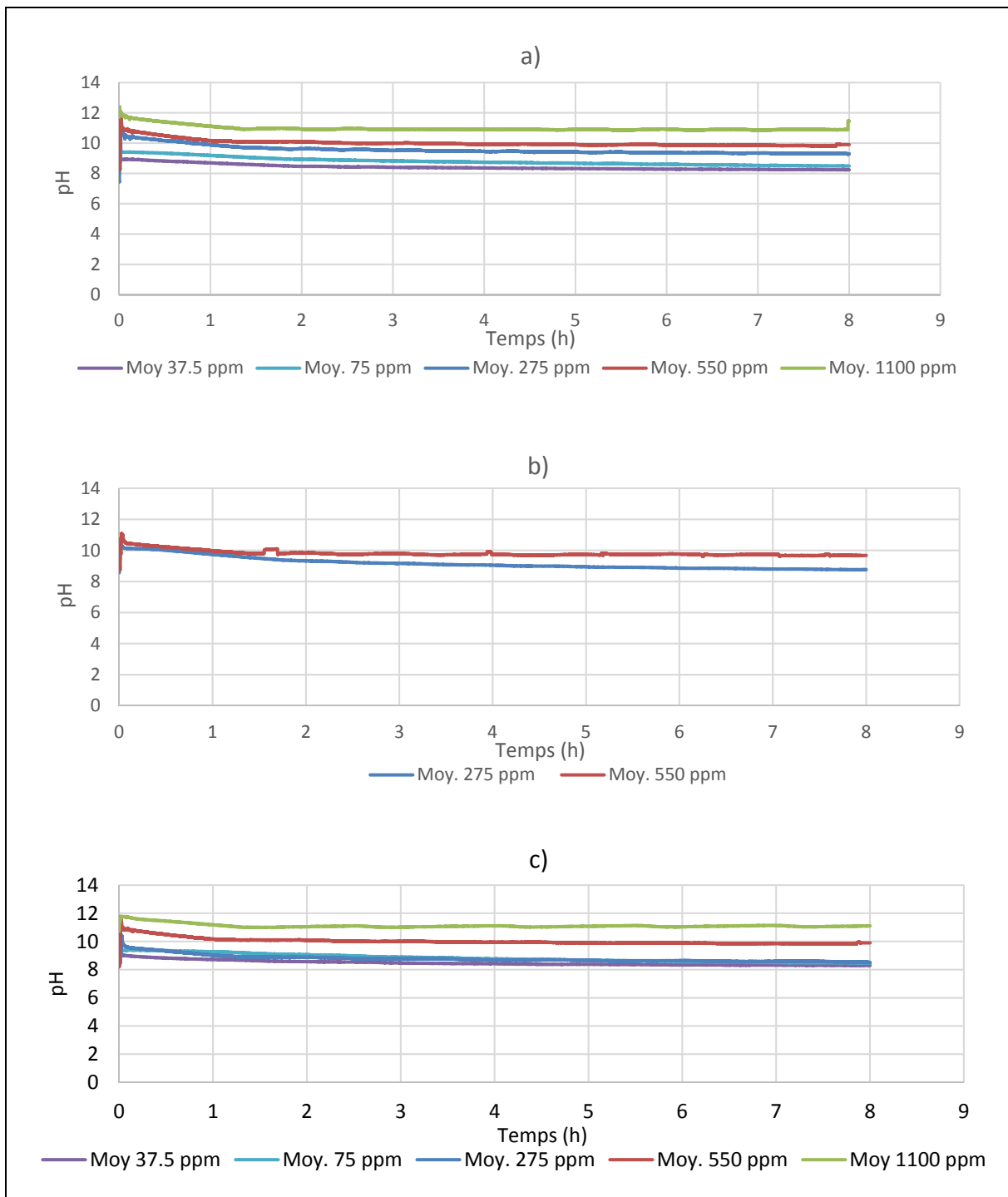
Figure 3.5 Variation du pH en fonction du temps pour différentes vitesses : a) 0,05 m/s, b) 0,91 m/s, c) 2,13 m/s
