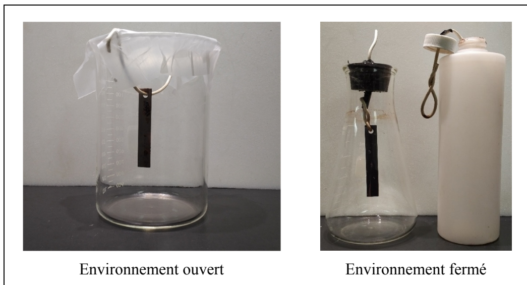
Figure 2.5 Montages expérimentaux pour les essais en laboratoire sur l'oxygène
