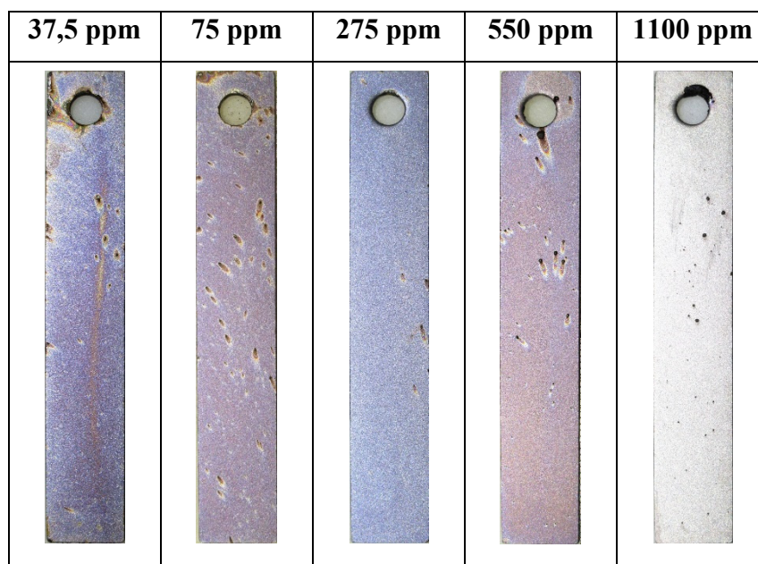
Figure 3.3 Coupons soumis à un environnement fermé en absence d'oxygène
