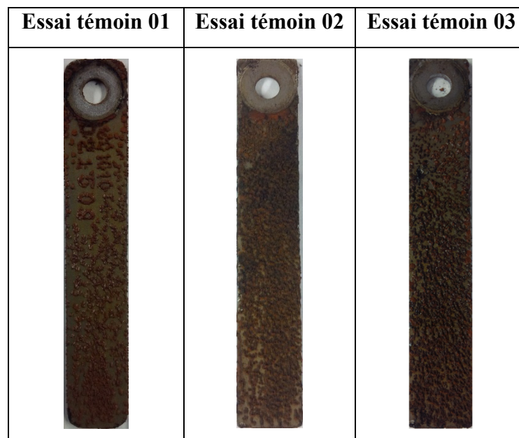
Figure 3.9 Aspect visuel des coupons en acier 1010 sans inhibiteur de corrosion
