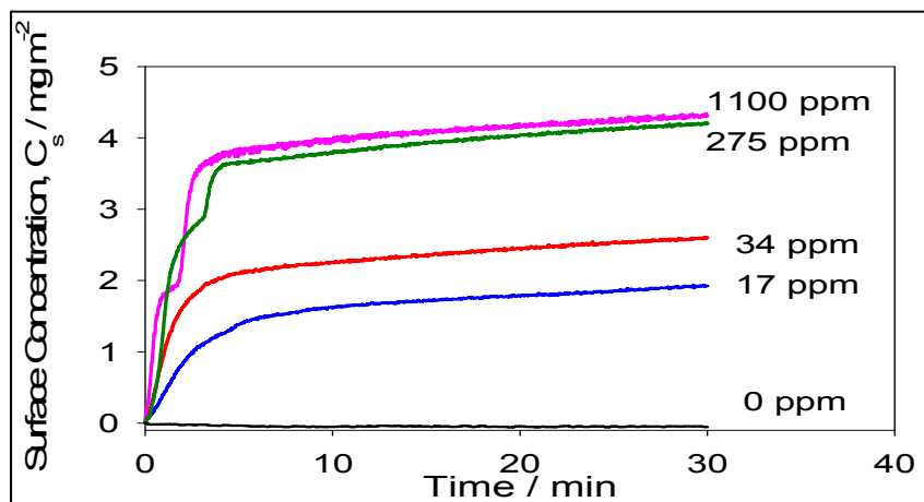
Figure 1.2 Concentration d'ingrédients actifs des tanins sur la surface d'acier doux en fonction du temps et de la concentration de tanins (Dargahi et al., 2015)
