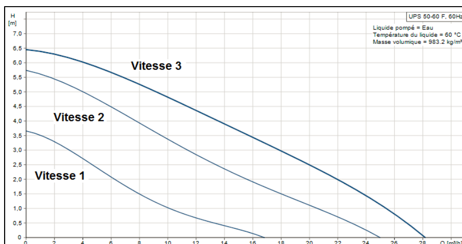
Figure 2.2 Courbe caractéristique pour chaque vitesse (1, 2 et 3) de la pompe Grundfos UPS 50-60F (Grundfos, 2014)
