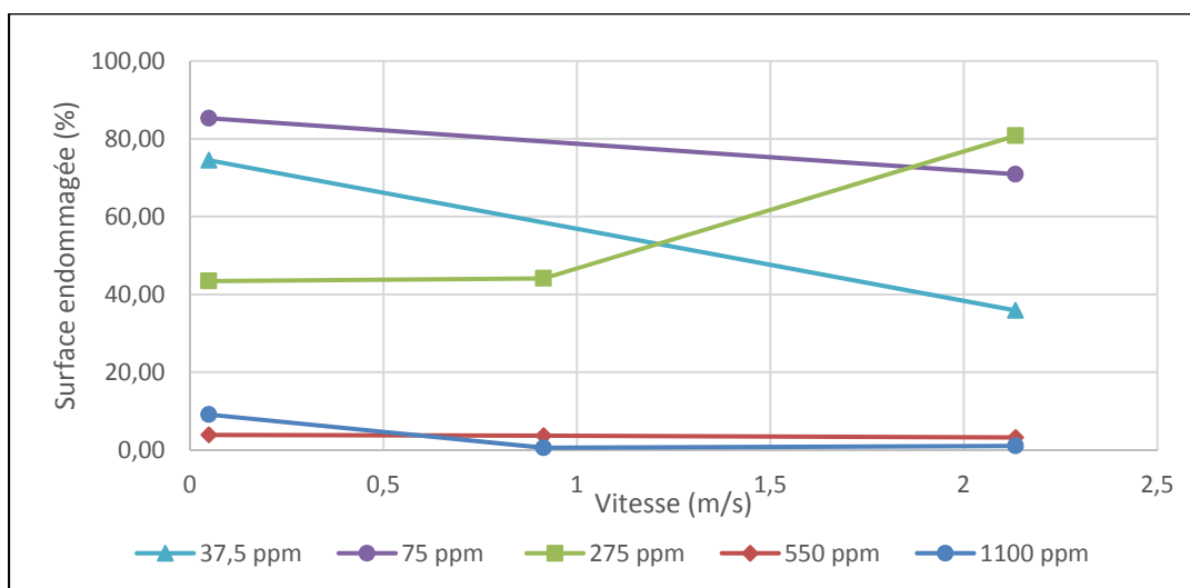
Figure 3.7 Variation de la surface relative endommagée des coupons en fonction de la vitesse d'écoulement pour un différentiel de tanins
