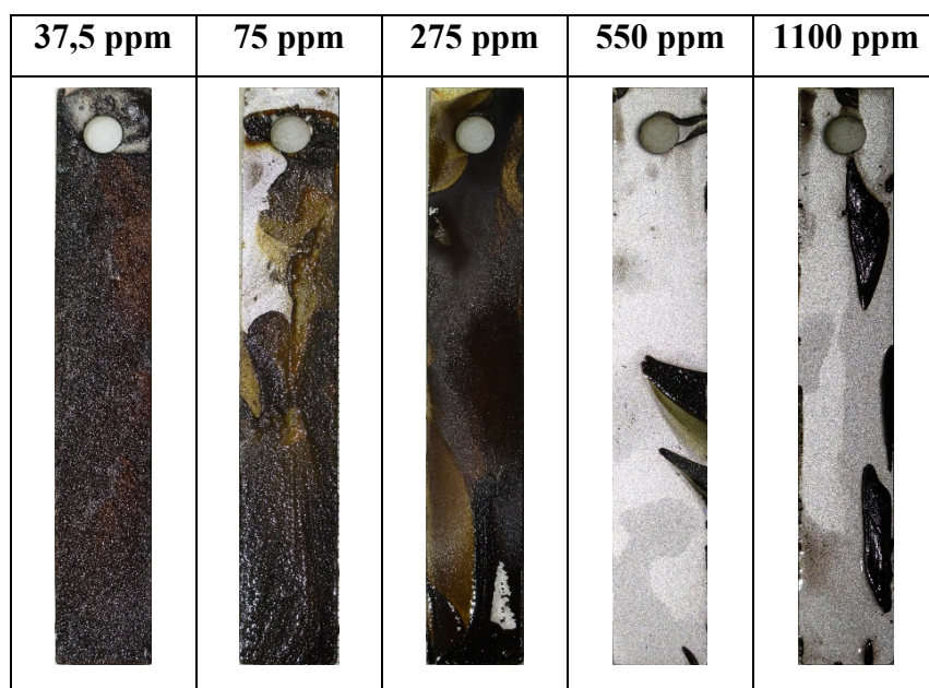
Figure 3.2 Coupons soumis à un environnement ouvert en présence d'oxygène
