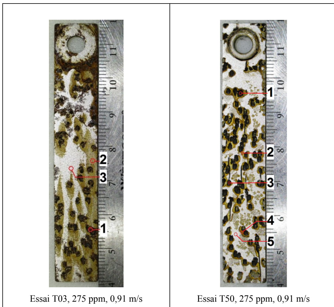
Figure 3.13 Coupons en acier doux Essais T03 et T50 analysés par diffraction rayon X
