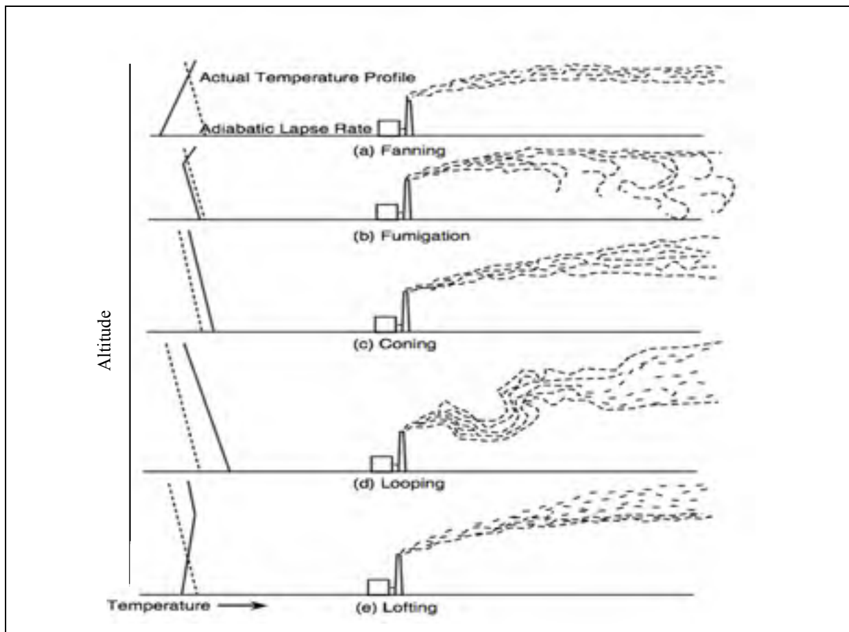
Figure 1.2 comportement d'un panache Adaptée d'Altwick (1999)
