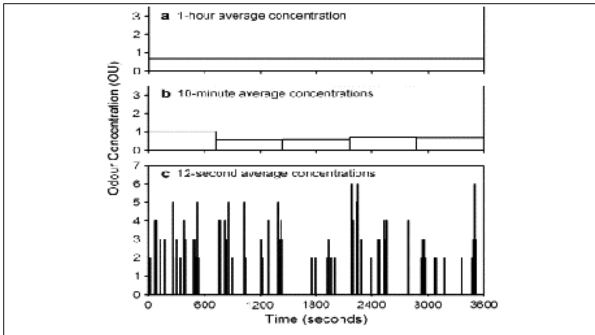
Figure 2.3 concentration des odeurs en fonction du temps Tirée de Nicell (2009)
