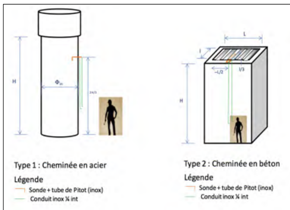
Figure 2.7 position des tubes de Pitot et des sondes sur les cheminées Tirée du dossier CRIQ n° 640-PE44099 (2013)
