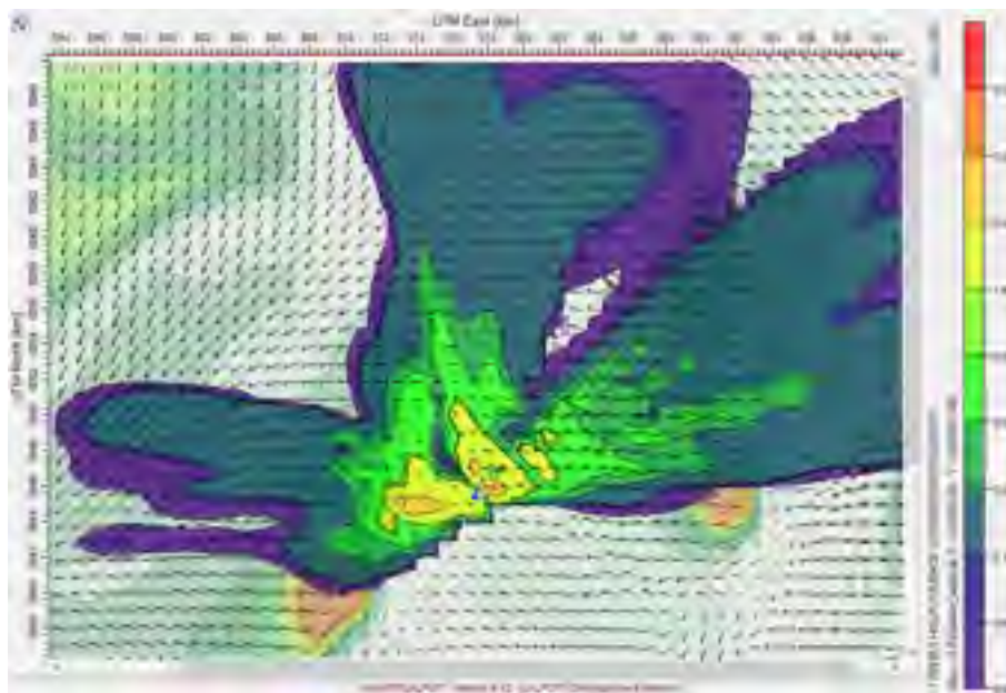
Figure-A I-5 concentration maximale odeur du scénario 10, banc d'essai 19
