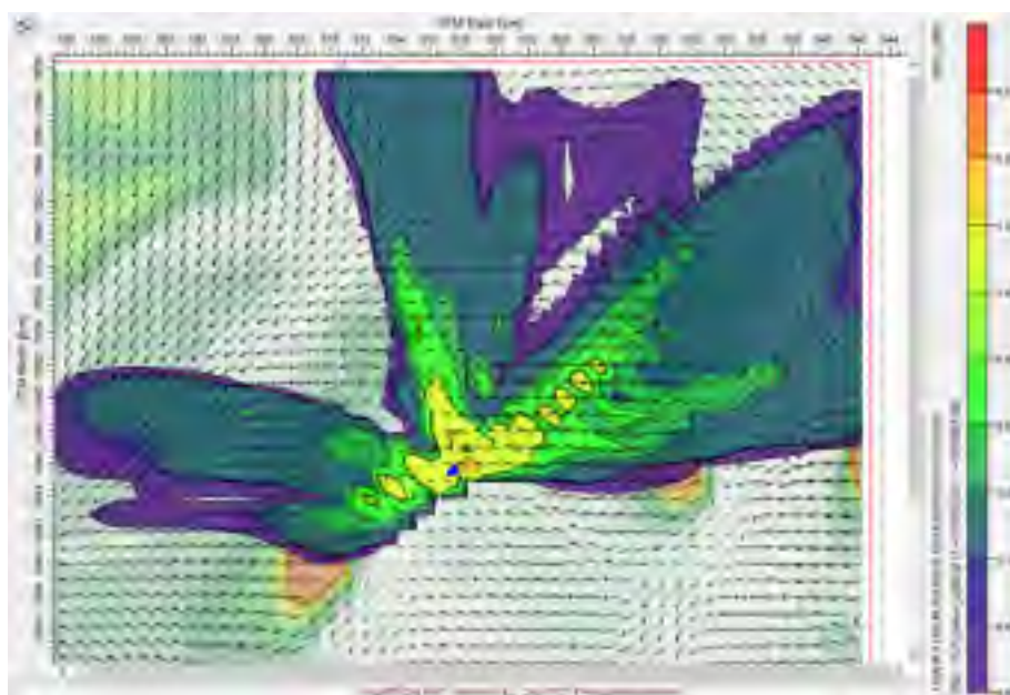
Figure-A I-4 concentration maximale odeur du scénario 4, banc d'essai 23
