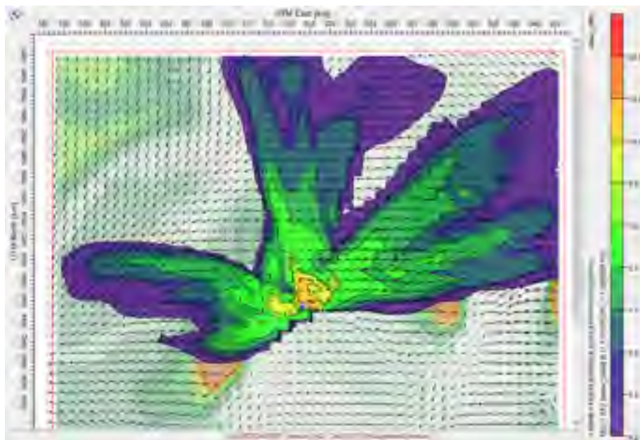
Figure-A II-2 concentration odeur maximale des scénarios 11 et 8
