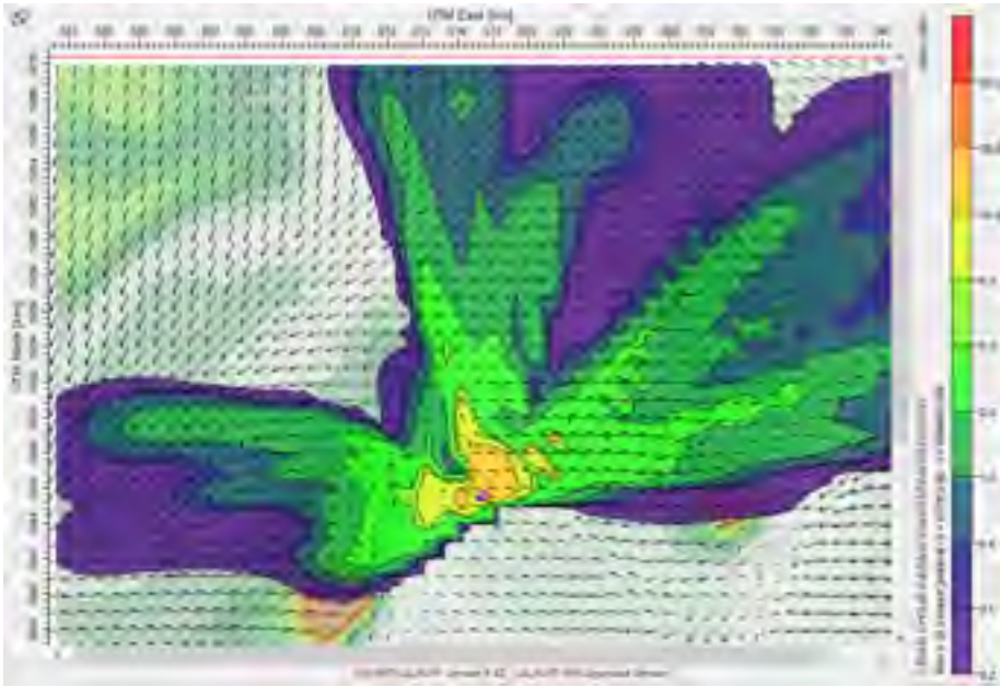
Figure-A II-7 concentration odeur maximale de 7 scénarios
