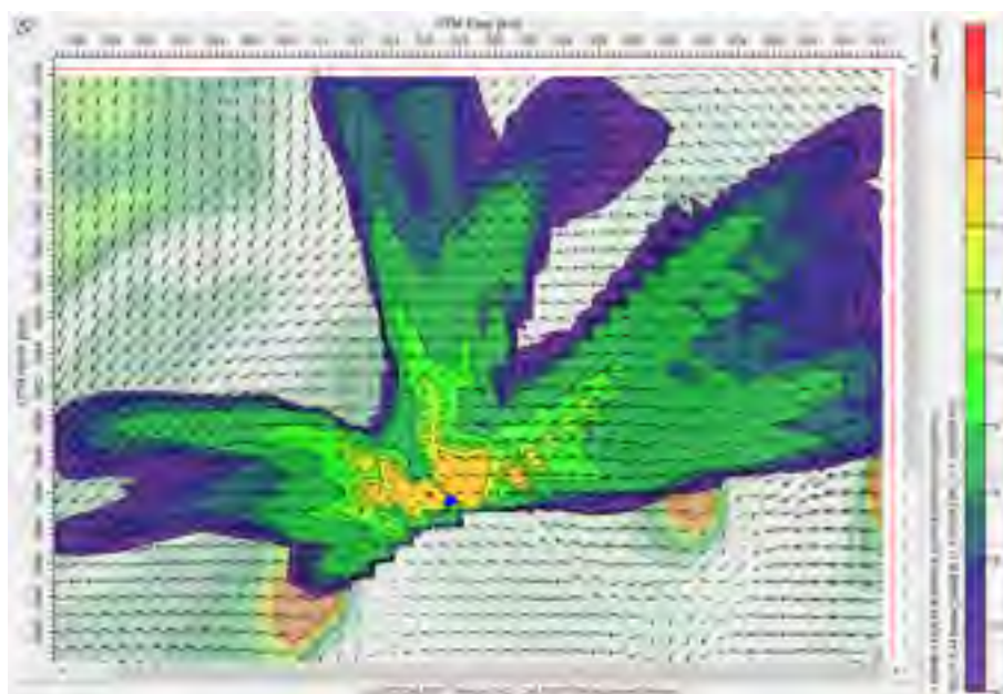
Figure-A I-6 concentration maximale odeur du scénario 5, banc d'essai 5
