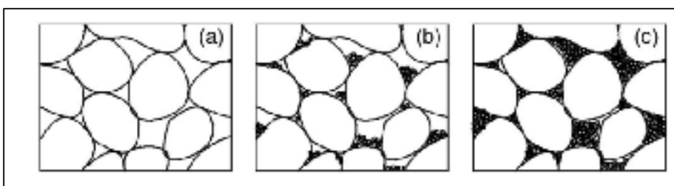
Figure 1.7 Distribution des particules fines dans une matrice de sol à grains grossiers
