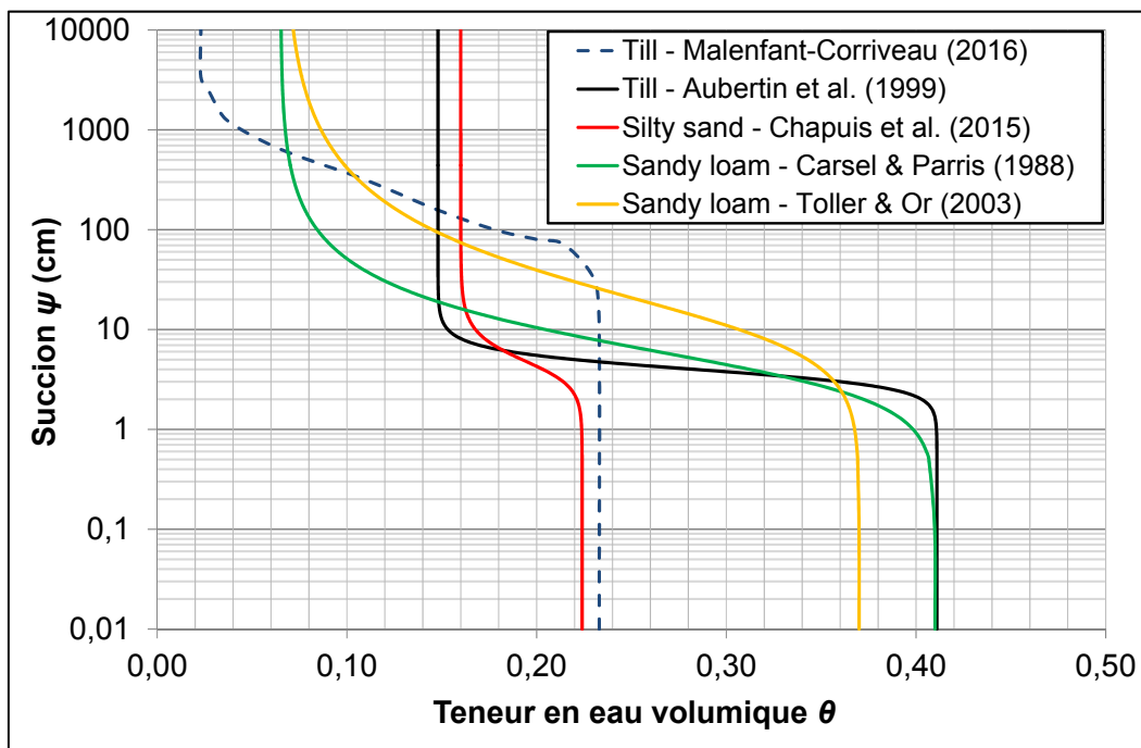
Figure 1.16 Exemples de courbes de rétention d'eau pour des matériaux s'apparentant au till du nord du Québec
