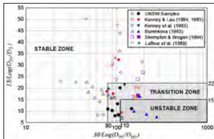
Figure 1.5 Potentiel de stabilité interne évalué par WF Tirée de Wan & Fell (2008)
