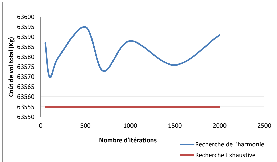
Figure 4.4 : Détermination du nombre d'itérations pour le vol à destination de Montréal- Honolulu (long-courrier)
