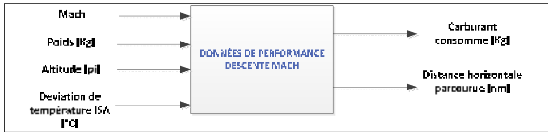
Figure 2.10: Données des entrées et des sorties de la phase de descente en Mach
