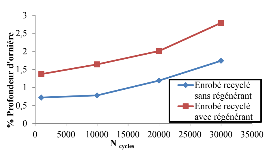
Figure 3.10 Variations du pourcentage de la profondeur d'orni re en fonction du nombre des cycles l'enrob  recycl    froid avec et sans r g n rant   40  C
