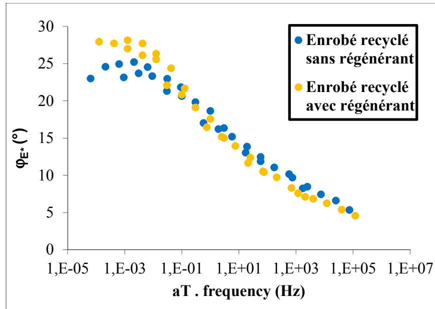
Figure 3.7 Courbe maîtresse de \phi_E des deux enrobés recyclés traités à froid à l'aide d'une émulsion de bitume avec et sans ajout d'un régénérant ( T_{ref} = 5\text{ °C} )
