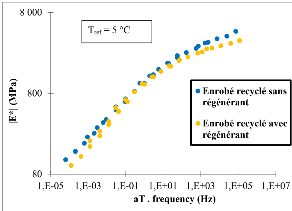
Figure 3.6 Courbe maîtresse de la norme du module complexe d'enrobé recyclé traité à froid à l'aide d'une émulsion de bitume et celui incorporant un régénérant ( T_{\text{ref}}=5\text{ °C} )
