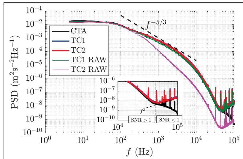
Figure 2.8 PSD de fluctuations de vitesse à y^+ = 114 .
