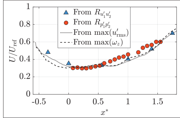
Figure 4.38 Vitesse de convection moyenne normalisée U_c/U_{\text{ref}} .
