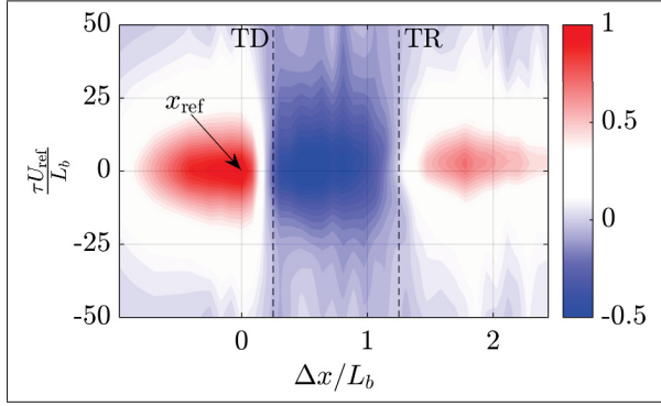
Figure 4.28 Cartographie de R_{p'_1 p'_2} pour la composante LF, x_{\text{ref}}^* = -0.25 .
