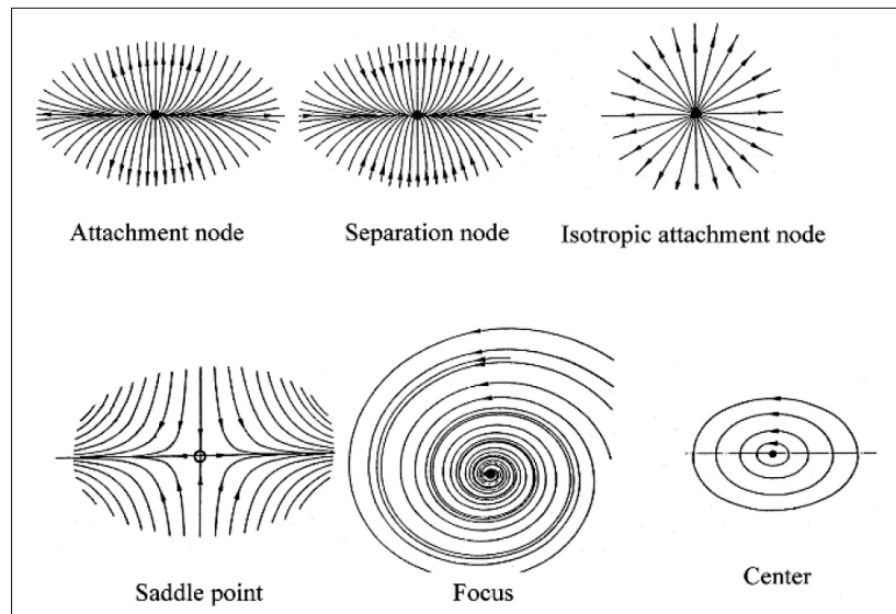
Figure 1.6 Les principaux points critiques pour la description topologique des écoulement 3D. Tirée de Délerly (2013).
