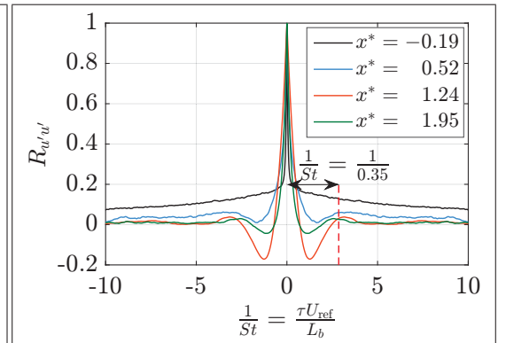
Figure 4.9 R_{u'u'} à quatre positions x^* de la figure 4.8.
