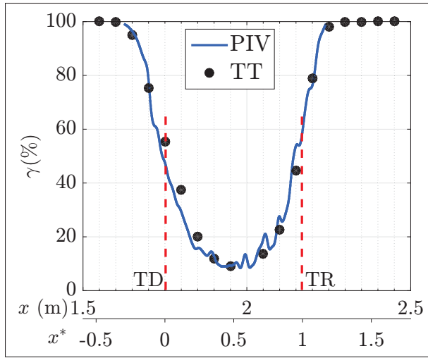
Figure 3.8 L'intermittence à y = 1 mm sur la ligne z = 0 .
