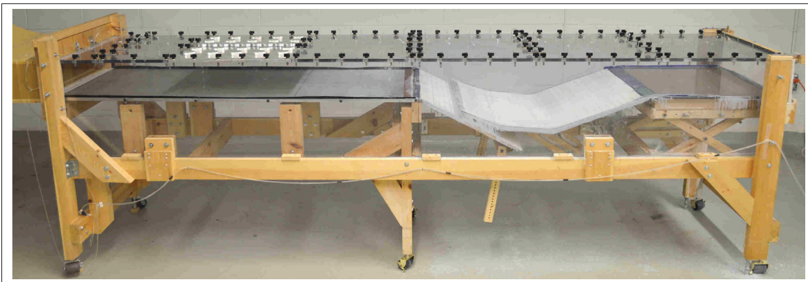
Figure 2.2 Photographie de la section d'essai.
