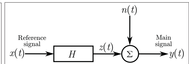
Figure 2.21 Schéma bloc du filtre soustracteur de cohérence, tirée de Bendat et Piersol (2010).
