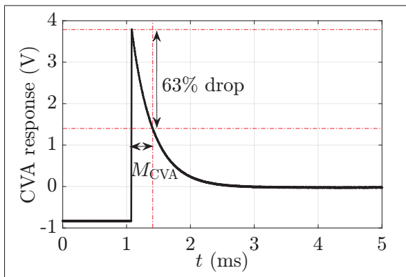
Figure 2.5 Réponse d'un fil chaud à un signal carré en fonctionnement CVA.
