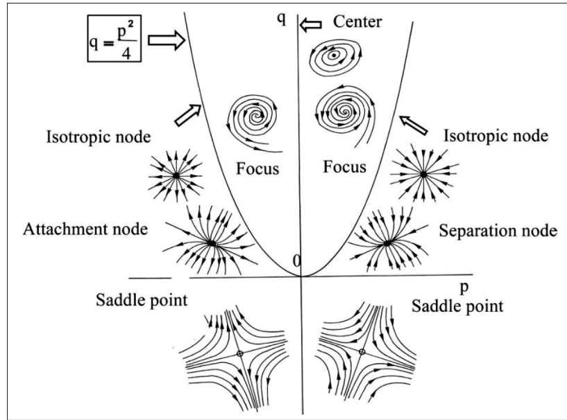
Figure 1.5 Classification des points critiques. Tirée de Délerly (2013).
