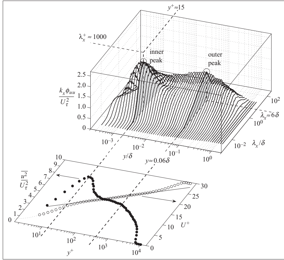
Figure 1.3 Spectrogram de fluctuations de vitesse longitudinale à Re_\tau = 7200 . Tirée de Hutchins et Marusic (2007b).
